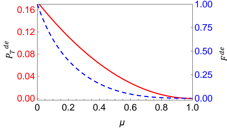
Hình 2.3: Tổng xác suất thành công P_T^{de} (đường liền nét) và độ tin cậy F^{de} (đường đứt nét) cho bởi các công thức (2.51) và (2.52) tương ứng là hàm của cường độ suy giảm liên kết \mu định nghĩa trong (2.53). Ở đây, chúng tôi chọn biên độ đầu vào \beta = 1.2 tương ứng với hệ số phản xạ tối ưu r^{\text{peak}} \approx 0.347 .
