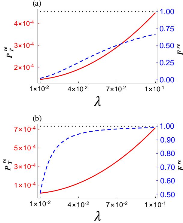
Hình 2.4: Tổng xác suất thành công P_T^{re} (đường liền nét) và độ tin cậy F^{re} (đường đứt nét) phụ thuộc vào cường độ SPDC loại II \lambda khi sử dụng (a) trạng thái nén chân không trong (2.54) với s = -0.43358 như một sự gần đúng của trạng thái con mèo Schrödinger chắn biên độ 0.7 và (b) trạng thái nén một photon trong (2.55) với s = 0.16056 như một sự gần đúng của trạng thái con mèo Schrödinger lẻ biên độ 0.7. Trong cả hai trường hợp, đường gạch ngang thể hiện độ tin cậy là tuyệt đối (nghĩa là khi trạng thái đầu vào là hoàn hảo) và hệ số phản xạ r được chọn là 0.1.
