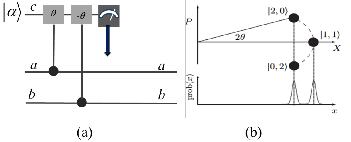
Hình 1.5: (a) Sơ đồ phép đo homodyne để phân biệt trạng thái cân bằng và trạng thái chùng. (b) Sơ đồ minh họa không gian pha của trạng thái |\psi_1\rangle trong công thức (1.45).
