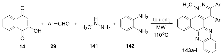
Bảng 3.11. Các hợp chất 143a-i
