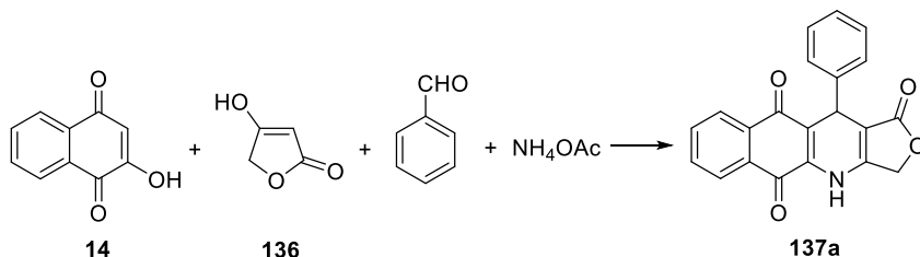
Sơ đồ 3.4. Tổng hợp hợp chất 137a
