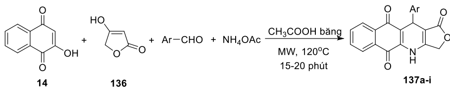
Bảng 3.4. Các hợp chất 137a-i
