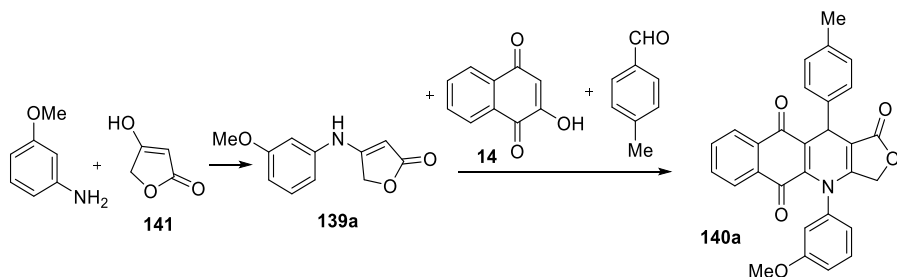
Sơ đồ 3.9. Tổng hợp hợp chất 140a
