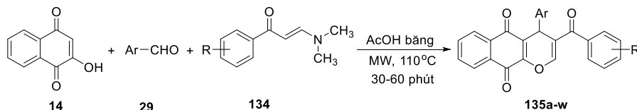
Bảng 3.2. Các hợp chất 135a-w
