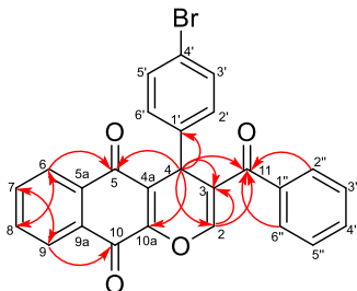
Bảng 3.3. Dữ liệu phổ NMR của hợp chất 135d
