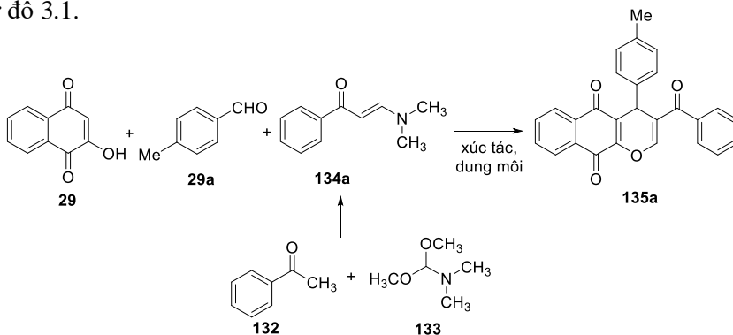
Sơ đồ 3.1. Tổng hợp hợp chất 135a
