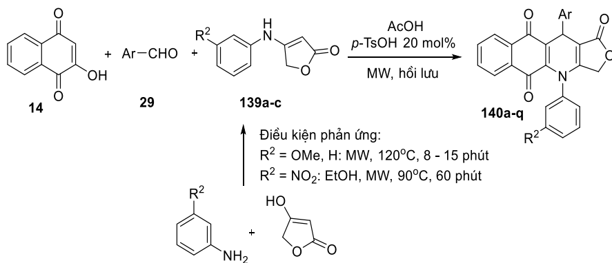
Sơ đồ 3.10. Tổng hợp hợp chất 140a-q
