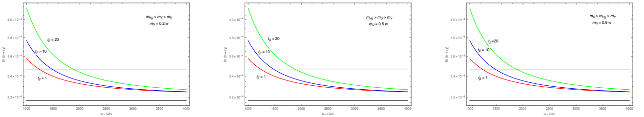
Hình 3.5: Sự phụ thuộc của tỉ lệ rẽ nhánh \text{Br}(b \rightarrow s\gamma) vào thang vật lý mới w trong giới hạn u, v \ll -f \sim w \sim \Lambda .
