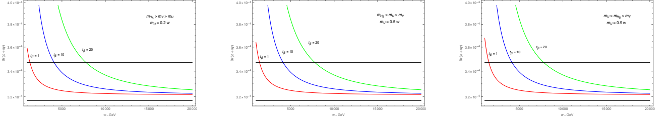
Hình 3.4: Sự phụ thuộc của \text{Br}(b \rightarrow s\gamma) vào thang vật lý mới w trong giới hạn, u, v \ll -f \frac{u^2+v^2}{uv} \sim w \sim \Lambda . Đường màu đen đậm thể hiện ràng buộc thực nghiệm hiện tại tại \text{Br}(b \rightarrow s\gamma) = (3.32 \pm 0.15) \times 10^{-4}
