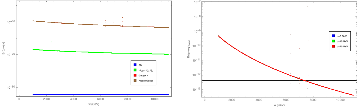
Hình 3.6: Kết quả khảo sát số tỷ lệ rã nhánh \text{Br}(\mu \rightarrow e\gamma) vào thang w . Đường đậm màu đen thể hiện giới hạn trên thực nghiệm
