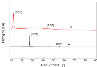
Hình 3.3. Giải đồ nhiễu xạ tia X của graphite (a) và GO (b)
