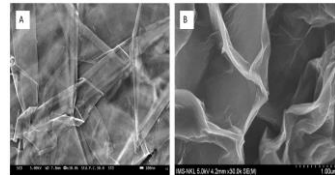
Hình 3.4. Ảnh FE-SEM của graphite (A) và GO (B)
