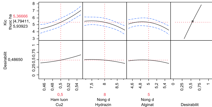
Hình 3.10. Biểu đồ dự đoán sự thay đổi kích thước hạt nano \text{Cu}_2\text{O-Cu} theo sự biến đổi của các yếu tố khảo sát
