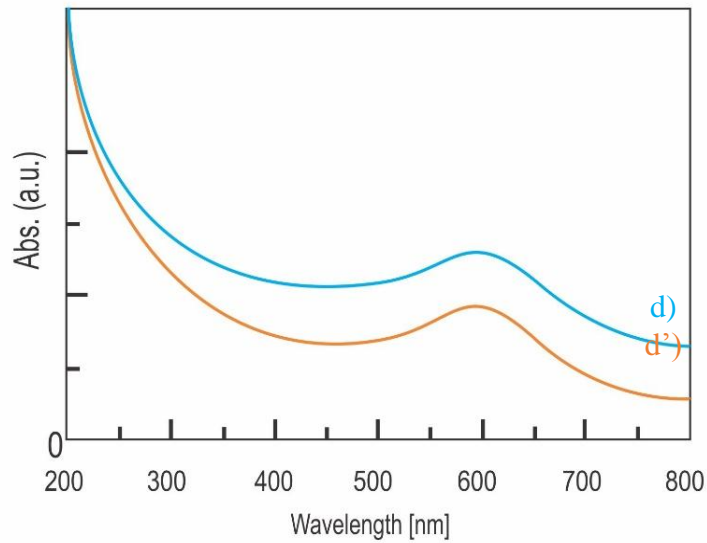
Hình 3.14. Phổ UV-vis của nano \text{Cu}_2\text{O-Cu/alginate} 80 mM Cu ban đầu (d) và nano \text{Cu}_2\text{O-Cu/alginate} 80 mM Cu tinh chế bằng phương pháp kết tủa trong \text{C}_2\text{H}_5\text{OH} (d')
