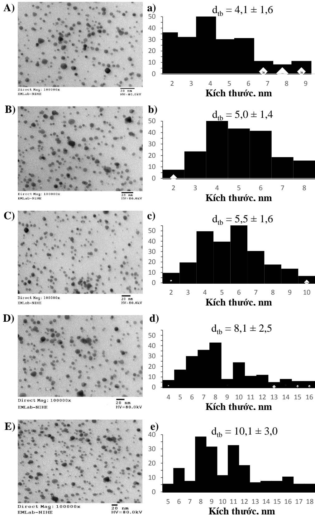
Hình 3.3. Ảnh TEM (A,B,C,D,E) và phân bố kích thước hạt (a,b,c,d,e) của nano \text{Cu}_2\text{O-Cu} phụ thuộc vào nồng độ \text{Cu}^{2+} : 60 mM (A,a), 70 mM (B,b), 80 mM (C,c), 90 mM (D,d) và 100 mM (E,e)
