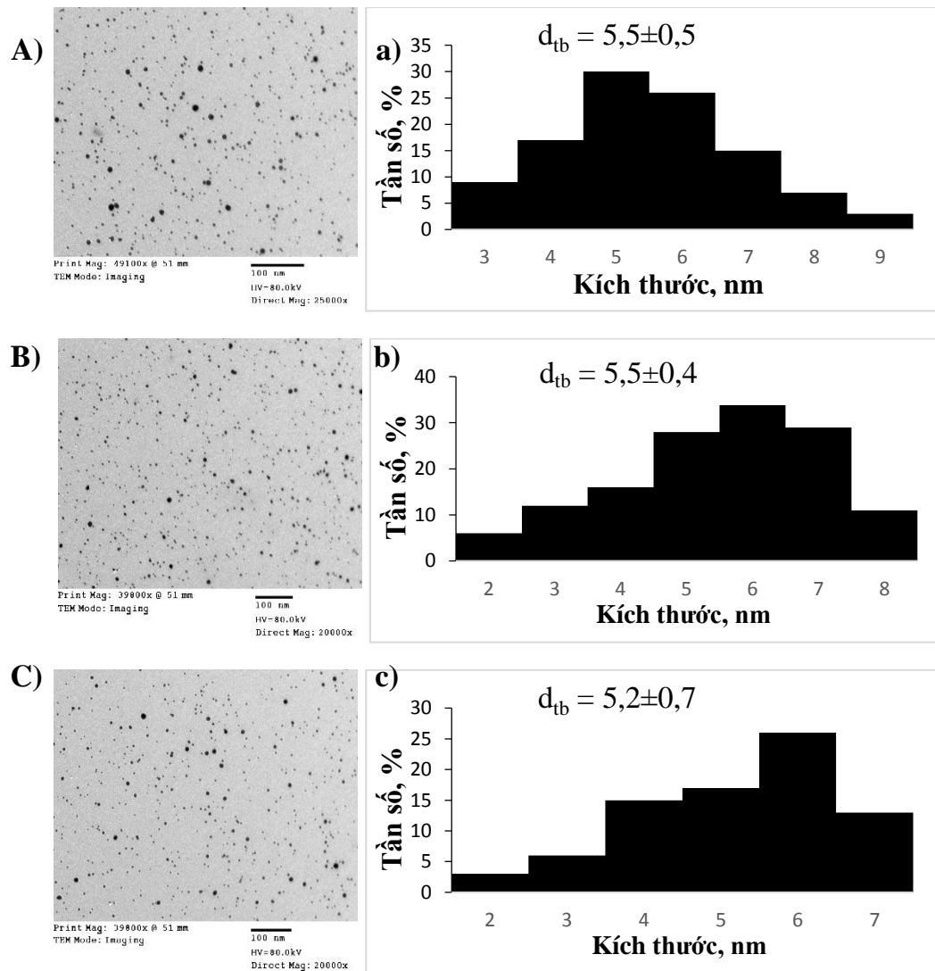
Hình 3.12. Ảnh TEM (A,B,C) và phân bố kích thước hạt (a,b,c) của nano \text{Cu}_2\text{O-Cu} nồng độ 80 mM Cu, \text{N}_2\text{H}_4 7,8% và alginate 5% (A,a; B,b; C,c ký hiệu các lần lặp lại)
