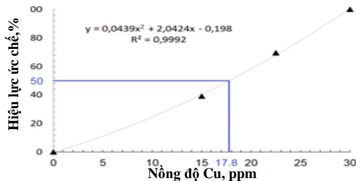
Hình 3.25. Hiệu lực ức chế nấm Pyricularia oryzae của nano \text{Cu}_2\text{O-Cu/alginate} sau 7 ngày
