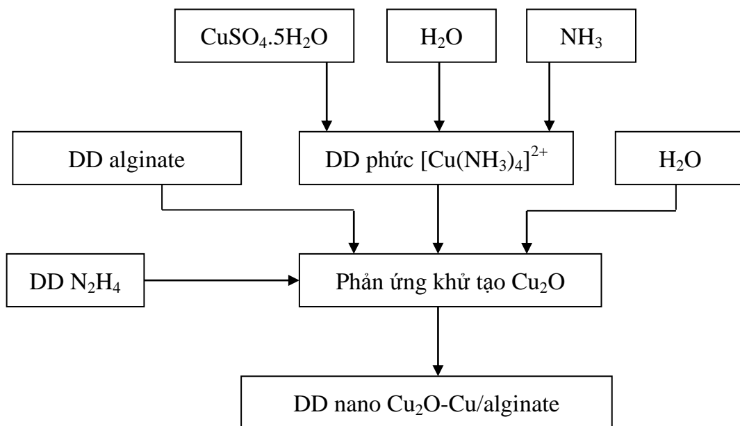
Hình 2.1. Quy trình điều chế vật liệu nano Cu 2 O-Cu/alginate
