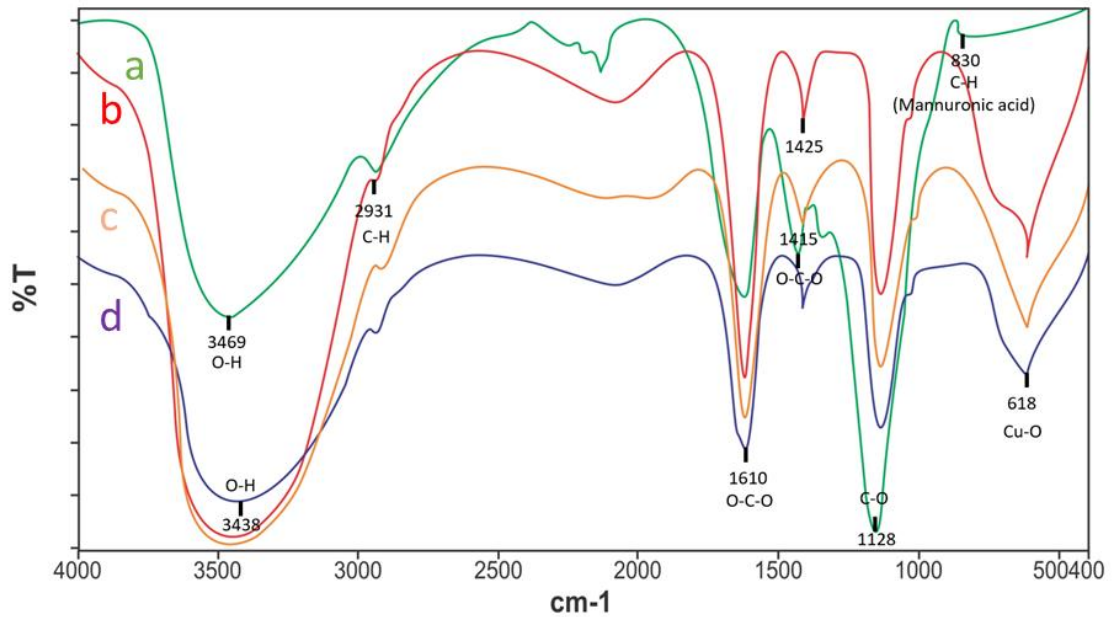
Hình 3.16. Phổ FT-IR của alginate chiết suất từ rong nâu (a) và nano Cu 2 O-Cu/alginate có 60 mM Cu (b); 80 mM Cu, (c); 100 mM Cu (d)
