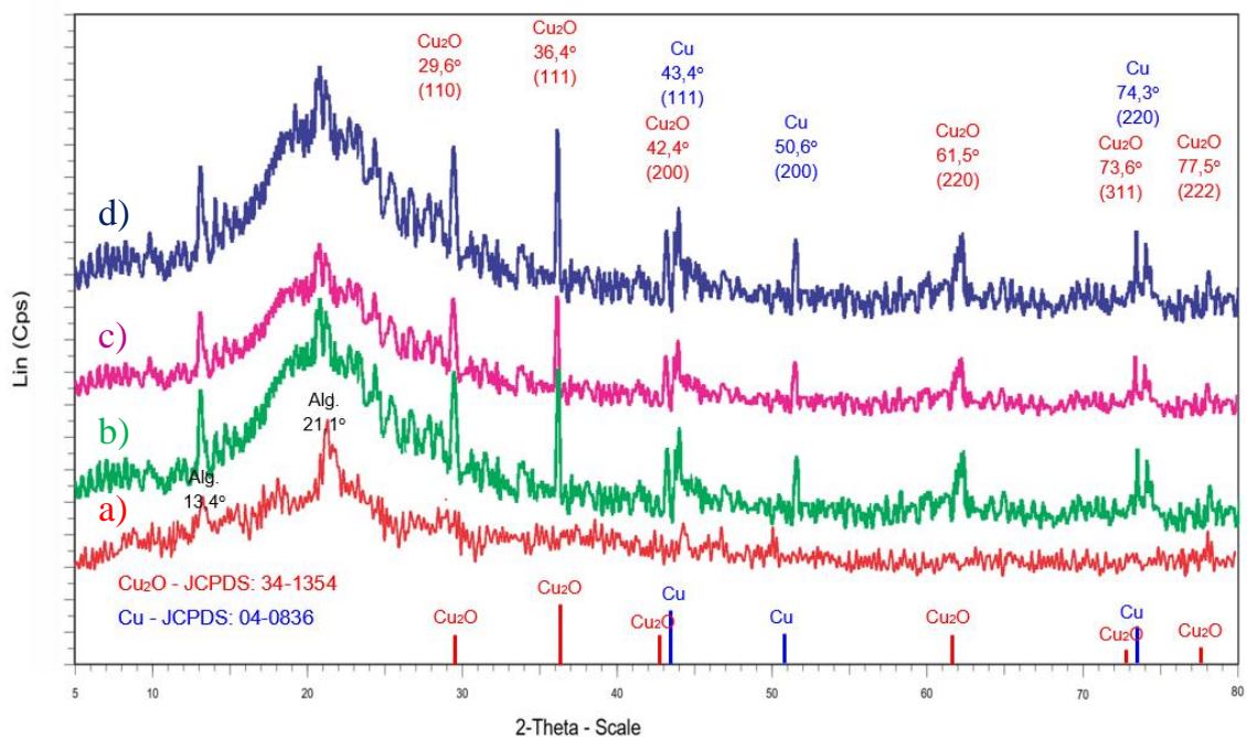
Hình 3.15. Giản đồ XRD của natri alginate (a) và nano \text{Cu}_2\text{O} -Cu/alginate với nồng độ Cu 60 mM (b), 80 mM (c), 100 mM (d)
