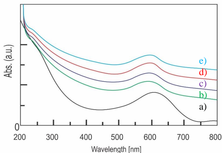
Hình 3.13. Phổ UV-vis của phức Cu[(NH 3 ) 4 ] 2+ /alginate (a), nano Cu 2 O-Cu/alginate 60 mM Cu (b), nano Cu 2 O-Cu/alginate 70 mM Cu (c), nano Cu 2 O-Cu/alginate 80 mM Cu (d), nano Cu 2 O-Cu/alginate 100 mM Cu (e)
