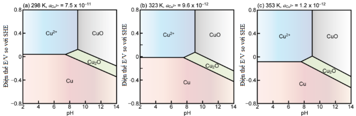
Hình 1.7: Biểu đồ điện thế - pH ở các hoạt động cân bằng của ion \text{Cu}^{2+} ở pH 9, nhiệt độ (a) 298, (b) 323, và (c) 353 K và dạng tồn tại của \text{Cu}^{2+} , \text{CuO} , \text{Cu}_2\text{O} , \text{Cu} [185]
