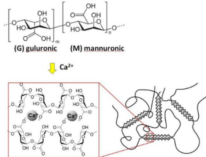
Hình 1.6: Mô hình tạo gel của alginate với ion hóa trị [180]
