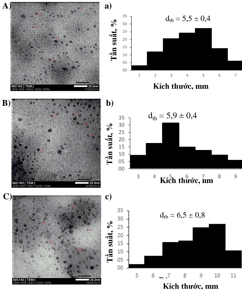
Hình 3.5. Ảnh TEM (A, B, C) và phân bố kích thước hạt (a, b, c) của nano Cu_2O-Cu phụ thuộc vào nồng độ chất khử hydrazine 8% (A, a), 12% (B, b) và 16% (C, c).
