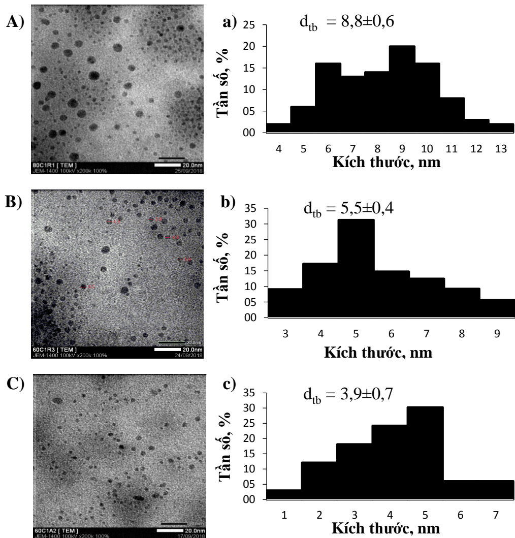
Hình 3.6. Ảnh TEM (A,B,C) và phân bố kích thước hạt (a,b,c) của nano Cu 2 O-Cu phụ thuộc vào nồng độ chất ổn định alginate 4% (A,a), 5% (B,b) và 6% (C,c)
