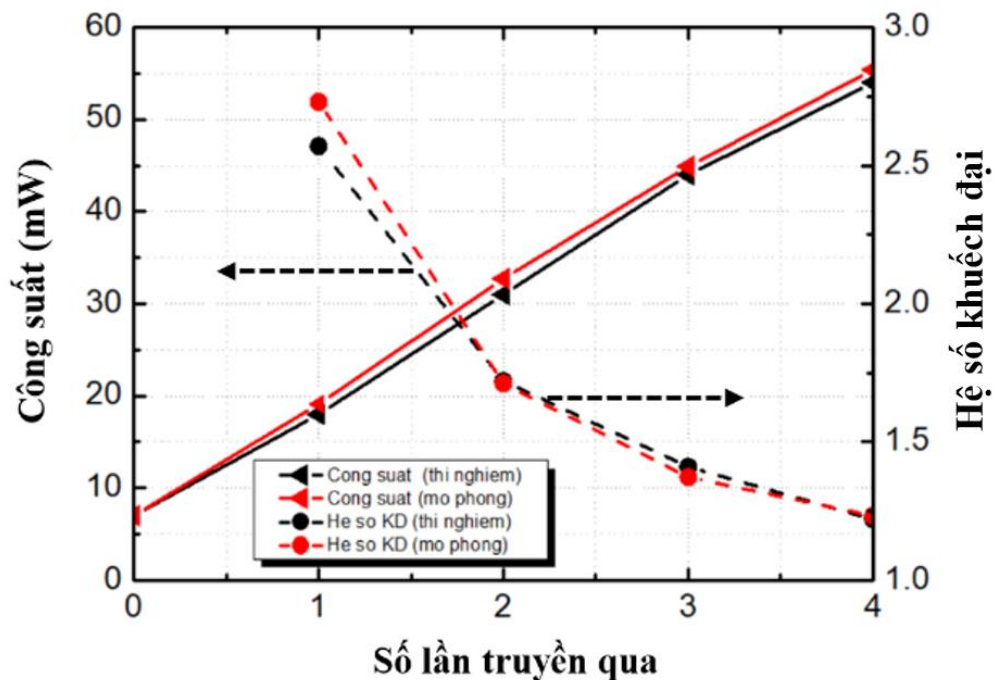
Hình 3.7. Kết quả mô phỏng và thực nghiệm khuếch đại các xung laser băng rộng.
