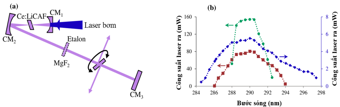
Hình 1.15. a) Hệ laser Ce:LiCAF điều chỉnh bước sóng sử dụng tấm etalon.
