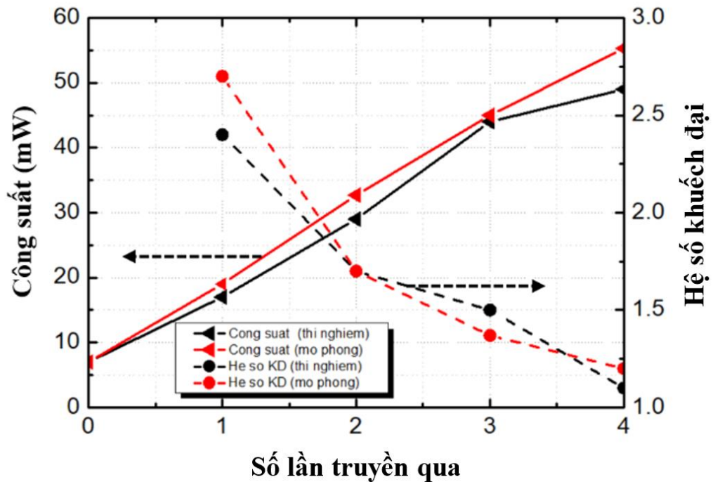
Hình 3.22. Kết quả mô phỏng và thực nghiệm khuếch đại các xung laser băng hẹp.
