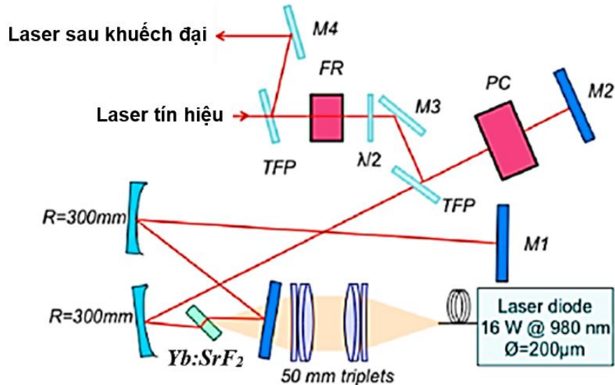
Hình 1.8. Sơ đồ hệ khuếch đại tái phát Yb:SrF_2 [46].
