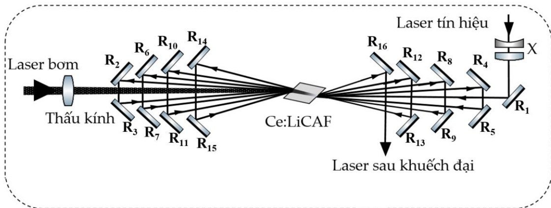
Hình 2.1. Cấu hình hệ khuếch đại các xung laser UV nhiều lần truyền qua sử dụng tinh thể Ce:LiCAF.
