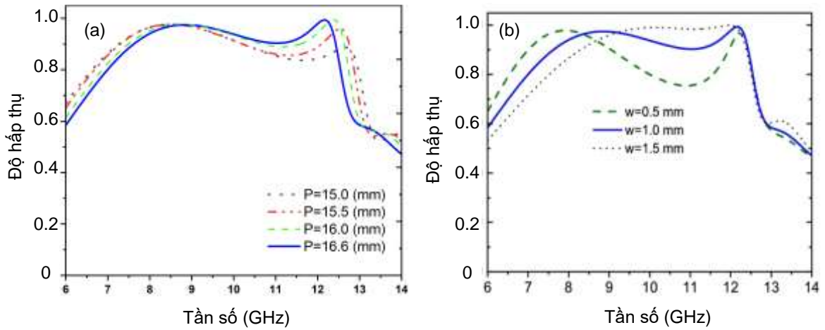
Hình 3.16. Độ hấp thụ của BMPA các giá trị khác nhau của (a) P và (b) w .
