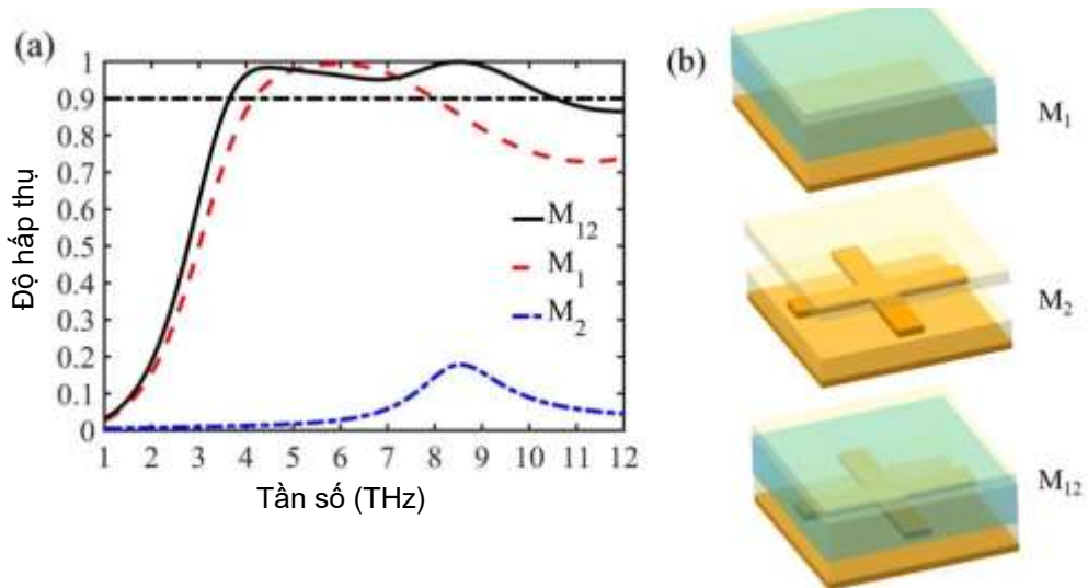
Hình 1.46. Độ hấp thụ BMPA với các cách ghép tầng khác nhau [72].
