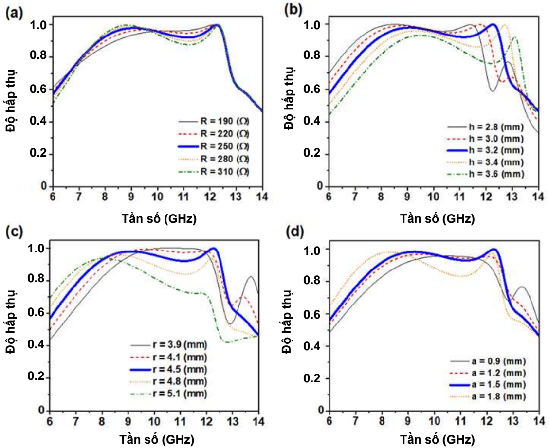
Hình 3.15. Phổ hấp thụ của BPA đề xuất cho các giá trị khác (a) giá trị phần tử điện trở R , và các thông số cấu trúc khác (b) h , (c) r , (d) a , cho phân cực TE với góc tới vuông góc [109].
