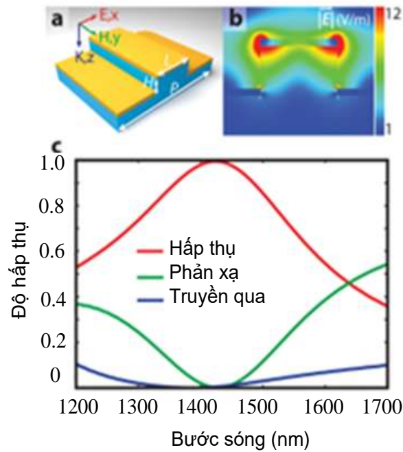
Hình 1.55. (a) Cấu trúc hình học của ô cơ sở với các cộng hưởng (Au) tích hợp với bán dẫn (màu xanh), (b) phân bố trường điện của MPA với phân cực TM, (c) hệ số phản xạ, truyền qua và hấp thụ của MPA [92].
