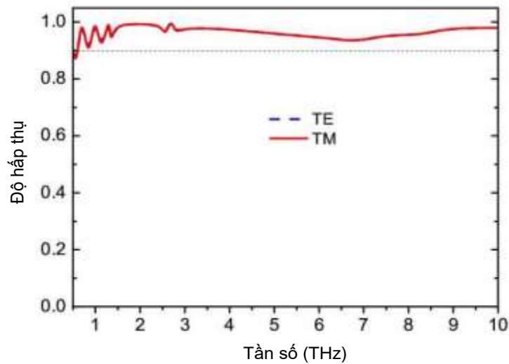
Hình 4.16. Độ hấp thụ của BMPA đề xuất với góc tới vuông góc cho phân cực TE và TM [134].
