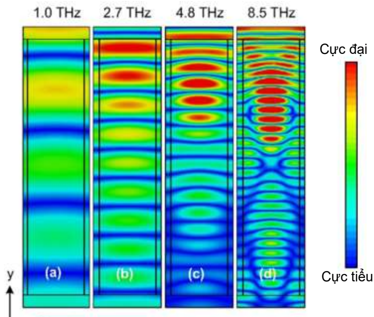
Hình 4.22. [Từ trái qua phải] Phân bố từ trường của BMPA tại các tần số khác nhau (a) 1.0 THz, (b) 2.7 THz, (c), 4.8 THz and (d) 8.5 THz [134]
