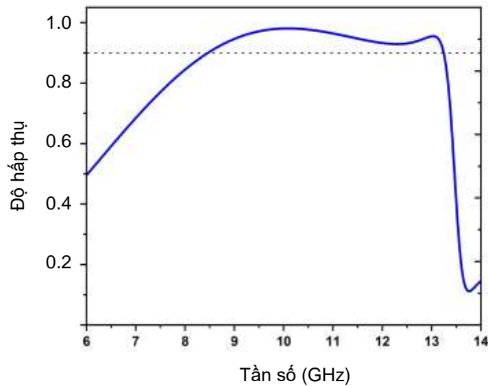
Hình 3.17. Độ hấp thụ của BMPA với vật liệu điện môi polyimide.
