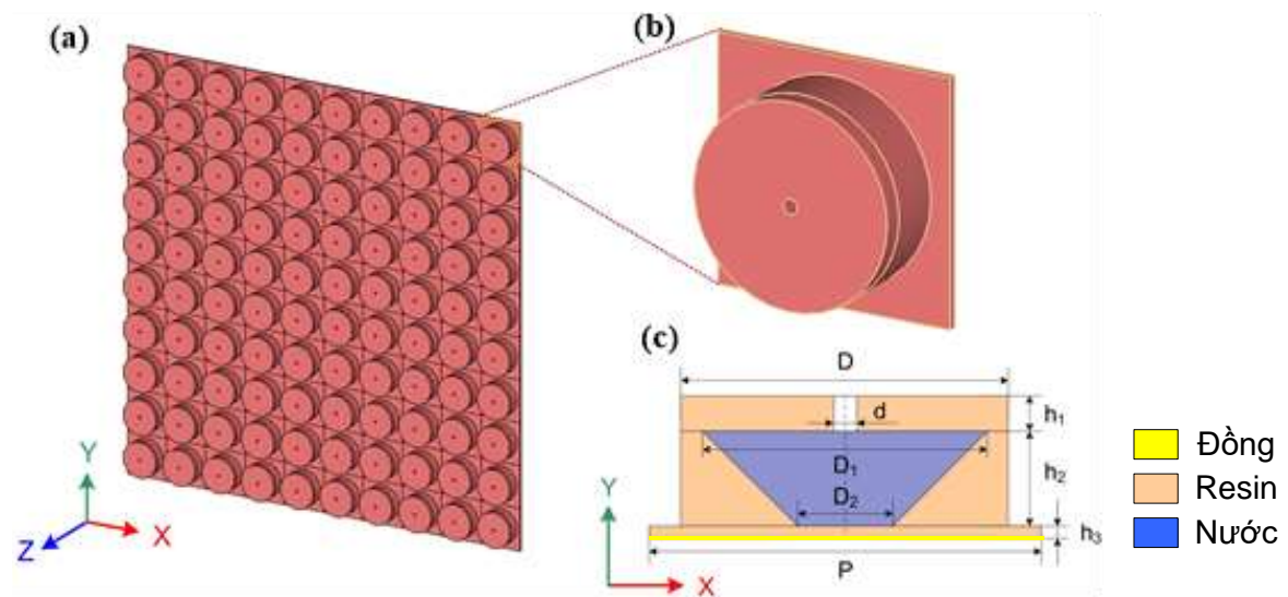
Hình 4.2. Cấu trúc của BMPA tích hợp nước hoạt động ở vùng tần số GHz.
