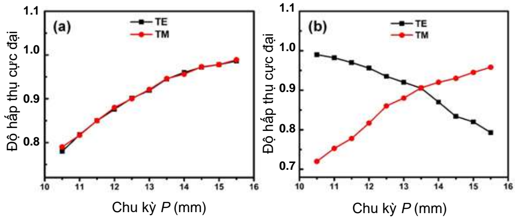
Hình 1.9. Ảnh hưởng của thông số P tới độ hấp thụ của MPA hình bông hoa 8 cánh với trường hợp góc tới (a) 0^\circ và (b) 70^\circ [38].
