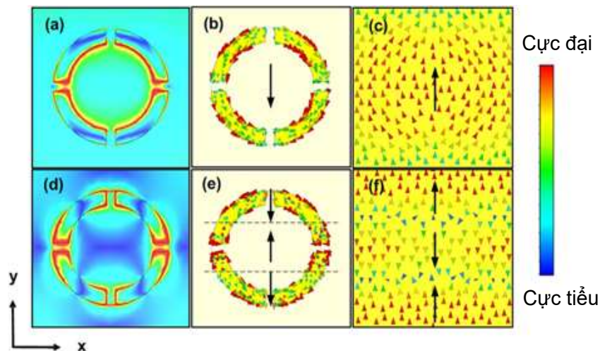
Hình 3.23. [Từ trái sang phải] Phân bố điện trường, dòng điện cảm ứng ở mặt trên và mặt dưới của BMPA tại các tần số cộng hưởng: (a)-(c) 9.1 GHz và (d)-(f) 12.2 GHz [109].
