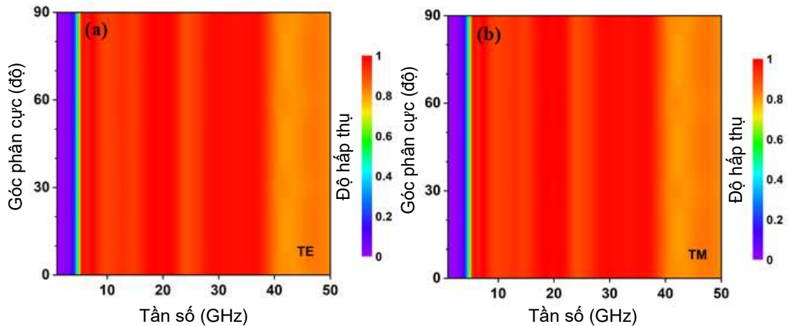
Hình 4.12. Phổ hấp thụ của BMPA khi thay đổi góc phân cực.
