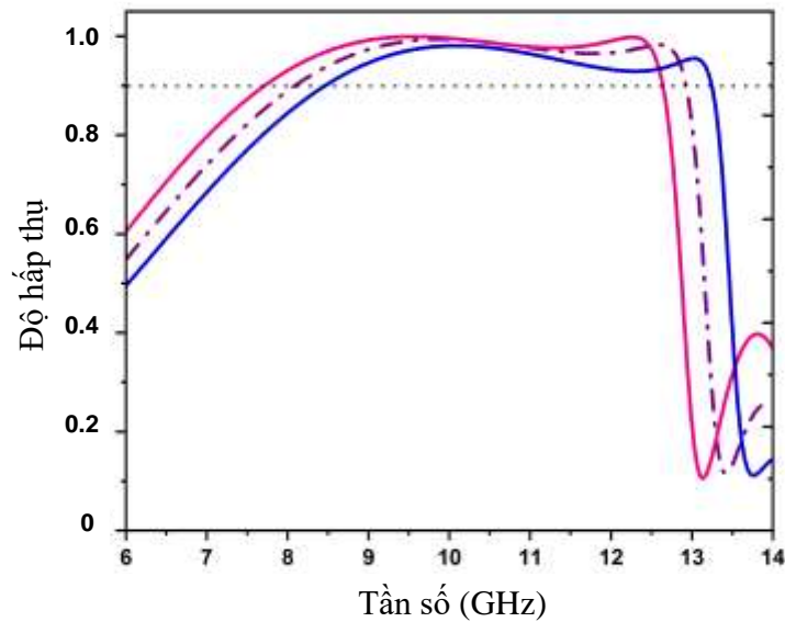
Hình 3.18. Độ hấp thụ của BMPA với độ dày khác nhau của lớp polyimide.
