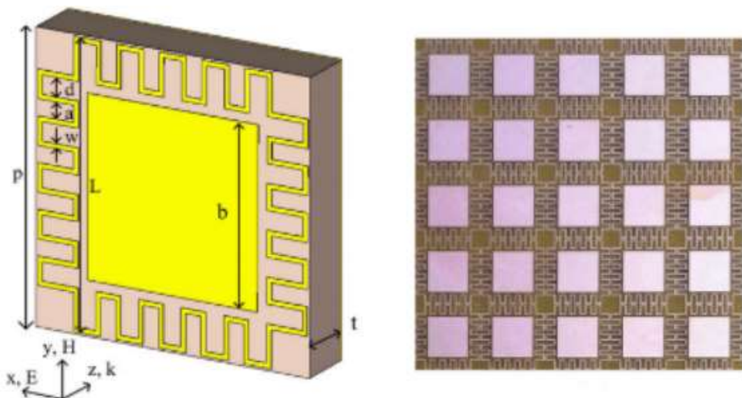
Hình 1.19. Ví dụ về MPA với cấu trúc dạng zig-zag làm tăng độ tự cảm [45].
