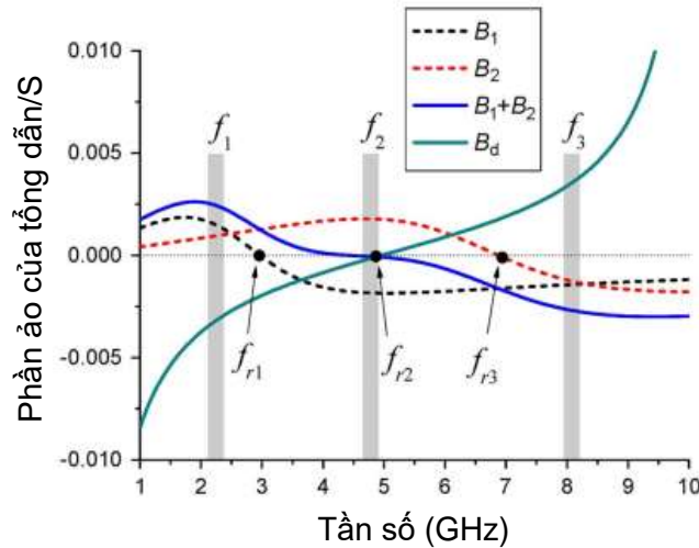
Hình 2.6. Đường cong phản ảo của tổng dẫn theo tần số [102]
