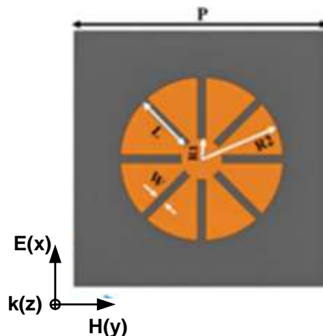
Hình 1.24. Cấu trúc hấp thụ với 8 sectors [51].
