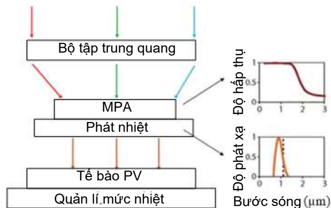
Hình 1.50. Sơ đồ hệ thống STPV với BMPA, bộ hấp thụ và bộ phát xạ điện hình hoạt động trên 1000 K trong khi tế bào PV hoạt động tại nhiệt độ phòng [12].
