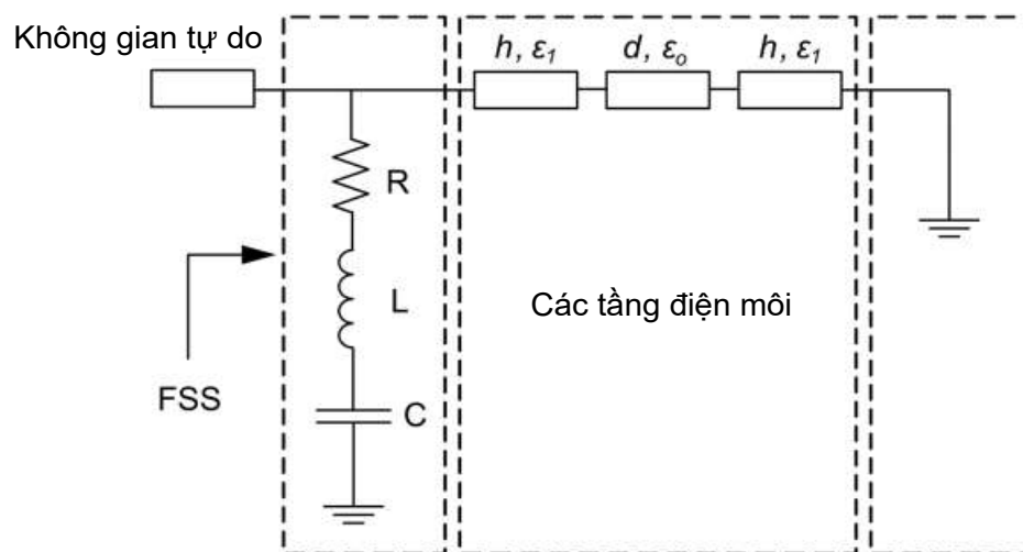
Hình 3.35. Mô hình mạch cho thiết kế BMPA với nhiều lớp điện môi [118].
