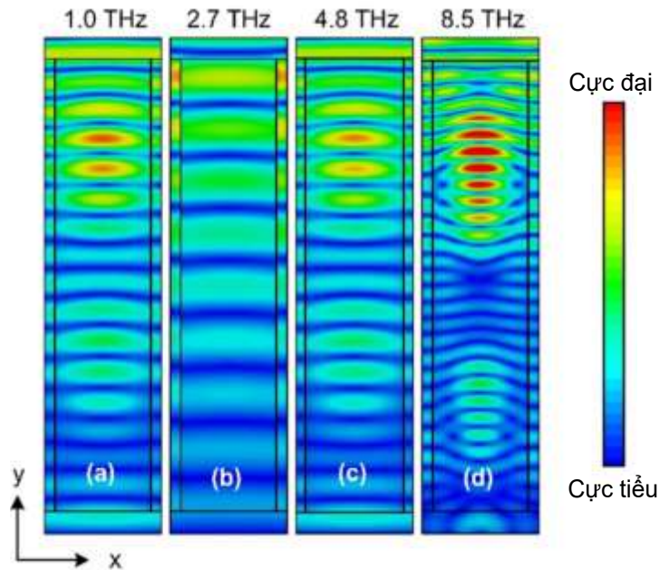
Hình 4.21. [Từ trái qua phải] Phân bố điện trường của BMPA tại các tần số khác nhau (a) 1.0 THz, (b) 2.7 THz, (c) 4.8 THz và (d) 8.5 THz [134]
