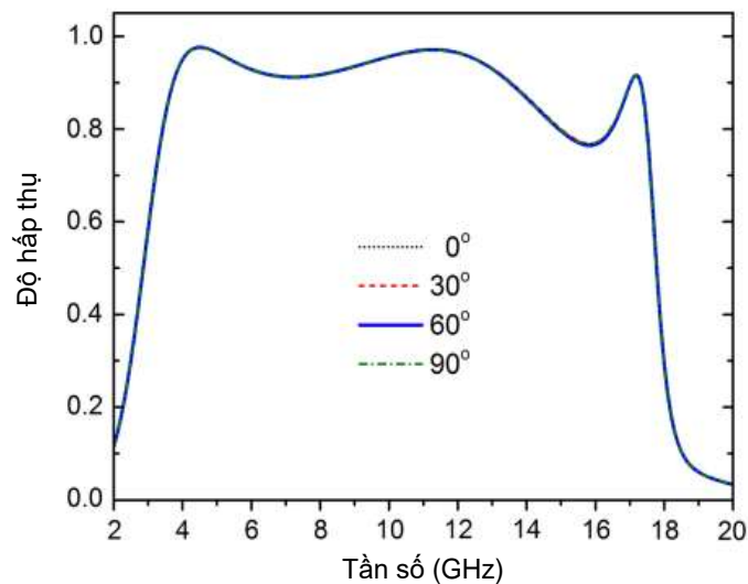
Hình 3.34. Phổ hấp thụ của BIPA với các góc phân cực khác nhau cho phân cực TE trong trường hợp góc tới vuông góc [118].
