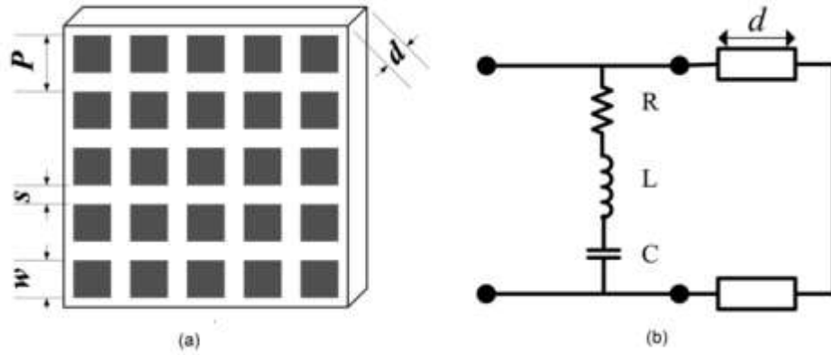
Hình 2.1. (a) Mô hình MPA đều xuất và (b) sơ đồ mạch tương đương [101].
