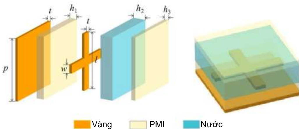
Hình 1.45. BIPA với tầng điện môi gồm lớp nước được đóng gói [72].
