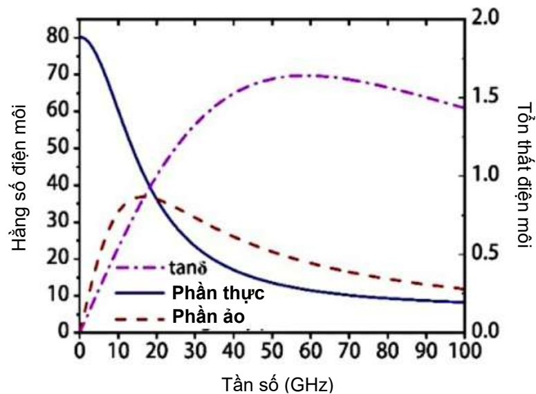
Hình 4.1. Đường cong điện môi và tổn thất điện môi của nước [133].
