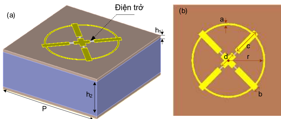
Hình 3.25. BIPA đề xuất cho băng S và băng C (a) mô hình 3D và (b) mặt trên của ô cơ sở.
