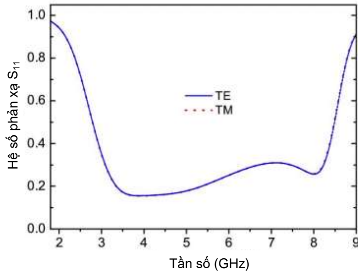
Hình 3.26. Hệ số phản xạ S_{11} của BMPA cho phân cực TE và phân cực TM.
