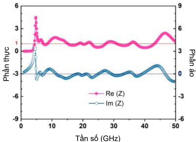
Hình 4.5. Trở kháng Z của BMPA tích hợp nước hoạt động ở vùng tần số GHz.
