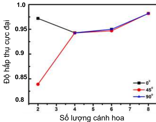
Hình 1.7. Độ hấp thụ cực đại của MPA có cấu trúc bất đẳng hướng tại các góc tới khác nhau cho phân cực TE [38].
