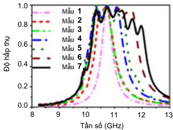
Hình 1.32. Phổ hấp thụ của MPA [66].
