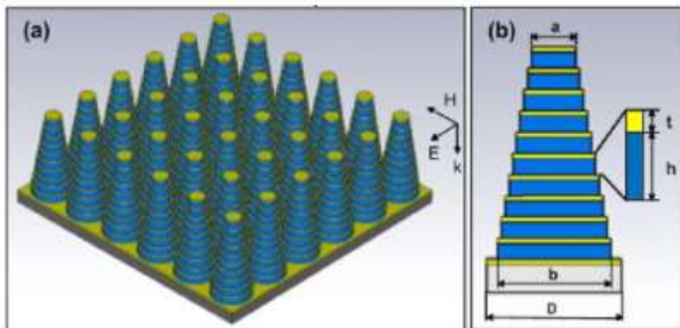
Hình 1.34. BMPA với cấu trúc đa tầng [14].
