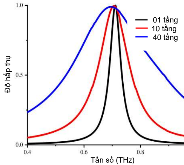
Hình 1.37. Phổ hấp thụ của BIPA đa tầng có cấu trúc cộng hưởng giống nhau [68].
