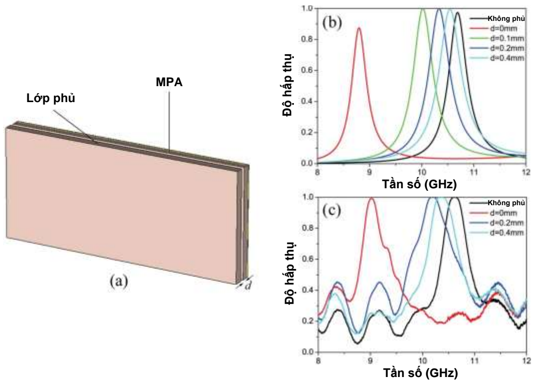
Hình 1.43. (a) MPA có tấm điện môi phủ trợ (b) Độ hấp thụ của MPA theo mô phỏng (c) Độ hấp thụ của MPA theo thực nghiệm [71].
