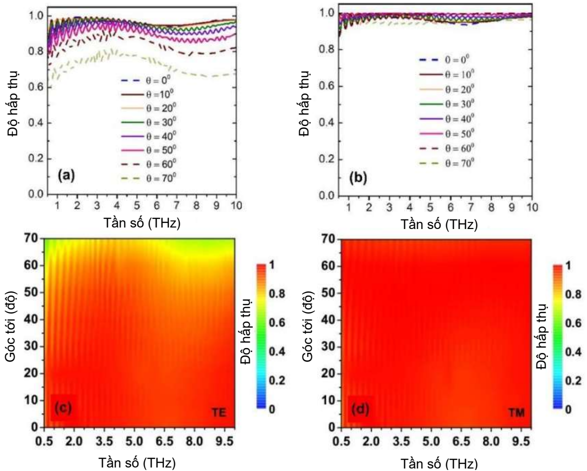
Hình 4.24. Phổ hấp thụ của BMPA với góc tới khác nhau (a, c) cho phân cực TE và (b,d) cho phân cực TM [134].
