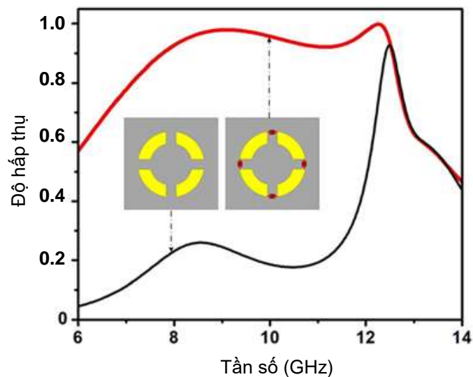
Hình 3.19. Độ hấp thụ của MPA đề xuất trong trường hợp tích hợp và không tích hợp phân tử điện trở [109].
