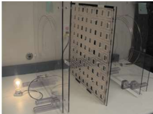
Hình 1.5. Hệ thí nghiệm mô hình WPT [36].
