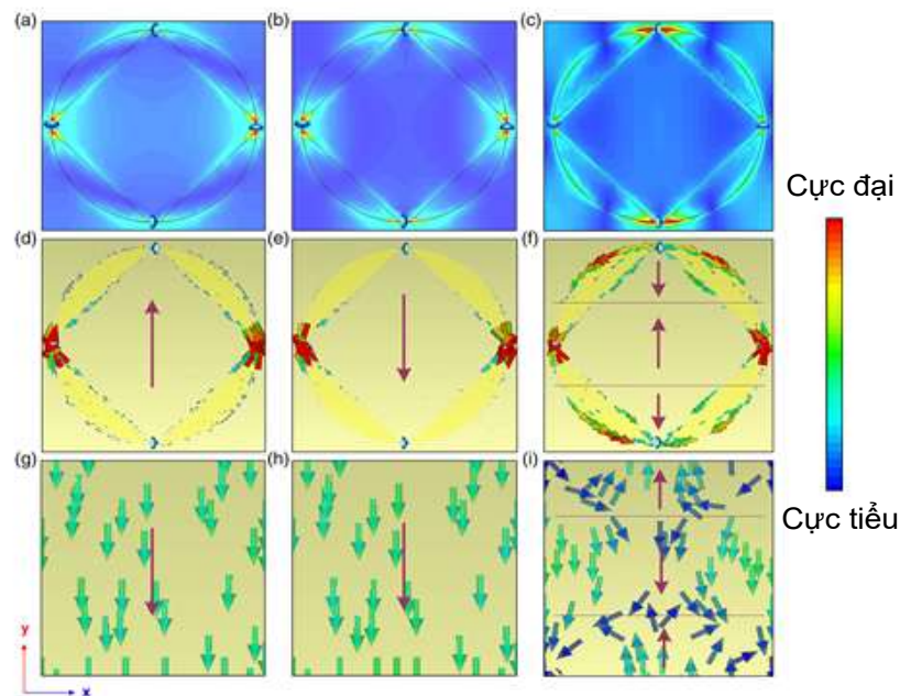
Hình 3.38. Phân bố dòng điện (a,b,c) và dòng điện cảm ứng ở mặt trên (d, e, f) và mặt dưới (g, h, i) của BMPA tại các tần số 4.5 GHz, 11.4 GHz và 17.2 GHz [118].
