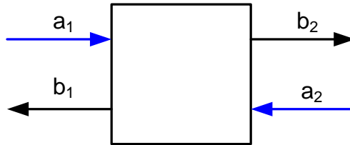
Hình 1.16. Sơ đồ mô tả tín hiệu phát và tín hiệu thu khi sóng điện từ đi qua môi trường hiệu dụng của MMs [29].
