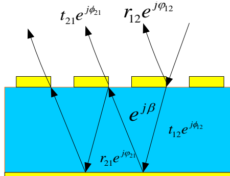
Hình 1.14. Mô hình vật liệu hấp thụ.
