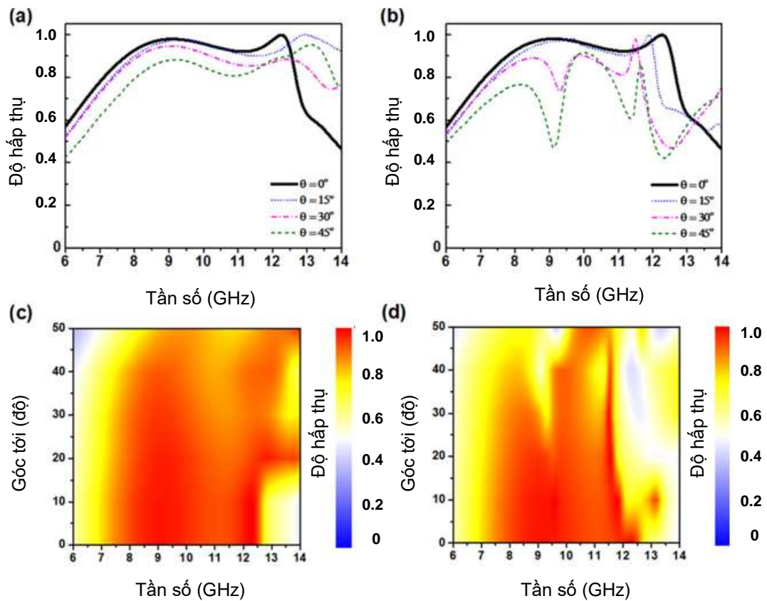
Hình 3.21. Phổ hấp thụ của BPA với các góc tới khác nhau (a) và (c) cho phân cực TE và (b) và (d) cho phân cực TM [109].
