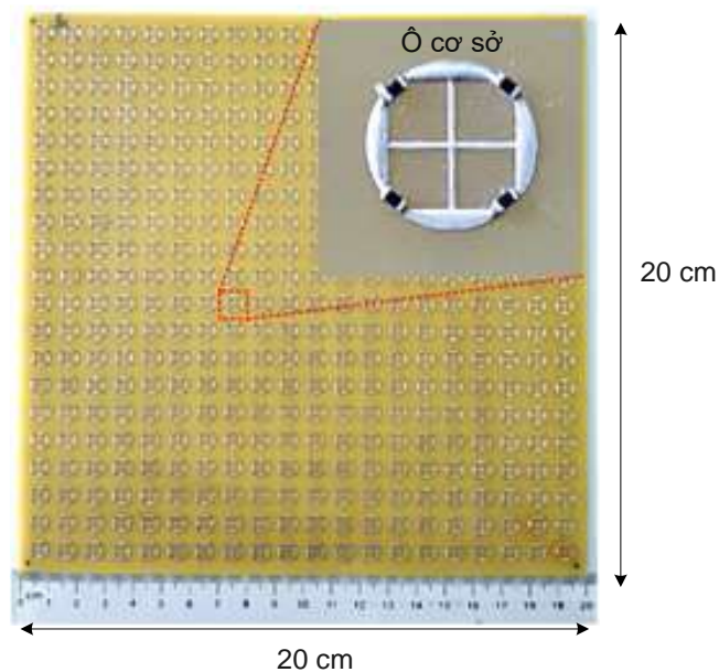
Hình 3.47. Mẫu BMPA đã chế tạo hoạt động ở băng tần X và Ku [123].
