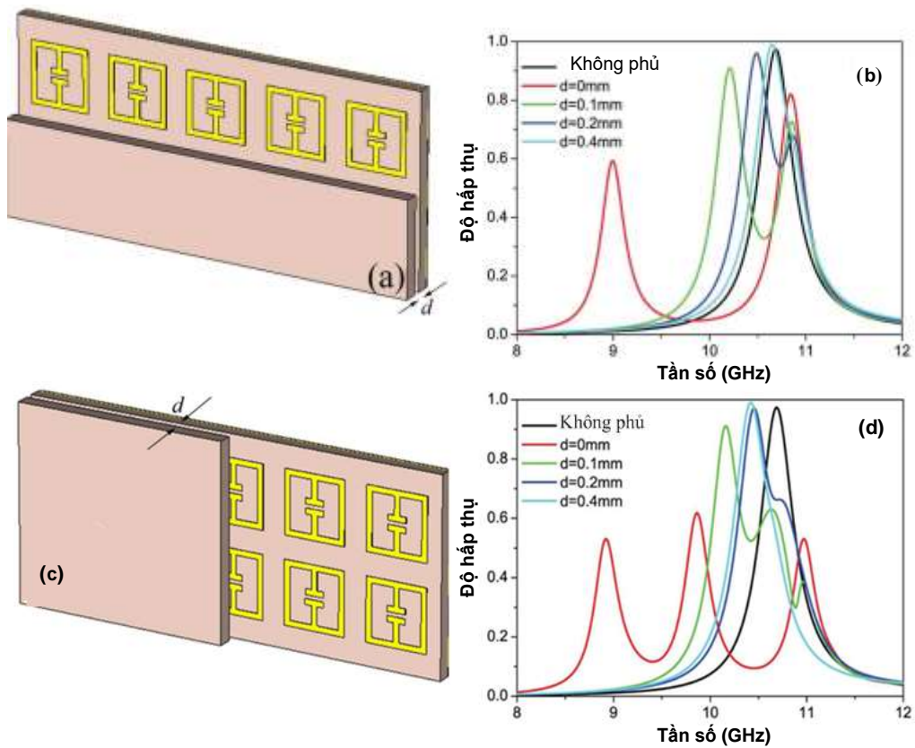
Hình 1.44. Các đỉnh hấp thụ mới được tạo ra khi thay đổi kích thước tấm điện môi phủ trợ (a-b) giảm \frac{1}{2} diện tích theo chiều dọc, (c-d) giảm \frac{1}{2} diện tích theo chiều ngang [71].
