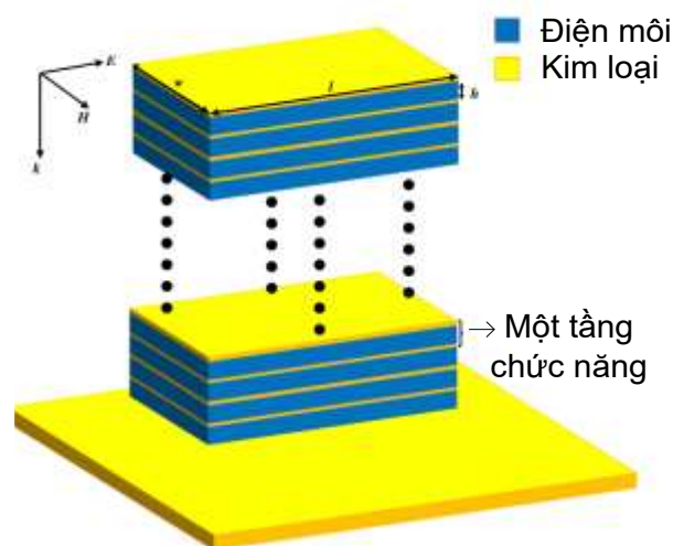
Hình 1.36. BIPA đa tầng với các cấu trúc cộng hưởng giống nhau [68].
