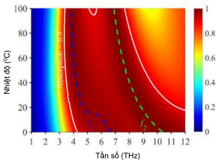
Hình 1.47. Phổ hấp thụ của BMPA thay đổi theo nhiệt độ [72].
