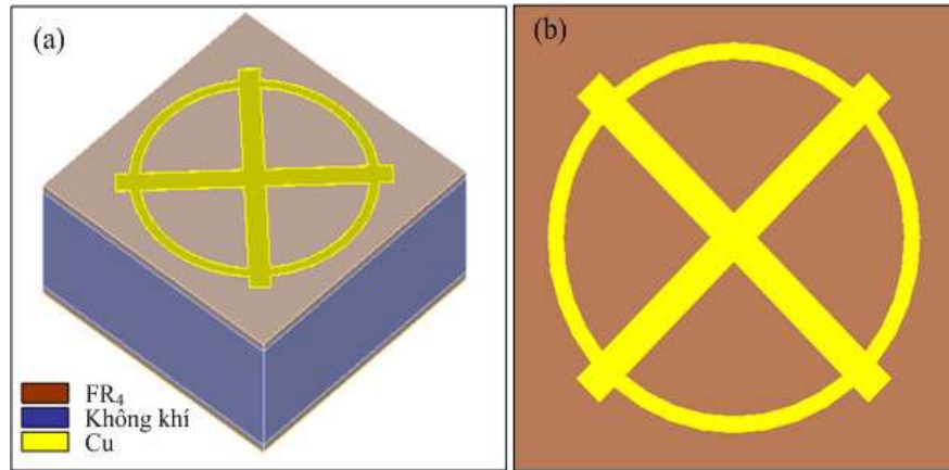
Hình 3.24. Cấu trúc MPA hình bánh xe.
