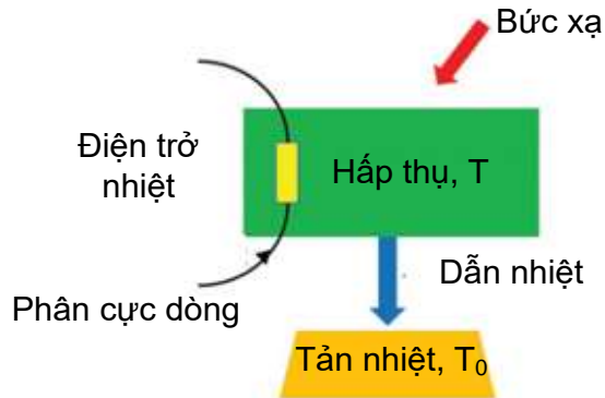
Hình 1.56. Một cấu trúc nhiệt kế bức xạ điện hình sử dụng BMPA [12].
