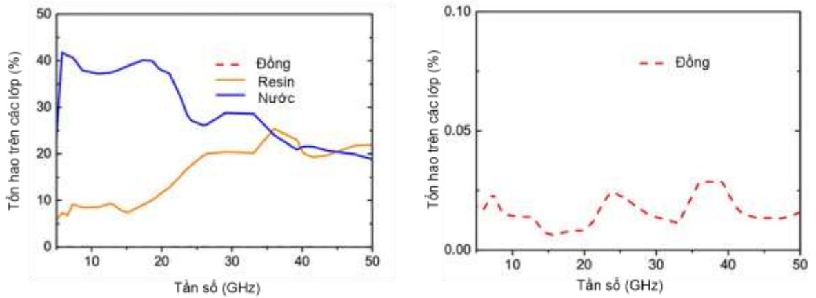
Hình 4.8. Tổn hao trên các lớp của BMPA tích hợp nước hoạt động ở vùng GHz.
