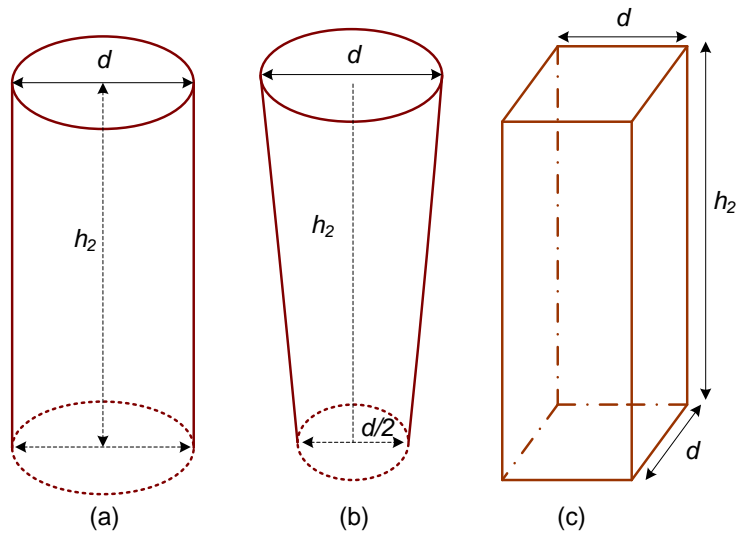
Hình 4.19. Hình dạng khác nhau của khối chứa nước.
