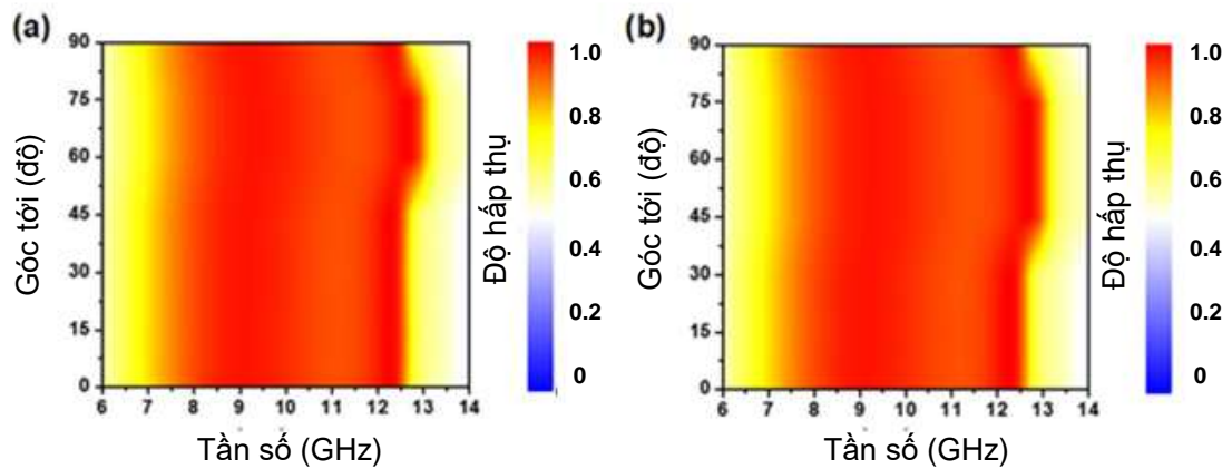
Hình 3.22. Phổ hấp thụ của BMPA với các góc phân cực khác nhau (a) cho phân cực TE và (b) cho phân cực TM [109].
