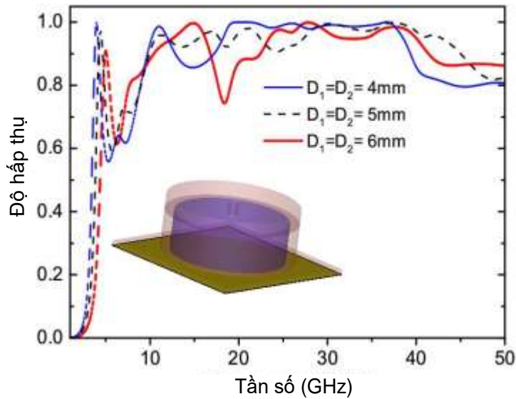
Hình 4.14. Độ hấp thụ của BMPA (II) khi thay đổi đường kính hình trụ tròn.
