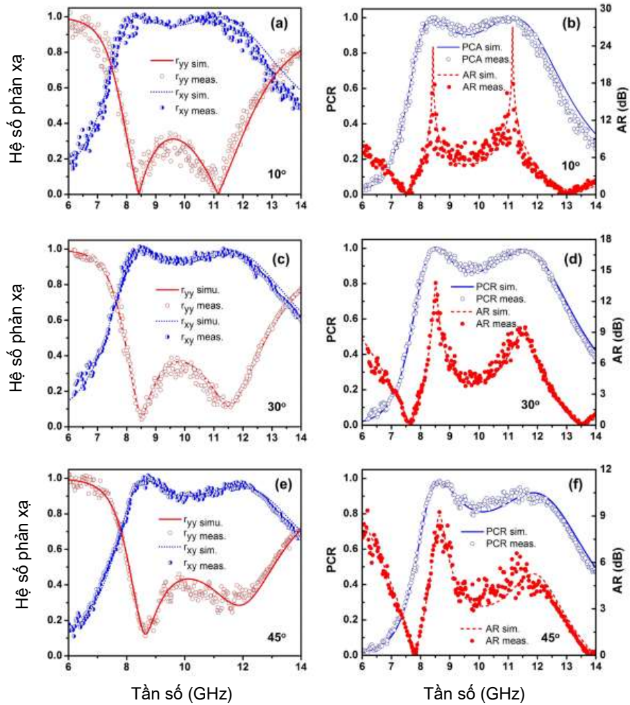
Hình 3.7. (a,c,e) Hệ số phản xạ đồng phân cực, hệ số phản xạ phân cực ngang, và PCR; (b,d,f) PCR của vật liệu biến hóa chuyển đổi phân cực sóng điện từ dưới các góc tới 10^\circ , 30^\circ , và 45^\circ tương ứng [103].
