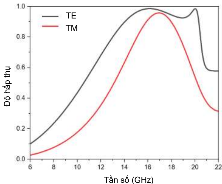
Hình 3.13. Độ hấp thụ của cấu trúc BMPA đề xuất có tích hợp điện trở ( R=150 \Omega , và P=10.2 mm) cho phân cực TE và TM khi góc tới vuông góc với bề mặt.
