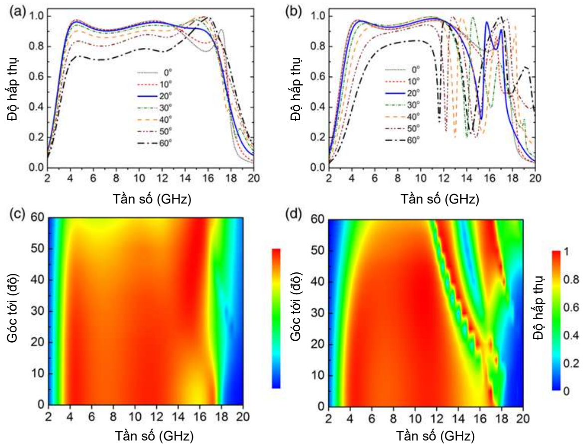
Hình 3.33. Phổ hấp thụ của BIPA với các góc tới khác nhau, (a) và (c) cho phân cực TE và (b) và (d) cho phân cực TM [118].
