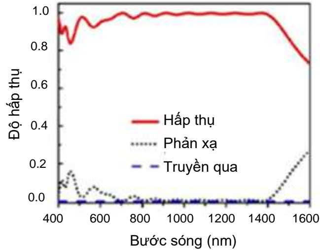
Hình 1.35. Phổ hấp thụ, phản xạ và truyền qua của BIPA [14].
