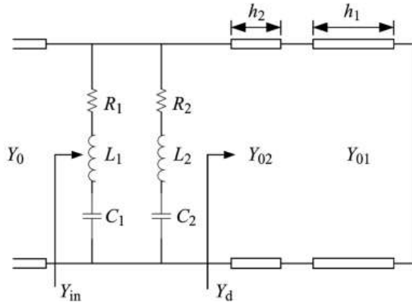
Hình 2.3. Mô hình tương đương của MPA [102].
