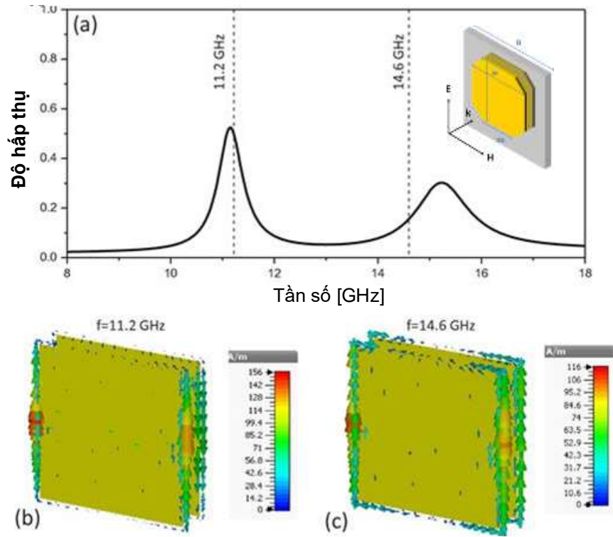
Hình 1.13. (a) Độ hấp thụ của cấu trúc CWP với a=14.8 mm và m=6 mm, (b) phân bố dòng cảm ứng bề mặt tại các tần số cộng hưởng [39].
