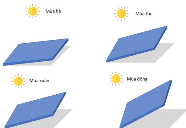
Hình 1.6. Nguyên lý thay đổi góc nghiêng theo mùa để đạt sản lượng tối đa
