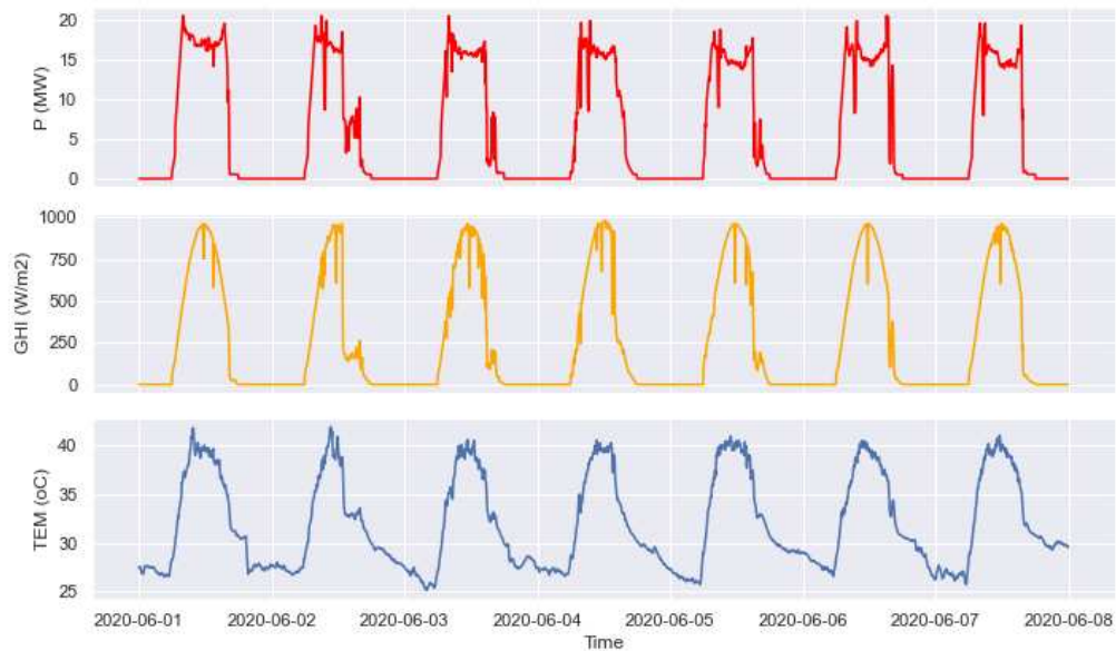
Hình 3.4. Dữ liệu quá khứ trong 1 tuần của nhà máy ĐMT
