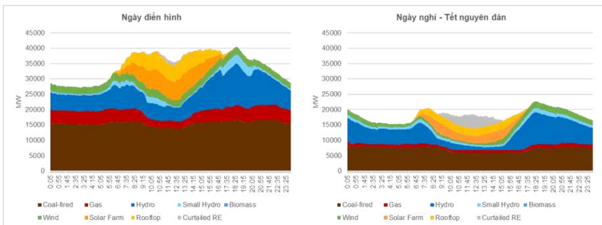
Hình MĐ.1.2. Cơ cấu nguồn ngày vận hành thông thường và ngày nghỉ lễ
