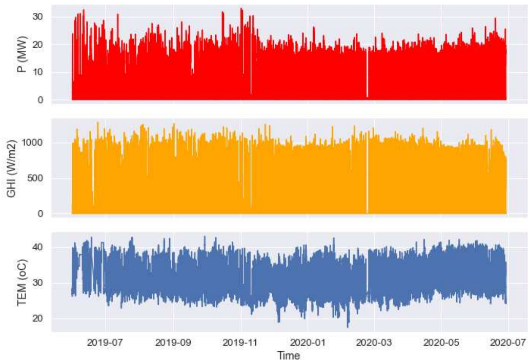
Hình 3.3. Dữ liệu vận hành nhà máy DMT
