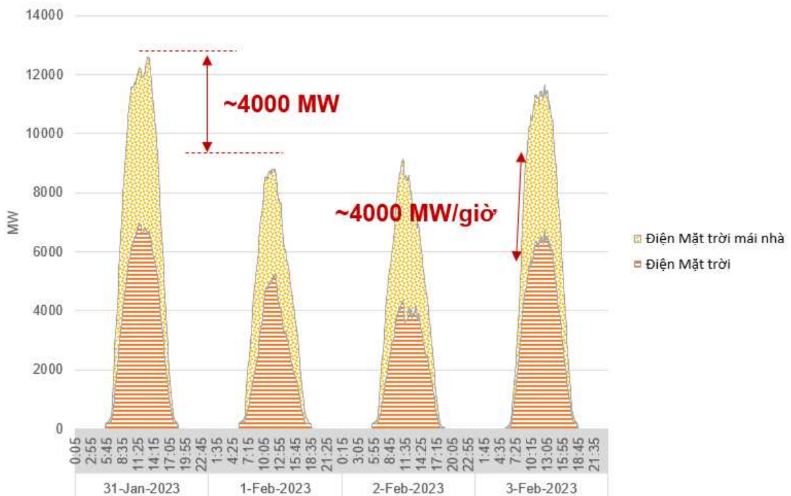
Hình MĐ.1.4. Mức độ biến động của ĐMT trong vận hành thực tế
