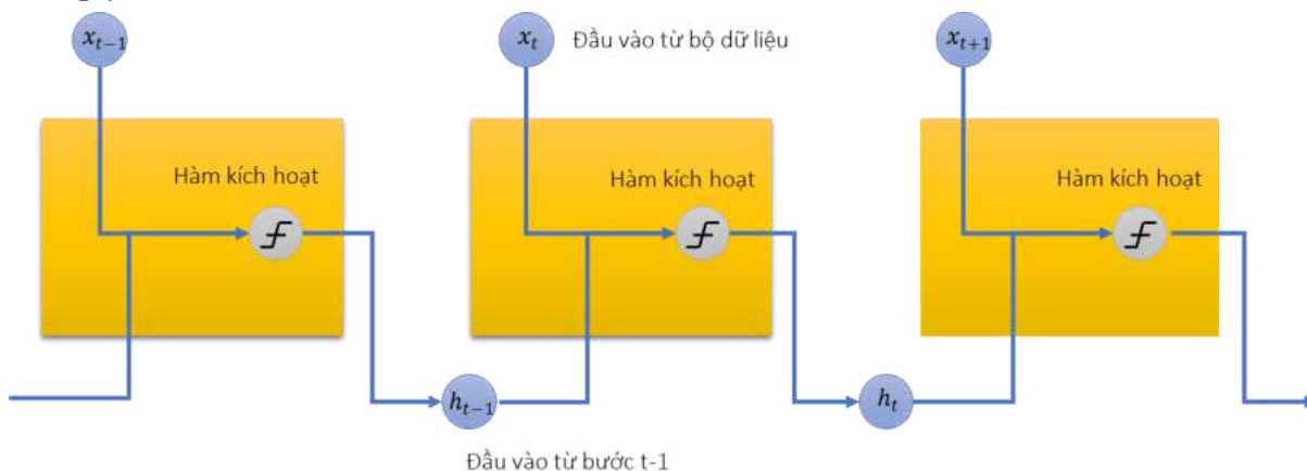
Hình 1.12. Các khối trong chuỗi khối của mạng nơ-ron hồi quy
