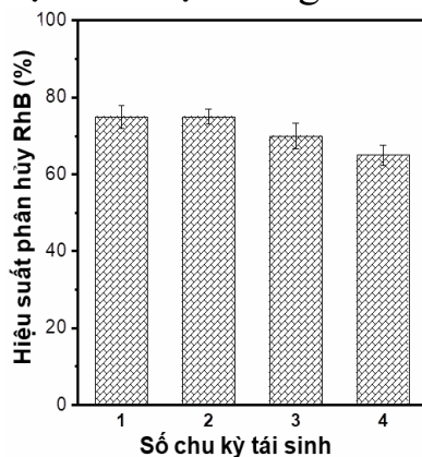
Hình 3.32. Khả năng tái sử dụng của cấu trúc nano TTOP lắp ráp với hàm lượng nước 90% làm chất xúc tác quang để loại bỏ phẩm màu RhB sau 4 chu kỳ x 360 phút/chu kỳ
