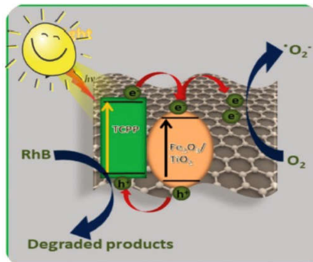
Hình 3.43. Cơ chế của chất xúc tác quang graphene/ \text{Fe}_2\text{O}_3\text{-TiO}_2\text{@porphyrin} để phân hủy quang RhB
