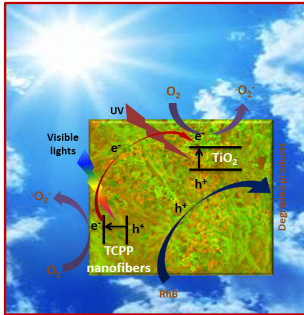
Hình 3.42. Cơ chế phản ứng quang xúc tác phân hủy RhB của vật liệu lai nano \text{TiO}_2/\text{TCPP} dưới chiếu xạ mô phỏng ánh sáng mặt trời
