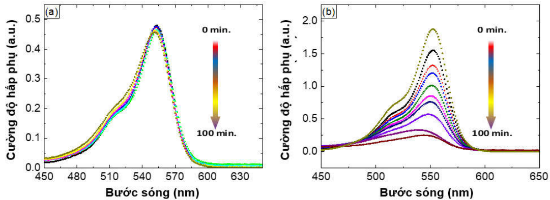
Hình 3.36. Hiệu suất quang xúc tác đối với sự phân hủy RhB của (a) TCPP đơn chất và (b) vật liệu lai graphene/Fe 2 O 3 -TiO 2 /TCPP theo thời gian
