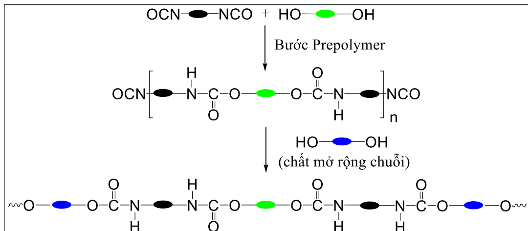
Hình 1.4. Phương trình chuẩn bị PU bằng phương pháp prepolymer
