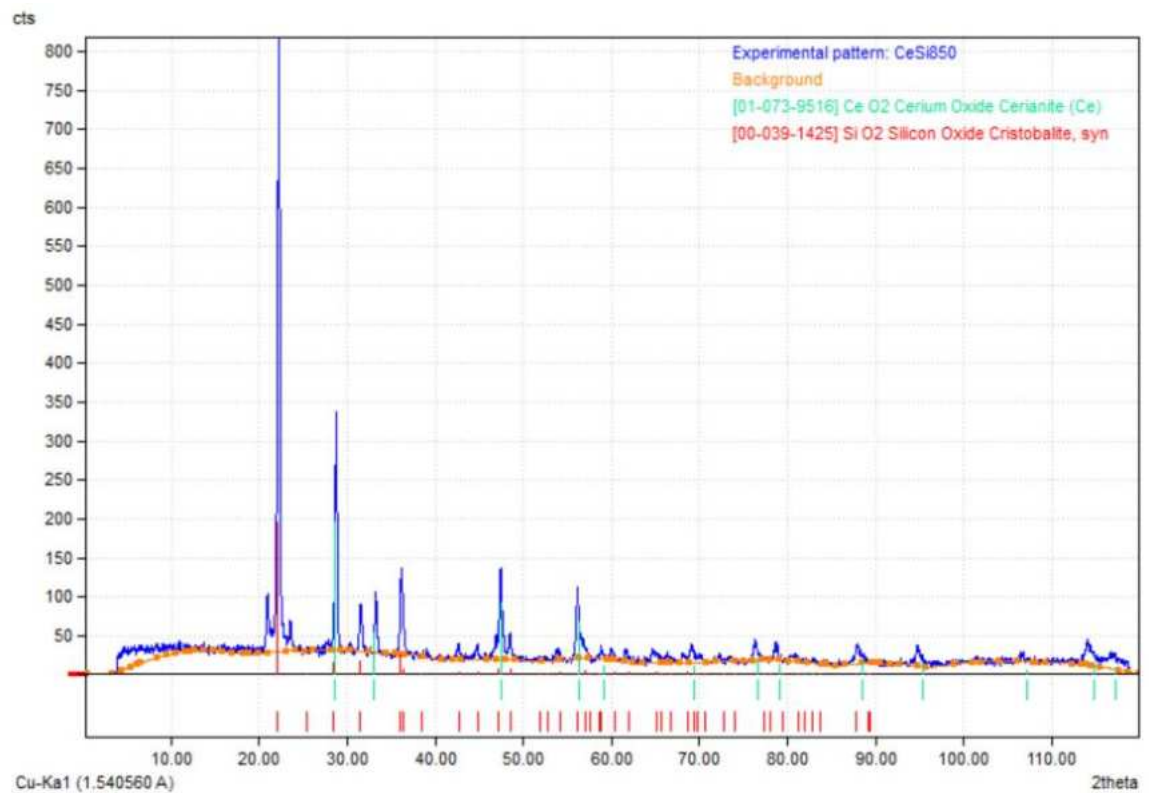
Hình S3. Phổ XRD gốc của mẫu nano \text{CeO}_2\text{-SiO}_2 được tổng hợp ở nhiệt độ nung 550, 650, 750 và 850 °C
