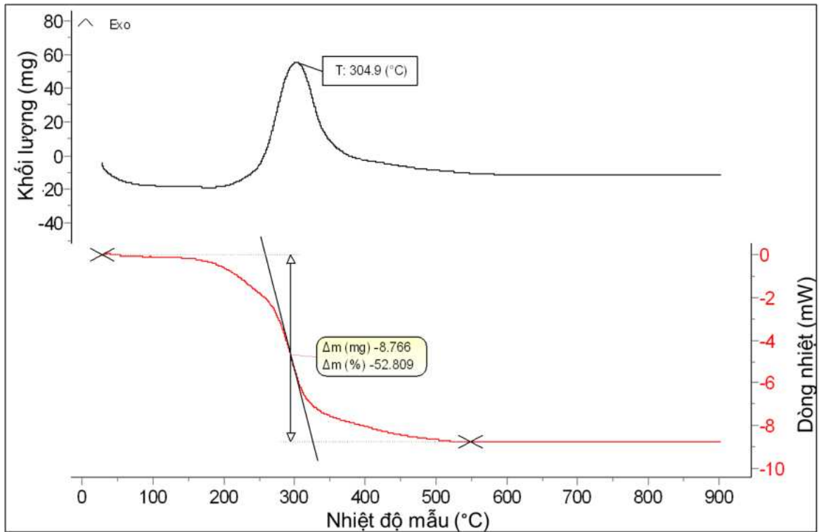
Hình 3.10. Kết quả phân tích TGA-DTA của mẫu gel khô ( \text{Si}^{4++}\text{PVA} )
