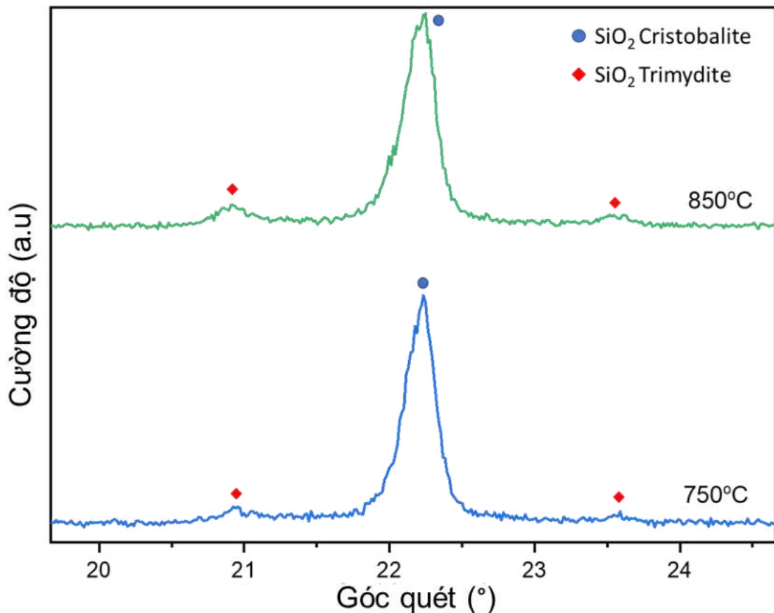
Hình 3.15. Giản đồ XRD của CS-NC được nung ở nhiệt độ 750 °C và 850 °C (CS750, CS850) tại góc quét 2θ từ 20° - 25°
