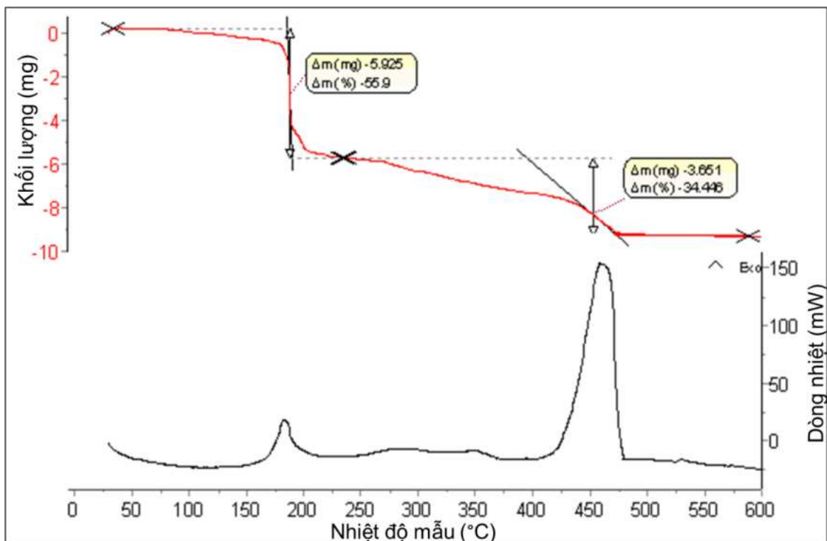
Hình 3.1. Biểu đồ TG-DTA của mẫu gel khô (Ce(NO 3 ) 3 +PVA).
