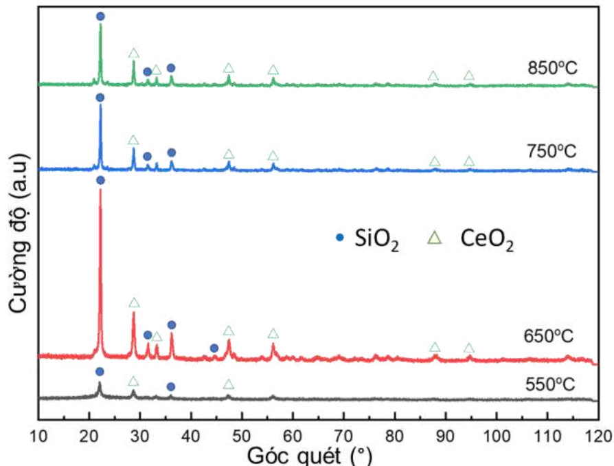
Hình 3.14. Giảm đồ nhiễu xạ XRD của vật liệu CS-NC ở các nhiệt độ nung khác nhau
