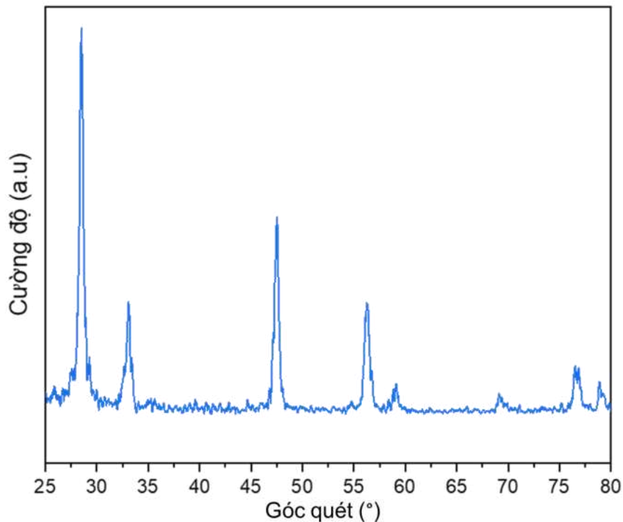
Hình 3.4. Phổ XRD của hạt nano CeO 2 tổng hợp ở nhiệt độ nung là 550 °C.
