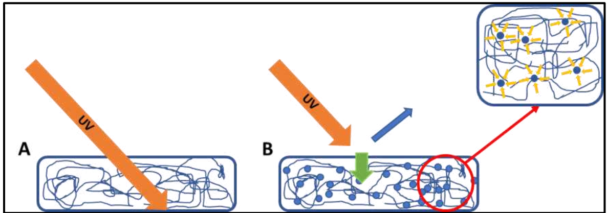
Hình 3.36. Cơ chế chung để cải thiện khả năng chống tia UV khi bổ sung vật liệu CS-NC. A) Lớp phủ PU không có vật liệu nano, B) Lớp phủ PU có sự hiện diện của vật liệu nano
