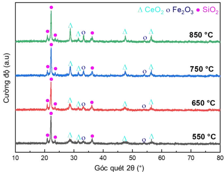
Hình 3.19. Giải đồ nhiễu xạ XRD của hạt nano \text{CeO}_2\text{-Fe}_2\text{O}_3\text{@SiO}_2
