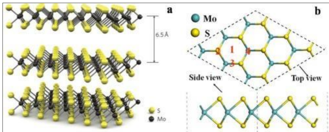
Hình 1.11. Sơ đồ minh họa cấu trúc hai chiều của \text{MoS}_2 (M là kim loại chuyển tiếp, X là một chalcogenide) [81].
