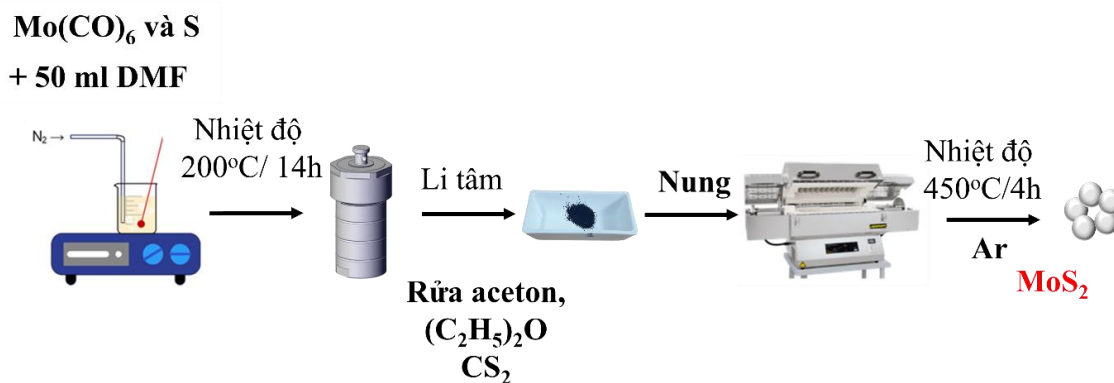
Hình 2.1. Sơ đồ quy trình tổng hợp MoS 2 bằng phương pháp nhiệt dung môi
