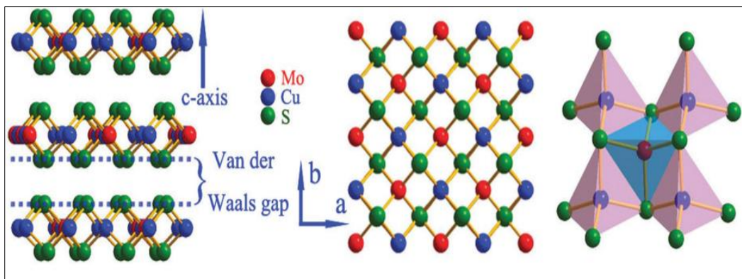
Hình 3.30. Mô hình I\text{-Cu}_2\text{MoS}_4 đề xuất bởi Wenxing Chen và cộng sự [127]
