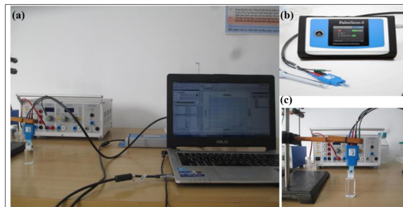
Hình 2.5. Sơ đồ hệ thiết bị hệ đo điện hóa tại phòng thí nghiệm Viện nghiên cứu Nano, Trường Đại học Phenikaa (a), hệ đo PalmSens 4 (b), thiết bị kết nối và điện cực SPE (c).
