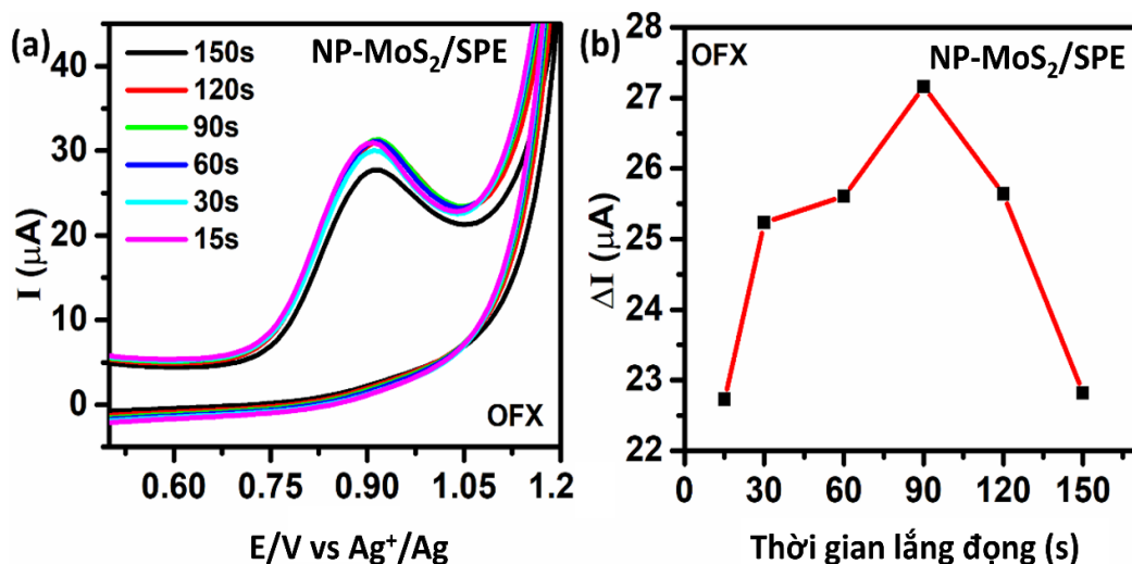
Hình 3.8. Kết quả đo CV (a), và kết quả khảo sát ảnh hưởng của thời gian lắng đọng tới tín hiệu điện hóa phát hiện OFX (b) của NP-MoS 2 /SPE, trong dung dịch PBS (pH = 7,0) có bổ sung OFX 100 μM với tốc độ quét 60 mV/s.
