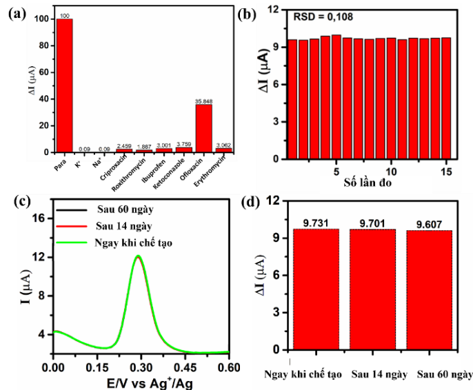
Hình 3.19. Kết quả khảo sát độ chọn lọc (a), độ lặp lại (b) và độ ổn định (c) của cảm biến điện hóa NP-MoS 2 /SPE, trong dung dịch PBS 0,1 M (pH = 3,0) chứa PAR 100 μM.
