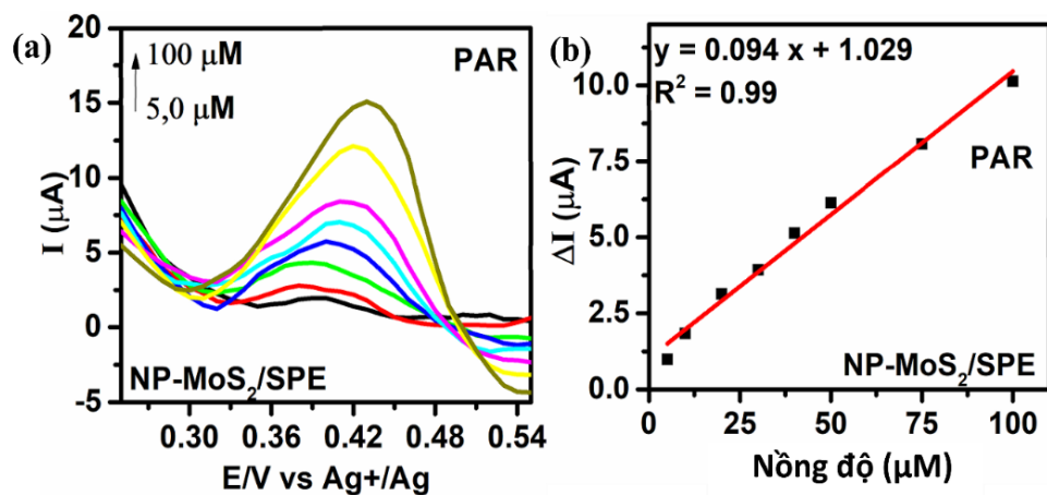
Hình 3.18. Đường DPV biểu diễn tín hiệu điện hóa (a) và đường chuẩn xác định PAR (b), của cảm biến NP-MoS 2 /SPE trong dung dịch PBS 0,1 M (pH = 3,0) có chứa PAR với nồng độ từ 5 đến 100 μM.
