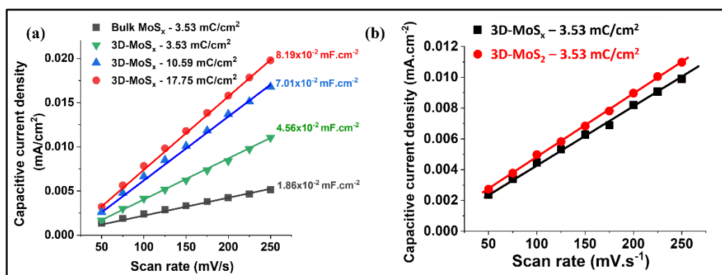
Hình 10. Biểu đồ biểu diễn mối quan hệ giữa giá trị điện dung lớp điện kép với tốc độ quét của các vật liệu: vật liệu 3D-MoS x (3,53 – 17,75 mC/cm 2 ) và MoS x 3,53 mC/cm 2 (a); vật liệu 3D-MoS x và 3D-MoS 2 (3,53 mC/cm 2 ) (b).
