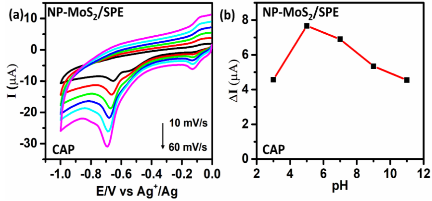
Hình 3.13. Kết quả khảo sát ảnh hưởng của tốc độ quét (a) và pH (b) tới tín hiệu điện hóa xác định CAP của điện cực NP-MoS 2 /SPE.
