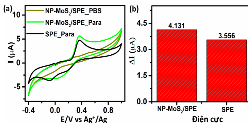
Hình 3.16. Kết quả đo CV (a) và biểu đồ hình cột tín hiệu (b), của điện cực NP-MoS 2 /SPE và SPE trong dung dịch PBS 0,1 M (pH = 7,0), có bổ sung thêm PAR 100 \mu M, với vận tốc quét 60 mV/s.
