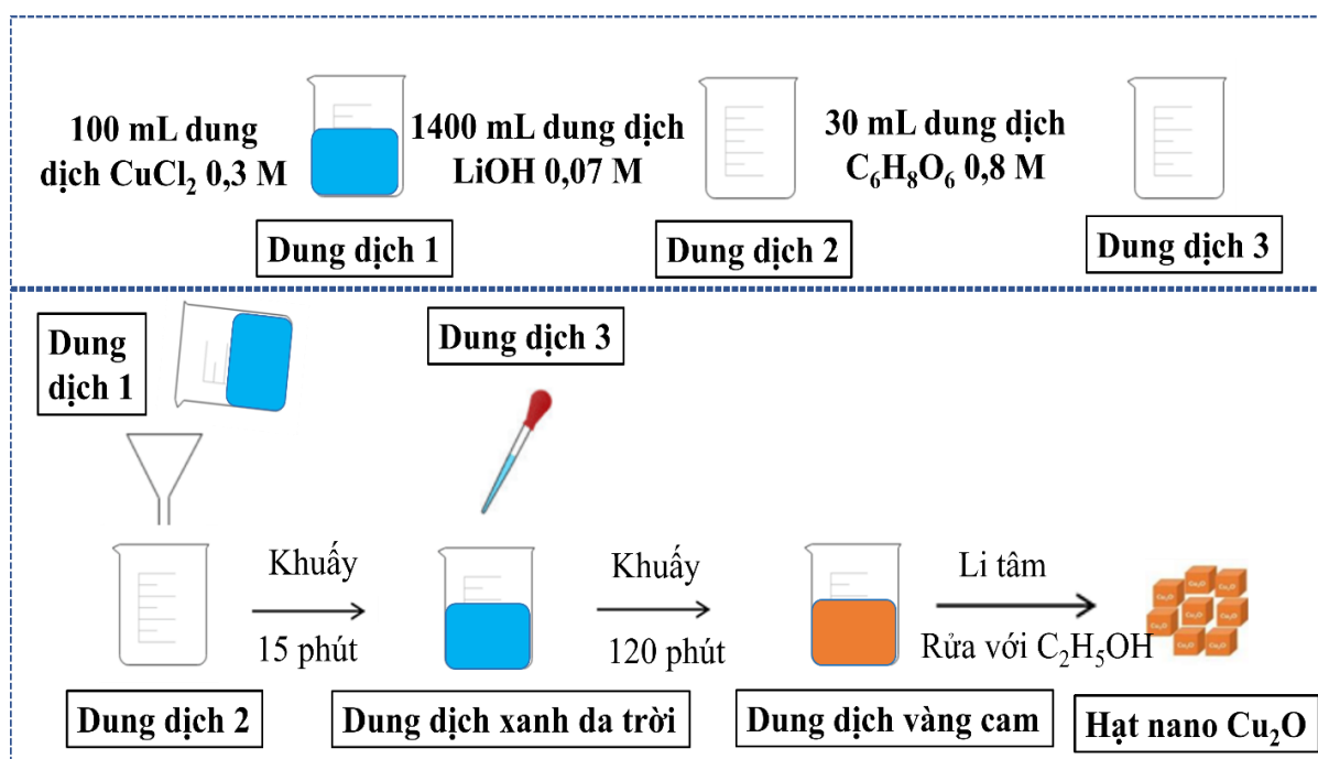
Hình 2.2. Quy trình chế tạo hạt nano \text{Cu}_2\text{O} [109].
