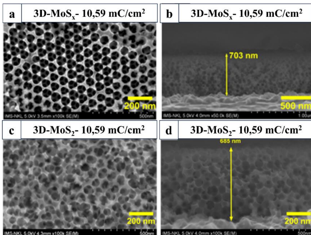
Hình 7. Hình ảnh SEM mô tả bề mặt và hình thái mặt cắt của điện cực 3D-MoS x /FTO (a, b) và điện cực 3D-MoS 2 /FTO (c, d).
