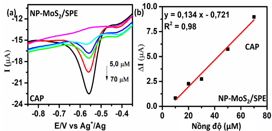
Hình 3.14. Kết quả đo DPV (a) và đường chuẩn biểu diễn mối liên hệ giữa cường độ dòng đỉnh và nồng độ CAP (b) của NP-MoS 2 /SPE trong dung dịch PBS 0,1 M (pH = 5,0) CAP thay đổi từ 5,0 đến 70 μM, tốc độ quét 60 mV/s.
