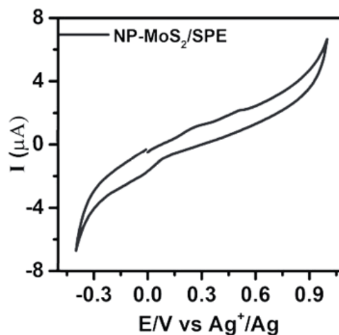
Hình 3.6. Kết quả đo CV của vật liệu NP-MoS 2 trong dung dịch PBS 0,1 M (pH = 7,0), với tốc độ quét 10 mV/s.
