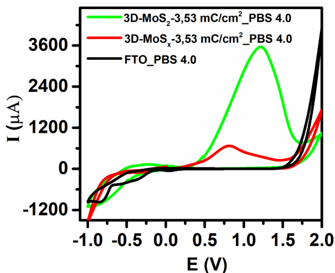
Hình 12. Đường CV của 3 điện cực 3D-MoS x - 3,53 mC/cm 2 /FTO; 3D-MoS 2 - 3,53 mC/cm 2 /FTO và FTO trong dung dịch PBS (pH = 4,0), với tốc độ quét 10 mV s -1 .
