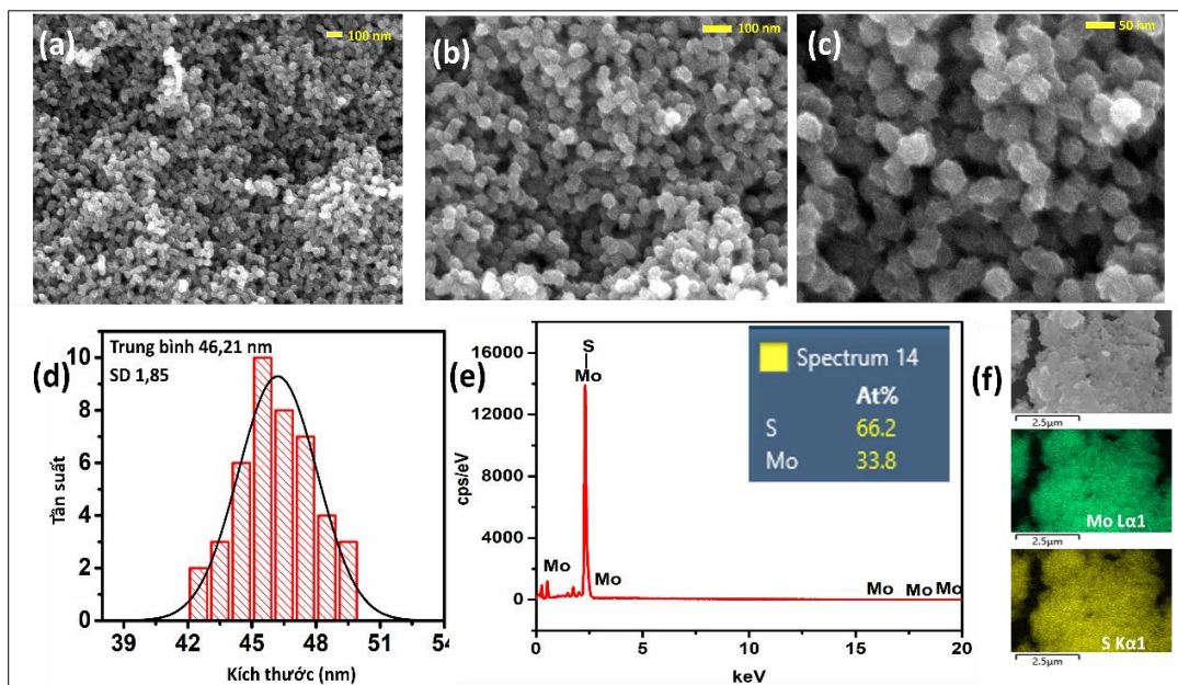
Hình 3.1. Ảnh FE-SEM với độ phóng đại khác nhau (a, b, c), biểu đồ phân bố kích thước đường kính hạt (d), giản đồ EDX và ảnh EDX mapping của vật liệu NP-MoS 2 tổng hợp bằng phương pháp nhiệt dung môi (e, f).
