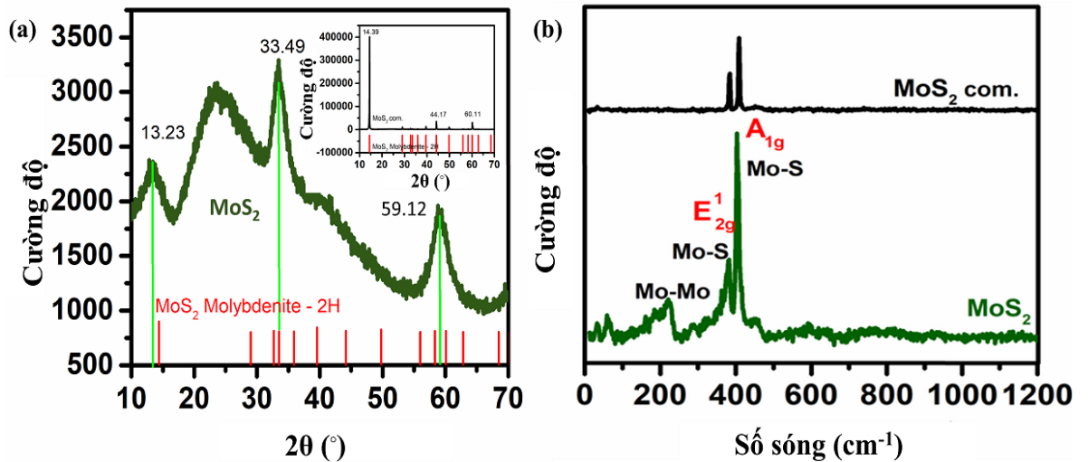
Hình 3.2. Giải đồ nhiễu xạ tia X (a) và phổ raman (b) của NP-MoS 2 tổng hợp bằng phương pháp nhiệt dung môi và MoS 2 thương mại.
