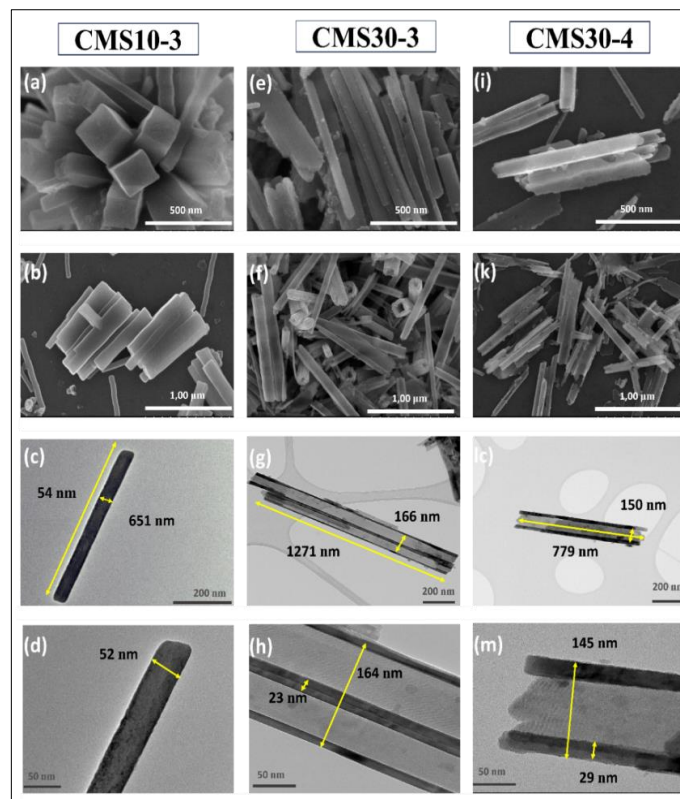
Hình 3.20. Ảnh FE-SEM và HR-TEM với độ phóng đại khác nhau của các mẫu CMS10-3 (a-d), CMS30-3 (e-h), CMS30-4 (i-m).
