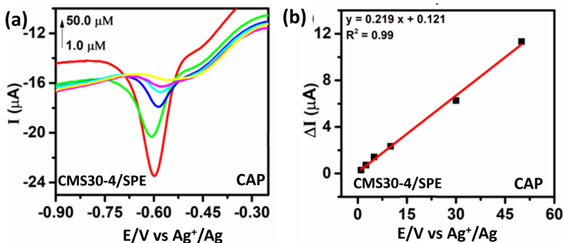
Hình 3.36. Kết quả đo DPV trong dung dịch PBS 0,1M (pH = 5,0) chứa CAP với nồng độ thay đổi từ 1,0 đến 50 \mu\text{M} (a) và đường chuẩn xác định CAP bằng điện cực CMS30-4/SPE (b).
