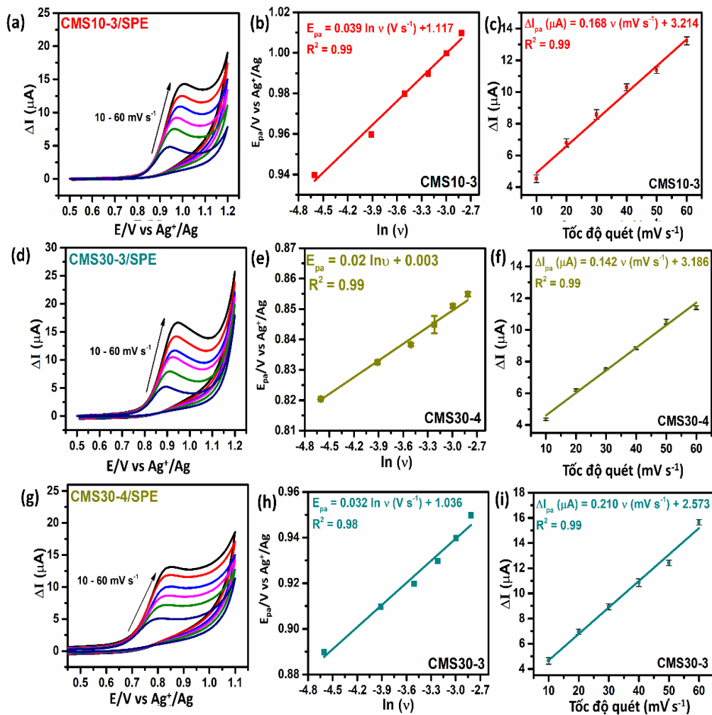
Hình 3.28. Kết quả đo CV của dung dịch PBS 0,1 M (pH = 7,0) chứa OFX 100 \mu\text{M} với các giá trị tốc độ quét từ 10 đến 60 \text{mV.s}^{-1} ; đường chuẩn biểu diễn mối quan hệ giữa các giá trị ( E_{pa} , \ln v ), ( \Delta I_{pa} , v ) của các điện cực CMS10-3/SPE (a, b, c), CMS30-3/SPE (d, e, f), và CMS30-4/SPE (g, h, i).
