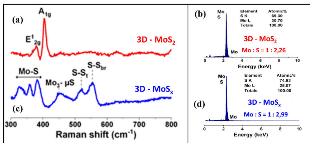
Hình 8. Phổ Raman và phổ EDX của vật liệu 3D-MoS 2 (a, b) và 3D-MoS x (c, d) được tổng hợp với điện tích lắng đọng 10,59 mC/cm 2 .
