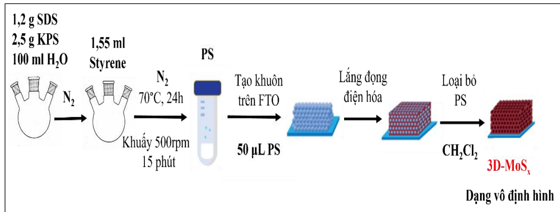
Hình 1. Sơ đồ quy trình tổng hợp 3D-MoS x bằng phương pháp lắng đọng điện hóa
