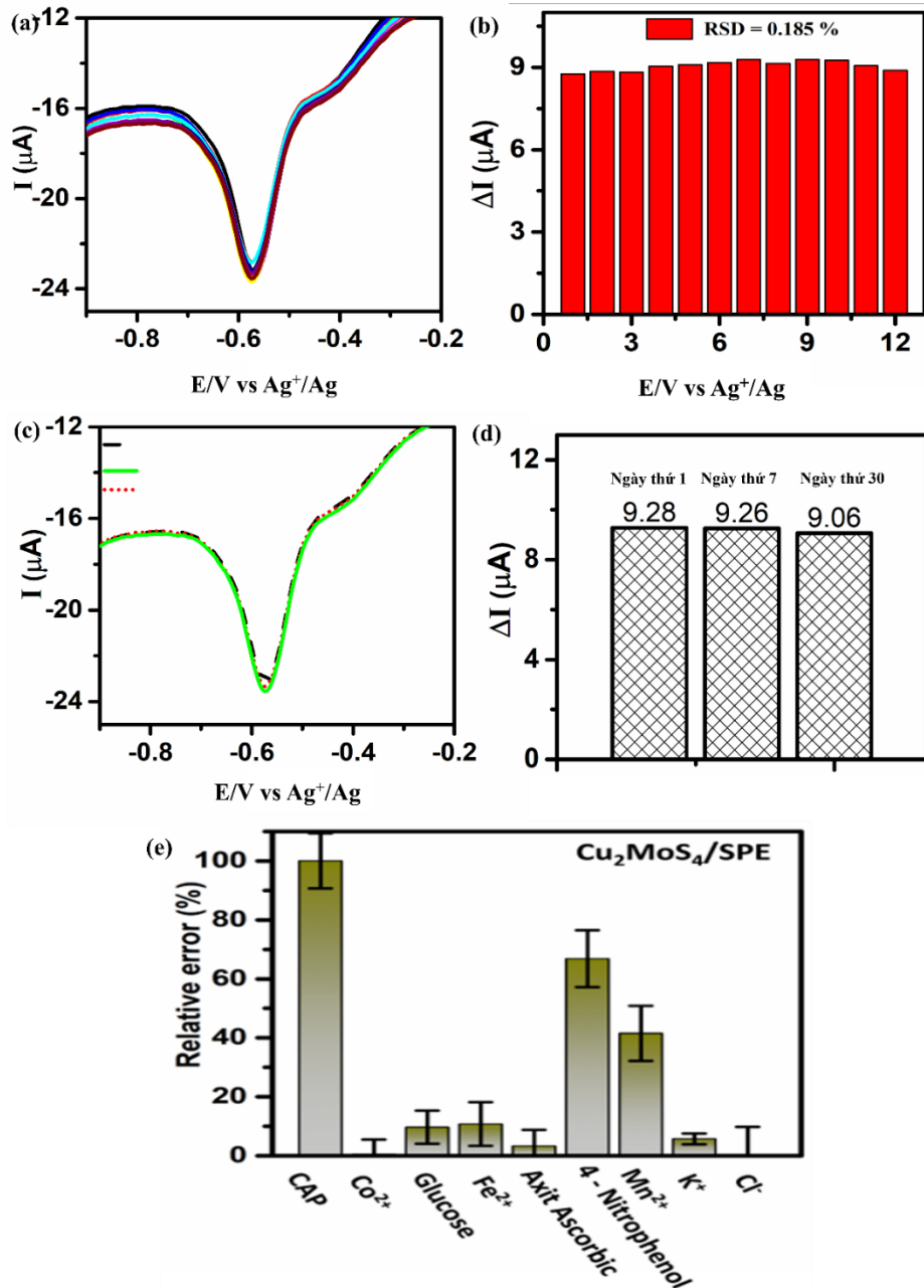
Hình 3.37. Đường DPV khảo sát độ ổn định (a, b), độ lặp lại (c, d), và độ chọn lọc (e) của điện cực CMS30-4/SPE trong dung dịch PBS 0,1M (pH = 5,0) có chứa CAP với nồng độ 100 \mu\text{M} .
