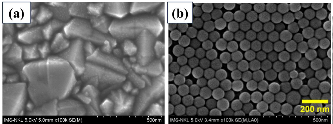
Hình 2. Ảnh SEM của bề mặt FTO trước (a) và sau khi phủ PS (b).
