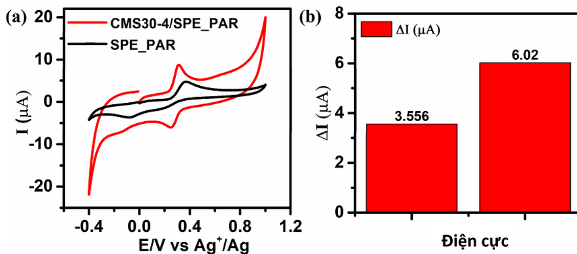
Hình 3.38. Đường CV a) và biểu đồ hình cột tín hiệu b) của các điện cực SPE và CMS30-4/SPE đối với PAR trong dung dịch PBS (pH = 7,4) chứa PAR 100 \mu\text{M} .
