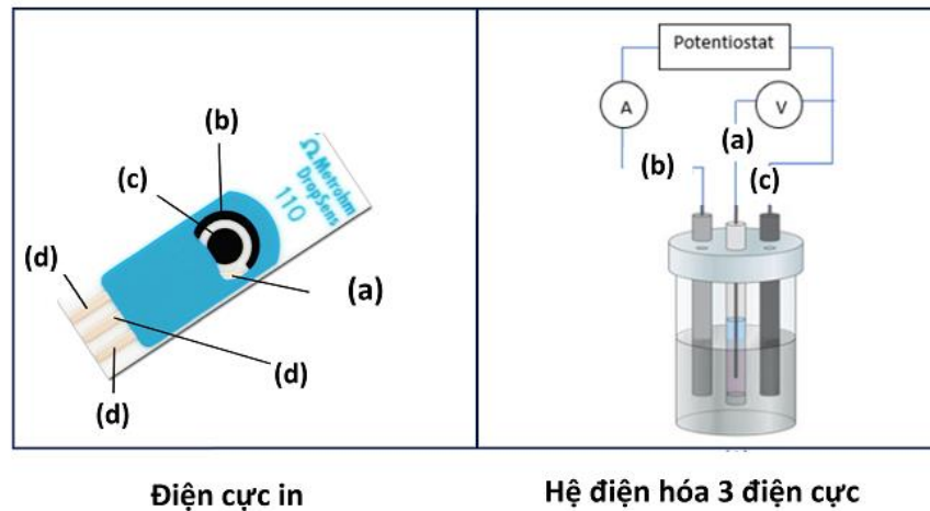
Hình 1.5. Điện cực in (SPE): điện cực so sánh (a); điện cực đối (b); điện cực làm việc (c), đầu kết nối (d) và hệ điện hóa ba điện cực.
