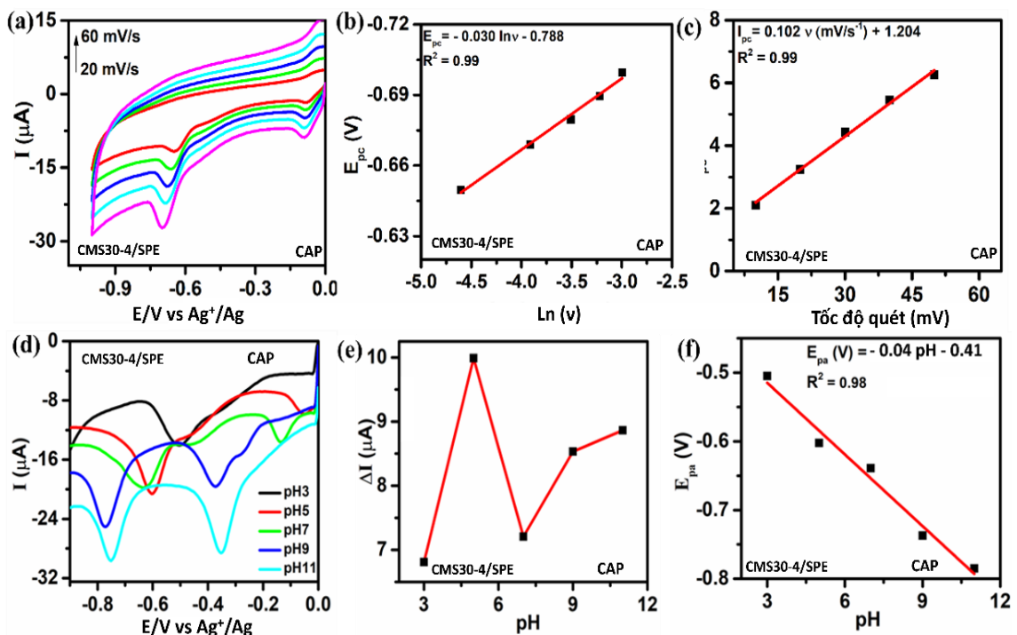
Hình 3.35. Kết quả khảo sát ảnh hưởng của tốc độ quét (a, b, c); pH (d, e, f) đối với khả năng phát hiện CAP của điện cực CMS30-4/SPE.
