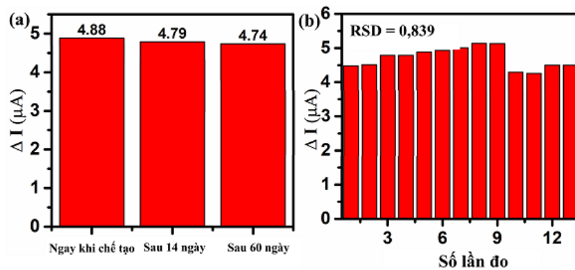
Hình 3.15. Kết quả đo DPV khảo sát độ lặp lại (a) và độ ổn định (b) của điện cực NP-MoS 2 /SPE trong dung dịch PBS 0,1M (pH = 5,0) có chứa CAP 50 \mu\text{M} , với tốc độ quét 60 mV/s.
