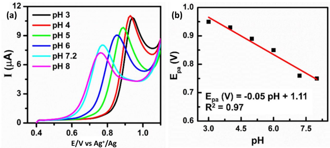
Hình 3.31. Kết quả khảo sát ảnh hưởng của pH đối với khả năng phát hiện OFX của điện cực CMS30-4/SPE.
