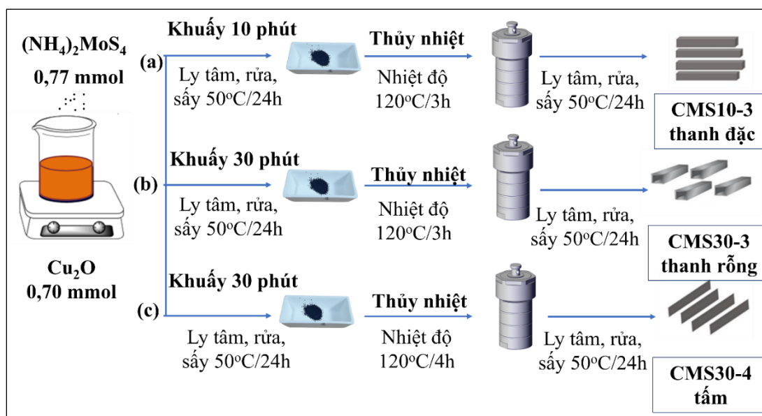
Hình 2.3. Sơ đồ quy trình tổng hợp vật liệu CMS bằng phương pháp thủy nhiệt CMS10-3 (a), CMS30-3 (b), CMS30-4 (c) [109].
