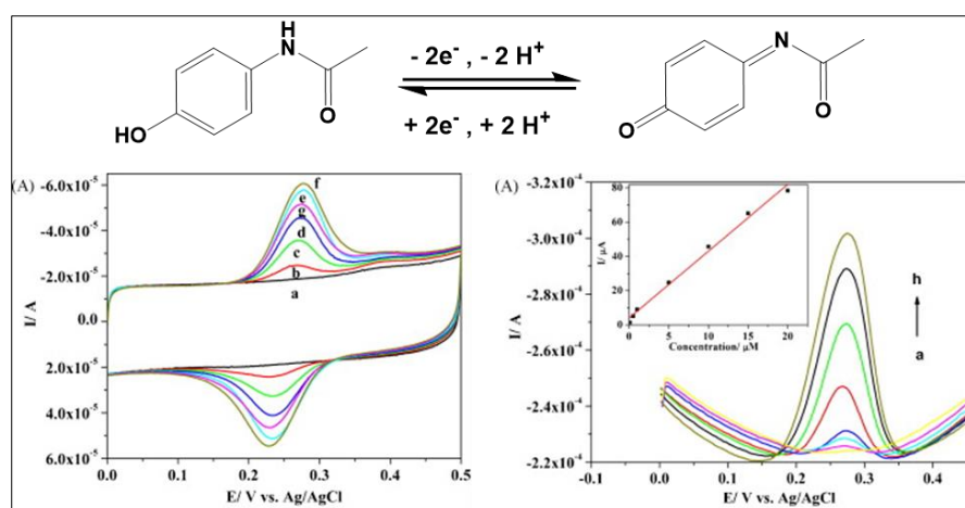
Hình 1.9. Phản ứng oxi hóa – khử và cảm biến điện hóa phát hiện PAR trên cơ sở graphen [46].
