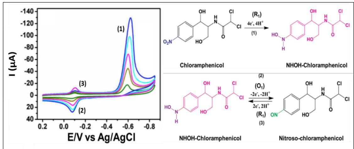
Hình 1.7. Phản ứng oxi hóa – khử của CAP [44].
