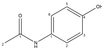
Hình 1.3. Cấu trúc của paracetamol
