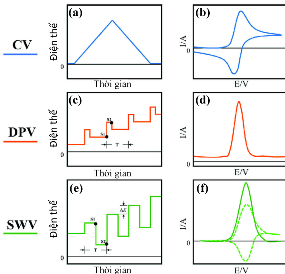
Hình 1.6. Mô hình điện thế áp dụng lên điện cực theo thời gian và đồ thị ghi nhận cường độ dòng phản hồi theo điện thế áp dụng đối với các kỹ thuật quét thế vòng tuần hoàn (CV), quét thế xung vi phân (DPV), quét thế xung vuông (SWV) [34].
