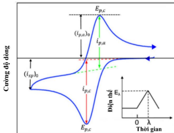
Hình 2.9. Đường CV trong trường hợp có chất hoạt động điện hóa và phản ứng xảy ra thuận nghịch [113].
