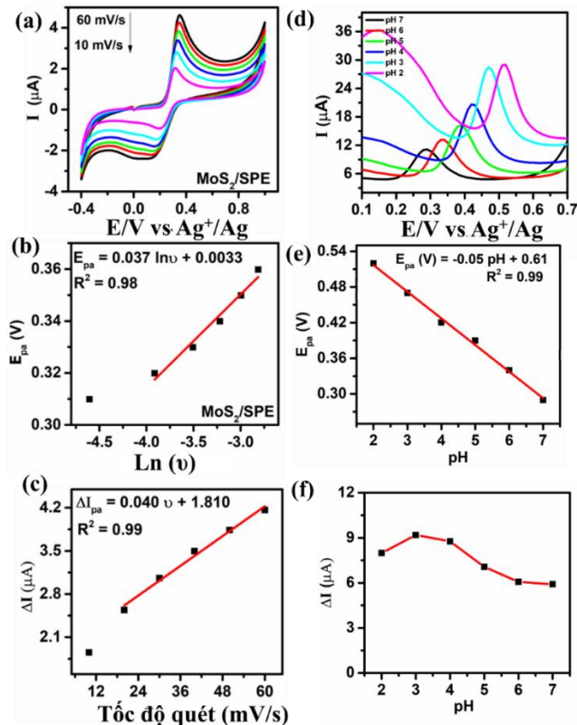
Hình 3.17. Khảo sát ảnh hưởng của tốc độ quét (a-c), pH (d-f) đến tín hiệu phát hiện PAR; trong dung dịch PBS 0,1 M có PAR với nồng độ 100 \mu\text{M} .
