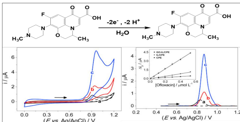
Hình 1.8. Phản ứng oxi hóa – khử của OFX và cảm biến điện hóa xác định OFX trên cơ sở graphene oxide [45].
