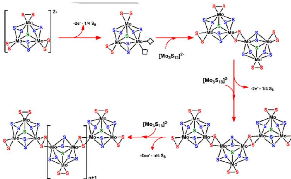
Hình 5. Sơ đồ cơ chế cho quá trình tổng hợp 3D-MoS x từ [Mo 3 S 13 ] 2- [100].
