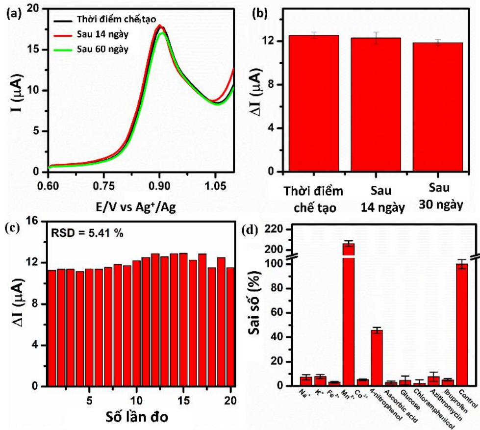
Hình 3.33. Kết quả đo DPV khảo sát độ ổn định (a, b), và độ lặp lại (c), độ chọn lọc của cảm biến CMS30-4/SPE trong dung dịch PBS 0,1M (pH = 4,0) có chứa OFX 100 \mu M.
