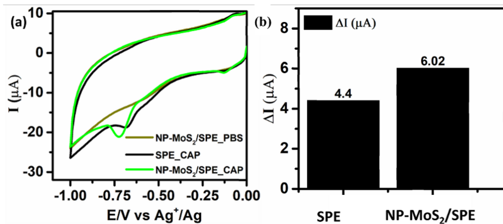
Hình 3.12. Kết quả đo CV (a), và biểu đồ hình cột (b) của điện cực NP-MoS 2 /SPE và SPE trong dung dịch PBS 0,1 M (pH = 7,0) có bổ sung thêm CAP 100 \mu M, với vận tốc quét 10 mV/s.
