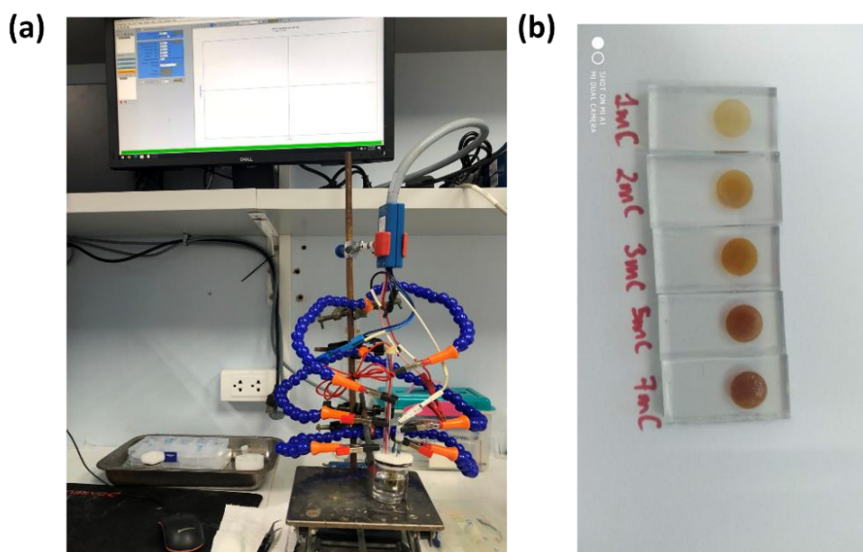
Hình 6. Sơ đồ hệ thiết bị hệ đo điện hóa đa năng Bio-LogicSP-300 tại phòng thí nghiệm Trường Đại học Khoa học và Công nghệ Hà Nội (a) và điện cực 3D-MoS x /FTO được tổng hợp với dung lượng khác nhau (b).
