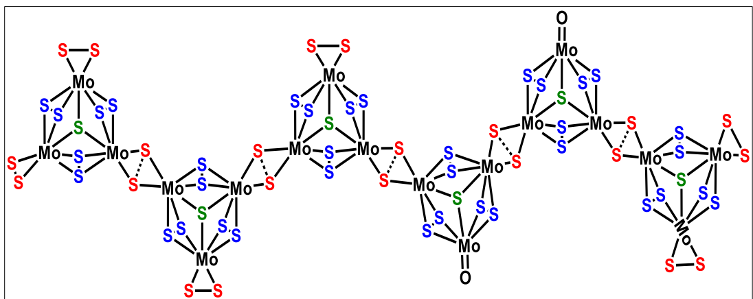
Hình 1.12. Cấu trúc MoS x vô định hình [82].
