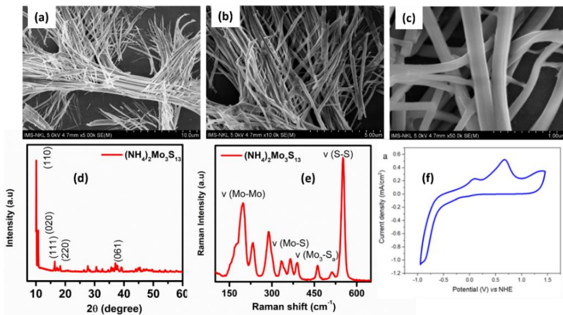
Hình 4. Ảnh SEM (a-c), giản đồ XRD (d), phổ Raman của (\text{NH}_4)_2\text{Mo}_3\text{S}_{13} (e) và đường CV của (\text{NH}_4)_2\text{Mo}_3\text{S}_{13} 1 mM trong dung dịch điện ly \text{LiClO}_4 0.1 M với tốc độ quét 20 mV/s (f).
