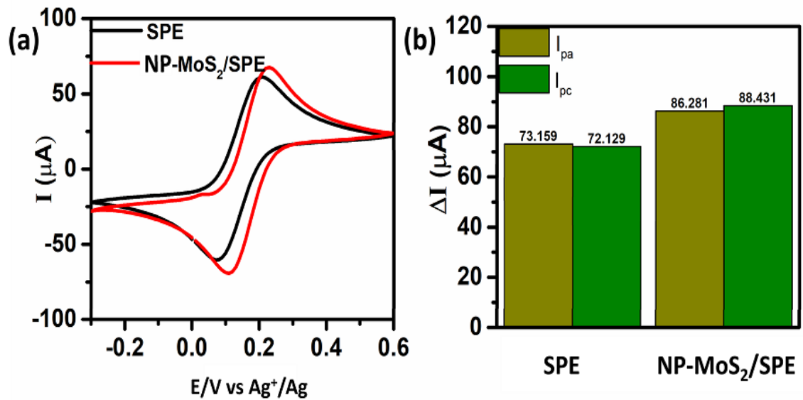
Hình 3.3. Kết quả đo CV (a) và đồ thị so sánh cường độ dòng oxi hóa, dòng khử (b) của 2 điện cực SPE và NP-MoS 2 /SPE trong dung dịch [Fe(CN) 6 ] 3-/4- 5 mM, tốc độ quét 10 mV. s -1 .
