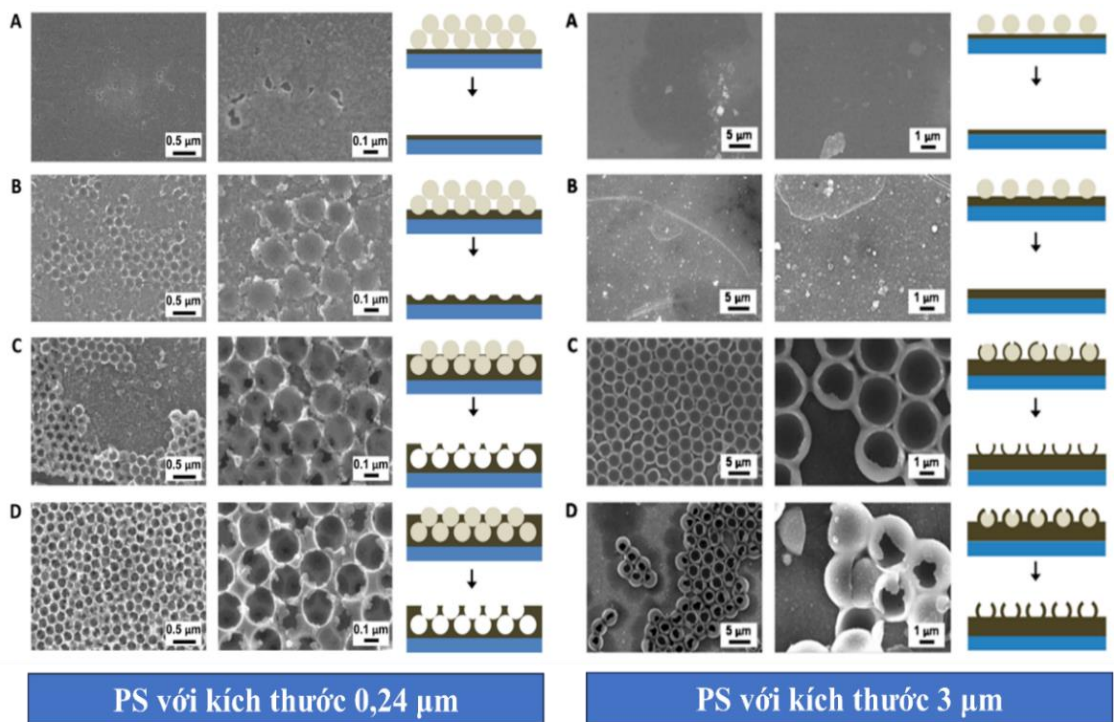
Hình 1.14. Ảnh SEM của màng \text{MoS}_x thu được sau khi loại bỏ PS trong toluen. Màng \text{MoS}_x được lắng đọng trên điện cực ITO trong 0 lần quét CV (A), 10 lần quét CV (B) [88].
