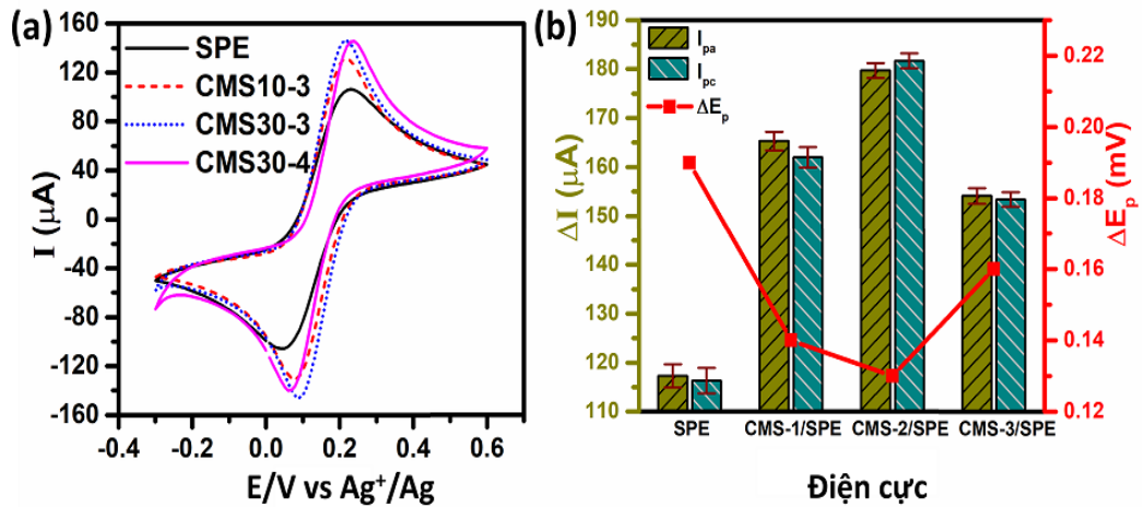
Hình 3.24. Đường CV (a), đồ thị hình cột so sánh cường độ dòng oxi hóa và khử (b), của điện cực SPE, CMS10-3/SPE, CMS30-3/SPE, và CMS30-4/SPE trong dung dịch KCl 0,1 M chứa [\text{Fe}(\text{CN})_6]^{3-/4-} 5 mM với tốc độ quét 50 \text{ mV s}^{-1} .
