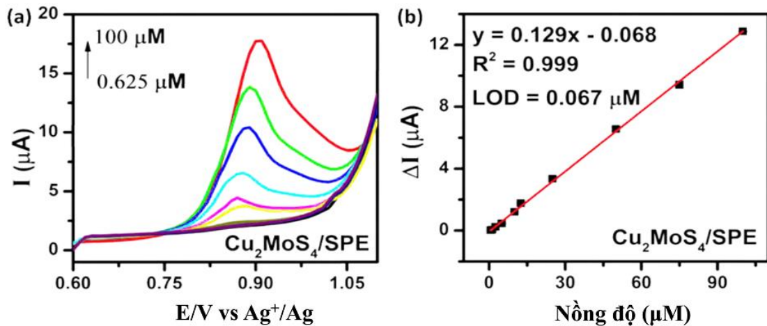
Hình 3.32. Đường DPV (a) và đường chuẩn biểu diễn mối liên quan giữa cường độ dòng đỉnh và nồng độ OFX (b) của \text{Cu}_2\text{MoS}_4/\text{SPE} trong dung dịch PBS 0,1M (pH = 4,0) có chứa OFX với nồng độ thay đổi từ 0,625 đến 100 \mu\text{M} .
