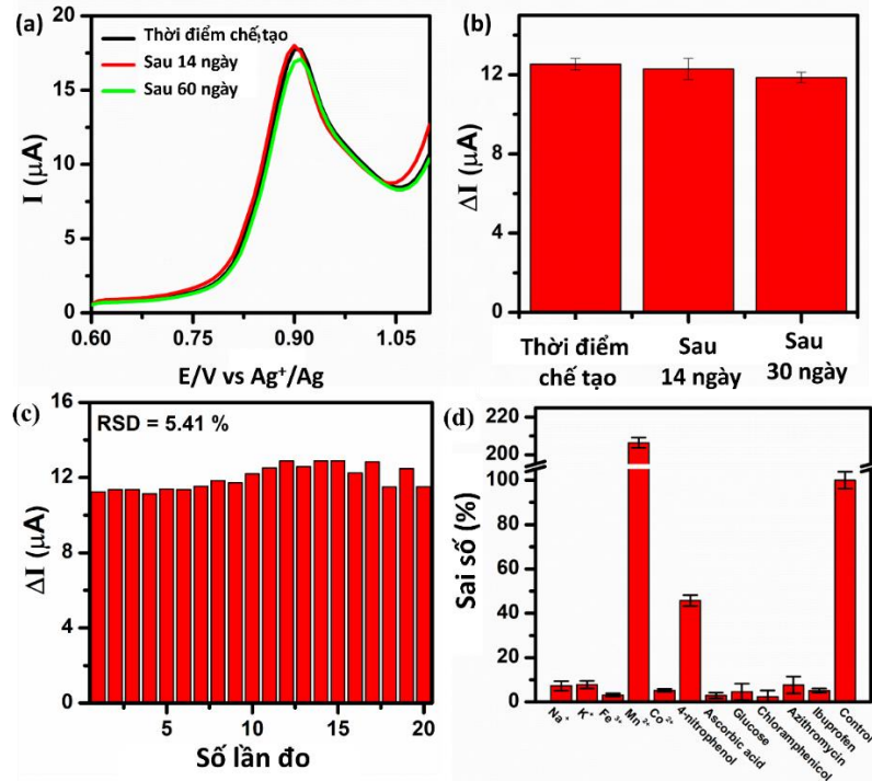
Hình 3.42. Độ ổn định (a, b), độ lặp lại (c), và độ chọn lọc (d) của cảm biến điện hóa của điện cực CMS30-4/SPE trong dung dịch PBS 0,1 M (pH = 6,0) có chứa PAR 100 \mu\text{M} .
