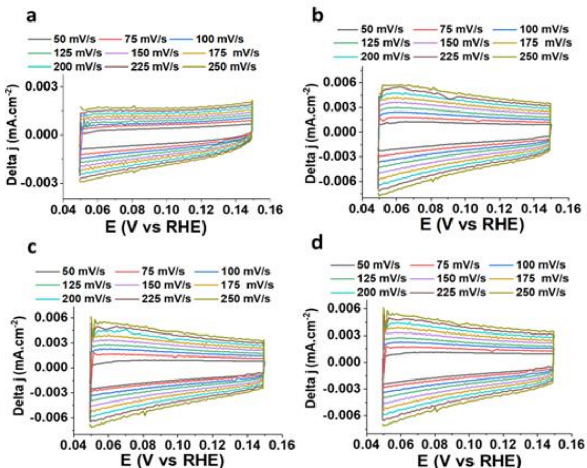
Hình 9. Đường CV ghi lại ở các tốc độ quét khác nhau trong vùng dòng điện dung trên các điện cực: 3D-MoS x 3,53 mC/cm 2 /FTO (a); MoS x 3,53 mC/cm 2 /FTO (b); 3D-MoS x 10,95 mC/cm 2 /FTO (c); và 3D-MoS x 17,75 mC/cm 2 /FTO (d), trong dung dịch H 2 SO 4 0,5 M (pH = 0,3).
