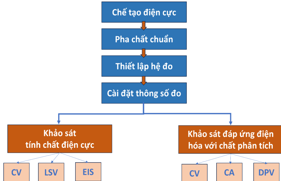
Hình 2.4. Quy trình tổng quát đo cảm biến điện hóa dựa trên vật liệu nano ứng dụng trong phân tích dược phẩm và thực phẩm
