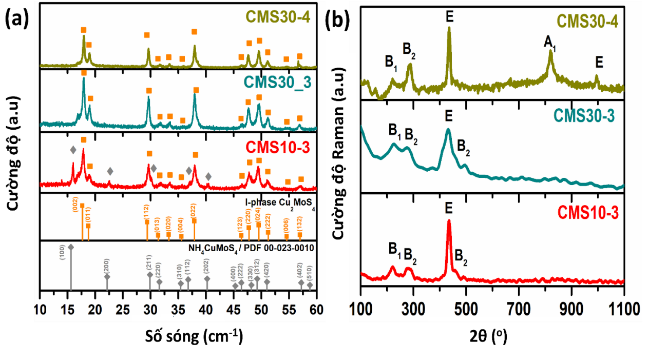
Hình 3.22. Giải đồ nhiễu xạ tia X (a) và phổ Raman của các mẫu CMS (b) của các mẫu vật liệu CMS.
