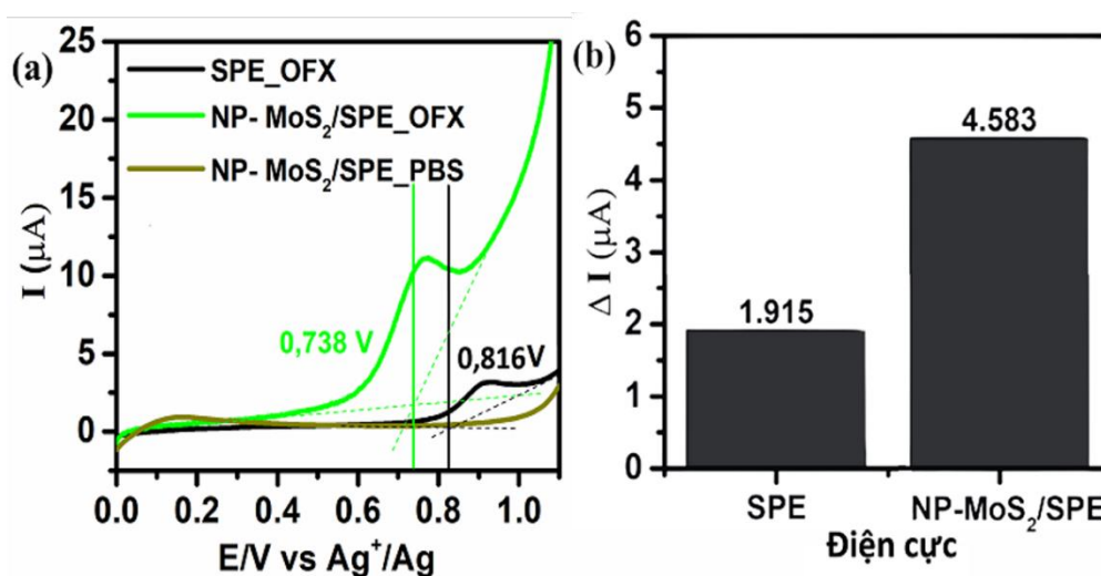
Hình 3.7. Kết quả đo LSV (a) và biểu đồ hình cột so sánh dòng oxi hóa OFX của điện cực SPE và NP-MoS 2 /SPE (b) trong dung dịch PBS (pH = 7,0) có bổ sung OFX 100 \mu M với tốc độ quét 10 mV/s.
