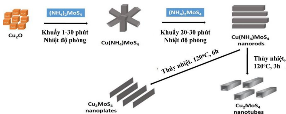
Hình 1.16. Sơ đồ quy trình chế tạo vật liệu CMS [103].
