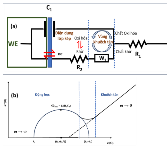
Hình 2.11. Mô hình mạch điện tương đương Randles (a) và giản đồ Nyquist (b) mô phỏng tính chất điện hóa của hệ điện cực trong dung dịch điện ly có cặp chất oxi hóa khử [117].
