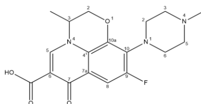
Hình 1.2. Cấu trúc của ofloxacin.
