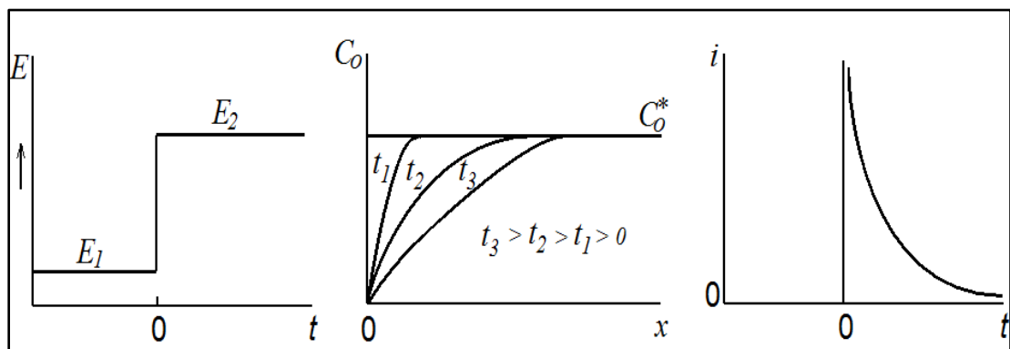
Hình 2.10. Bước nhảy điện thế (a), sự suy giảm nồng độ chất hoạt động điện hóa (b), và sự phụ thuộc của dòng điện đo được theo thời gian (c) [116].
