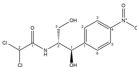
Hình 1.1. Cấu trúc chloramphenicol.
