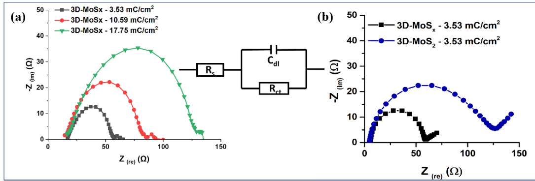
Hình 11. Phổ tổng trở ghi nhận trên các điện cực 3D-MoS x (3,53 – 17,75 mC/cm 2 ) (a), 3D-MoS x và 3D-MoS 2 (3,53 mC/cm 2 ) (b) trong môi trường H 2 SO 4 0.5M (-0.4 V với RHE) và mạch điện tương đương Randles áp dụng cho hệ.
