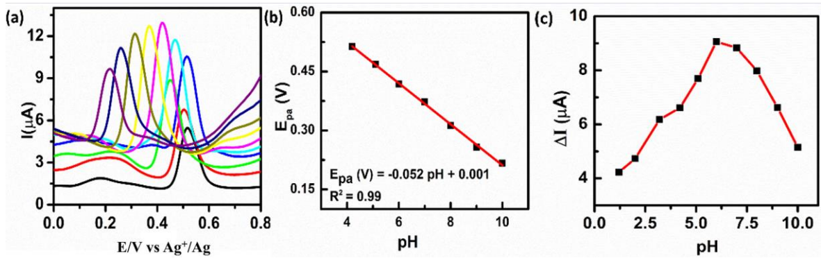
Hình 3.40. Khảo sát ảnh hưởng của pH tới tín hiệu phát hiện PAR của cảm biến điện hóa trên cơ sở vật liệu CMS30-4.
