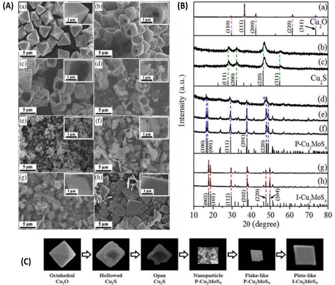
Hình 1.15. Ảnh SEM (A), giản đồ XRD (B) của tinh thể \text{Cu}_2\text{O} (a), của sản phẩm \text{Cu}_2\text{S} và CMS với các nồng độ \text{C}_2\text{H}_5\text{NS} khác nhau (b,h), và sơ đồ minh họa sự tiến hóa hình thái của \text{Cu}_2\text{S} và CMS từ mẫu \text{Cu}_2\text{O} bát diện (C) [104].
