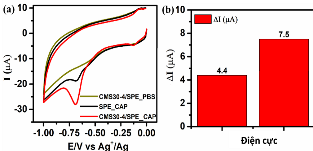
Hình 3.34. a) Đường cong CV của điện cực CMS30-4/SPE và điện cực SPE trong dung dịch PBS 0.1 M (pH = 5,0) bổ sung thêm CAP 100 \mu M, biểu đồ cột biểu diễn tín hiệu cường độ dòng đỉnh khử CAP.
