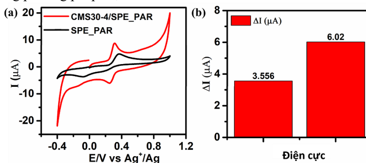
Hình 3.23. Đường CV a) và biểu đồ hình cột tín hiệu b) của các điện cực SPE và CMS30-4/SPE đối với PAR trong dung dịch PBS (pH = 7,4) chứa PAR 100 \mu\text{M} .
