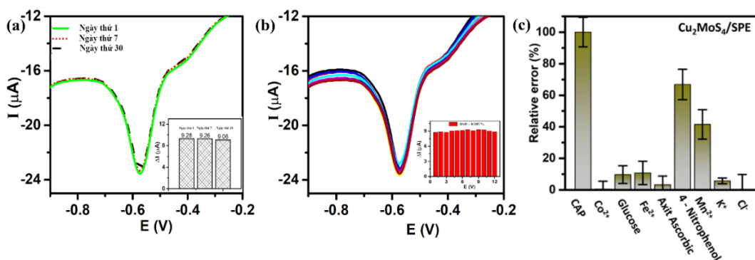
Hình 3.22: Đường DPV khảo sát độ ổn định (a), độ lặp lại (b), và độ chọn lọc (c) của điện cực CMS30-4/SPE trong dung dịch PBS 0,1M (pH = 5,0) có chứa CAP với nồng độ 100 \mu\text{M} .
