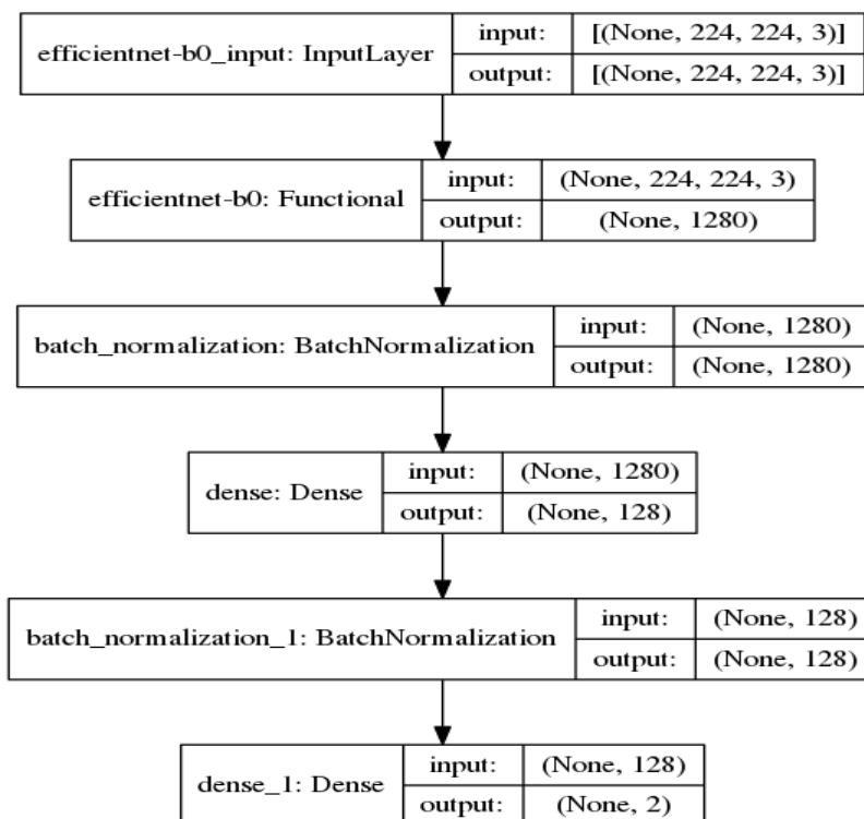
Hình 3. 10. Kiến trúc mạng EfficientNet(B0) cho trích chọn đặc trưng
