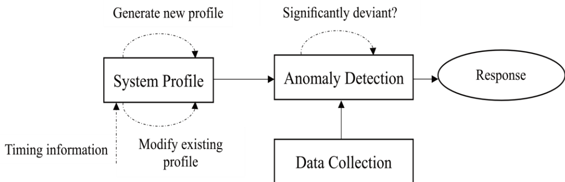
Hình 1. 7. Mô hình phương pháp phát hiện xâm nhập dựa trên bất thường
