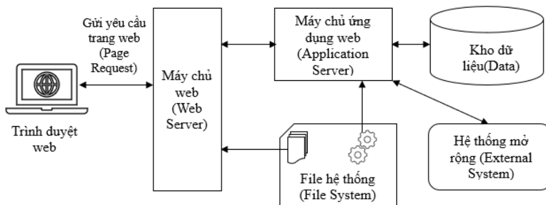
Hình 1. 1. Kiến trúc chuẩn của ứng dụng web [31]
