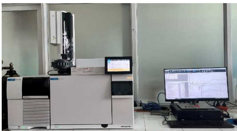
Hình 2.5. Bộ Thiết bị sắc ký khí GC-MS
