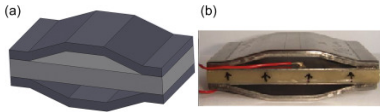
Hình 1.4 Kết cấu PEH kiểu chũm chọe, [3]
