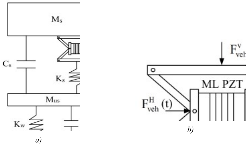
Hình 1.24 Thu thập năng lượng áp điện cho hệ thống treo với khung khuếch đại lực của Hendrowati và cộng sự, [105].
