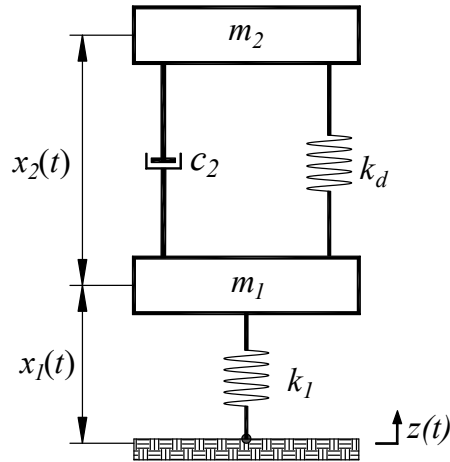
Hình 2.1 Mô hình kết cấu chính không cân với TMD chịu kích động nền
