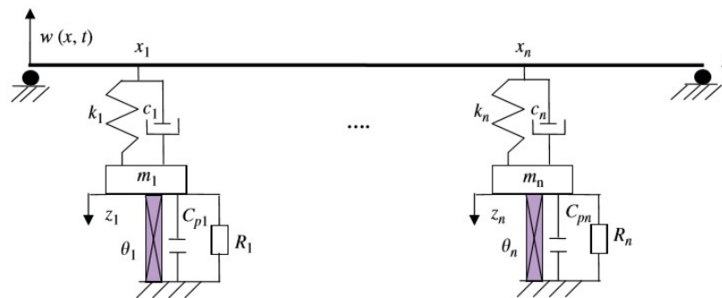
Hình 1.20 Mô hình TMD-PSEH gắn với dầm dao động của Ouled Chtiba và cộng sự, [102].
