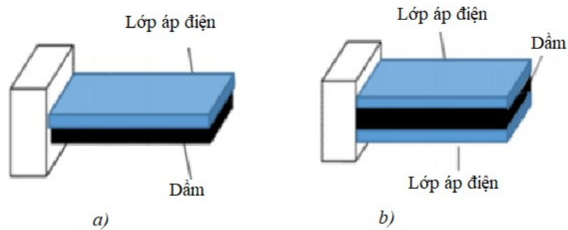
Hình 1.3 Kết cấu bộ PEH kiểu dầm công xôn dán 1 lớp và 2 lớp áp điện, [2]
