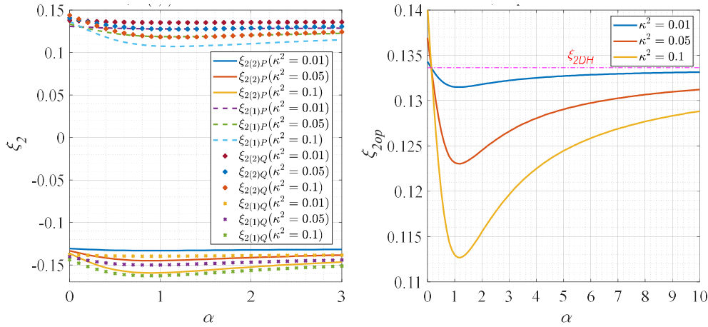
Hình 3.5 Đồ thị hệ số cản theo biến \alpha của hệ chịu kích động ngoài
