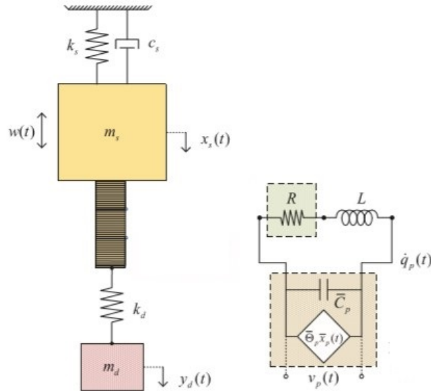
Hình 1.22 Mô hình TMD-PSEH không cân gắn với kết cấu chính có cân của Lai và cộng sự, [75].
