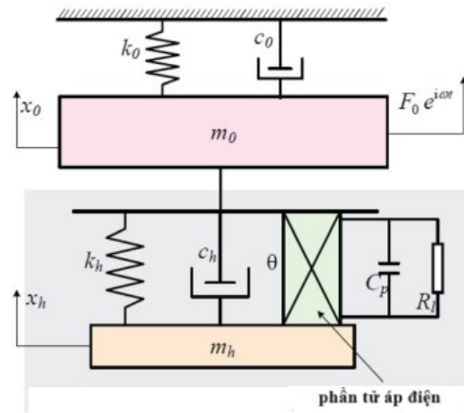
Hình 1.15 Mô hình DVA-PEH gắn trên kết cấu chính có cản của Ali và Adhikari, [98].
