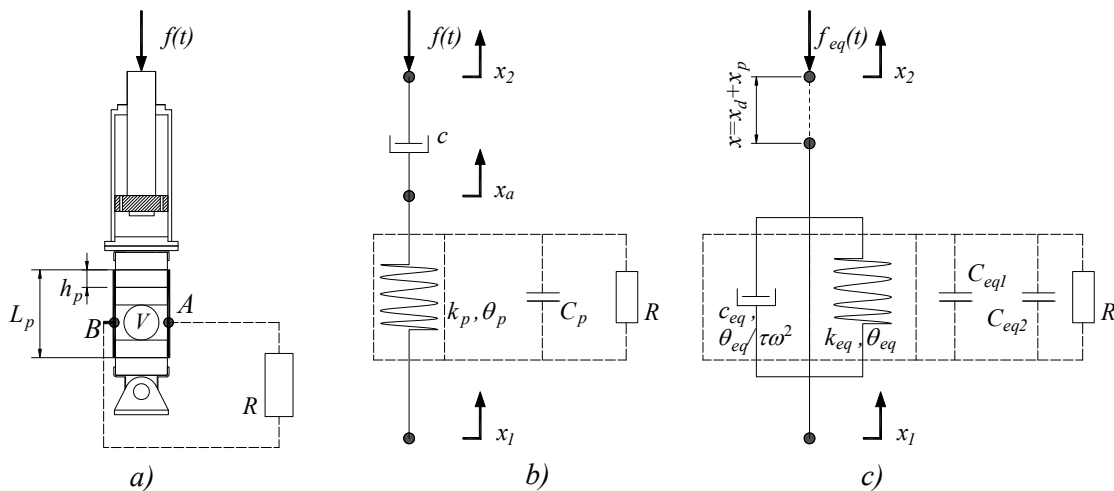
Hình 2.7 Mô hình của PSEH lắp nối tiếp với cản
