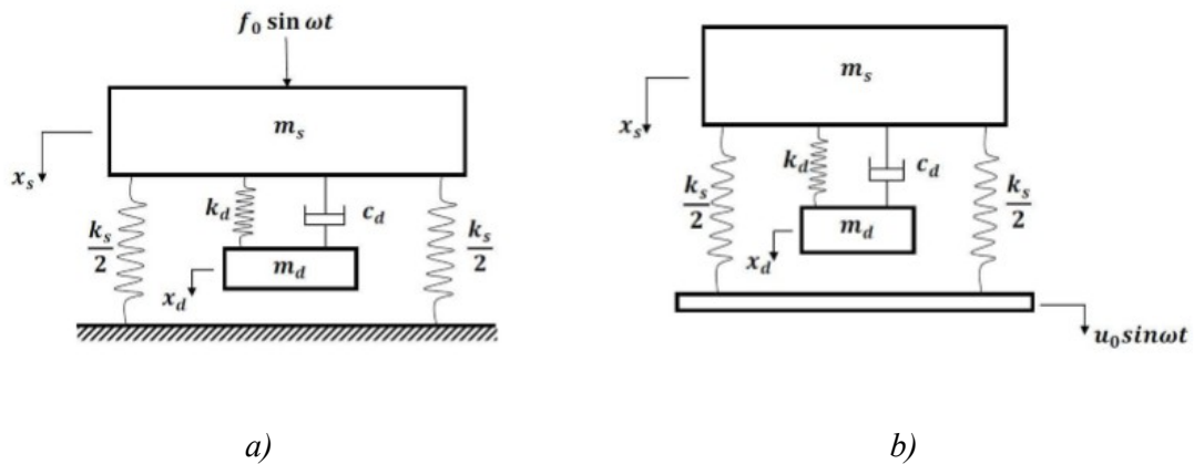
Hình 1.14 Hai kiểu mô hình bộ giảm chấn khối lượng lắp trên kết cấu chính không cân [82]-[84]
