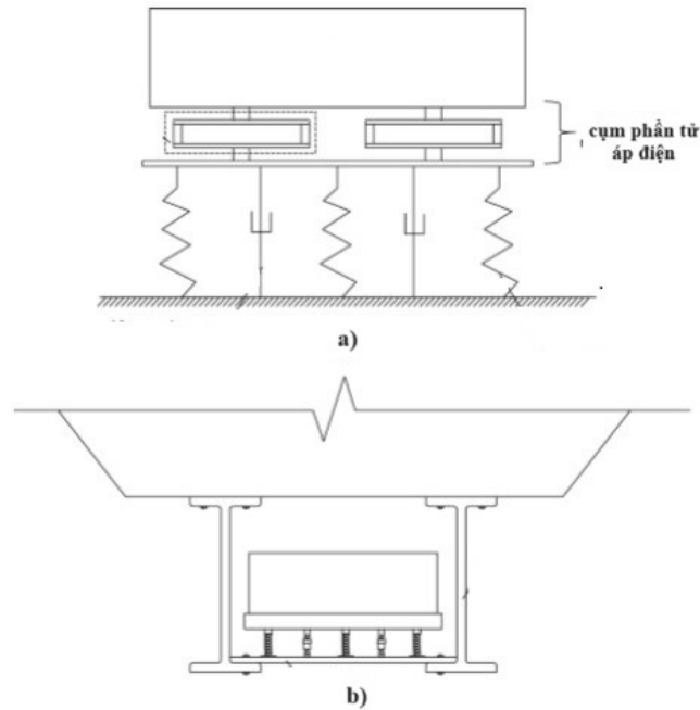
Hình 1.21 Mô hình TMD-PEH với PEH gắn nối tiếp với hệ lò xo và cản trong TMD của Pan và cộng sự, [103].
