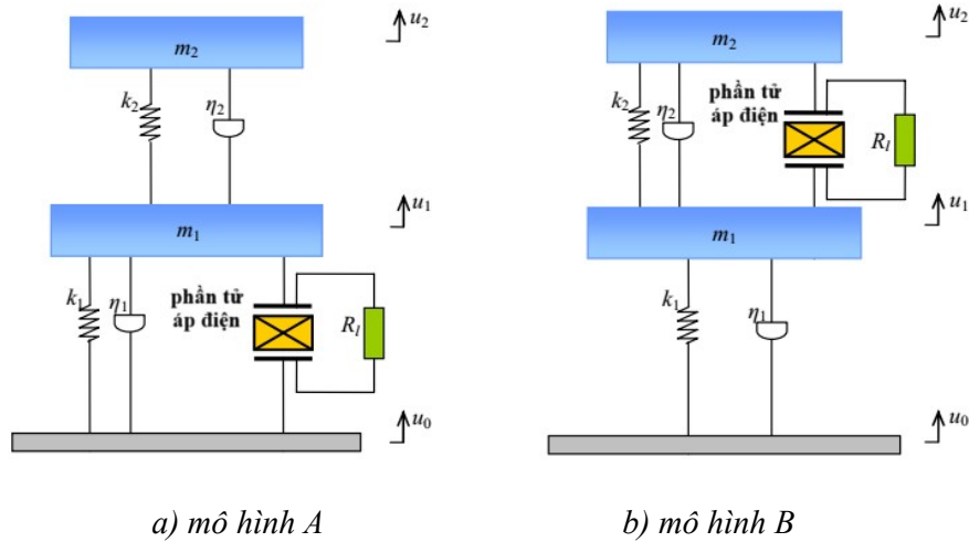
Hình 1.10 Hai kiểu mô hình thu thập năng lượng áp điện của hệ cơ học 2 bậc tự do chịu kích động nền, [72]
