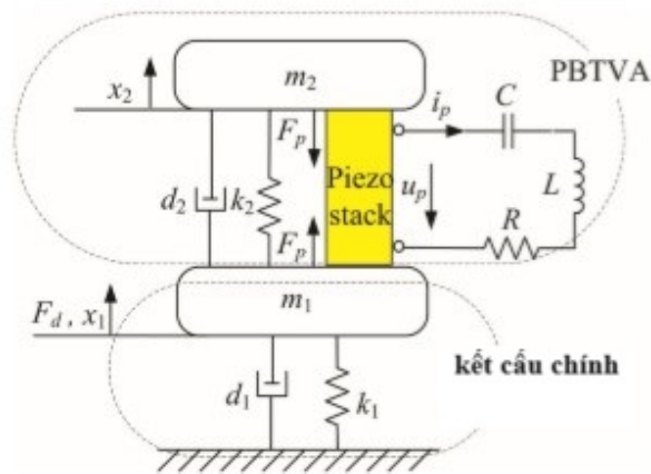
Hình 1.17 Mô hình DVA-PEH gắn trên kết cấu chính có cân của Zhao và cộng sự, [100].
