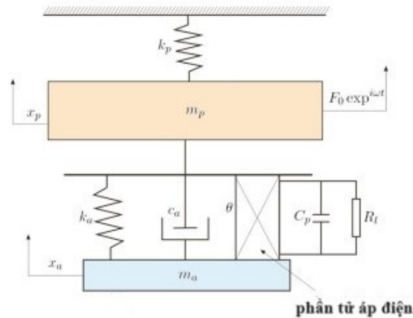
Hình 1.16 Mô hình DVA-PEH gắn trên kết cấu chính không cản của Zuppa và cộng sự, [99].
