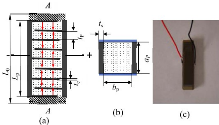
Hình 1.5 Kết cấu PEH kiểu xếp chồng, [3]
