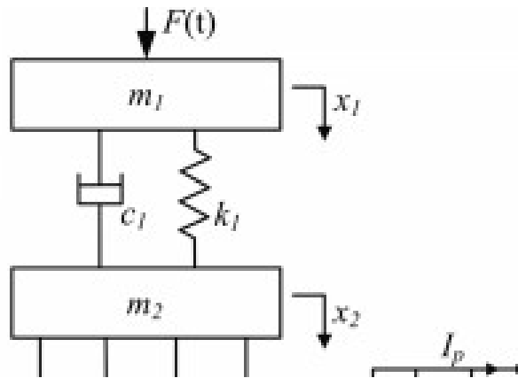
Hình 1.13 Mô hình hệ thống thu thập năng lượng áp điện từ rung động nền đường, [73]
