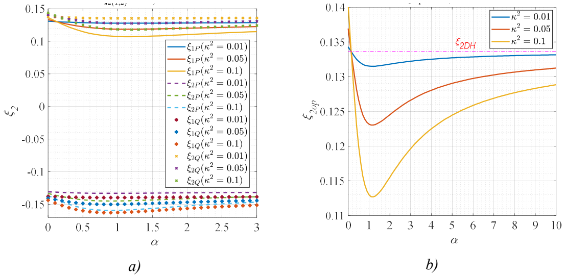
Hình 3.2 Đồ thị hệ số cản theo biến \alpha của hệ chịu kích động nền
