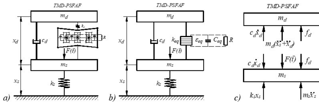
Hình 3.6 Mô hình kết cấu chính không cân với bộ thu thập năng lượng xếp chồng kết hợp khung khuếch đại lực kép
