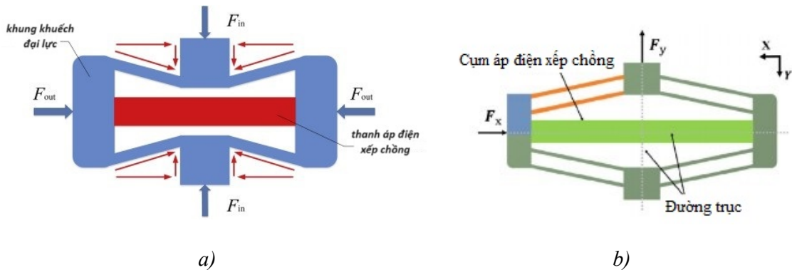
Hình 1.6 Cấu trúc cụm áp điện kiểu xếp chồng với khung khuếch đại lực, [6]
