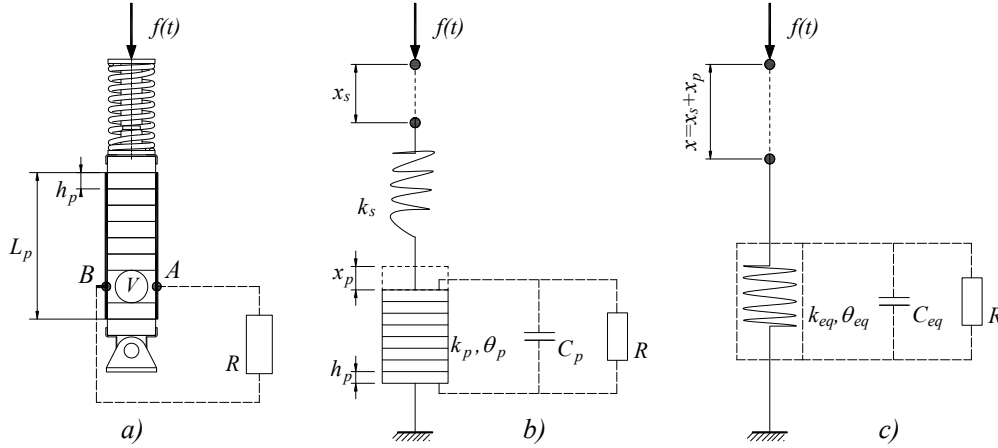
Hình 2.6 Mô hình của PSEH lắp nối tiếp với lò xo a) sơ đồ cấu tạo, b) mô hình cơ điện, c) mô hình tương đương.
