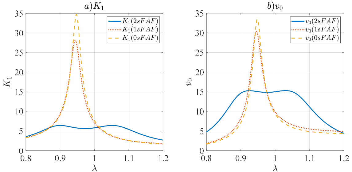
Hình 4.11 Đồ thị K_1, v_0 theo biến \lambda với \mu=0.05, \kappa^2=0.0242, \alpha=1 và k_d=0.946k_{adh} trong những trường hợp khác nhau
