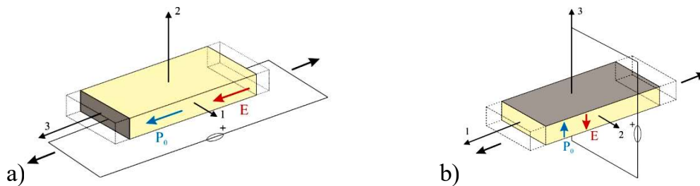
Hình 1. 2 Các kiểu hiệu ứng áp điện phân cực theo trục 3, [2]
