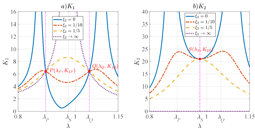
Hình 3.4 Các điểm cố định của đường cong hệ số khuếch đại của hệ kết cấu chính không cản với TMD-PSEH chịu kích động ngoài
