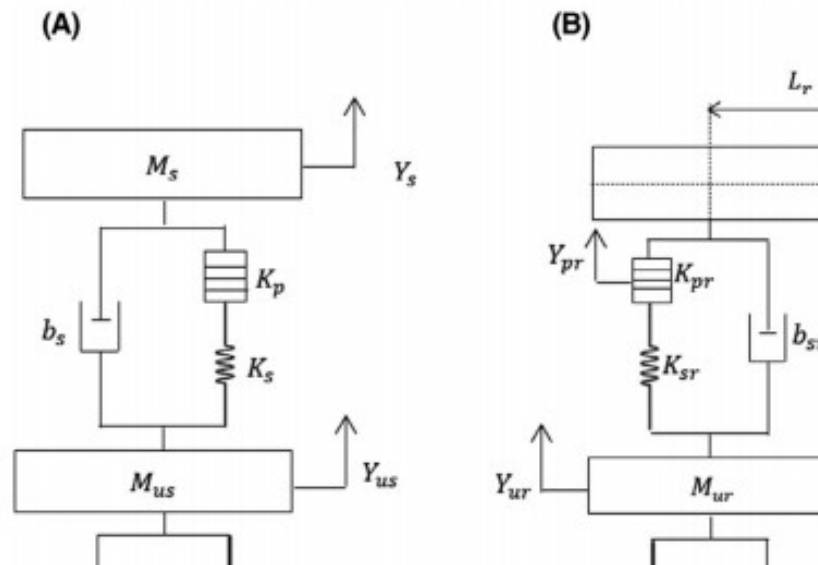
Hình 1.23 Mô hình thu thập năng lượng trên hệ thống treo của ô tô với phần tử áp điện kiểu xếp chồng lắp nối tiếp với lò xo của Al-Yafeai và cộng sự, [104].
