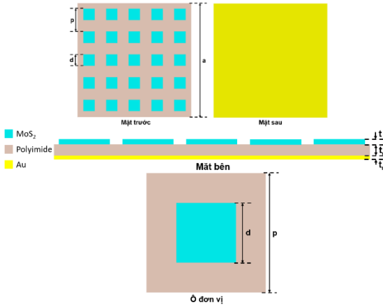
Hình 4.10. Mô hình vật liệu MPA-2DP tích hợp vật liệu MoS 2
