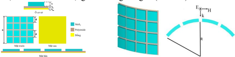
Hình 4.1. Minh họa cấu trúc ô cơ sở và trạng thái đàn hồi của MPA-2DP.
