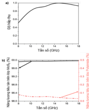
Hình 4.3. (a) Phổ hấp thụ của MPA-2DP đề xuất, (b) tỉ lệ năng lượng tiêu tán trong các lớp cấu trúc của vật liệu.
