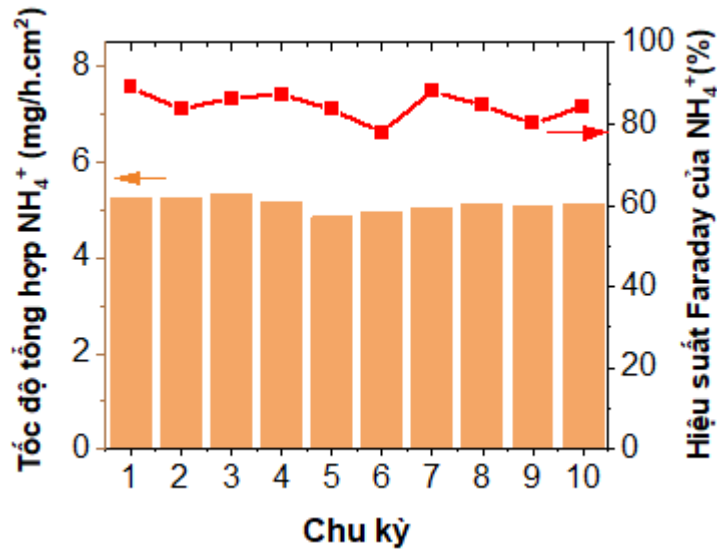
Hình 3.22. Tốc độ tổng hợp NH 4 + và hiệu suất Faraday NH 4 + của điện cực Cu-nanosphere đối với NO 3 RR ở -1,3 V trong dung dịch Na 2 SO 4 0,5 M + NaNO 3 0,1 M.
