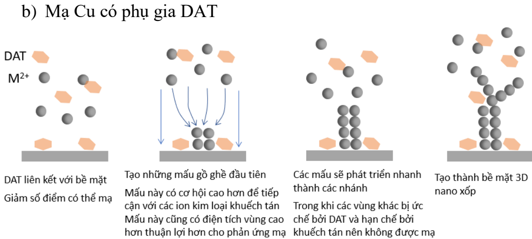
Hình 1.20. Cơ chế đề xuất quá trình mạ Cu a) Không có phụ gia DAT; b) Có phụ gia DAT [122].
