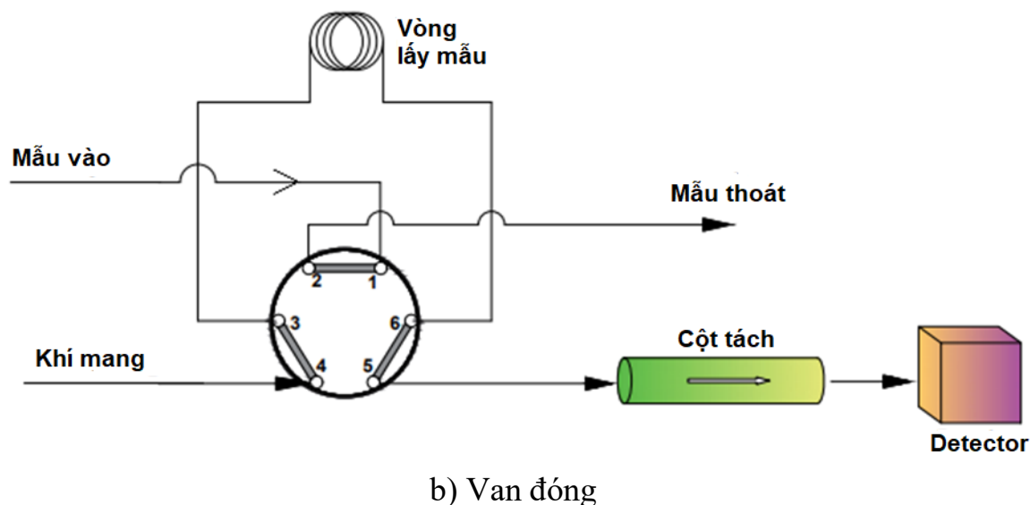
Hình 3.8. Sơ đồ bộ lấy mẫu ở trạng thái a) Van mở, và b) Van đóng.
