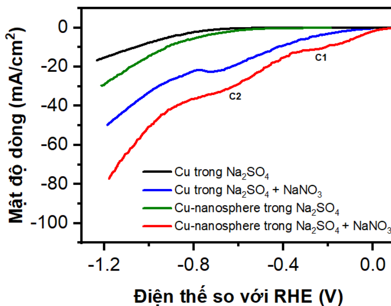
Hình 3.6. Đường quét thế tuyến tính LSV trong \text{Na}_2\text{SO}_4 có và không có \text{NaNO}_3 của điện cực Cu và Cu-nanosphere.
