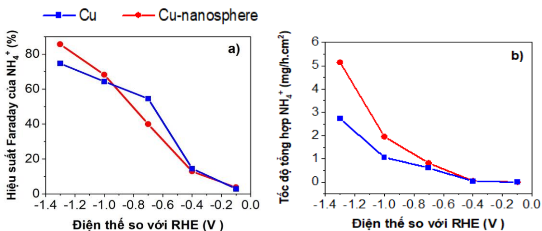
Hình 3.21. a) Hiệu suất Faraday (FE) của sự hình thành NH 4 + ; b) Tốc độ tổng hợp NH 4 + của Cu-nanosphere của NO 3 RR ở các thế khác nhau trong dung dịch Na 2 SO 4 0,5 M + NaNO 3 0,1 M.
