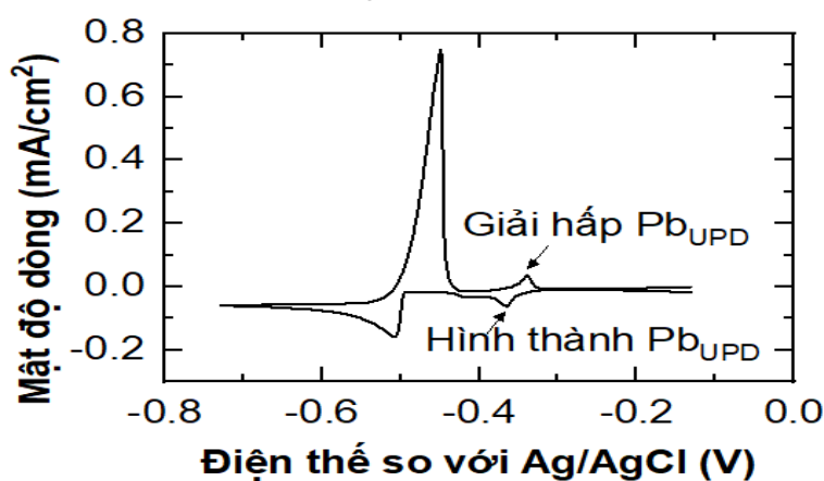
Hình 3.5. Đường cong CV của Pb trên nền Cu đa tinh thể trong dung dịch \text{HClO}_4 100 mM + \text{Pb}(\text{ClO}_4)_2 1 mM + KCl 20 mM.
