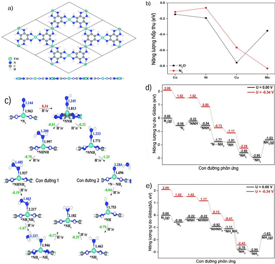
Hình 1.16. a) Mặt trên và mặt bên của MOF 2D. b) Năng lượng hấp phụ của các phân tử N_2 và H_2O trên các MOF khác nhau. c) Các mặt nhìn của các chất trung gian ở mỗi bước hydrogen hóa thông qua cả cơ chế xa (Con đường 1) và xen kẽ (Con đường 2) của NRR. d-e) Năng lượng tự do Gibbs của NRR trên MOF dựa trên Mo không có năng lượng đầu vào (màu đen) và điện thế ứng dụng (màu đỏ) có giá trị được xác định bằng cách giới hạn điện thế thông qua d) cơ chế xa và e) xen kẽ [103].
