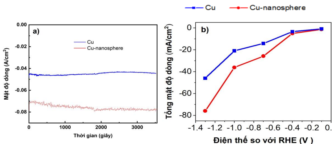
Hình 3.7. a) Đường dòng điện – thời gian CA của điện cực Cu và Cu-nanosphere trong dung dịch \text{Na}_2\text{SO}_4 0,5 M + \text{NaNO}_3 0,1 M tại thế khử -1,3 V vs. RHE; b) Tổng mật độ dòng của điện cực Cu và Cu-nanosphere tại các thế khác nhau.
