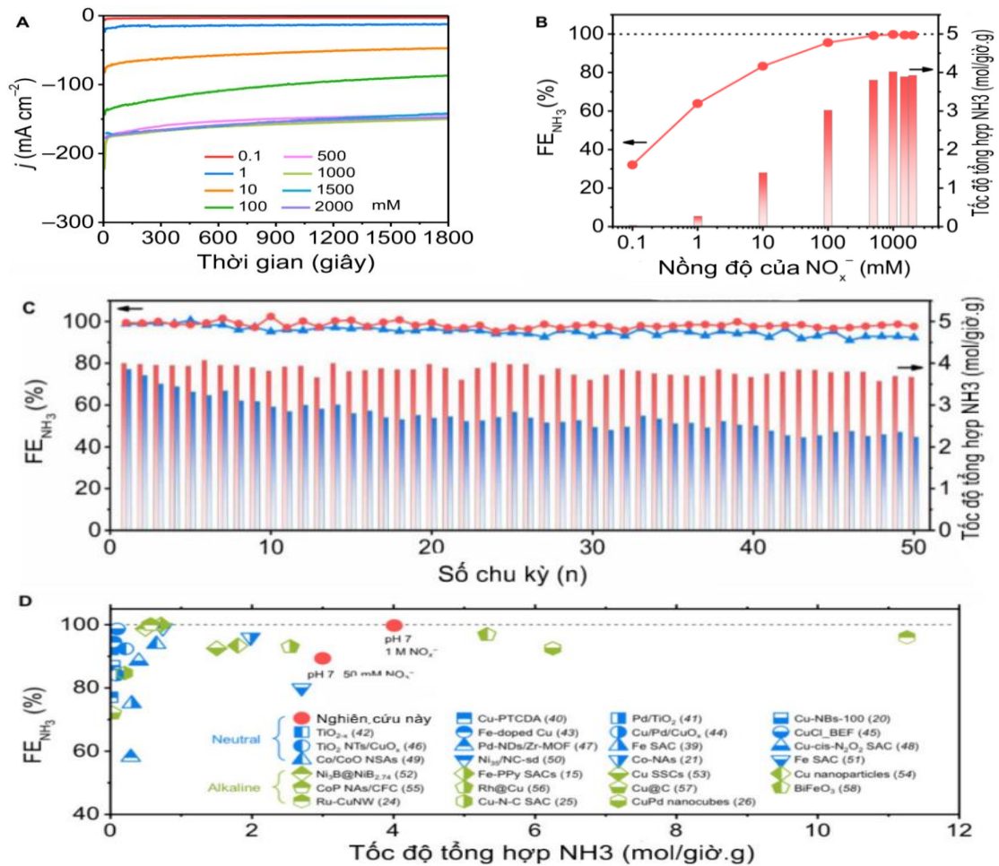
Hình 1.29. Hiệu suất phản ứng khử điện hóa nitrate thành \text{NH}_3 của Cu@hNCNC với các nồng độ \text{NO}_x^- khác nhau ở thế -1,5 V trong chất điện phân trung tính (pH = 7). (A) Đường cong i - t ; (B) Hiệu suất Faraday và tốc độ tạo ra \text{NH}_3 ; (C) độ ổn định điện xúc tác của Cu@hNCNC (màu đỏ) trong
