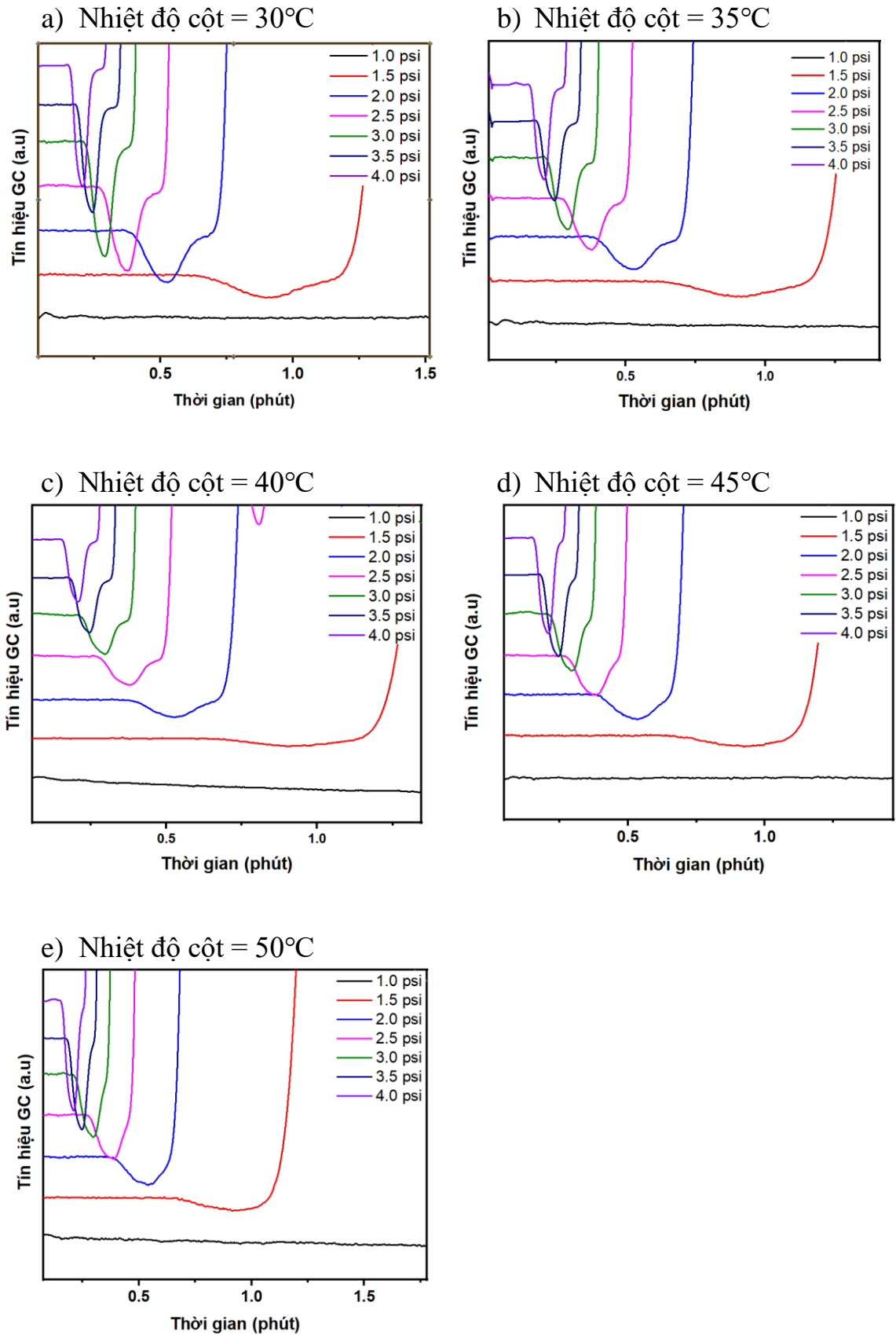
Hình 3.12. Sắc ký đồ GC của H 2 ở các áp suất cột khác nhau tại cùng một điều kiện nhiệt độ cột.
