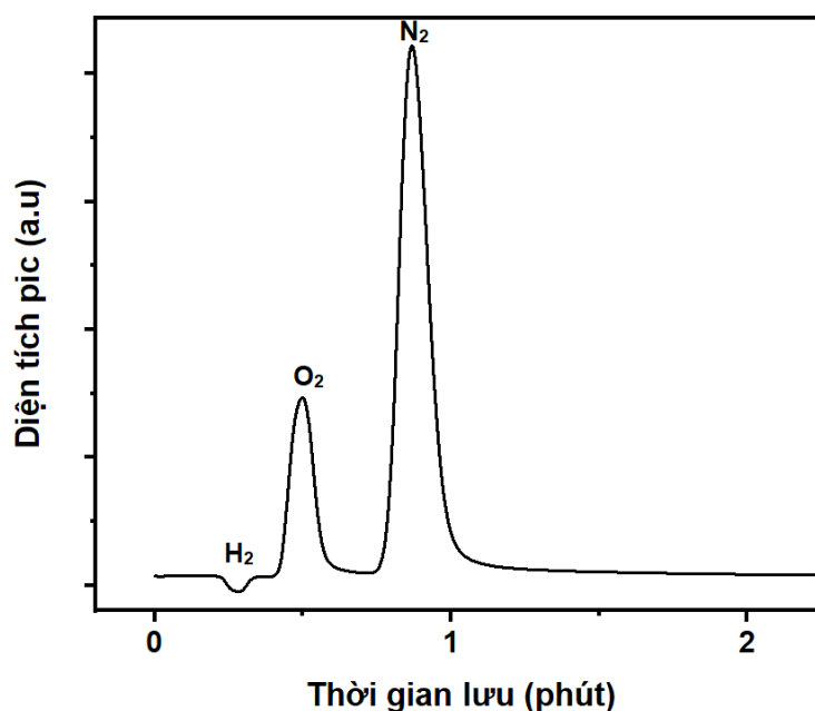
Hình 3.10. Sắc ký đồ của khí H 2 .
