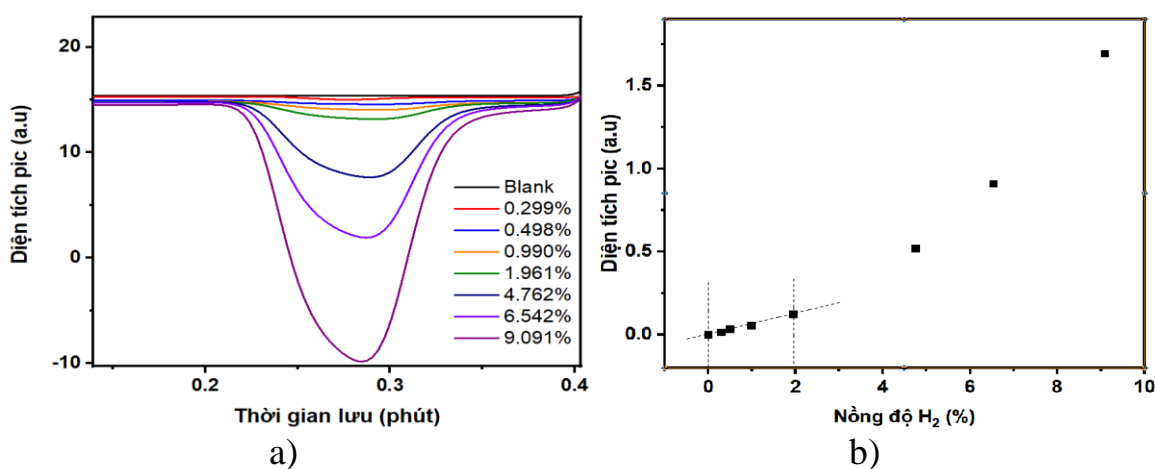
Hình 3.13. a) Sắc ký đồ GC của khí H 2 ở các nồng độ khác nhau; b) Khảo sát khoảng tuyến tính của phương pháp phân tích H 2 .
