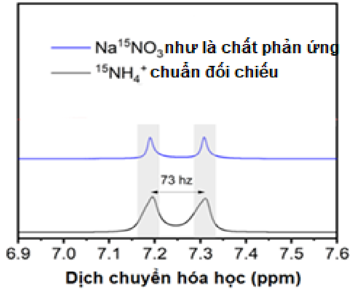
Hình 3.23. Phổ ^1\text{H} -NMR (600 MHz, DMSO- d_6 ) của ^{15}\text{NH}_4^+ được tạo ra từ \text{NO}_3\text{RR} sử dụng \text{Na}^{15}\text{NO}_3 làm chất phản ứng.
