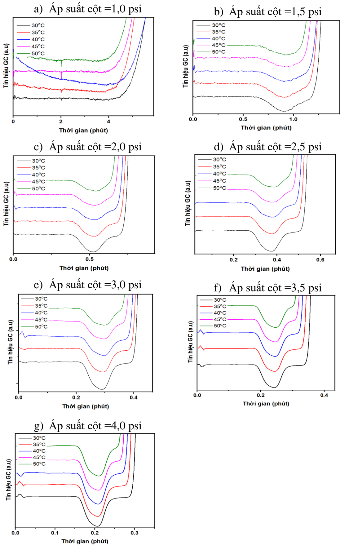
Hình 3.11. Sắc ký đồ GC của H 2 ở các nhiệt độ cột khác nhau tại cùng một điều kiện áp suất cột.
