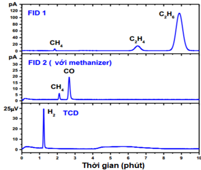
Hình 1.27. Tập hợp các sắc ký đồ đại diện của các sản phẩm ở thể khí sinh ra trong quá trình khử \text{CO}_2 . Điện thế áp dụng -1,0\text{ V} [170].
