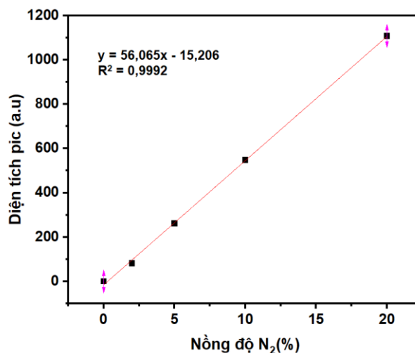
Hình 3.18. Đường chuẩn N 2 sau khi trừ nền trực tiếp pic N 2 mẫu = pic N 2 đo được – pic N 2 nền.
