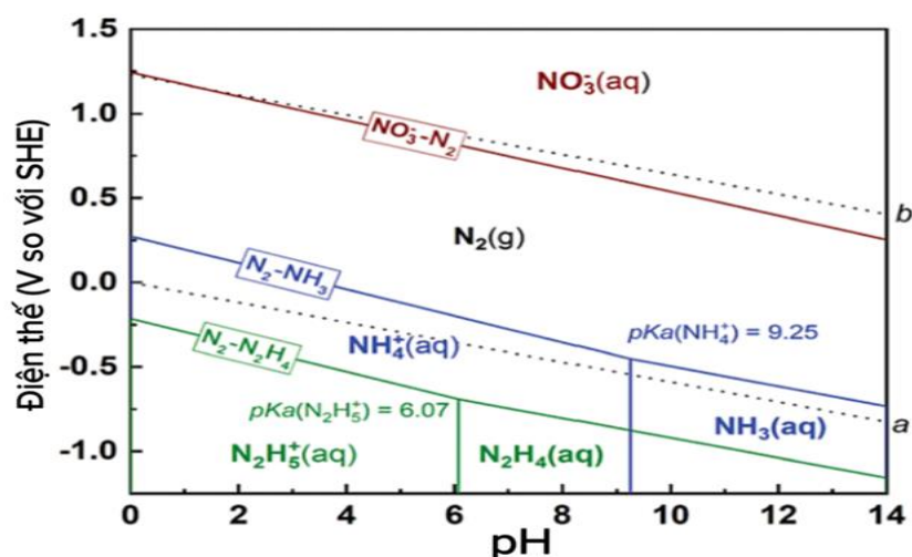
Hình 1.3. Biểu đồ Pourbaix của hệ \text{N}_2\text{-H}_2\text{O} và các sản phẩm nitrogen. Đường liền tương ứng với các phản ứng oxi hoá khử giữa \text{NO}_3^- , \text{N}_2 , \text{NH}_3 , và \text{NH}_4^+ . Vùng giữa đường kẻ đứt a (HOR/HER) và b (OER/ORR) là trạng thái nước bền [27-29].
