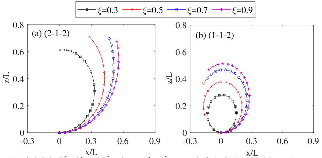
Hình 2.24. Cầu hình biến dạng của dầm sandwich CNTRC chịu mô-men với các giá trị khác nhau của tham số kết tụ \xi ( L/h = 10 , V_{CNT} = 0.1 , \alpha_F = 0.4 , \zeta = 0.9 , (k_1, k_2) = (50, 0.5) ).
