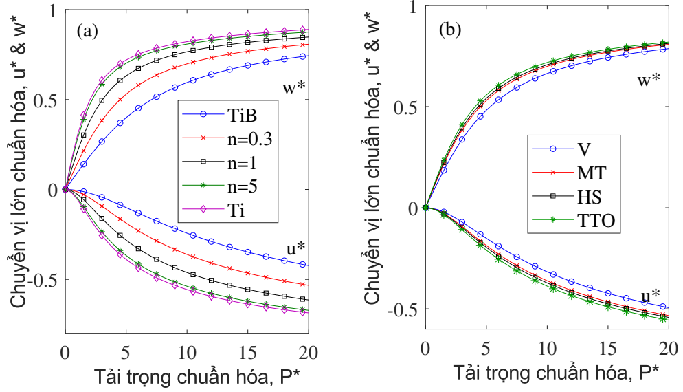
Hình 2.8. Đường cong tải-chuyển vị của đầm (2-1-2) loại A :
