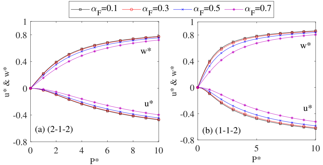
Hình 2.26. Ảnh hưởng của tham số nền đàn hồi \alpha_F tới chuyển vị lớn của dầm CNTRC chịu tải P ( L/h = 10 , \alpha_F = 0.4 , (\xi, \zeta) = (0.4, 0.7) , (k_1, k_2) = (50, 0.5) ).
