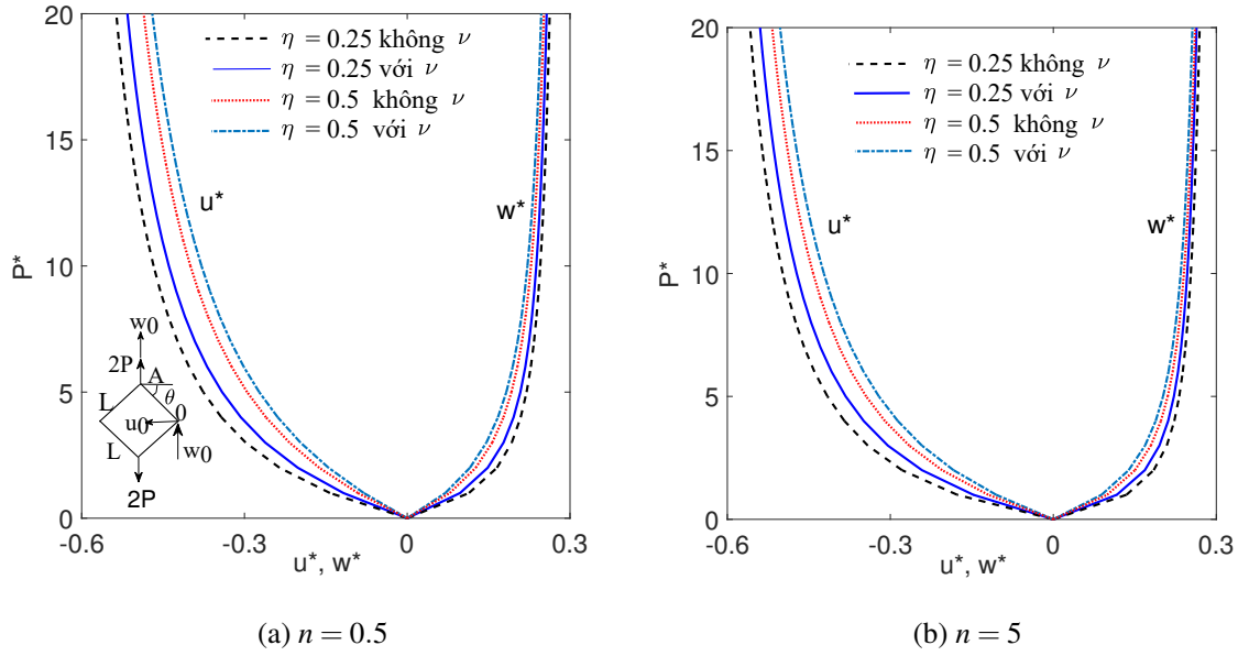
Hình 3.19. Đường cong tải-chuyển vị của khung FGM hình vuông kích thước micro chịu tải trọng kéo với các giá trị khác nhau của tham số tỷ lệ.
