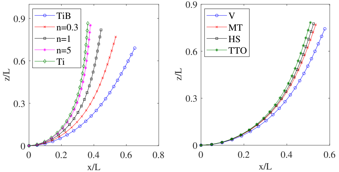
Hình 2.9. Cấu hình biến dạng của đầm loại A tương ứng với P^* = 5 : (a) Mô hình MT và n thay đổi; (b) n = 0.3 và các mô hình đồng nhất hóa khác nhau.
