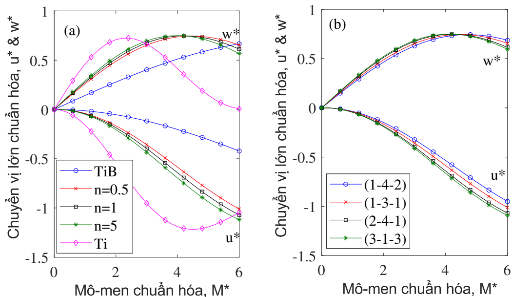
Hình 2.14. Đường cân bằng của đầm loại B chịu mô-men: (a) đầm (1-3-1) và n thay đổi; (b) n = 0.5 và tỉ số chiều dày các lớp khác nhau (mô hình MT).
