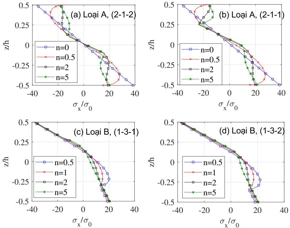
Hình 2.12. Ảnh hưởng của tham số vật liệu lên sự phân bố theo chiều cao của ứng suất dọc trục tại thiết diện ngàm của dầm FGSW với P^* = 15 .
