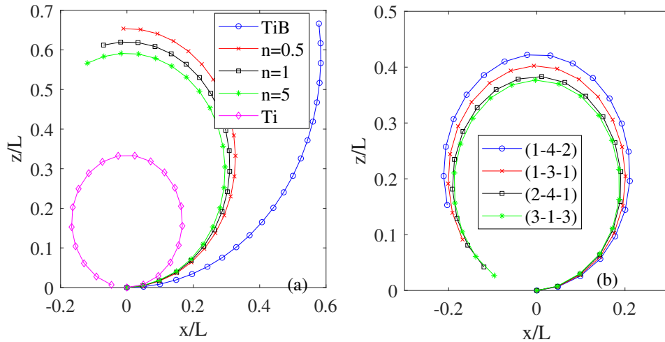
Hình 2.16. Cấu hình biến dạng của dầm loại B: (a) Dầm (2-1-2) và n thay đổi; (b) n = 0.5 , M^* = 10 và tỉ số chiều dày các lớp khác nhau.
