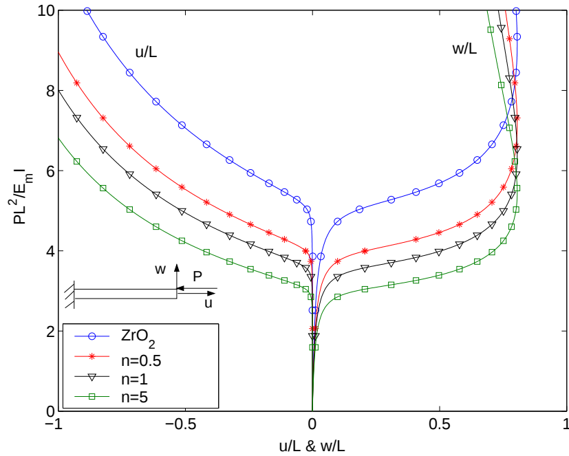
Hình 3.7. Đường cong tải-chuyển vị của dầm công-xôn \text{ZrO}_2/\text{Al} với các giá trị khác nhau của tham số vật liệu n .
