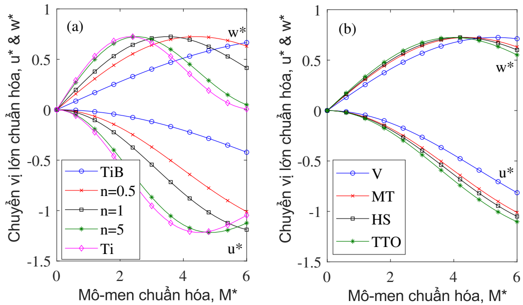
Hình 2.13. Đường cân bằng của đầm loại A (2-1-2) chịu mô-men: (a) mô hình MT và n thay đổi; (b) n = 0.5 và các mô hình đồng nhất hóa khác nhau.
