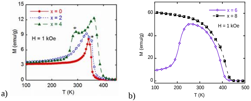
Hình 4.8. Đường M(T) của băng hợp kim Ni_{50-x}Co_xMn_{29}Ga_{21} với x = 0, 2, 4 (a) và x = 6, 8 (b) trong từ trường 1 kOe.
