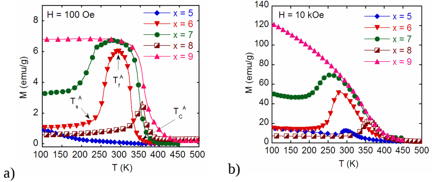
Hình 4.16. Các đường M(T) của băng hợp kim \text{Ni}_{50-x}\text{Co}_x\text{Mn}_{50-y}\text{Al}_y với y = 18 trong từ trường: 0,1 kOe (a) và 10 kOe (b).
