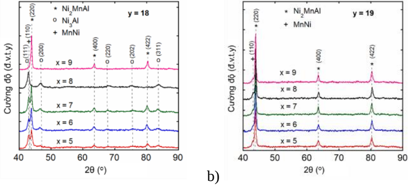
Hình 4.13. Giản đồ XRD của MSMA \text{Ni}_{50-x}\text{Co}_x\text{Mn}_{50-y}\text{Al}_y : y = 18 (a) và y = 19 (b).
