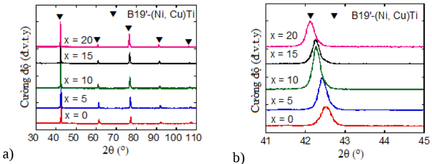
Hình 3.4. Giải đồ XRD của băng hợp kim \text{Ni}_{50-x}\text{Ti}_{50}\text{Cu}_x ( x = 0, 5, 10, 15 và 20 ) (a) và phần mở rộng của chúng với góc 2\theta trong khoảng 41-45^\circ (b).
