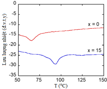
Hình 3.8. Đường cong DSC của SMA \text{Ni}_{50-x}\text{Ti}_{50}\text{Cu}_x với x = 0 và 15 khi nung nóng.
