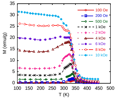
Hình 4.3. Đường M(T) của MSMA Ni_{50}Mn_{30}Ga_{20} ở các từ trường 0,1-10 kOe.
