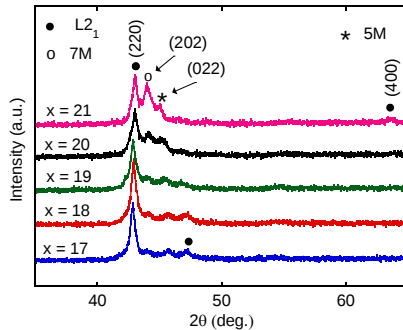
Hình 4.1. Giải đồ XRD của các MSMA Ni_{50}Mn_{50-x}Ga_x ( x = 17-21 ).
