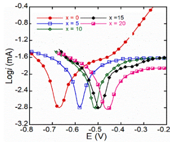
Hình 3.12. Đường cong phân cực anốt của SMA \text{Ni}_{50-x}\text{Ti}_{50}\text{Cu}_x ( x = 0, 5, 10, 15 và 20).
