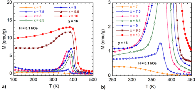
Hình 4.28. Đường M(T) của MSMA Ni_{50-x}Co_xMn_{35}Al_{15} với x = 7 - 10 và y = 16 trong từ trường 0,1 kOe (a) và vùng mở rộng xung quanh nhiệt độ chuyển pha (b).
