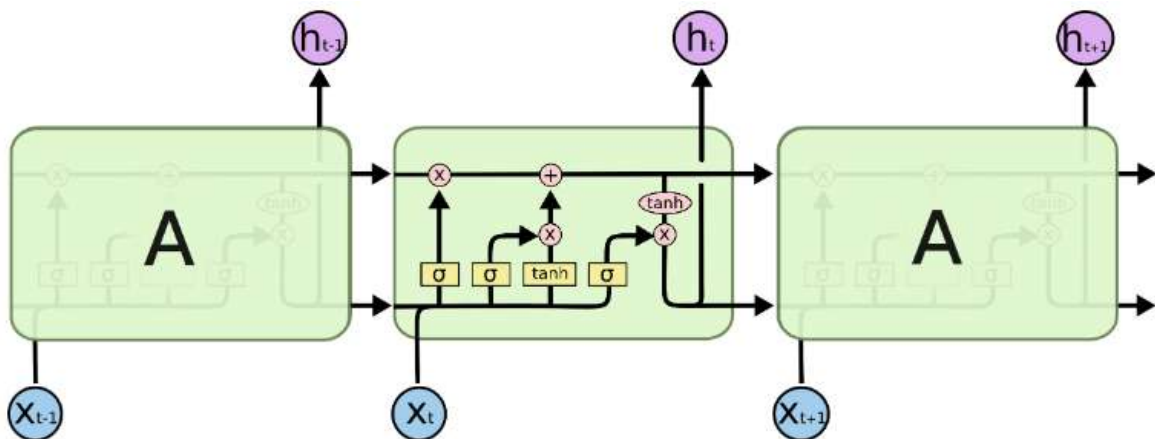
Hình 1.13. Sự lặp lại cấu trúc mô-đun trong mạng LSTM chứa bốn tầng ẩn (3 sigmoid và 1 tanh ) tương tác
