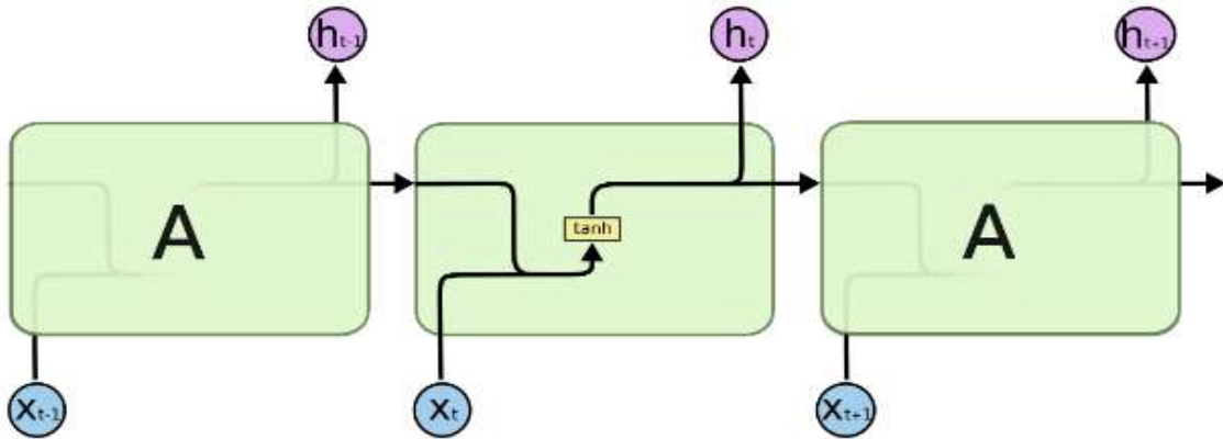
Hình 1.12. Sự lặp lại cấu trúc mô-đun trong mạng RNN chứa một tầng ẩn
