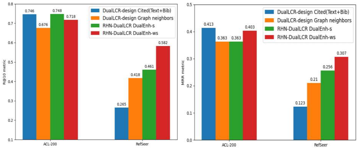
Hình 3.9. So sánh hiệu suất của các chiến lược lấy mẫu phù định của thiết kế DualLCR [13] với RHN-DualLCR
