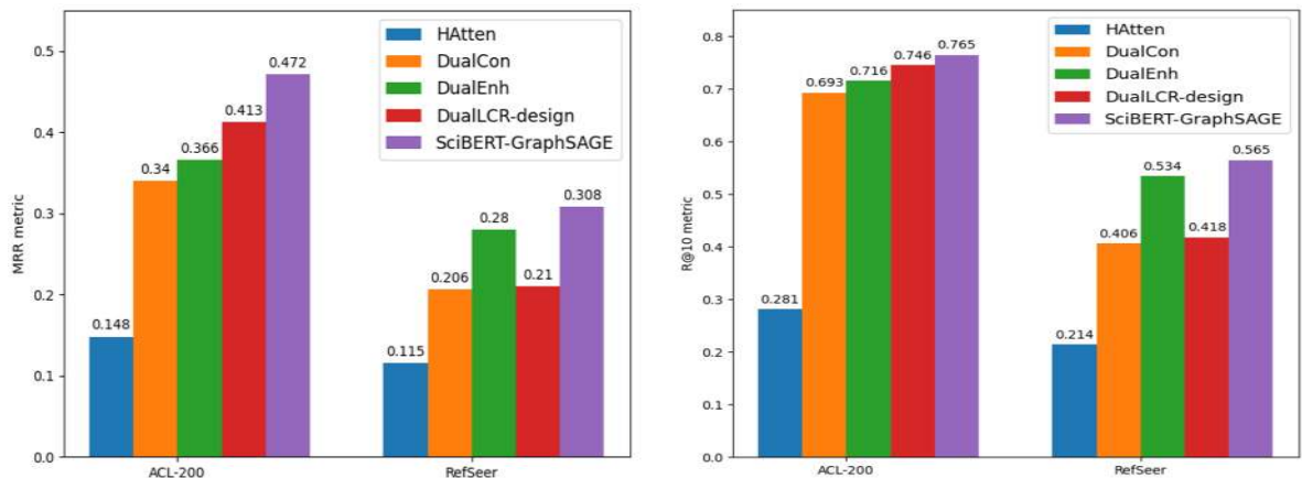
Hình 4.6. Kết quả so sánh hiệu năng của mô hình SciBERT-GraphSAGE với 4 mô hình tiên tiến nhất trên 2 tập dữ liệu ACL-200 và RefSeer
