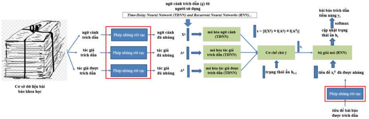
Hình 2.1. Kiến trúc của mô hình NCN
