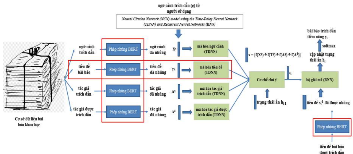
Hình 2.3. Kiến trúc của mô hình Enhanced-NCN
