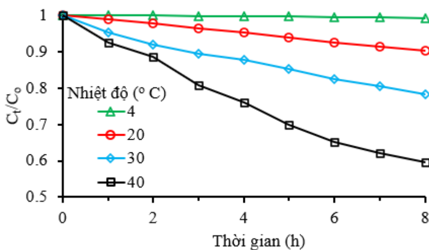
Hình 3.25. Ảnh hưởng của nhiệt độ tới độ bền của dung dịch ferrate (Điều kiện thí nghiệm: Nồng độ ferrate ban đầu 418,6 mg/L)
