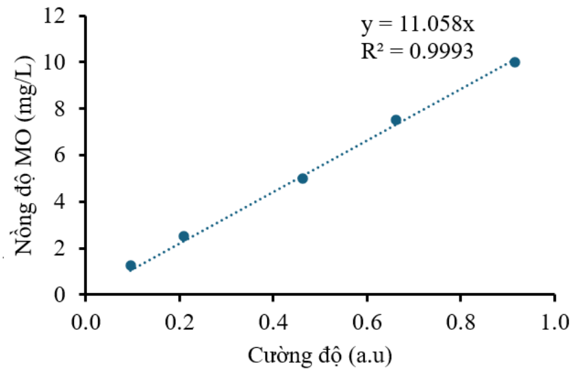
Hình PL2.3. Đường chuẩn xác định nồng độ dung dịch MO
