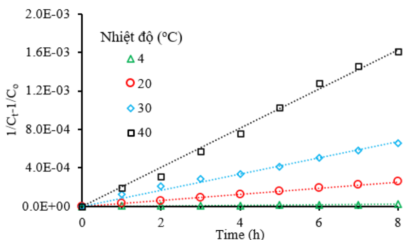
Hình 3.28. Mối quan hệ giữa (\frac{1}{C_t} - \frac{1}{C_0}) và thời gian t
