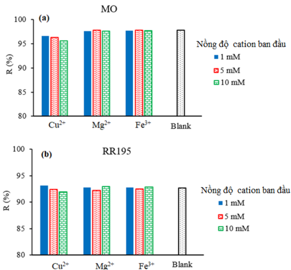
Hình 3.33. Ảnh hưởng của cation tới hiệu suất phân hủy (a) MO, (b) RR195 bằng ferrate
