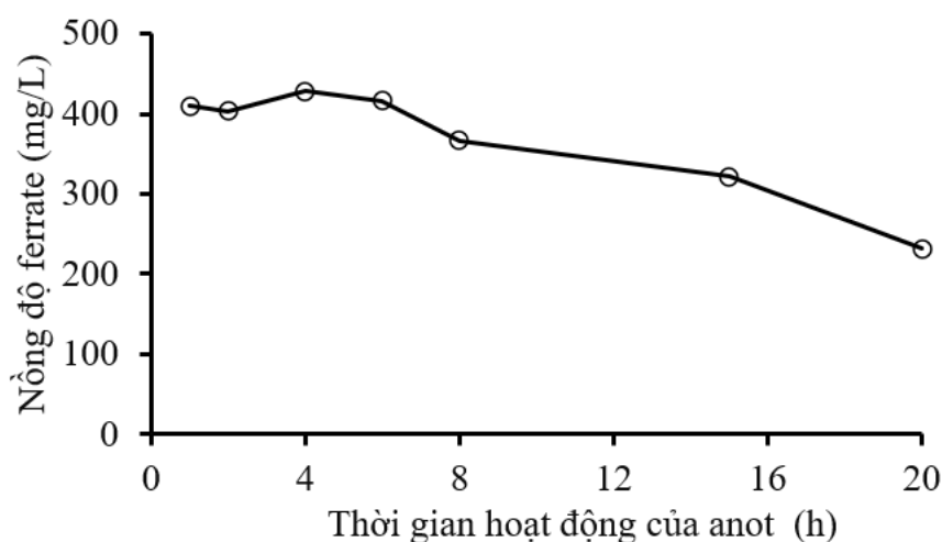
Hình 3.24. Ảnh hưởng thời gian hoạt động của anot tới nồng độ ferrate tạo thành (Điều kiện thí nghiệm: Dung dịch điện ly NaOH 14 M, mật độ dòng 40 mA/cm 2 , nhiệt độ 30°C, thời gian tổng hợp 1 h)
