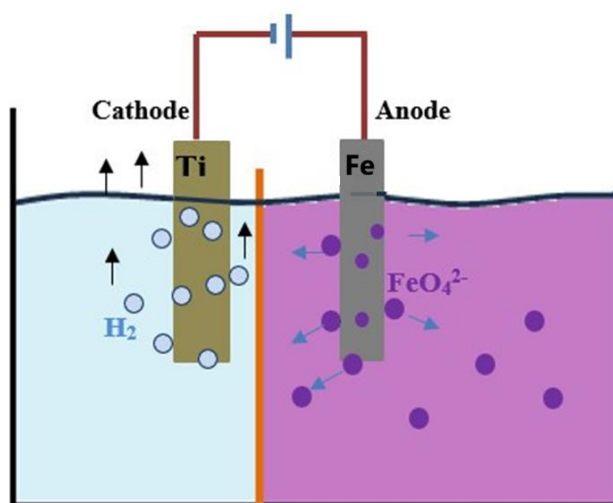
Hình 1.3. Mô hình điện hóa tổng hợp ferrate bằng phương pháp điện hóa sử dụng anot hòa tan
