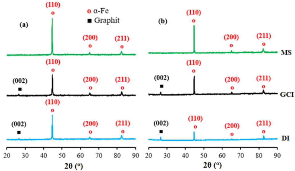
Hình 3.10. Giản đồ nhiễu xạ tia X của các vật liệu DI, GCI và MS (a) trước và (b) sau tổng hợp ferrate 3 h
