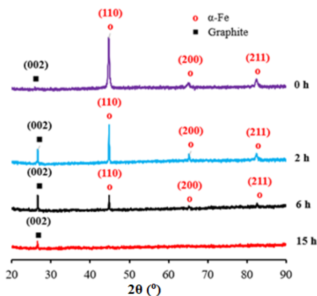
Hình 3.18. Giản đồ XRD của anot DI trước và sau thời gian điện phân khác nhau.
