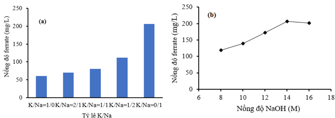
Hình 3.13. (a) Ảnh hưởng của tỷ lệ mol K/Na trong dung dịch hỗn hợp KOH-NaOH có nồng độ \text{OH}^- 14 M đến nồng độ ferrate, (b) Ảnh hưởng của nồng độ NaOH đến nồng độ ferrate tạo thành.
