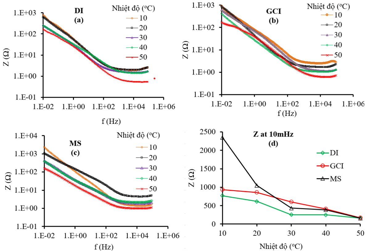
Hình 3.6. Phổ tổng trở dạng Bode tại các nhiệt độ khác nhau của các vật liệu anot (a) DI, (b) GCI, (c) MS và (d) tổng trở tại tần số 10 mHz.
