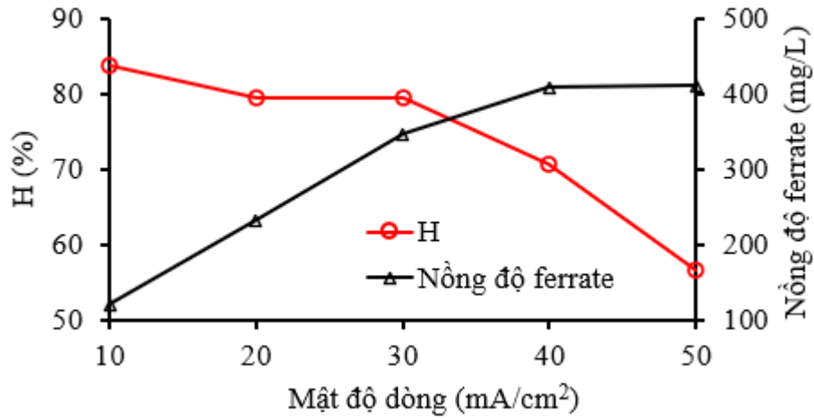
Hình 3.15. Ảnh hưởng của mật độ dòng tới hiệu suất và nồng độ ferrate tạo thành (Điều kiện thí nghiệm: dung dịch điện ly NaOH 14 M, thời gian điện phân 1 giờ, nhiệt độ tổng hợp 30 °C)
