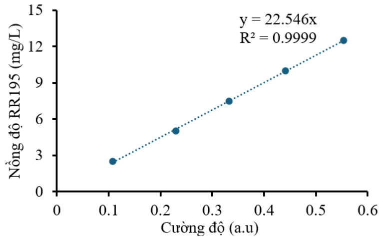
Hình PL2.4. Đường chuẩn xác định nồng độ dung dịch RR195
