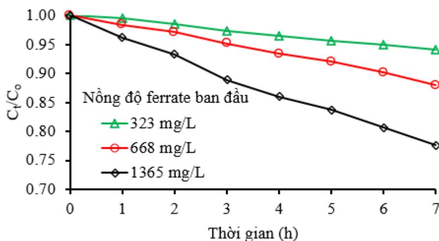
Hình 3.26. Ảnh hưởng của nồng độ ferrate ban đầu tới quá trình phân hủy ferrate (Điều kiện thí nghiệm: dung dịch NaOH 14 M)
