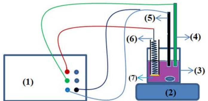
Hình 2.1. Mô hình tổng hợp ferrate điện hóa
