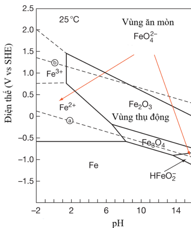
Hình 1.4. Đồ thị Pourbaix Fe-H 2 O [55]
