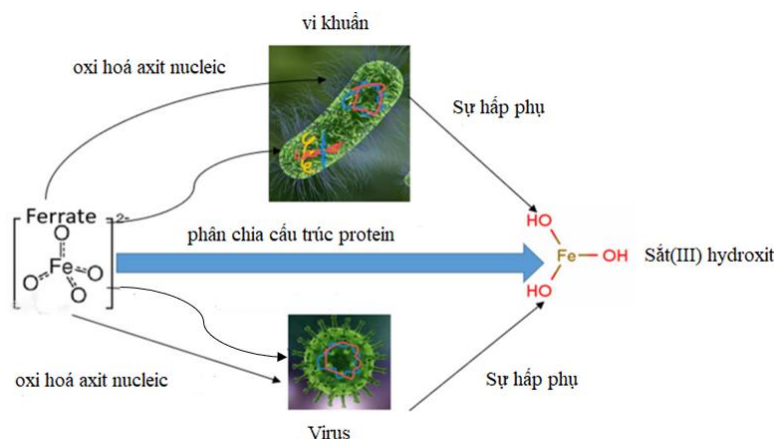
Hình 1.10. Sơ đồ khử trùng của ferrate[15]
