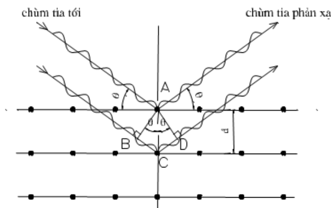
Hình 2.6. Sự nhiễu xạ tia X trên bề mặt tinh thể
