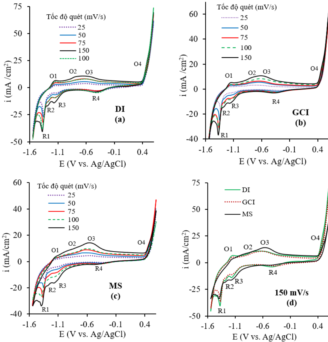
Hình 3.1. Phổ CV của các vật liệu anot (a) DI, (b) GCI, (c) MS trong dung dịch NaOH 14 M tại các tốc độ quét khác nhau, (d) So sánh phổ CV giữa các vật liệu tại tốc độ quét 150 mV/s (nhiệt độ 20 °C).
