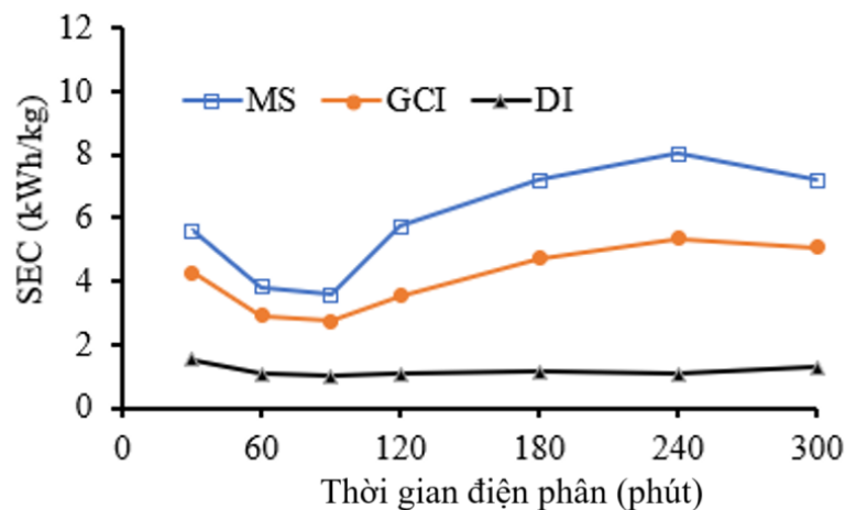
Hình 3.9. Năng lượng tiêu thụ riêng của quá trình tổng hợp ferrate điện hoá sử dụng các vật liệu anot DI, GCI và MS
