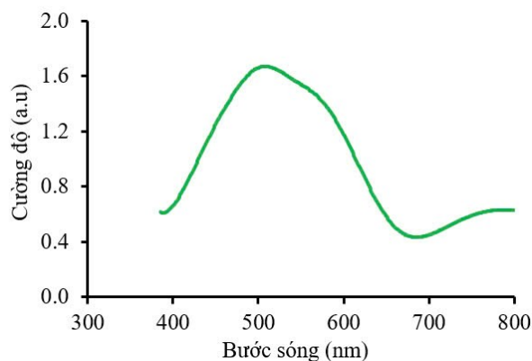
Hình 2.7. Phổ UV-vis của dung dịch ferrate
