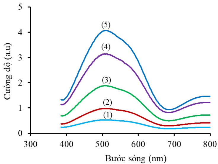
Hình PL2.1. Phổ UV-vis của các mẫu ferrate
