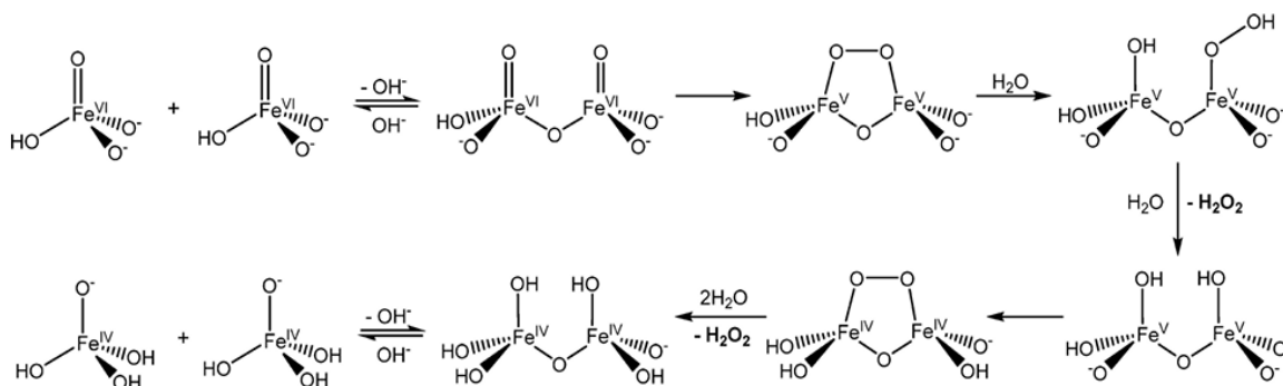
Hình 1.8. Cơ chế phân hủy từ Fe(VI) thành Fe(IV)[65]
