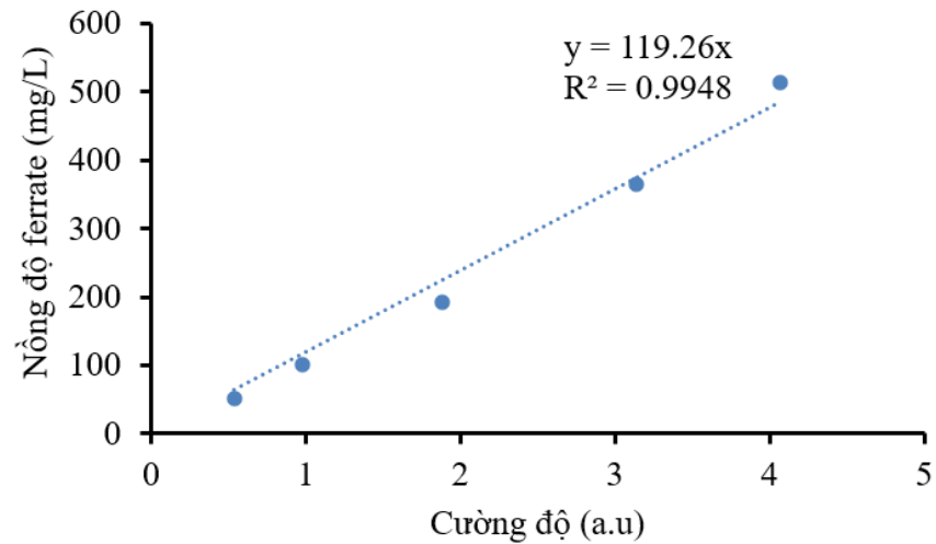
Hình PL2.2. Đường chuẩn xác định nồng độ dung dịch ferrate (VI)
