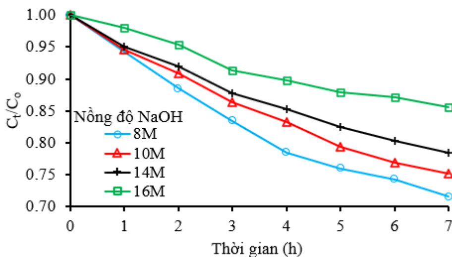
Hình 3.27. Ảnh hưởng của nồng độ NaOH tới quá trình phân hủy ferrate (Điều kiện thí nghiệm: Nồng độ ferrate ban đầu 461,5 mg/L)
