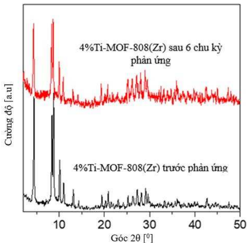
Hình 3.74. Giảm đồ XRD của 4%Ti–MOF-808(Zr) trước và sau 6 chu kỳ phản ứng
