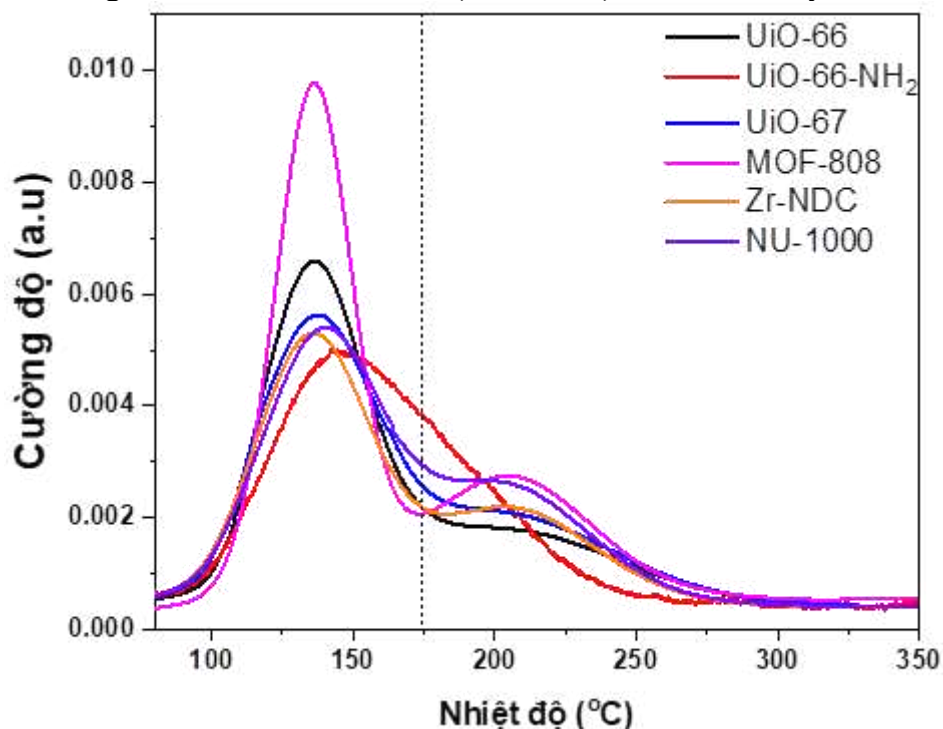
Hình 3.40. Giải đồ NH 3 -TPD của Zr-MOFs-TM
