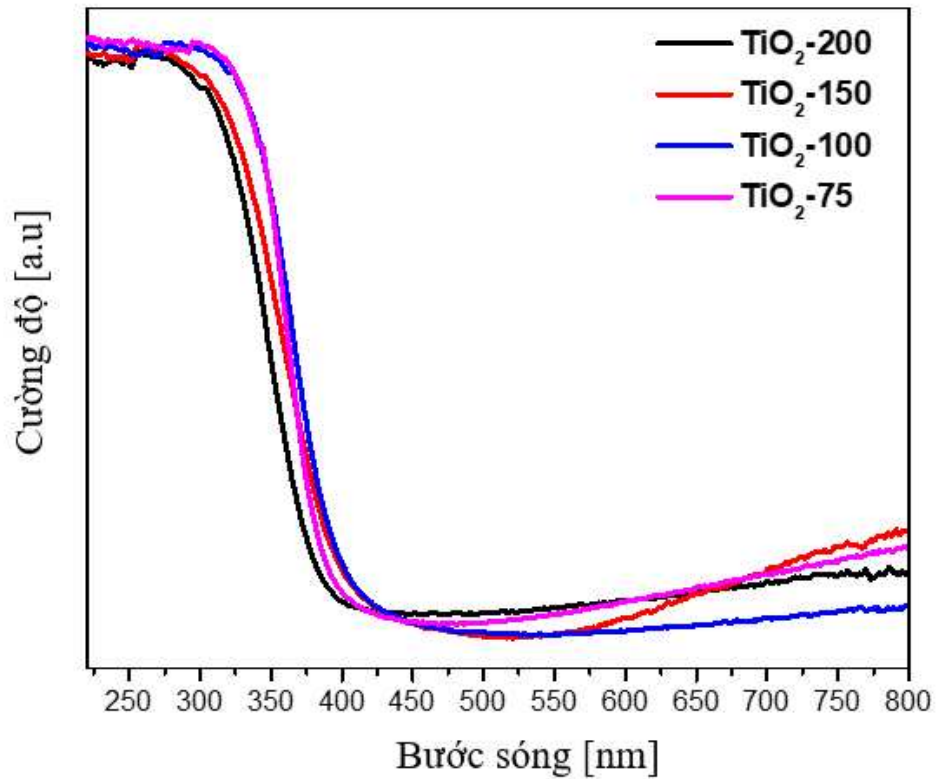
Hình 3.5. Phổ UV-Vis DRS của nano \text{TiO}_2
