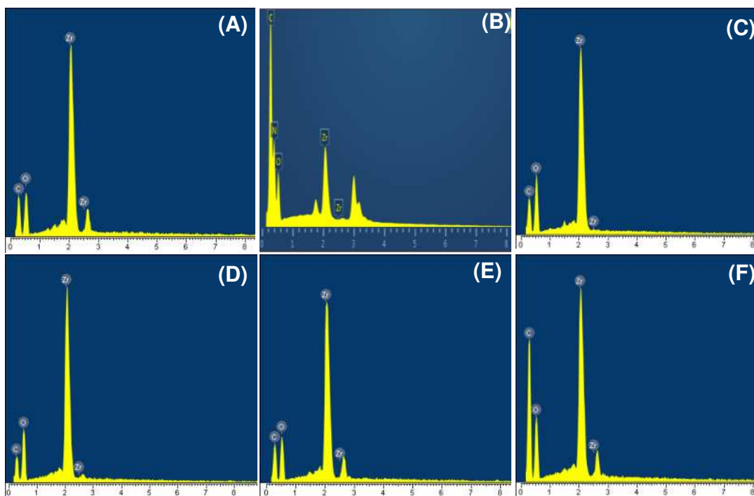
Hình 3.39. EDS của UiO-66 (A), UiO-66-NH 2 (B), UiO-67 (C), MOF-808 (D), Zr-NDC (E) và NU-1000 (F)
