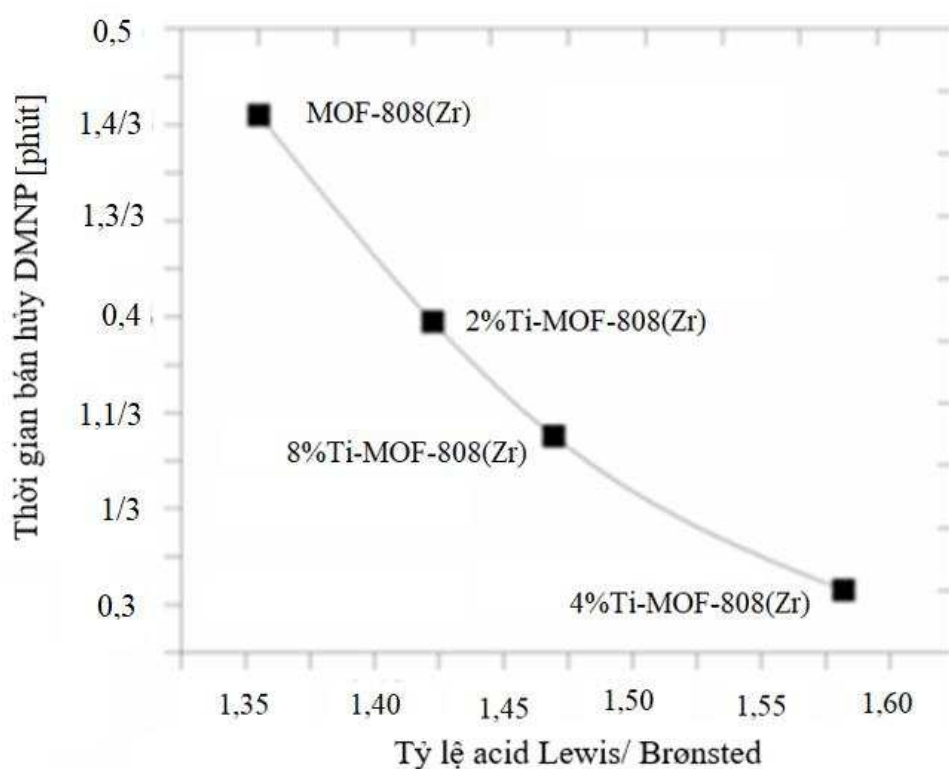
Hình 3.59. Mối quan hệ giữa tỉ lệ acid Lewis/Brønsted và thời gian bán hủy DMNP trên vật liệu MOF-808(Zr) và (2, 4, 8%)Ti–MOF-808(Zr)
