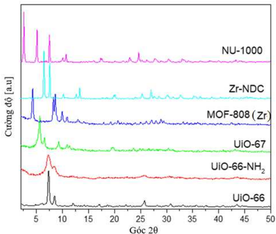
Hình 3.35. Giảm đồ XRD của UiO-66, UiO-66-NH 2 , UiO-67, MOF-808(Zr), Zr-NDC và NU-1000
