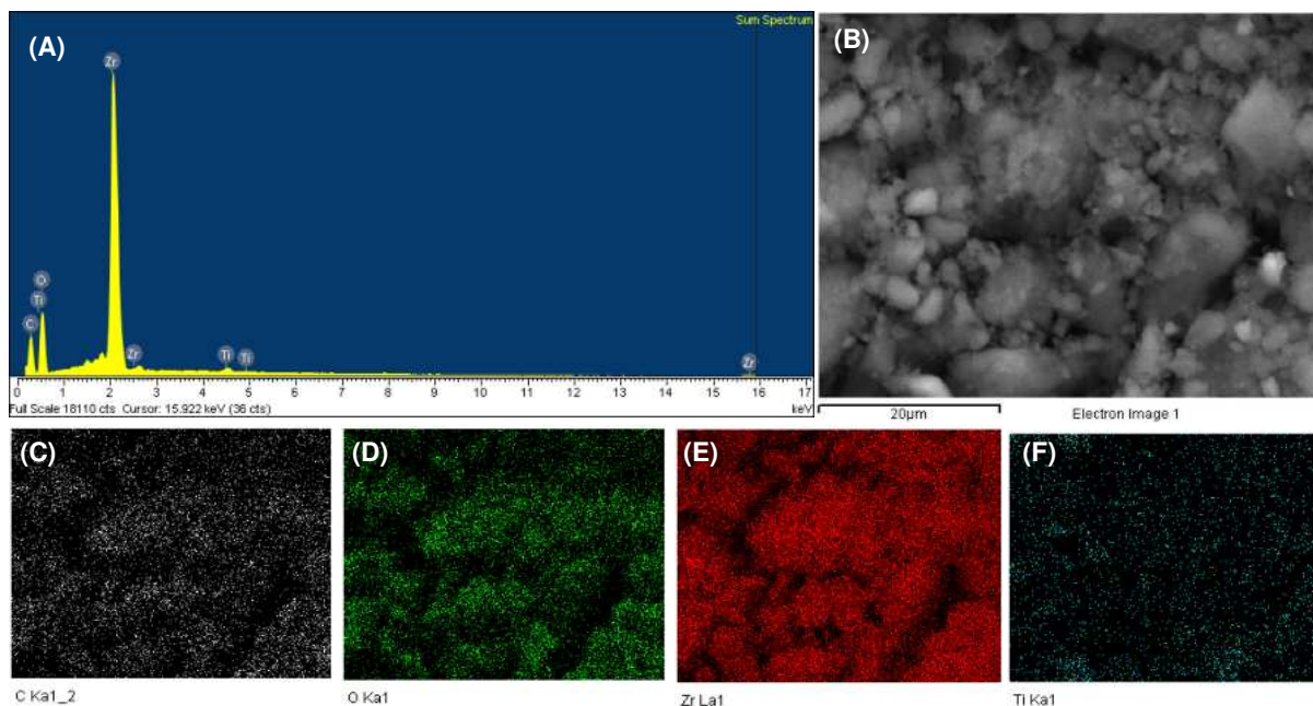
Hình 3.52. (A) Phổ EDS, (B) EDS lớp nguyên tố, ảnh điện tử EDS-mapping của nguyên tố C (C), O (D), Zr (E) và Ti (F) của mẫu 4%Ti–MOF-808(Zr)
