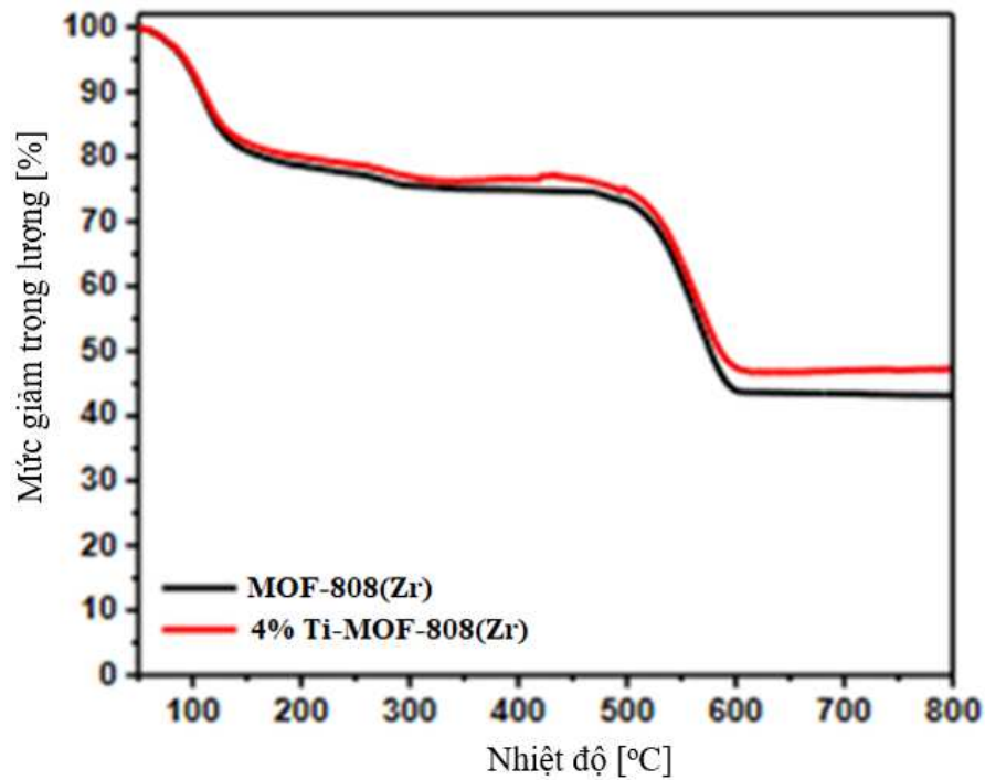
Hình 3.53. Đường cong TGA của mẫu MOF-808(Zr) và 4%Ti–MOF-808(Zr)
