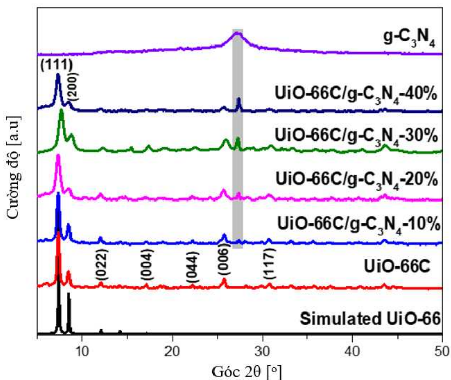
Hình 3.12. Giảm đồ XRD của mẫu vật liệu g- C_3N_4 , UiO-66C và UiO-66C/g- C_3N_4
