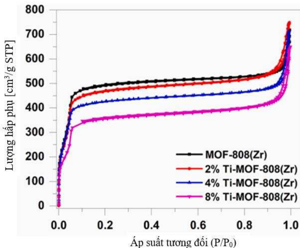
Hình 3.47. Đường đẳng nhiệt hấp phụ-giải hấp phụ N_2
