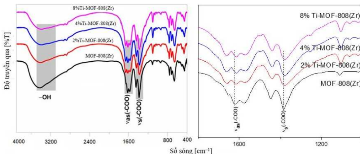
Hình 3.44. Phổ FTIR của mẫu MOF-808(Zr) và Ti-MOF-808(Zr)
