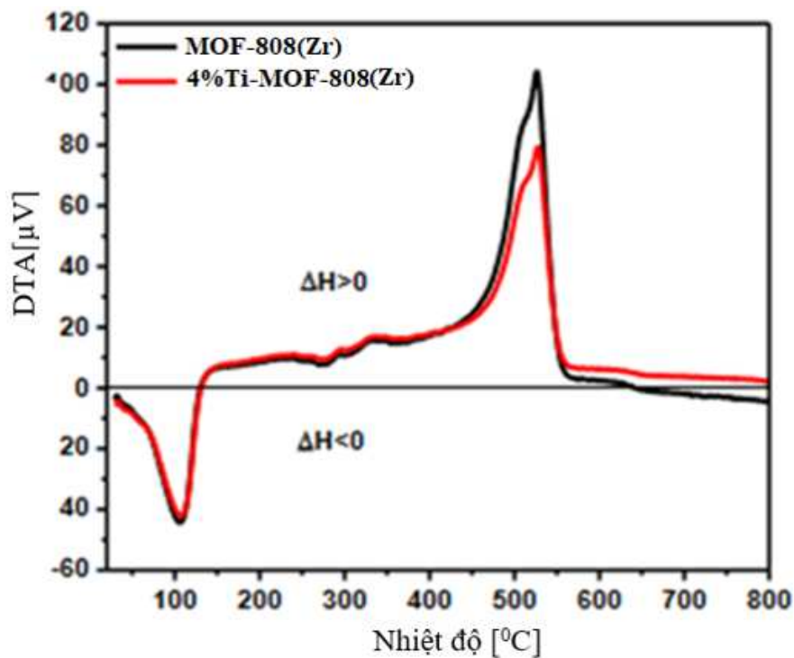
Hình 3.54. Đường cong DTA của mẫu MOF-808(Zr) và 4%Ti–MOF-808(Zr)
