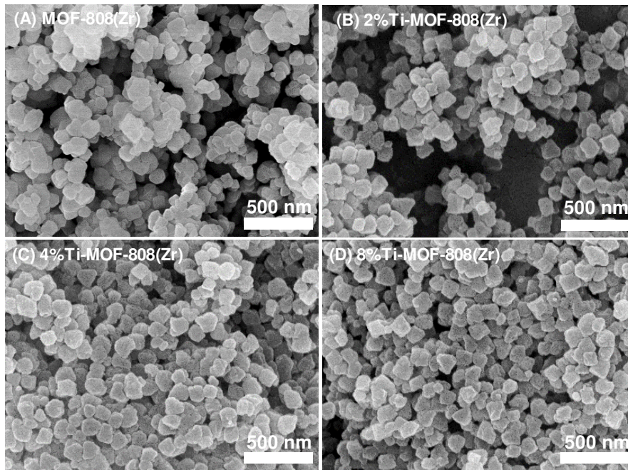
Hình 3.45. Ảnh SEM của mẫu MOF-808 (Zr) và Ti-MOF-808 (Zr)
