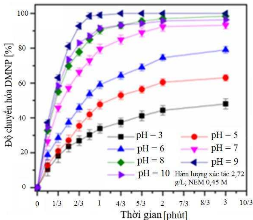
Hình 3.71. Độ chuyển hóa của DMNP trên 4%Ti-MOF-808(Zr) với giá trị pH khác nhau
