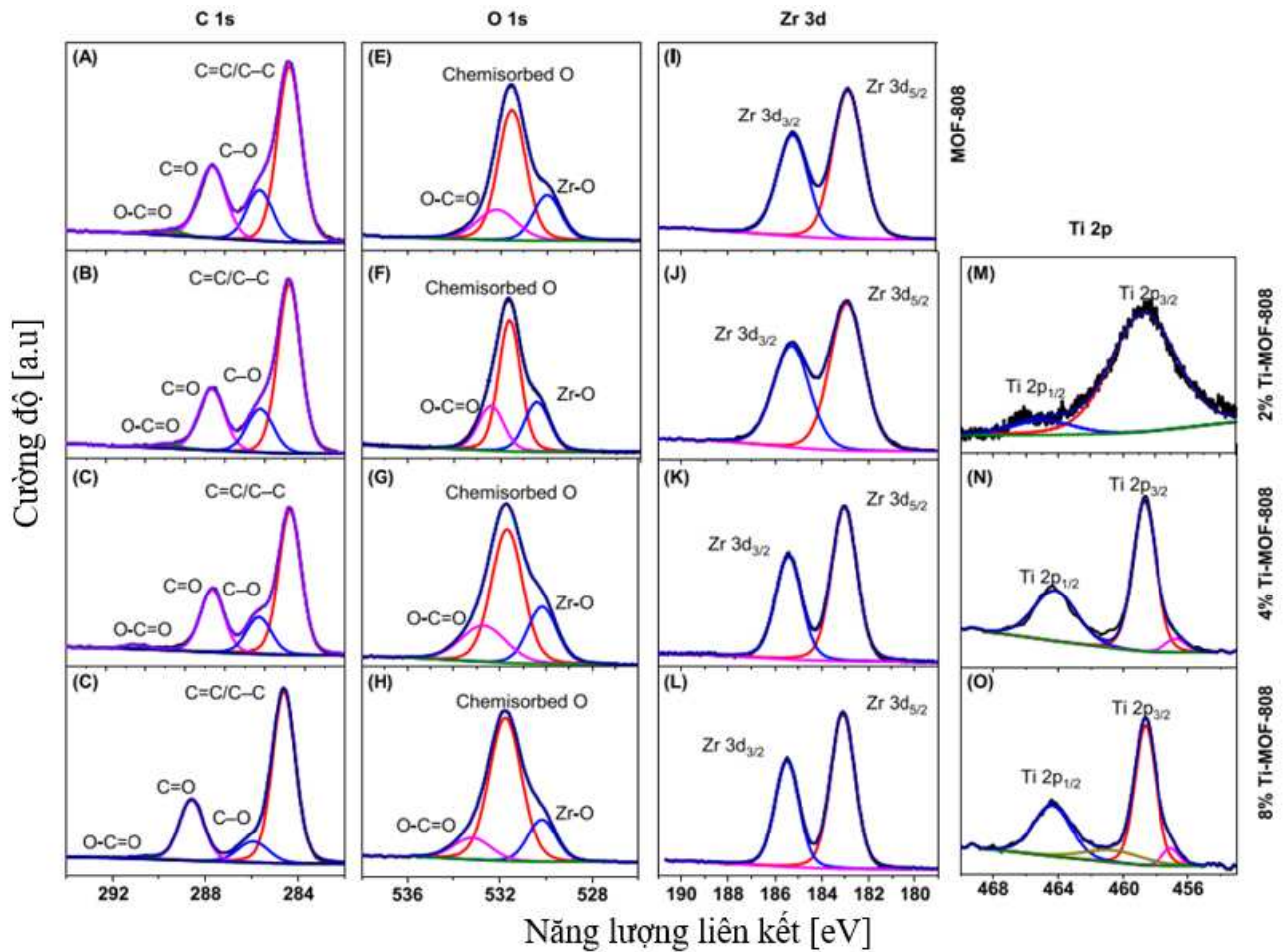
Hình 3.50. Phổ XPS của MOF-808(Zr) và Ti–MOF-808(Zr)
