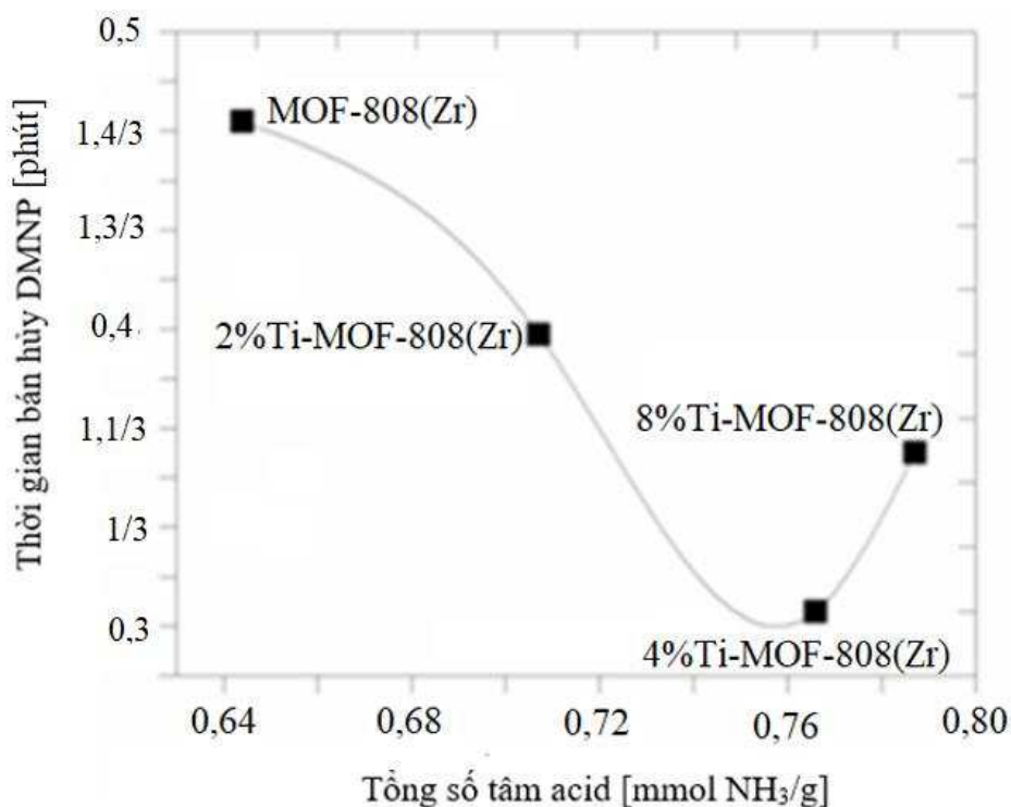
Hình 3.60. Mối quan hệ tổng số tâm acid (mmol \text{NH}_3/\text{g} ) và thời gian bán hủy DMNP trên MOF-808(Zr) và (2, 4, 8%)Ti–MOF-808(Zr)
