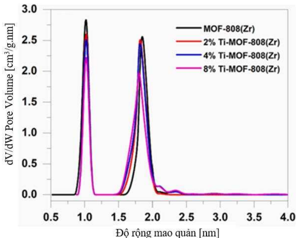
Hình 3.48. Sơ đồ phân bố mao quản (theo DFT) của MOF-808(Zr) và Ti-MOF-808(Zr)
