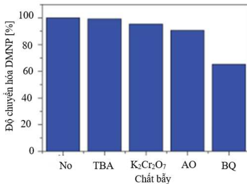
Hình 3.33. Thí nghiệm bắt điện tử
