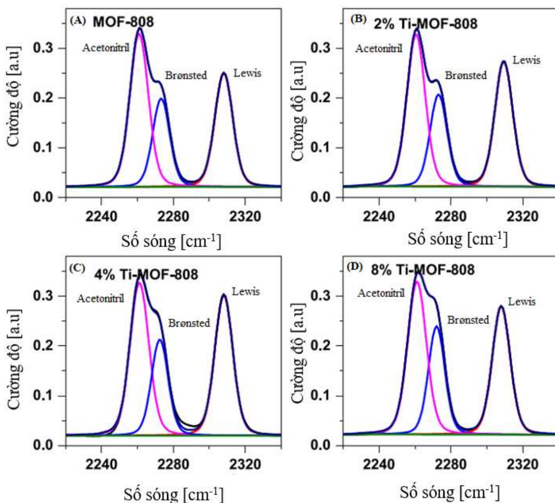
Hình 3.56. Phổ FTIR-CD 3 CN của MOF-808(Zr) và (2, 4, 8%) Ti-MOF-808(Zr)
