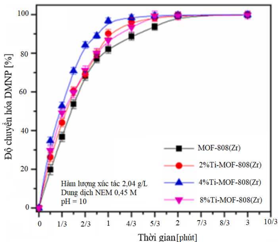
Hình 3.61. Hiệu suất chuyển hóa DMNP theo thời gian phản ứng trên các mẫu \text{MOF-808(Zr)} và (2, 4, 8\%)\text{Ti-MOF-808(Zr)}
