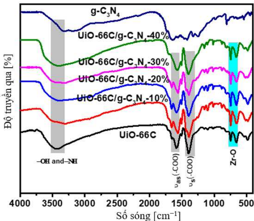
Hình 3.13. Phổ FT-IR của UiO-66C và UiO-66C/ g\text{-C}_3\text{N}_4
