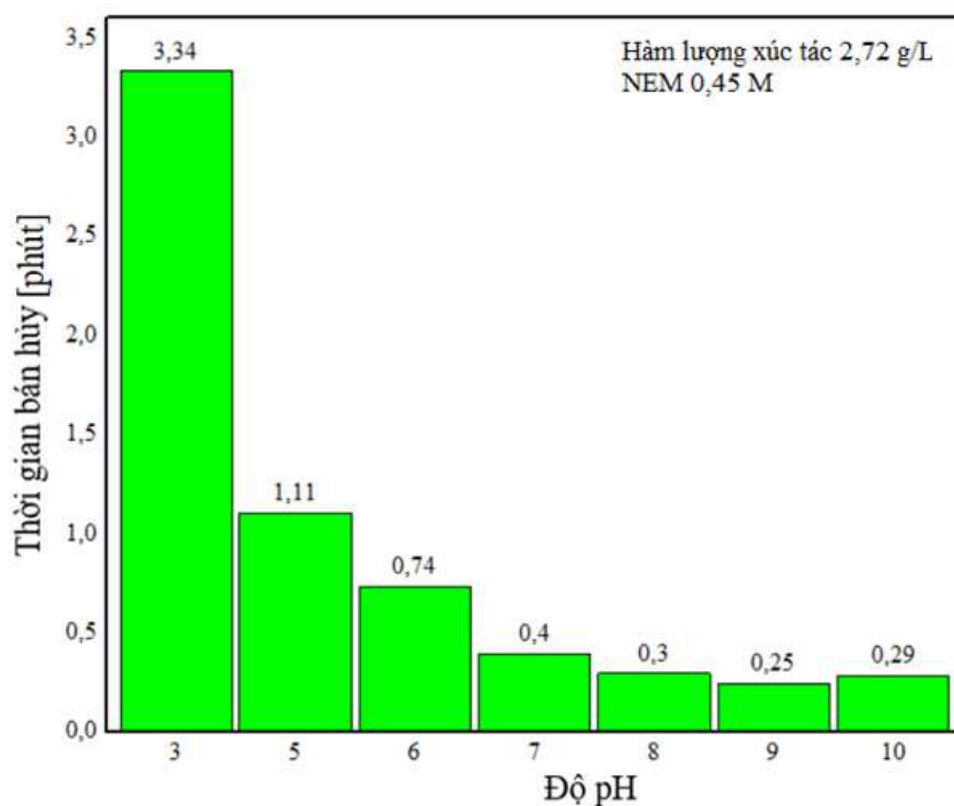
Hình 3.72. Thời gian bán hủy của DMNP trên 4% \text{Ti-MOF-808(Zr)} với giá trị pH khác nhau
