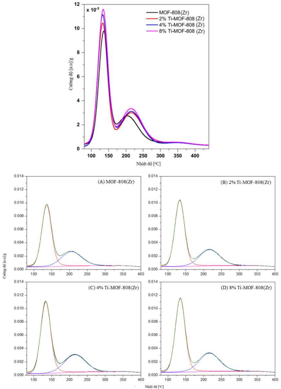
Hình 3.55. Giải đồ \text{NH}_3 -TPD của MOF-808(Zr) và (2, 4, 8%) Ti–MOF-808(Zr)
