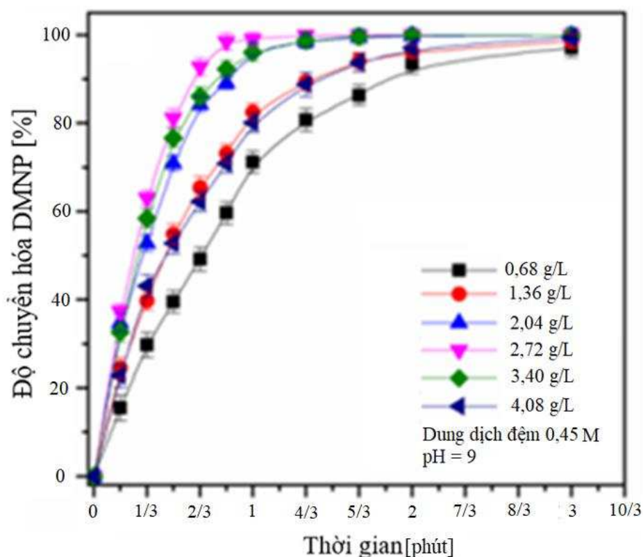
Hình 3.65. Độ chuyển hóa của DMNP với các lượng khác nhau của 4%Ti-MOF-808(Zr)
