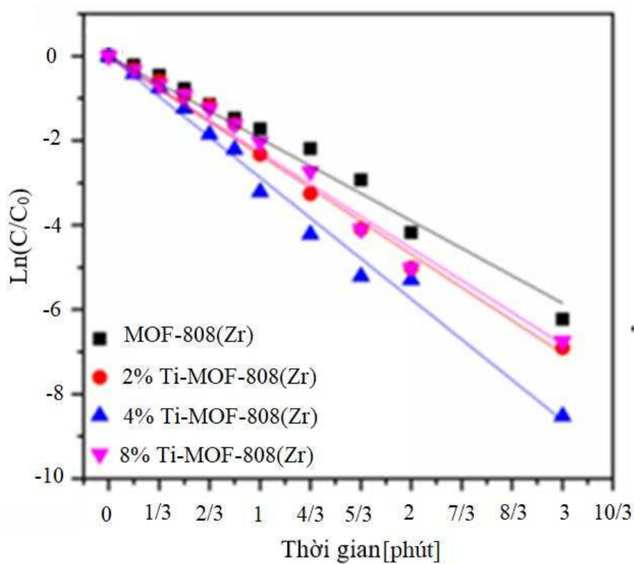
Hình 3.63. Động học phản ứng bậc nhất của phân hủy DMNP trên MOF-808(Zr) và (2, 4, 8%)Ti-MOF-808(Zr)
