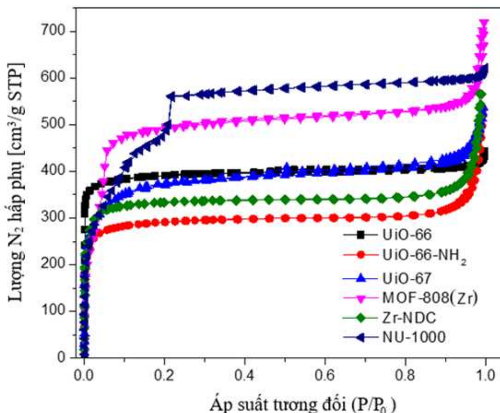
Hình 3.37. Đường đẳng nhiệt hấp phụ-giải hấp phụ N 2 của UiO-66, UiO-66-NH 2 , UiO-67, MOF-808(Zr), Zr-NDC và NU-1000
