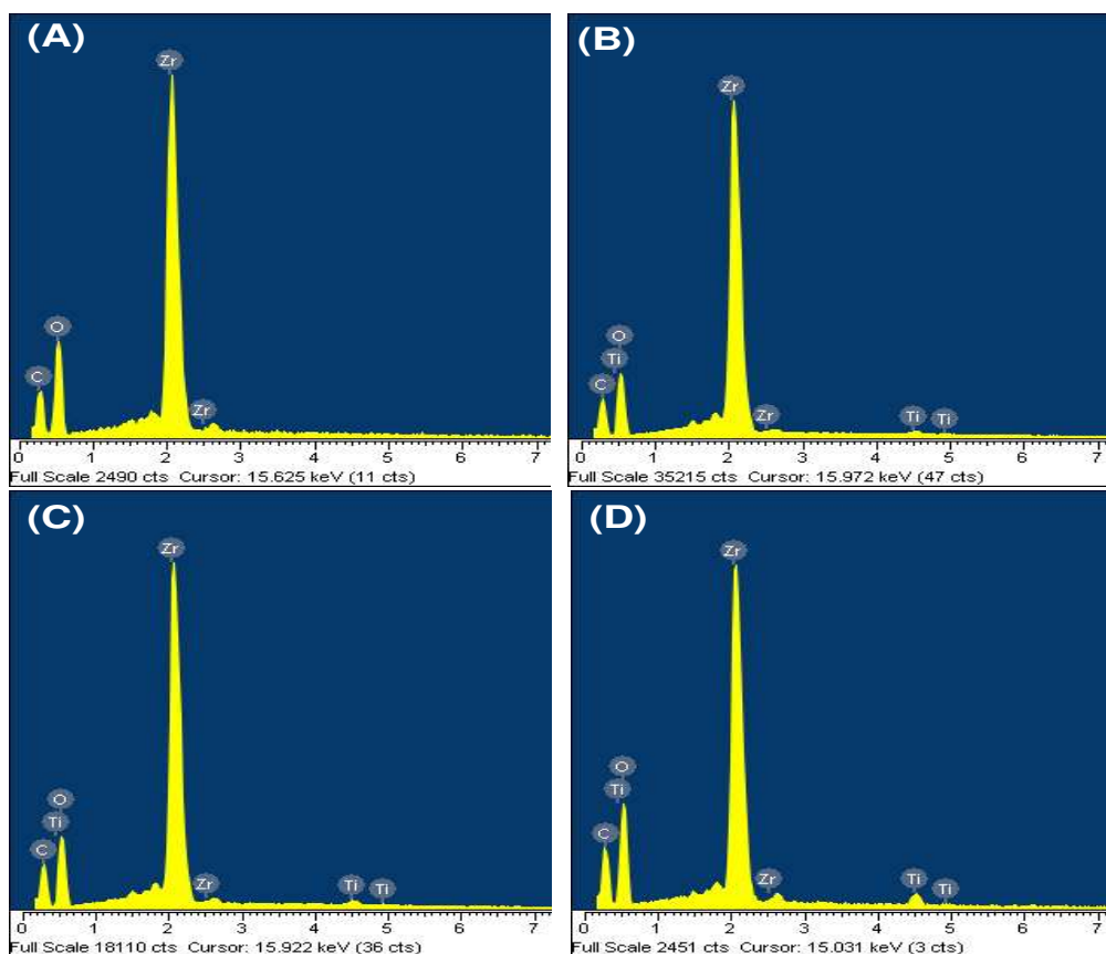
Hình 3.51. Phổ EDS của MOF-808(Zr) (A), 2%Ti–MOF-808(Zr) (B), 4%Ti–MOF-808(Zr) (C) và 8%Ti–MOF-808(Zr) (D)
