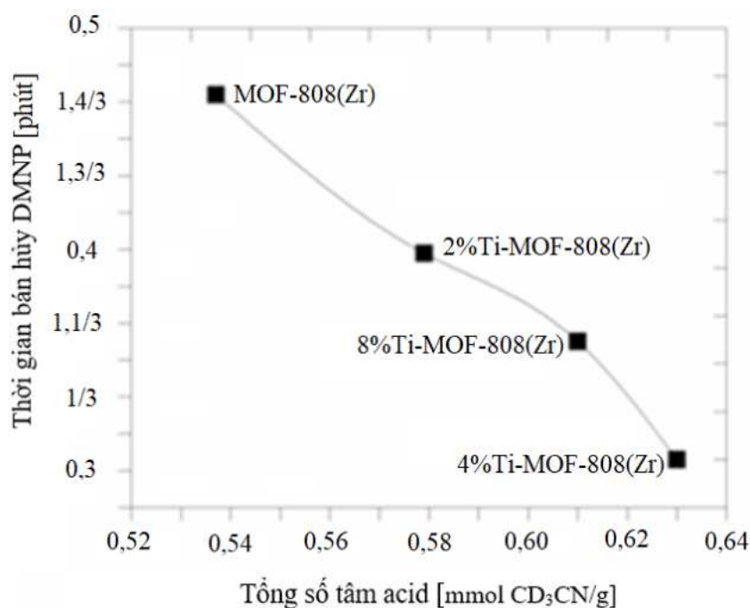
Hình 3.58. Mối quan hệ giữa tổng số tâm acid (mmol \text{CD}_3\text{CN}/\text{g} ) và thời gian bán hủy của DMNP trên MOF-808(Zr) và (2, 4, 8%)Ti-MOF-808(Zr)
