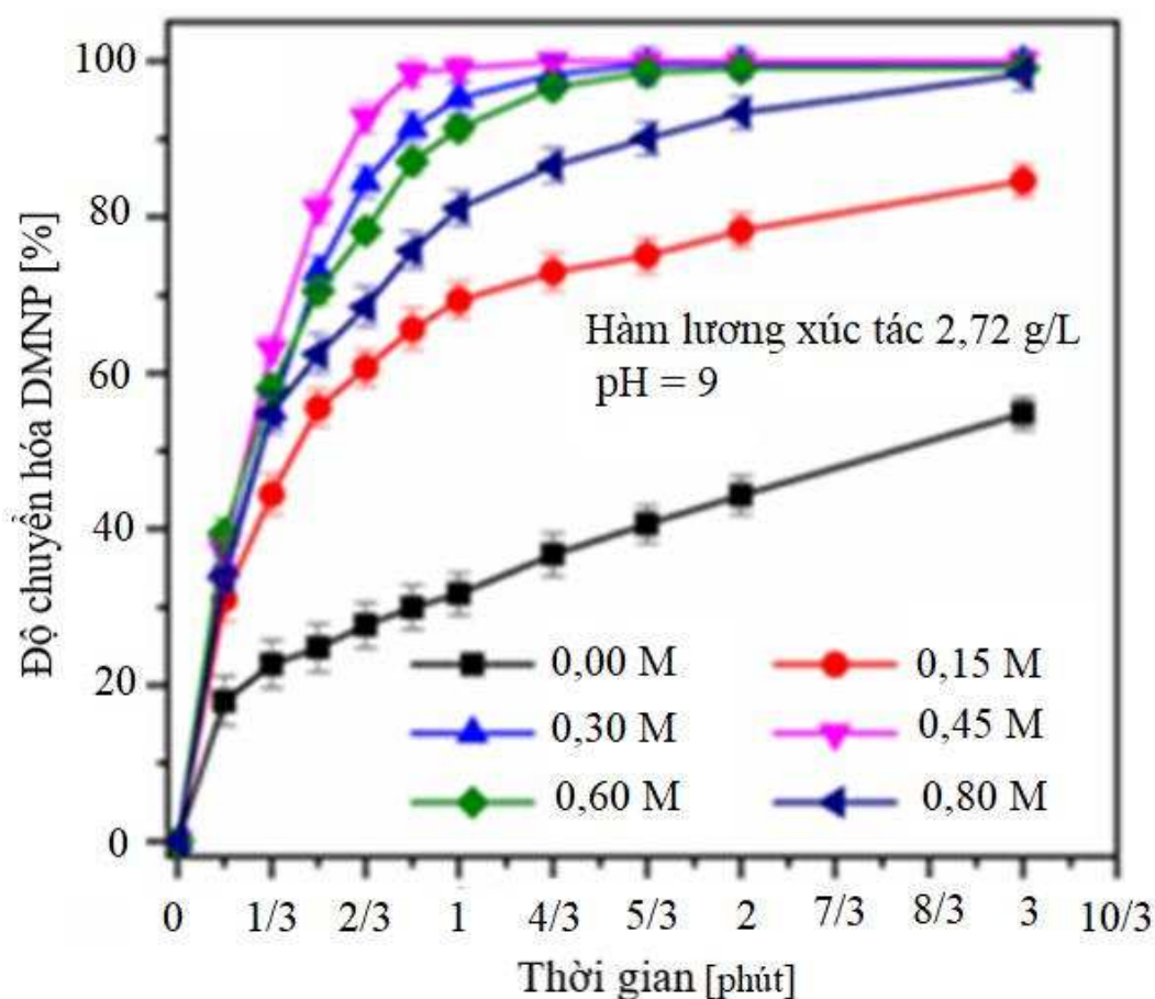
Hình 3.67. Độ chuyển hóa của DMNP trên 4%Ti–MOF-808(Zr) với giá trị nồng độ dung dịch đệm NEM khác nhau
