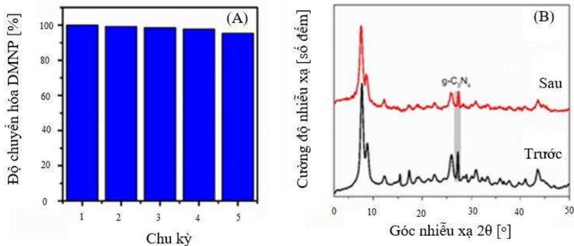
Hình 3.32. (A) Độ chuyển hóa DMNP trên UiO-66C/g-C 3 N 4 -30% ở các chu kỳ khác nhau; (B) Giản đồ XRD của UiO-66C/g-C 3 N 4 -30% trước và sau phản ứng
