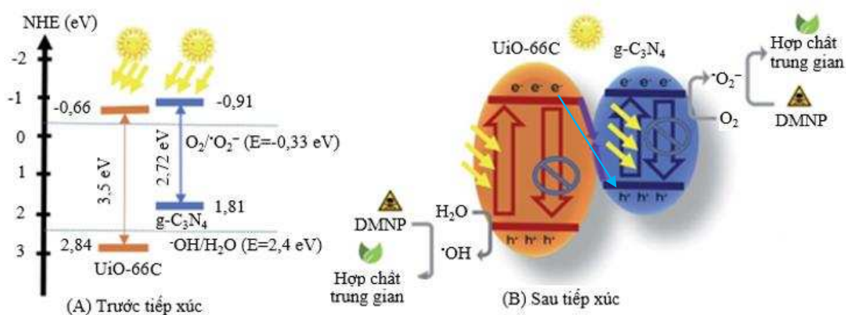
Hình 3.34. Cơ chế phân tách và chuyển electron/lỗ trống của UiO-66C/g-C 3 N 4 trước khi tiếp xúc (A) và sau khi tiếp xúc (B)
