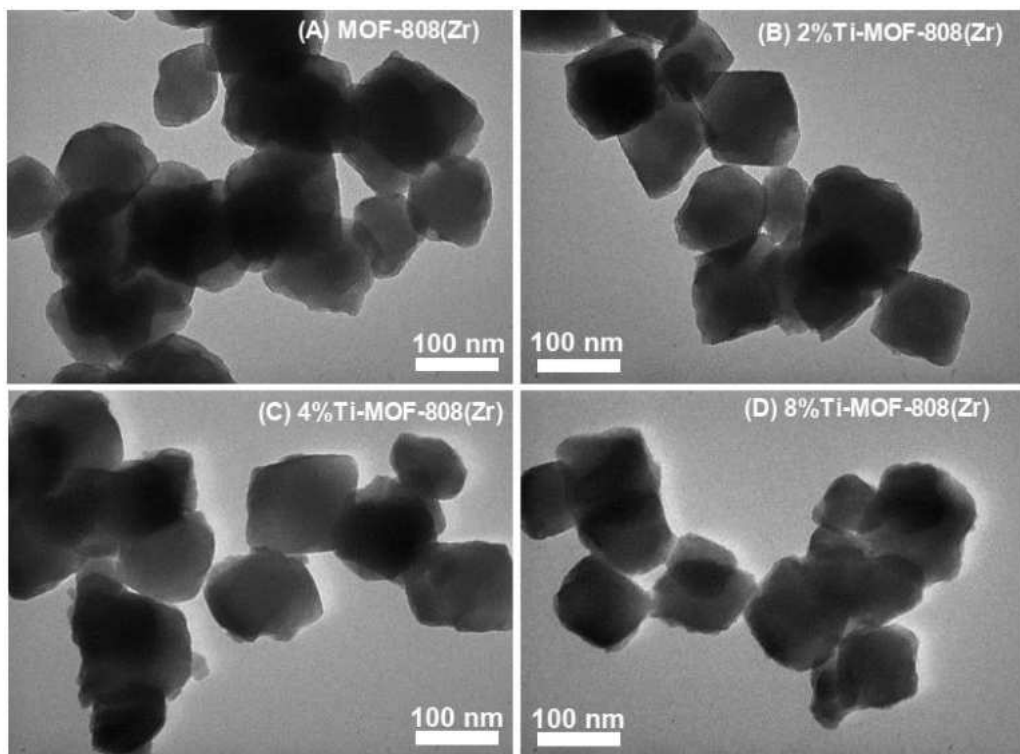
Hình 3.46. Ảnh TEM của mẫu MOF-808 (Zr) và Ti-MOF-808 (Zr)
