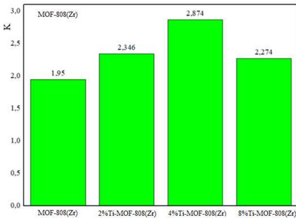
Hình 3.64. Hằng số tốc độ phản ứng phân hủy DMNP trên các xúc tác MOF-808 và (2, 4, 8%)Ti-MOF-808(Zr)
