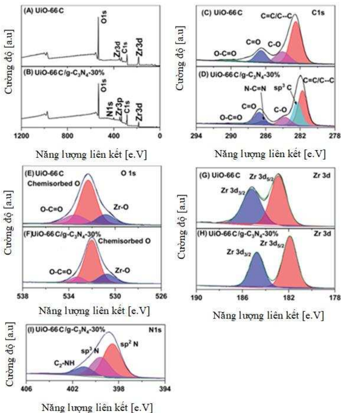
Hình 3.18. Phổ XPS của UiO-66C và UiO-66C/g-C 3 N 4 -30%
