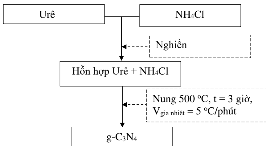
Hình 2.4. Sơ đồ điều chế g-C 3 N 4
