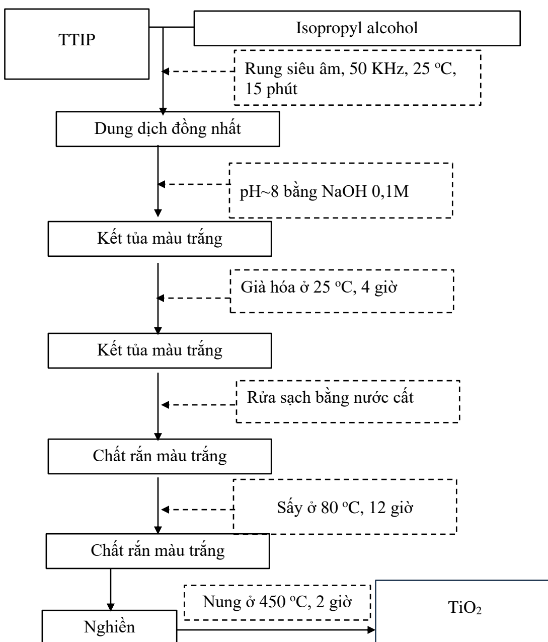
Hình 2.1. Sơ đồ tổng hợp \text{TiO}_2
