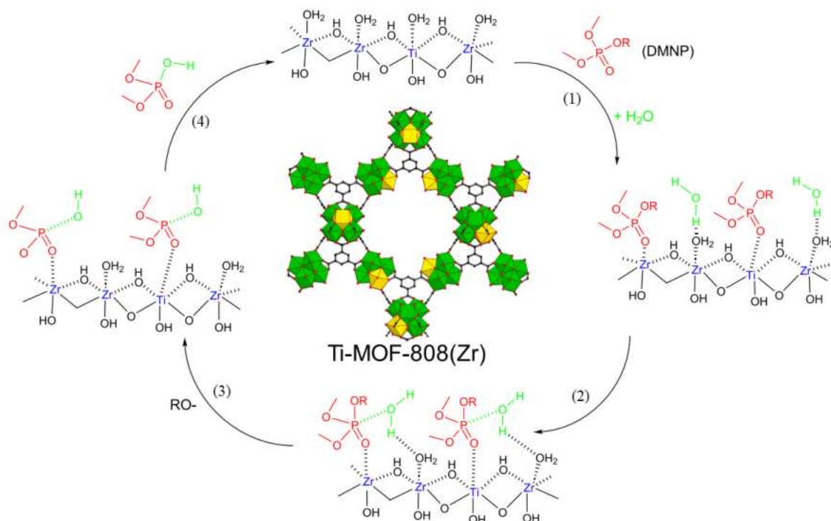
Hình 3.78. Cơ chế thủy phân DMNP trên xúc tác Ti-MOF-808(Zr)
