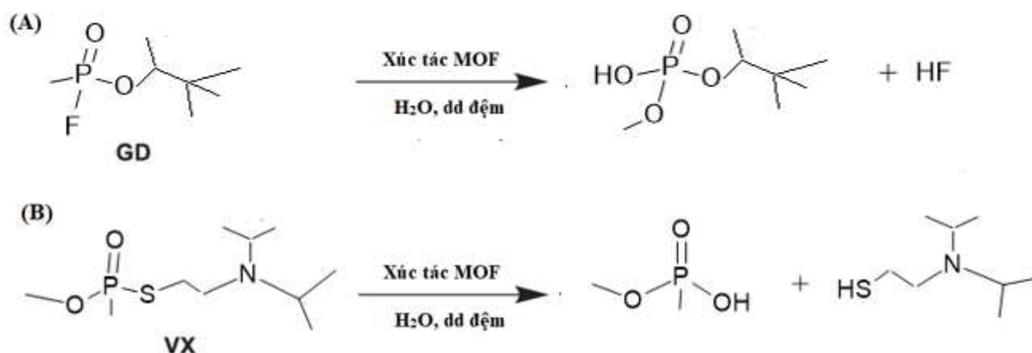
Hình 1.9. Sơ đồ phản ứng thủy phân chất độc thần kinh cơ photpho GD (A) và VX (B) bằng \text{Zr-MOFs} [26]
