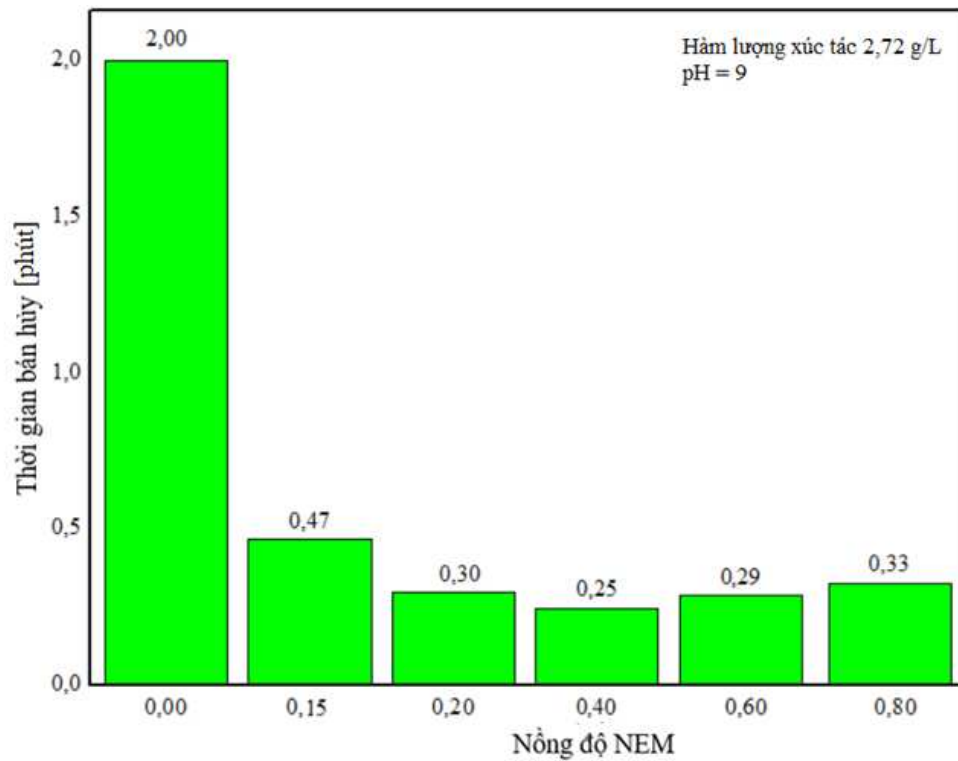
Hình 3.68. Thời gian bán hủy của DMNP trên xúc tác 4%Ti–MOF-808(Zr) với giá trị nồng độ dung dịch đệm NEM khác nhau
