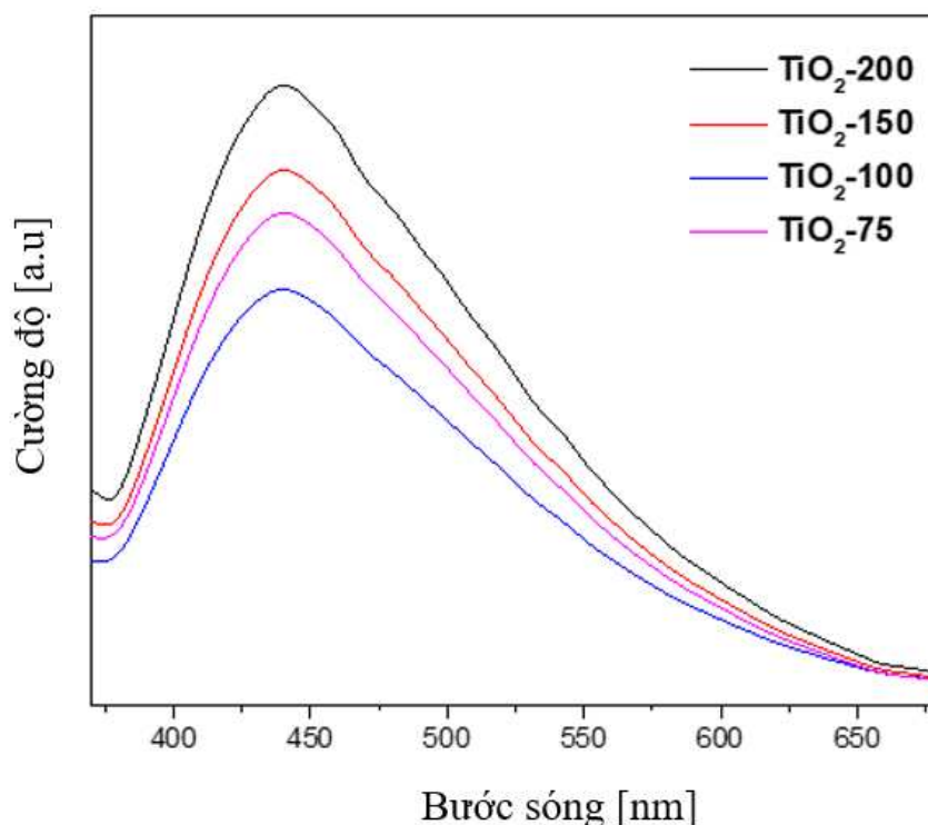
Hình 3.7. Phổ phát quang của \text{TiO}_2
