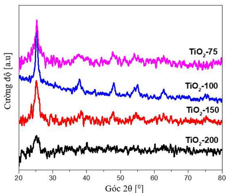
Hình 3.1. Giải đồ nhiễu xạ tia X (XRD) của các mẫu vật liệu nano \text{TiO}_2
