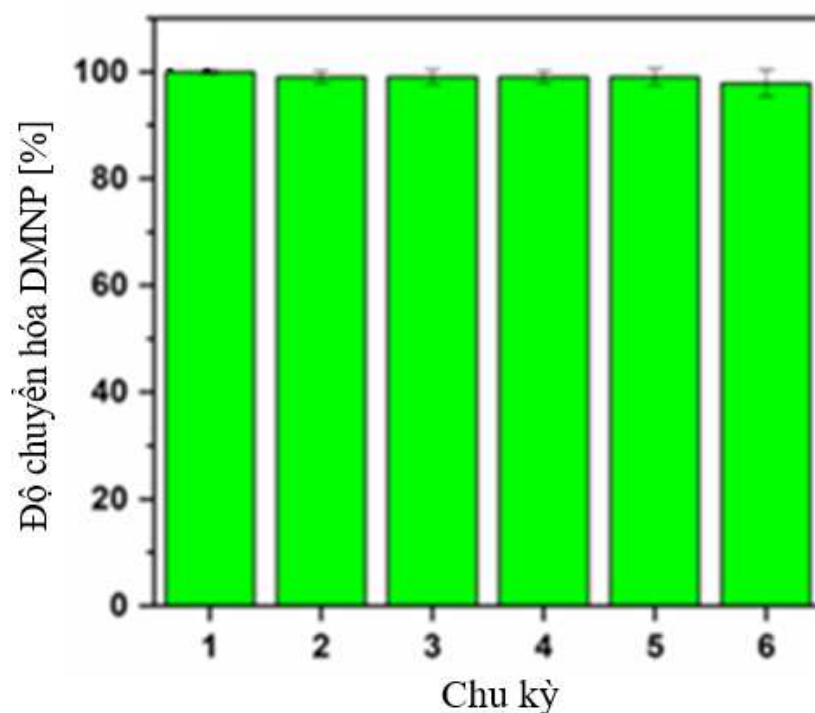
Hình 3.73. Khả năng tái sử dụng của vật liệu 4%Ti–MOF-808(Zr) để phân hủy DMNP (6,2 g/L) sau thời gian phản ứng 1,34 phút
