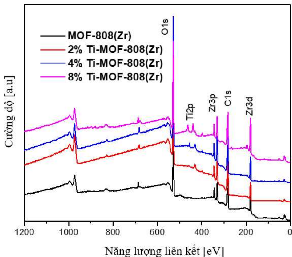
Hình 3.49. Phổ XPS của MOF-808(Zr) và Ti–MOF-808(Zr)
