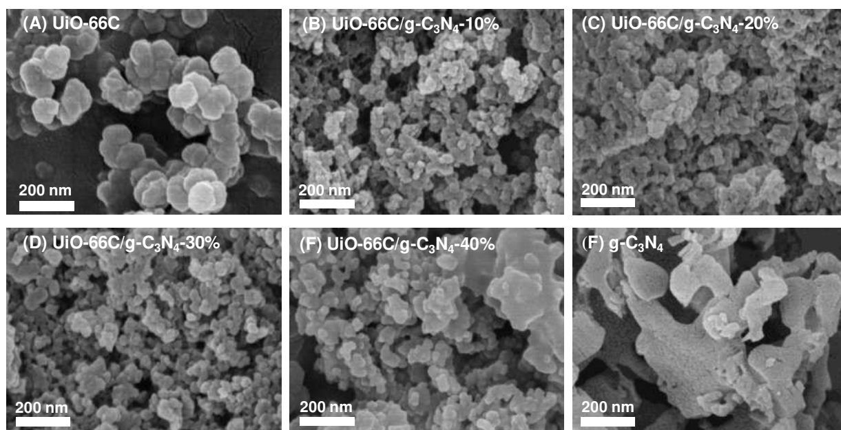
Hình 3.14. Ảnh SEM của g- C_3N_4 , UiO-66C và UiO-66C/ g- C_3N_4
