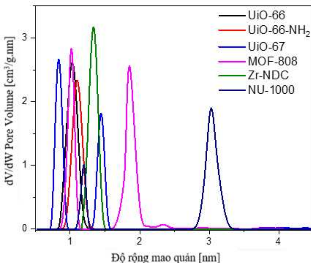
Hình 3.38. Sự phân phân bố mao quản (tính theo DFT) của UiO-66, UiO-66-NH 2 , UiO-67, MOF-808(Zr), Zr-NDC và NU-1000
