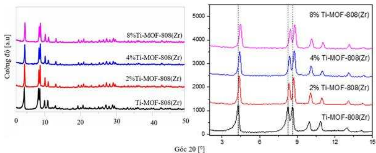
Hình 3.43. Giải đồ XRD của MOF-808(Zr) và (2, 4, 8%)Ti-MOF-808(Zr)
