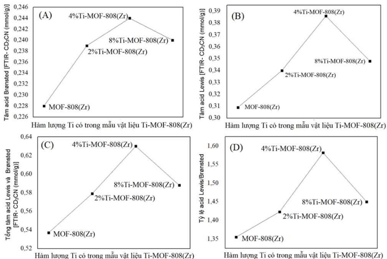
Hình 3.57. Biến đổi tâm acid Brønsted (A), tâm acid Lewis (B) và tổng số tâm acid Lewis và Brønsted (C) [mmol FTIR- CD 3 CN/g] và tỉ lệ acid Lewis/ Brønsted (D) theo hàm lượng Ti có trong các mẫu Ti–MOF-808(Zr)
