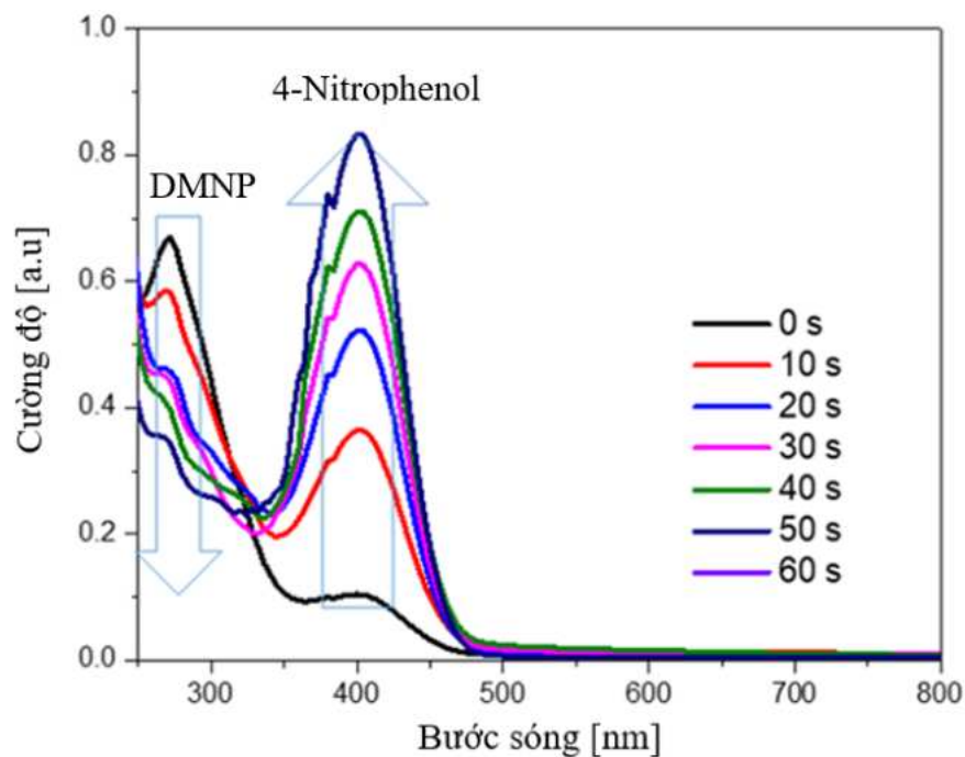
Hình 3.69. Phổ UV-vis của DMNP trong dung dịch đệm NEM 0,15 M tại các thời điểm phản ứng khác nhau
