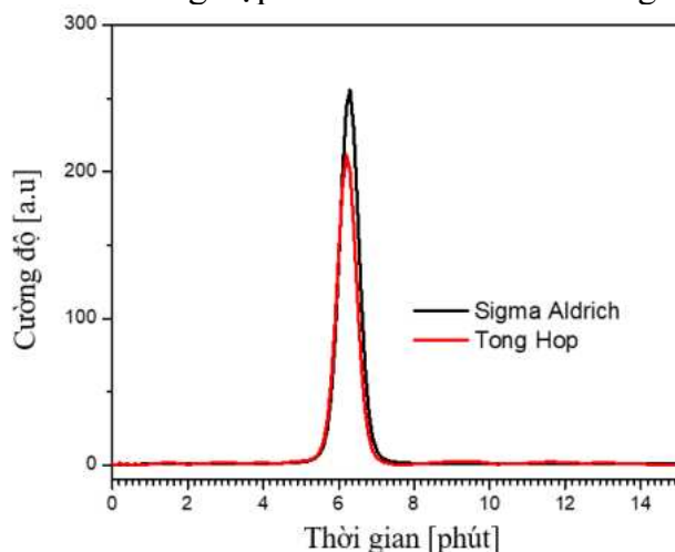
Hình 2.3. Sắc ký đồ sắc ký lỏng hiệu năng cao (HPLC) của sản phẩm H 2 BDC
