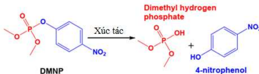
Hình 2.9. Phân hủy xúc tác DMNP [133]
