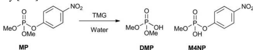
Hình 3.31. Sơ đồ phân hủy methyl paraoxon (MP)
