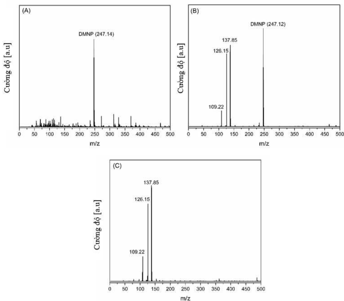
Hình 3.76. Phổ LC-MS sản phẩm phân hủy DMNP bằng xúc tác 4%Ti–MOF-808(Zr) với thời gian phản ứng khác nhau (A) 0 s, (B) 10 s và (C) 80 s
