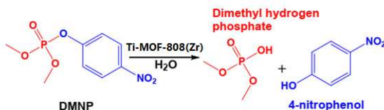
Hình 3.77. Phản ứng phân hủy DMNP bằng Ti–MOF-808(Zr)
