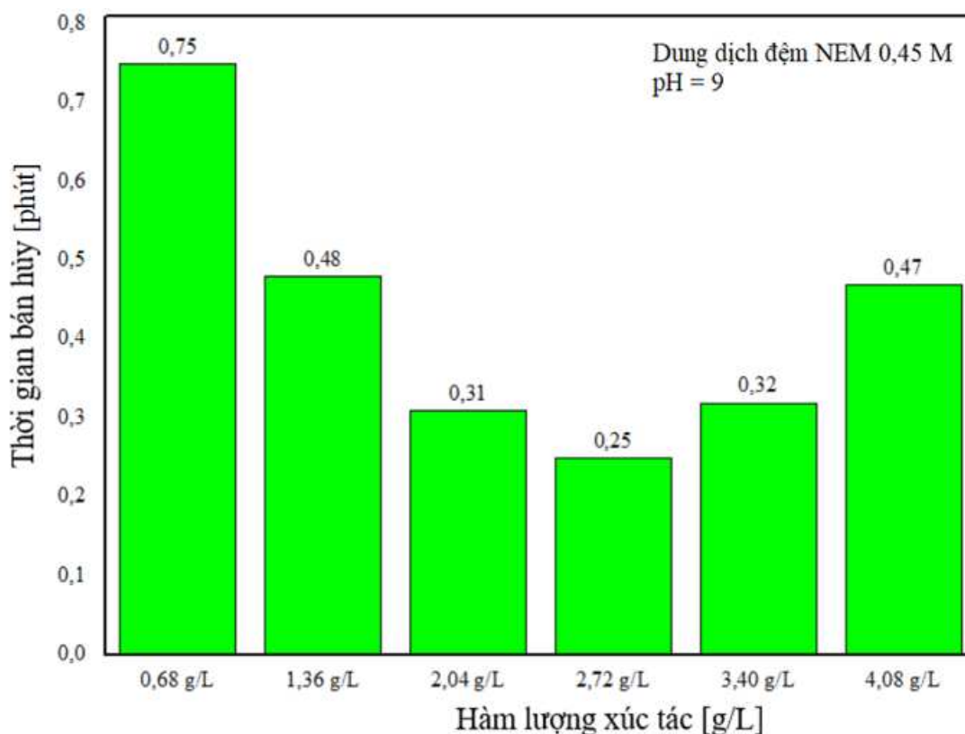
Hình 3.66. Mối quan hệ giữa thời gian bán hủy của DMNP với các hàm lượng khác nhau của chất xúc tác 4%Ti–MOF-808(Zr)
