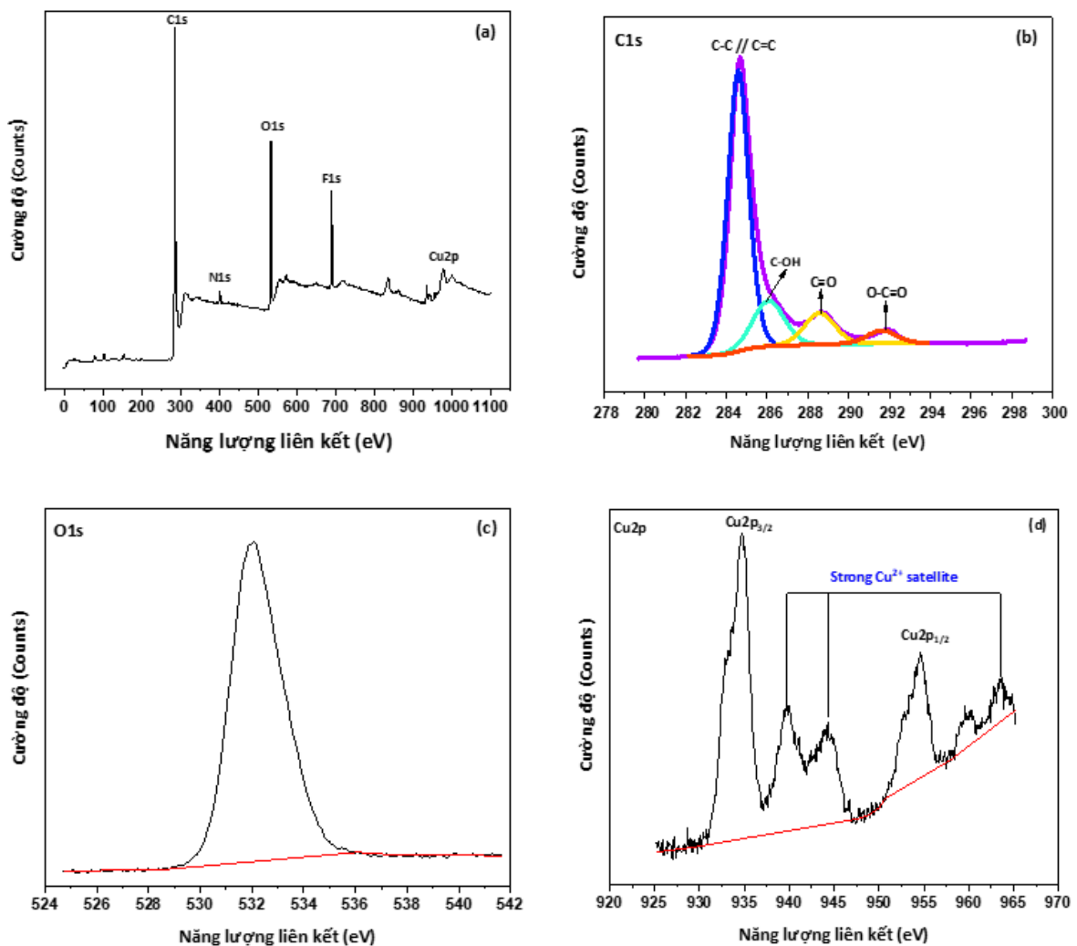
Hình 3. 45. Phổ XPS đầy đủ (a) và phổ C1s (b), O1s (c), Cu2p (d) của Cu-BTC tổng hợp bằng phương pháp kết tủa điện hóa
