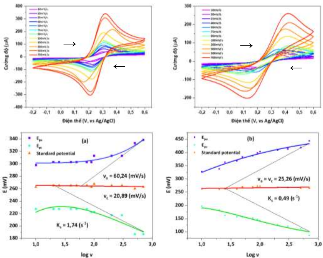
Hình 3. 50. Đường CV của điện cực Cu-BTC/GCE (a) và GCE (b) được ghi nhận trong dung dịch KCl 1M và hỗn hợp K_3[Fe(CN)_6]/K_4[Fe(CN)_6] 5mM với tốc độ quét từ 10 - 700mV/s
