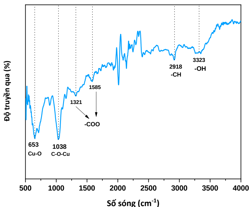
Hình 3. 43. Phổ FTIR của Cu-BTC tổng hợp bằng phương pháp kết tủa điện hóa
