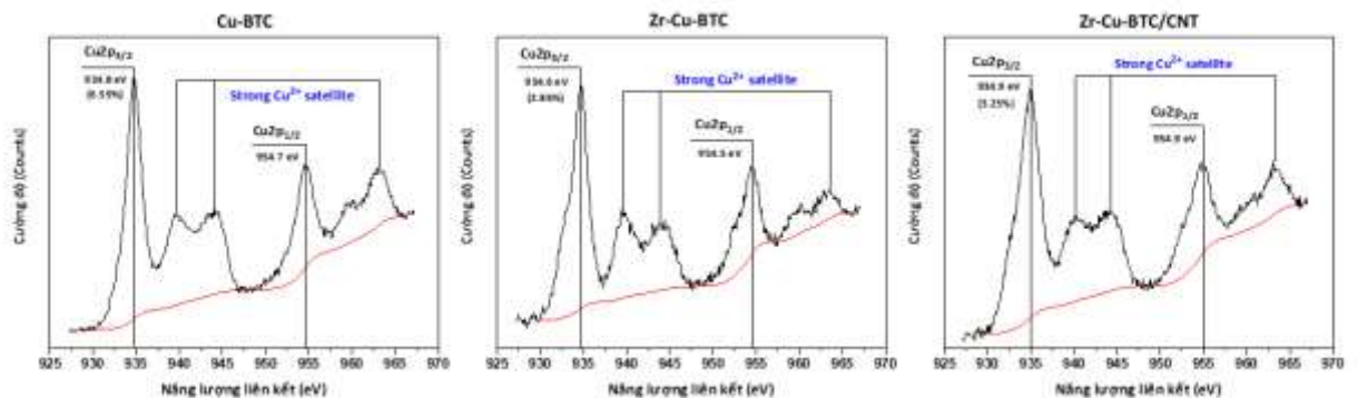
Hình 3. 6. Phổ XPS Cu2p của các mẫu Cu-BTC; Cu,Zr-BTC và Cu,Zr-BTC/CNT
