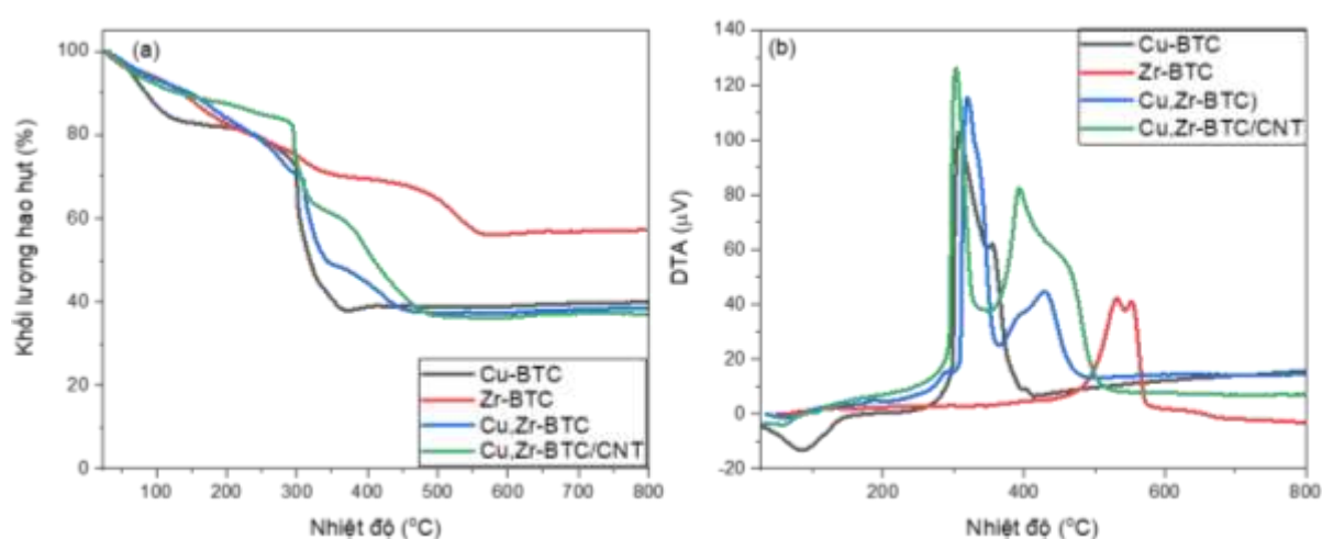
Hình 3. 13. Giảm đồ TG/DTA của vật liệu Cu-BTC; Zr-BTC; Cu,Zr-BTC và Cu,Zr-BTC/CNT
