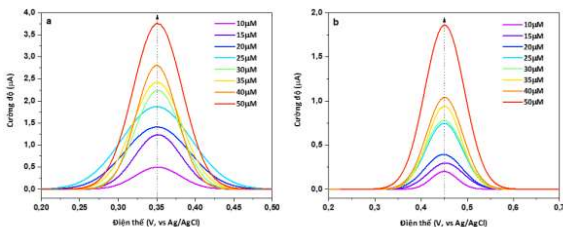
Hình 3. 59. Đường SWV của điện cực Cu-BTC/GCE (a) và GCE (b) ở các nồng độ PA khác nhau
