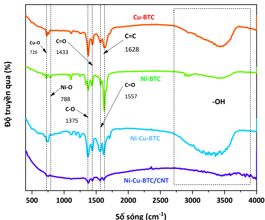
Hình 3. 31. Phổ FTIR của Cu-BTC; Ni-BTC; Cu,Ni-BTC; Cu,Ni-BTC/CNT
