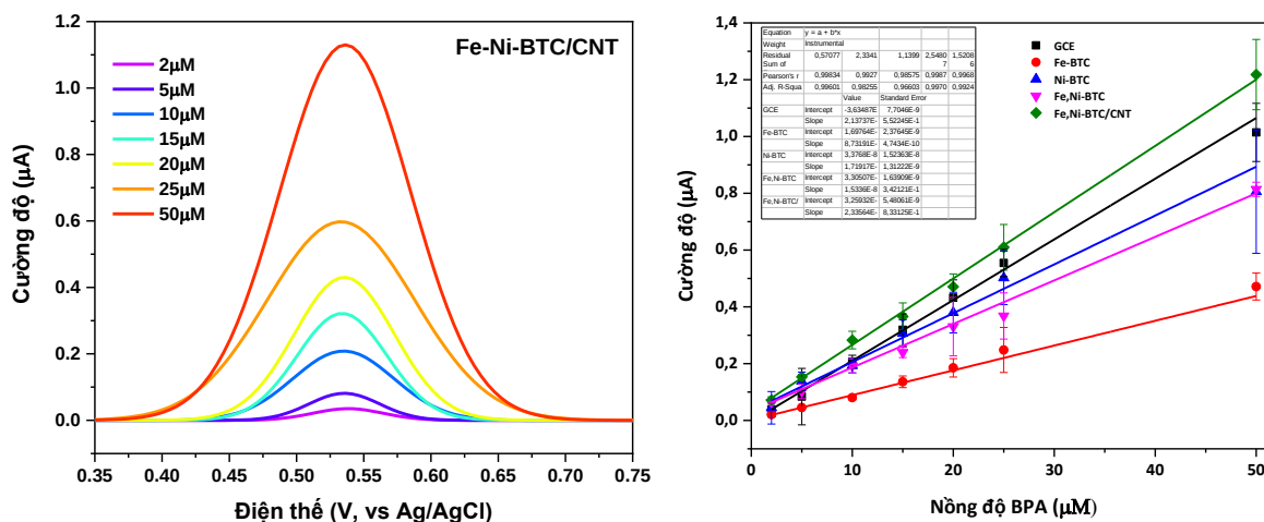
Hình 3. 29. Phổ DPV ghi trên điện cực Fe-Ni-BTC/CNT và đường chuẩn I-C của các điện cực biến tính và GCE
