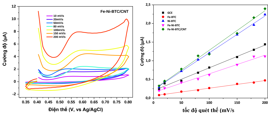
Hình 3. 28. Phổ CV ghi trên điện cực Fe-Ni-BTC/CNT trong dung dịch PBS 0,1M chứa BPA 50 \mu\text{M} và đường chuẩn I – v (ở dòng peak oxi hóa) với điện cực biến tính khác nhau
