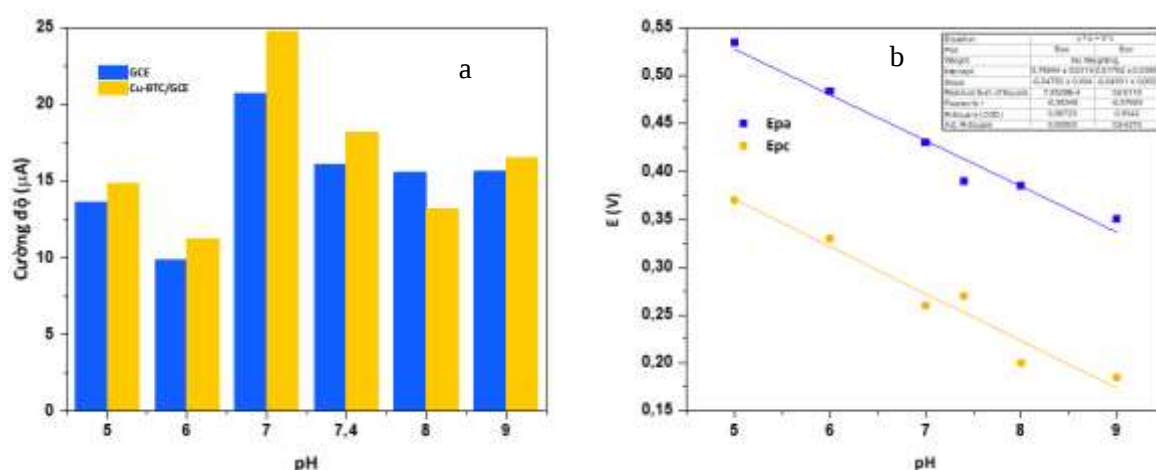
Hình 3. 58. Ảnh hưởng của pH đến cường độ đỉnh (a) và thế oxy hóa của PA (b)
