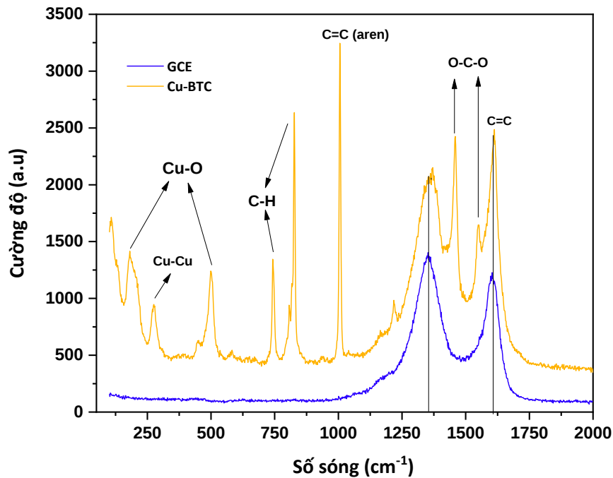
Hình 3. 44. Phổ Raman của GCE và Cu-BTC tổng hợp bằng phương pháp kết tủa điện hóa trên điện cực GCE
