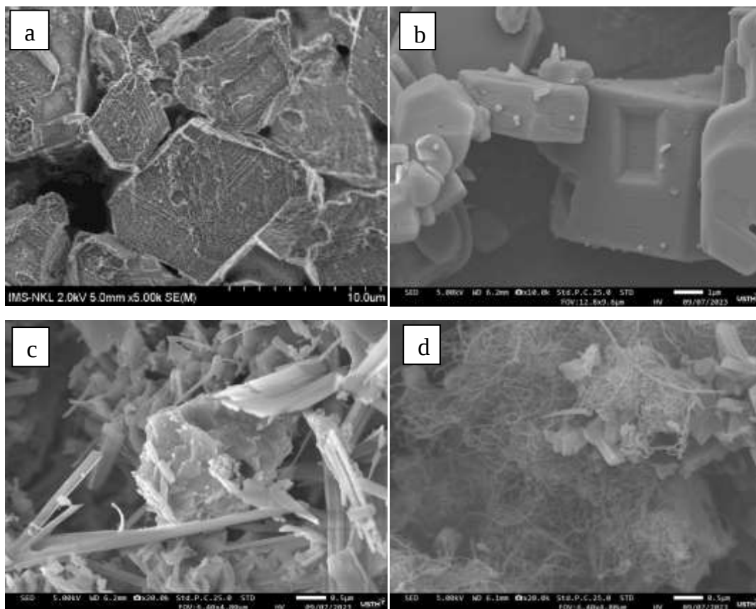
Hình 3. 30. Ảnh SEM của các mẫu vật liệu Cu-BTC (a), Ni-BTC (b), Cu,Ni-BTC (c) và Cu,Ni-BTC/CNT (d)
