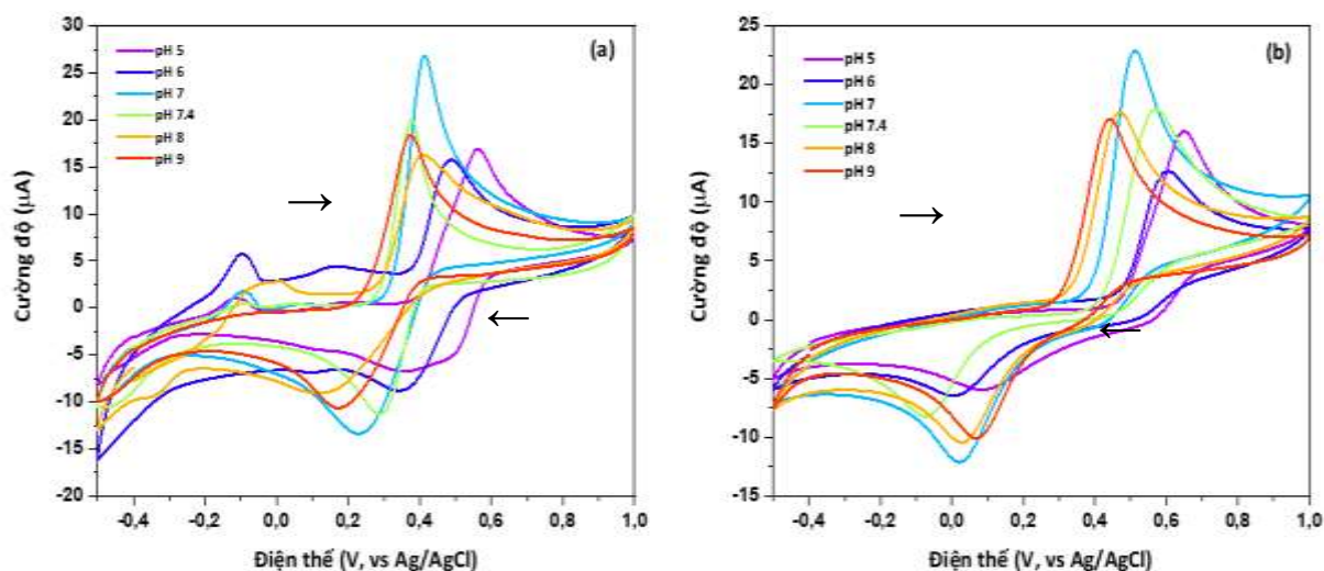
Hình 3. 57. Đường CV khảo sát ảnh hưởng của pH (5 - 9) trong dung dịch PA 1mM của điện cực Cu-BTC/GCE (a) và GCE (b)
