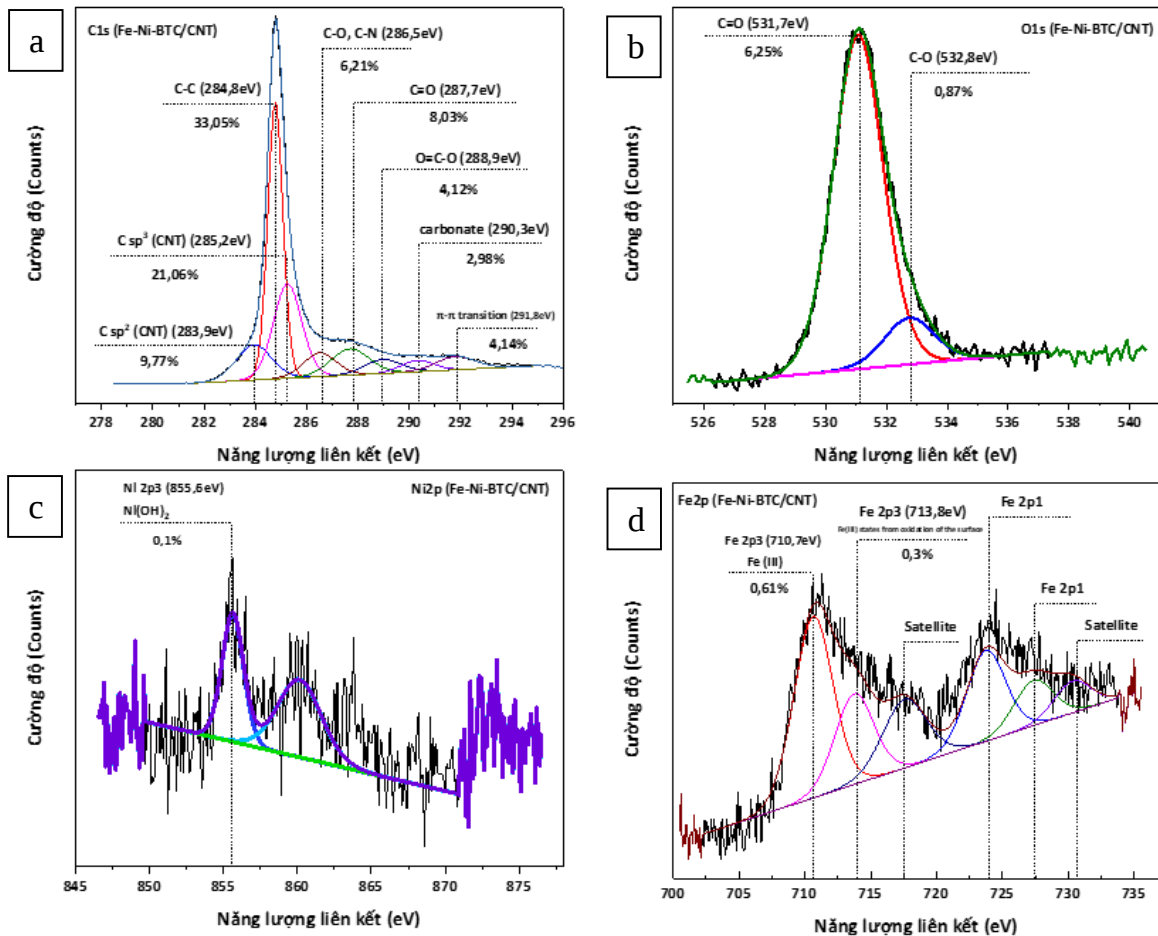
Hình 3. 24. Phổ XPS của Fe,Ni-BTC/CNT, (a) C1s, (b) O1s, (c) Ni2p, (d) Fe2p
