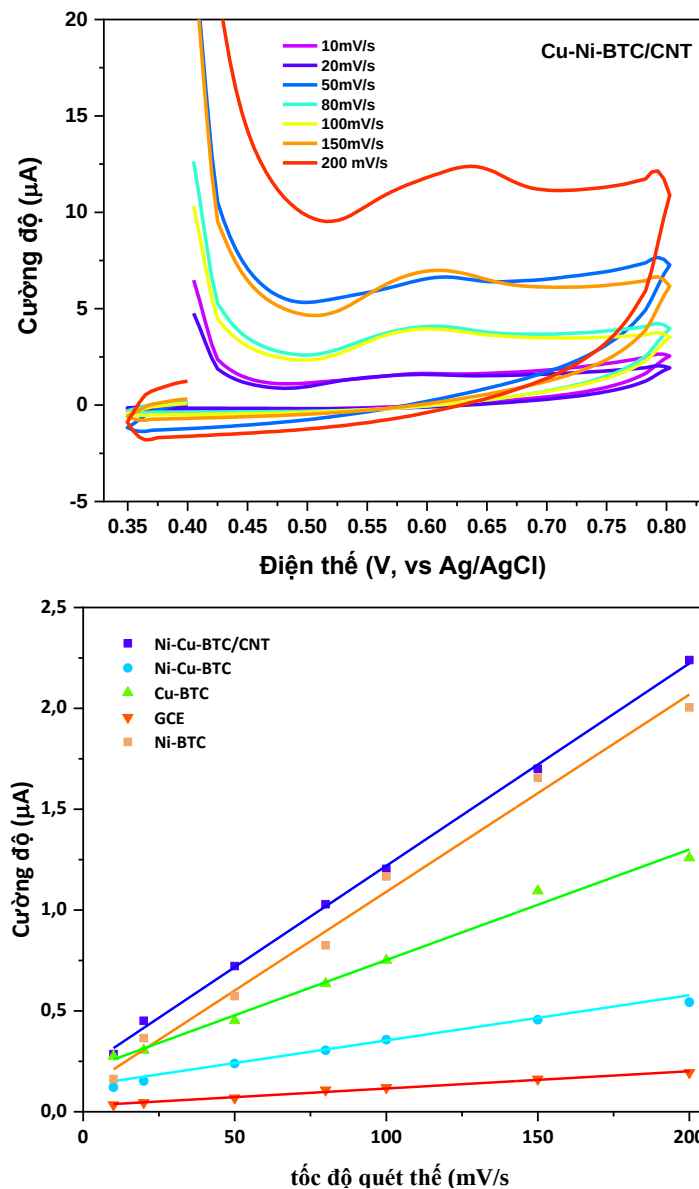
Hình 3. 37. Phổ CV ghi trên điện cực Cu,Ni-BTC/CNT trong dung dịch PBS 0,1M chứa BPA 50 \mu M và đường chuẩn I - \nu (ở dòng peak oxy hóa) với điện cực biến tính khác nhau
