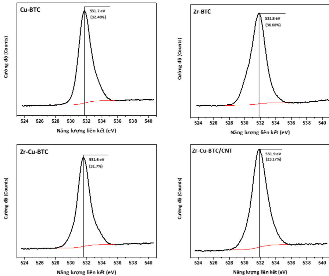
Hình 3. 5. Phổ XPS O1s của các mẫu
