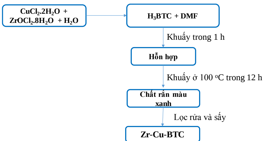
Hình 2. 2. Quy trình tổng hợp vật liệu Cu,Zr-BTC
