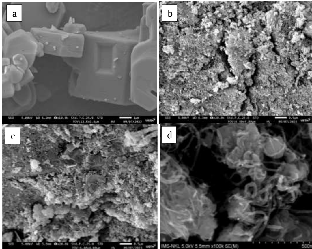
Hình 3. 20. Ảnh SEM của vật liệu Ni-BTC (a), Fe-BTC (b), Fe,Ni-BTC (c) và Fe,Ni- BTC/CNT (d)
