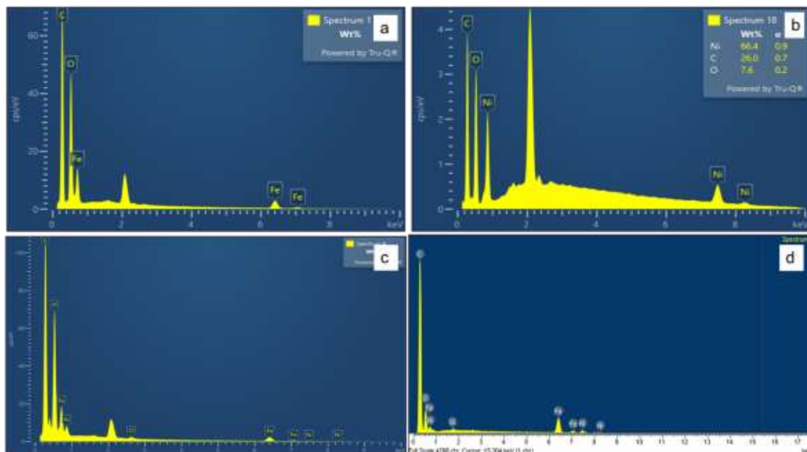
Hình 3. 21. Giản đồ EDX của vật liệu Fe-BTC (a), Ni-BTC (b), Fe,Ni-BTC (c) và Fe,Ni- BTC/CNT (d)
