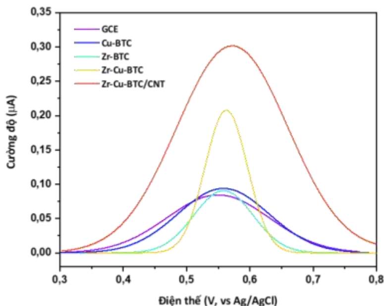
Hình 3. 18. Đường cong DPV ghi trên các điện cực khác nhau trong dung dịch PBS 0,1M chứa BPA 2 \mu M.
