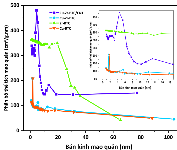
Hình 3.11. Đồ thị phân bố kích thước mao quản
