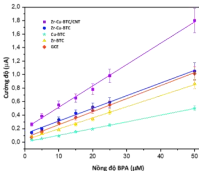
Hình 3. 1912. Đường chuẩn của BPA trên điện cực Cu,Zr-BTC/CNT/GCE
