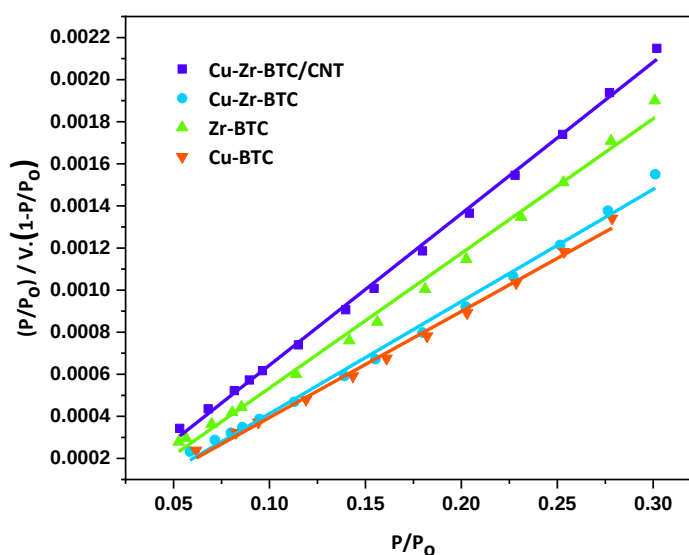
Hình 3.12. Đồ thị tuyến tính của phương trình BET
