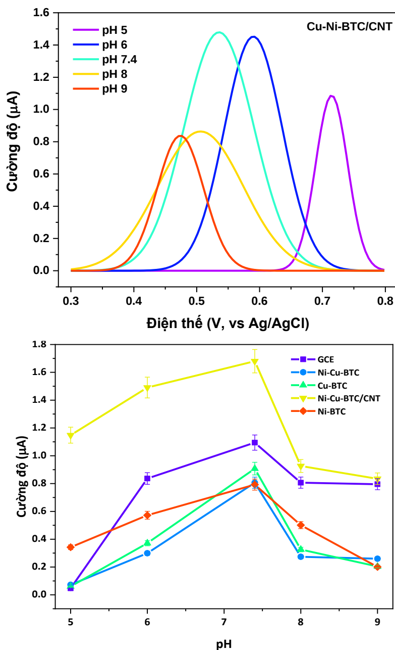
Hình 3. 35. Đồ thị biểu diễn cường độ peak của GCE biến tính bởi các vật liệu và GCE tại các pH khác nhau trong dung dịch BPS 0,1M chứa BPA 50 \mu M
