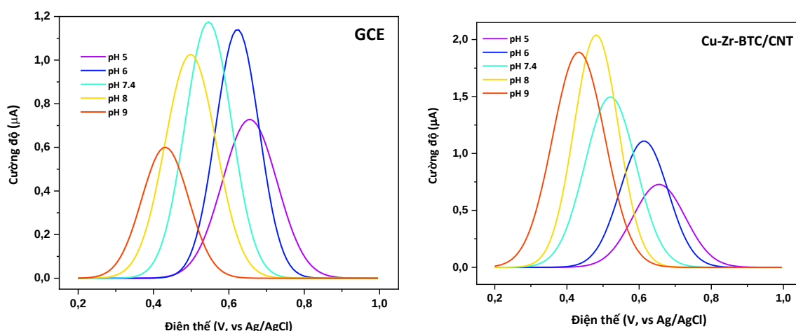
Hình 3. 1511. Ảnh hưởng của pH đến quá trình oxy hóa BPA trên bề mặt điện cực
