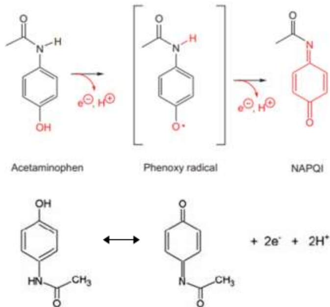
Hình 3. 56. Sơ đồ cơ chế oxi hóa của PA
