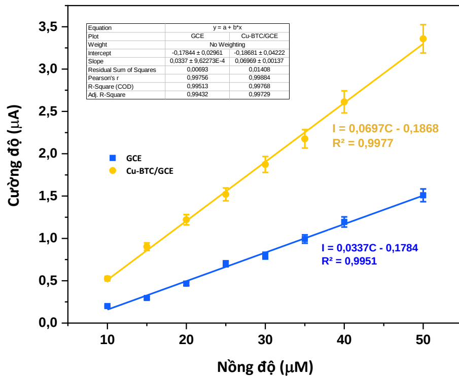
Hình 3. 60. Đường chuẩn I - C của PA trên điện cực Cu-BTC/GCE và GCE
