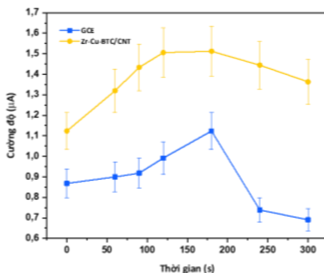
Hình 3. 16. Ảnh hưởng của thời gian hấp phụ BPA trên bề mặt điện cực
