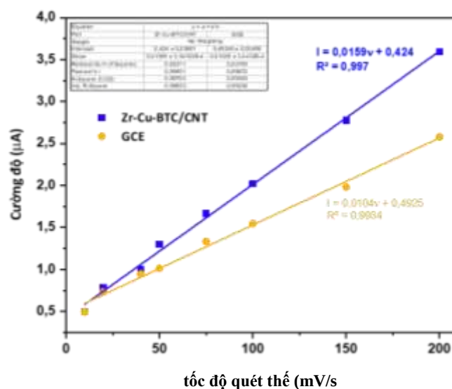
Hình 3. 17. Ảnh hưởng của tốc độ quét đến quá trình oxy hóa BPA trên bề mặt điện cực
