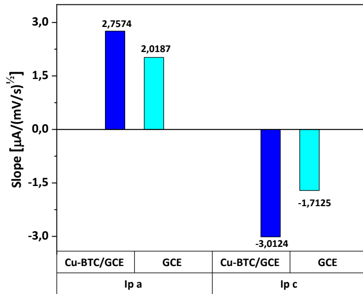
Hình 3. 55. Độ dốc của I_{pa} - v^{1/2} và I_{pc} - v^{1/2} của điện cực GCE và Cu-BTC/GCE
