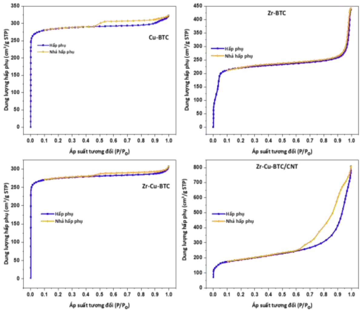
Hình 3. 10. Đường đẳng nhiệt hấp phụ-khử hấp phụ N_2 của các mẫu Cu-BTC; Zr-BTC; Cu,Zr-BTC và Cu,Zr-BTC/CNT
