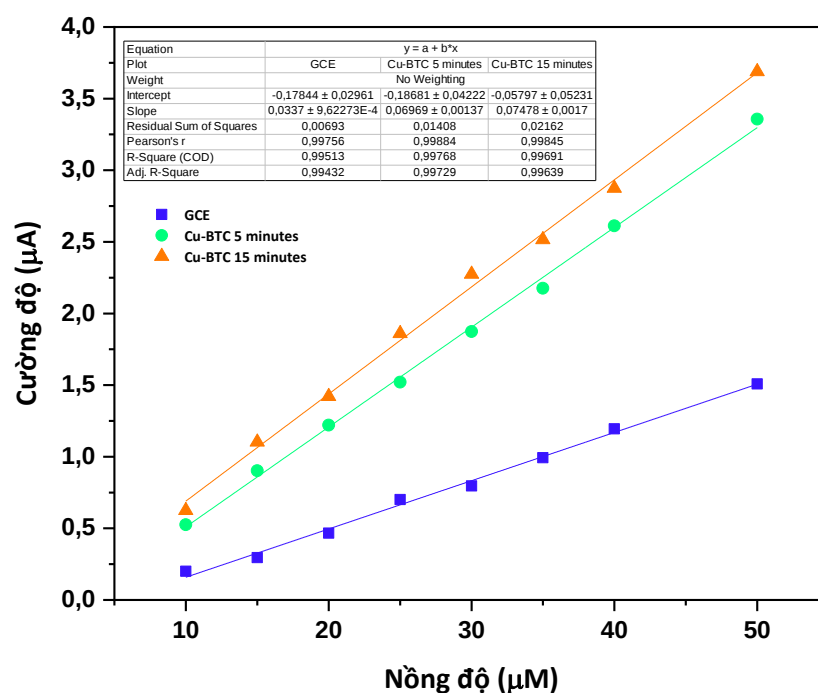
Hình 3. 61. Đường chuẩn I - C của của PA trên các điện cực GCE và Cu-BTC/GCE trong thời gian tổng hợp khác nhau
