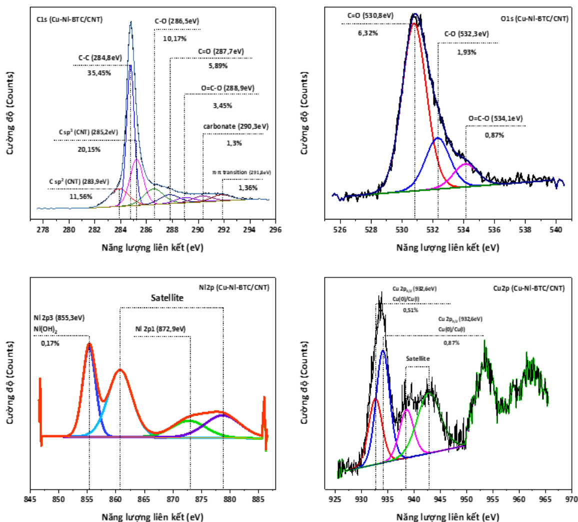
Hình 3. 34. Phổ C1s, O1s, Cu2p và Ni2p của Cu,Ni-BTC/CNT
