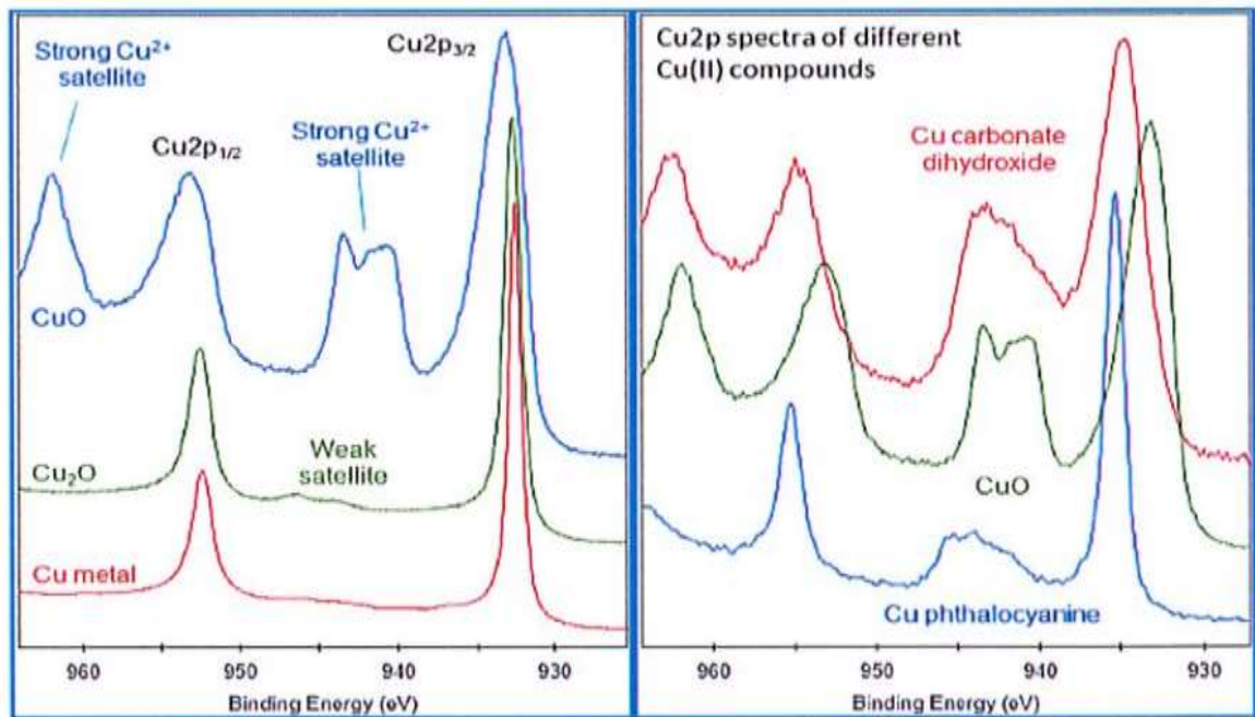
Hình 3. 46. Các trạng thái khác nhau của Cu được tìm thấy trong cấu trúc Cu-BTC tổng hợp bằng phương pháp kết tủa điện hóa
