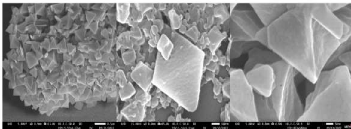
Hình 3. 42. Ảnh SEM của Cu-BTC tổng hợp bằng phương pháp kết tủa điện hóa trên GCE
