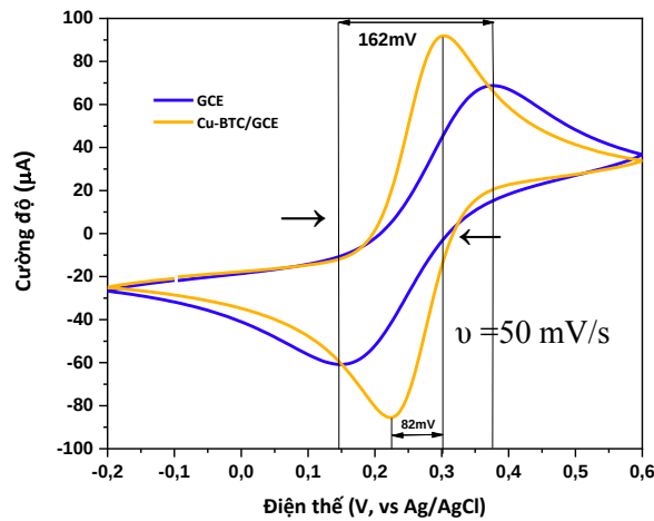
Hình 3. 49. Đường CV trong dung dịch K_3[Fe(CN)_6] / K_4[Fe(CN)_6] của điện cực GCE và Cu-BTC/GCE với tốc độ quét 50mV/s
