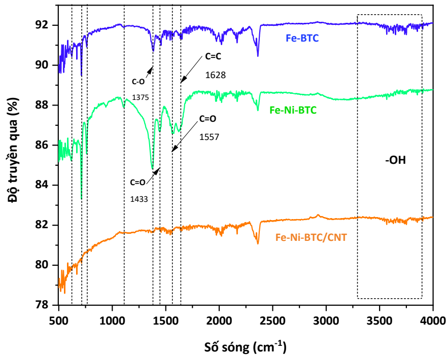
Hình 3. 22. Phổ FTIR của Fe-BTC, Fe,Ni-BTC và Fe,Ni-BTC/CNT
