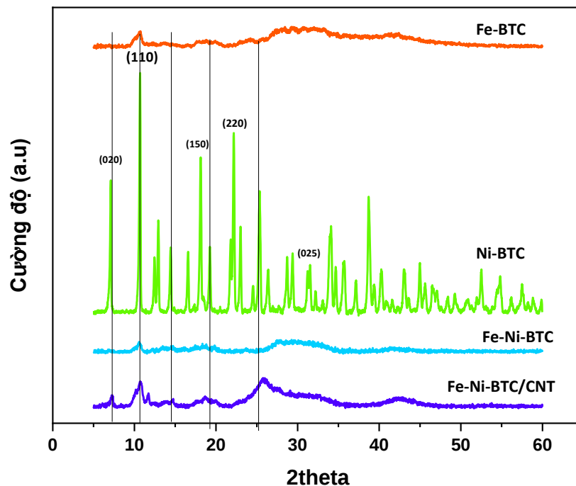
Hình 3. 23. Giản đồ XRD của của Fe-BTC; Ni-BTC; Fe,Ni-BTC và Fe,Ni-BTC/CNT
