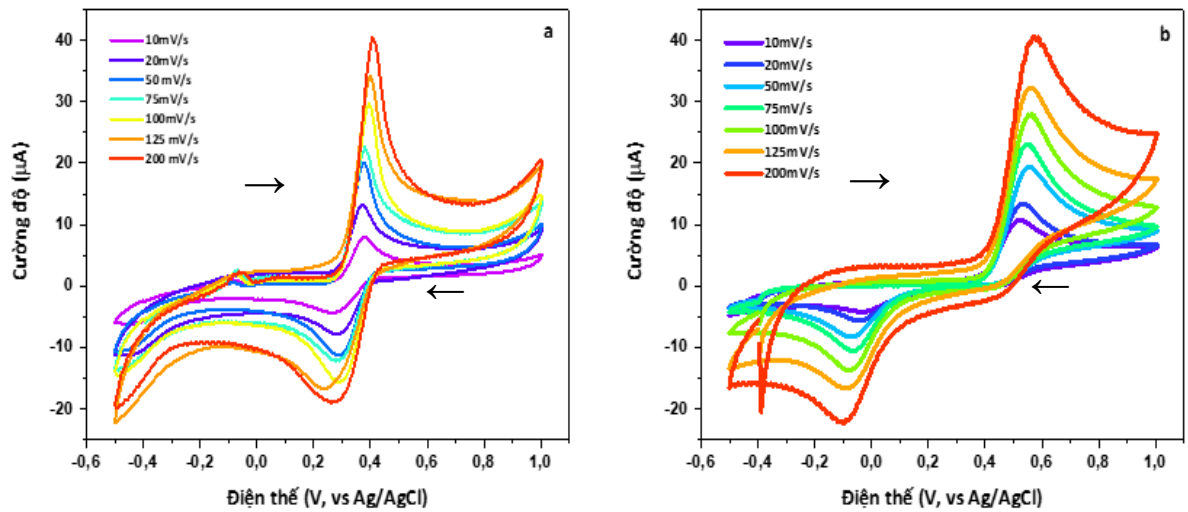
Hình 3. 53. Đường CV của điện cực Cu-BTC/GCE (a) và GCE (b) trong dung dịch PA 1mM khi thay đổi tốc độ quét
