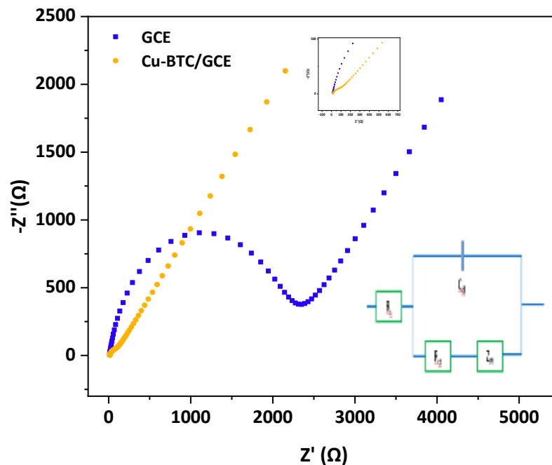
Hình 3. 51. Đồ thị Nyquist giữa điện cực GCE và Cu-BTC/GCE trên dải tần số từ 10^{-1} - 10^5 Hz với biên độ E_o = 190 mV
