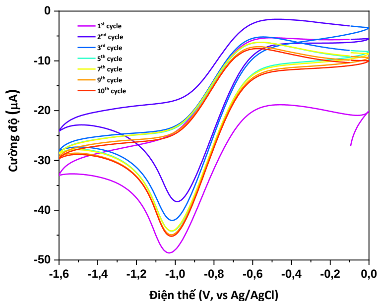
Hình 3. 39. Đường CV tổng hợp Cu-BTC
