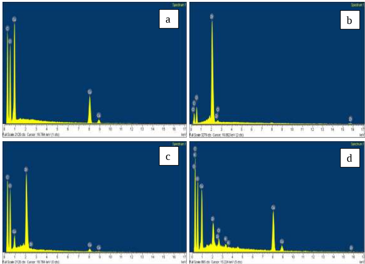
Hình 3. 2. Giải đồ EDX của vật liệu Cu-BTC (a), Zr-BTC (b), Cu,Zr-BTC (c) và Cu,Zr-BTC/CNT (d)
