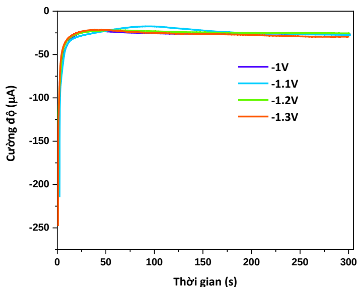
Hình 3. 41. Đường CA tổng hợp Cu-BTC khi áp các thế khác nhau
