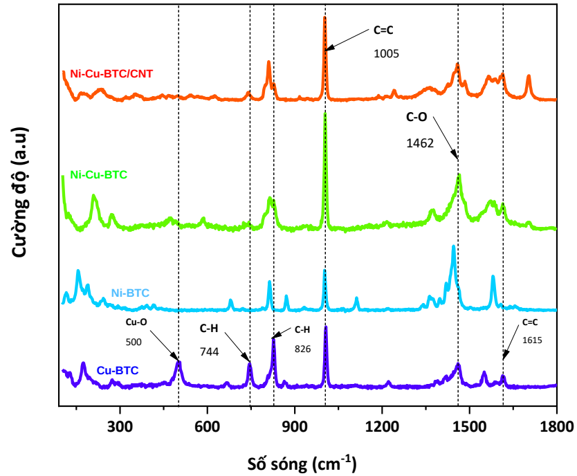
Hình 3. 32. Phổ Raman của Ni-BTC; Cu-BTC; Cu,Ni-BTC; Cu,Ni-BTC/CNT
