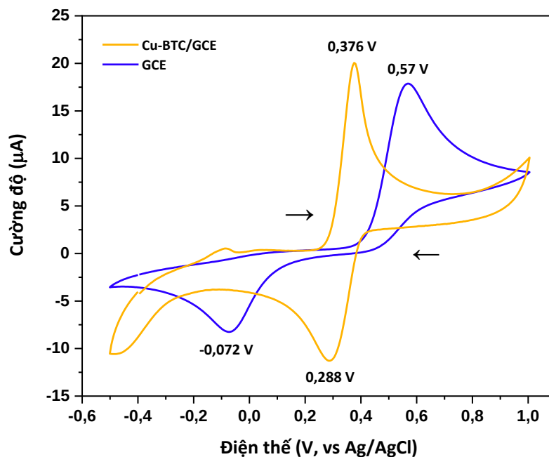
Hình 3. 52. Đường CV của điện cực Cu-BTC/GCE và GCE trong dung dịch chứa PA 1mM trong PBS (pH7,4)
