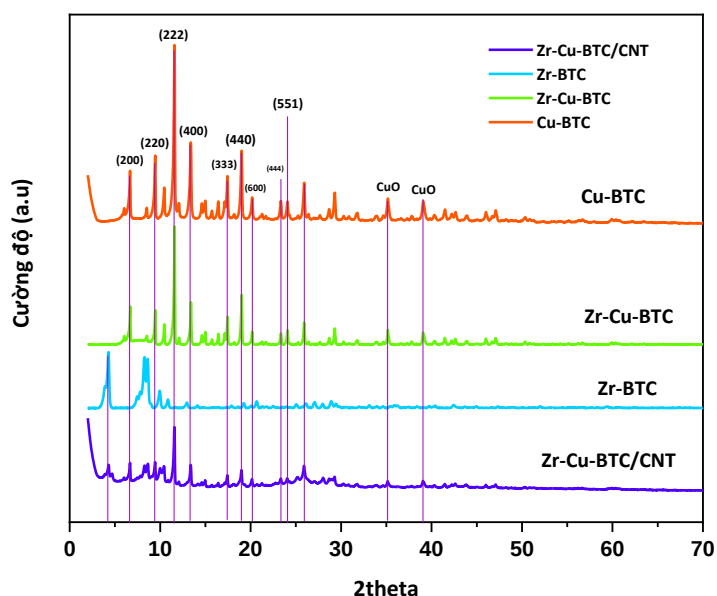
Hình 3. 8. Biểu đồ XRD của vật liệu Cu-BTC; Zr-BTC; Cu,Zr-BTC và Cu,Zr-BTC/CNT
