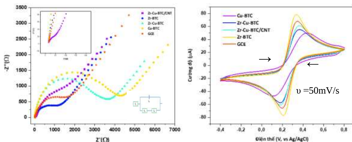
Hình 3. 14. Giảm đồ EIS và CV của vật liệu Cu-BTC; Zr-BTC; Cu,Zr-BTC và Cu,Zr-BTC/CNT
