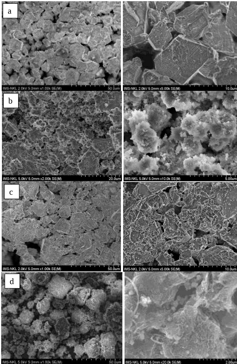
Hình 3. 1. Ảnh SEM của vật liệu Cu-BTC (a), Zr-BTC (b), Cu,Zr-BTC (c) và Cu,Zr-BTC/CNT (d) ở các độ phóng đại khác nhau
