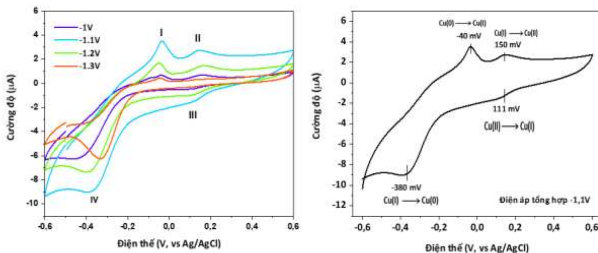
Hình 3. 48. Đường CV của điện cực Cu-BTC/GCE trong KCl 100mM
