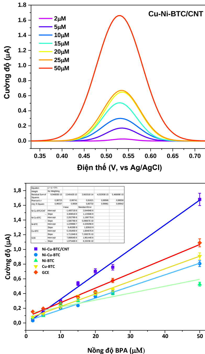
Hình 3. 38. Phổ DPV ghi trên điện cực Cu,Ni-BTC/CNT và đường chuẩn I-C của các điện cực biến tính và GCE
