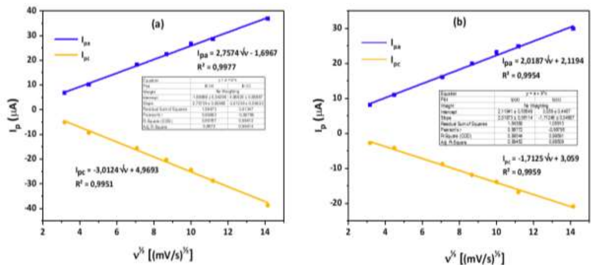
Hình 3. 54. Đường chuẩn I_p - v^{1/2} với điện cực Cu-BTC/GCE (a) và GCE (b)
