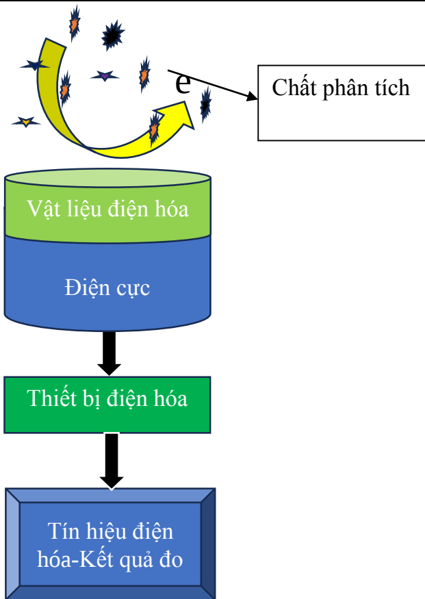
Hình 1. 9. Sơ đồ nguyên lý của cảm biến điện hóa
