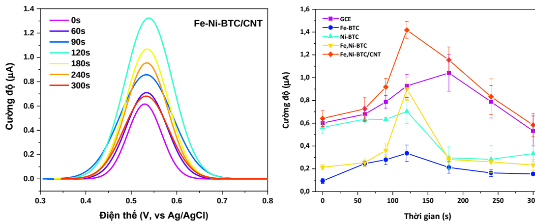
Hình 3. 27. Đồ thị biểu diễn cường độ dòng peak của Fe,Ni-BTC/CNT/GCE và GCE tại thời gian hấp phụ khác nhau trong dung dịch chứa BPA 50μM
