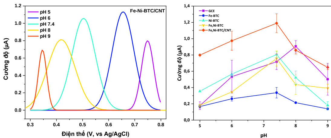
Hình 3. 26. Đồ thị biểu diễn cường độ dòng peak của Fe,Ni-BTC/CNT/GCE và GCE tại các pH khác nhau của dung dịch chứa BPA 50μM
