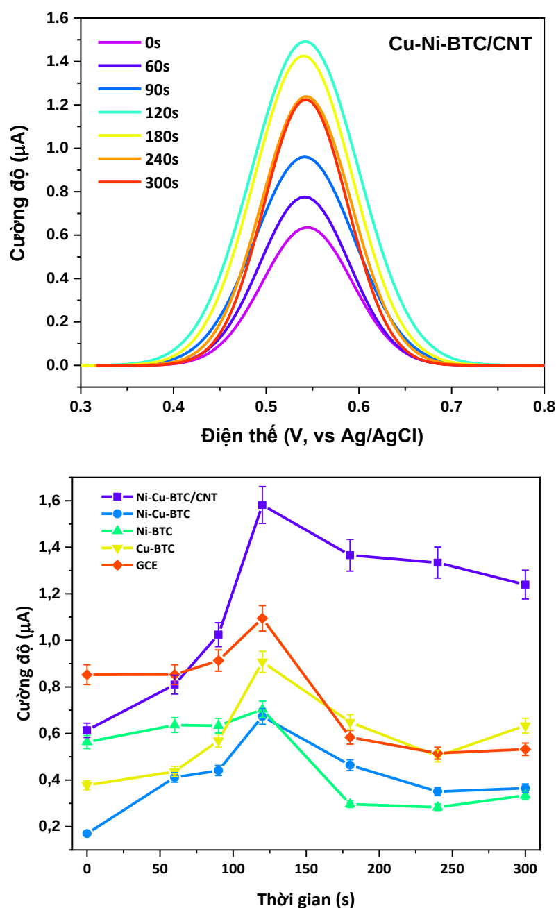
Hình 3. 36. Ảnh hưởng của thời gian hấp phụ BPA trên bề mặt điện cực
