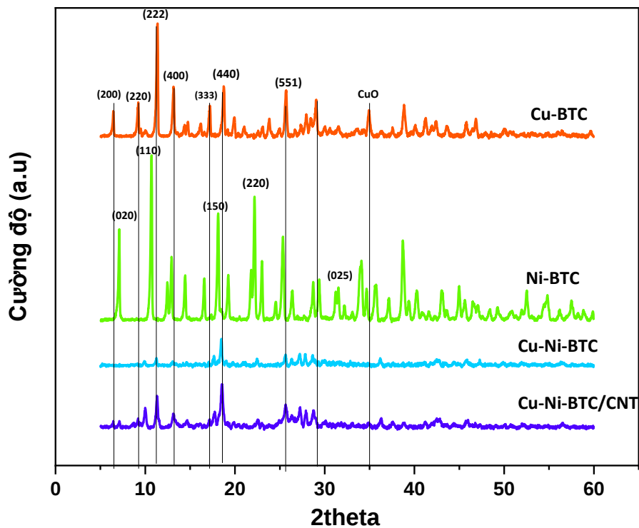
Hình 3. 33. Giảm đồ XRD của các vật liệu
