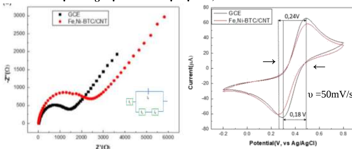
Hình 3. 25. Giải đồ EIS và CV của Fe,Ni-BTC/CNT/GCE và GCE
