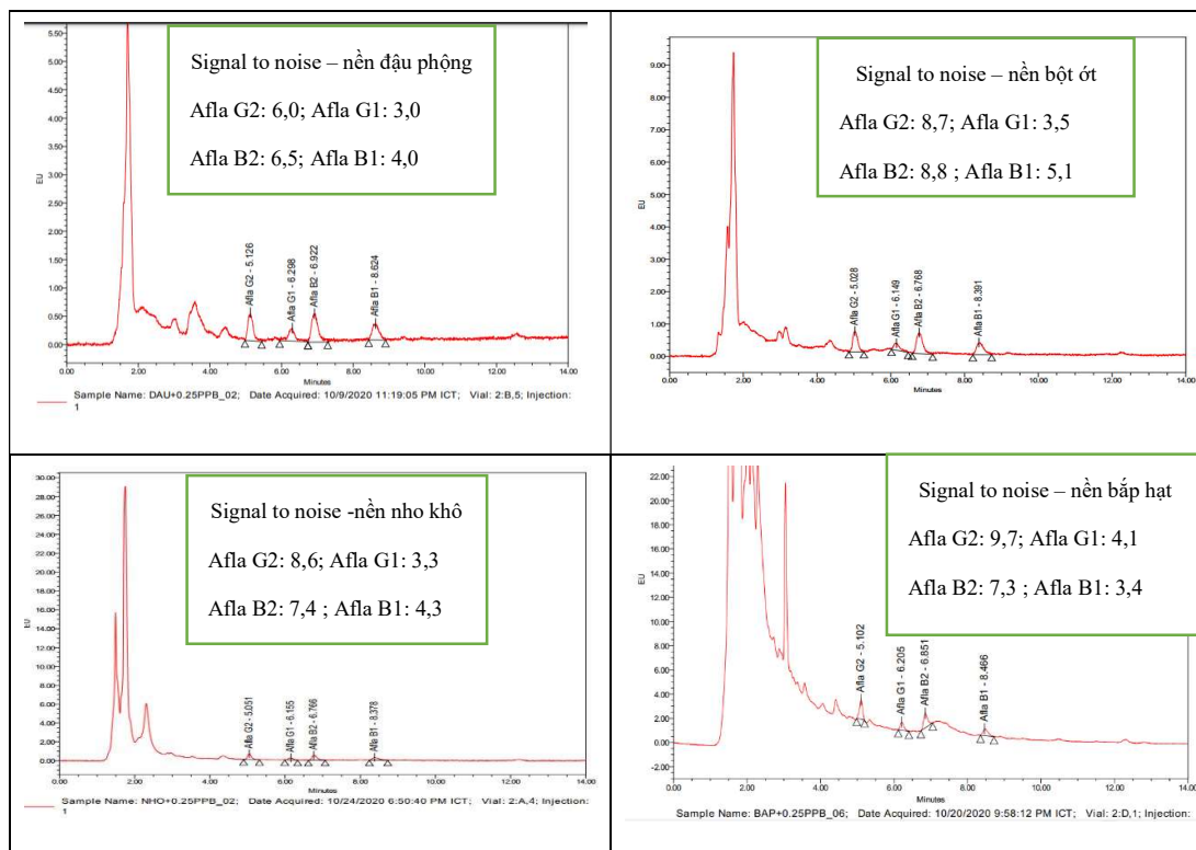
Hình 3.6: Sắc ký đồ giới hạn phát hiện của phương pháp trên nền mẫu đậm phồng, bột ột, nhỏ khô và bắp hạt
