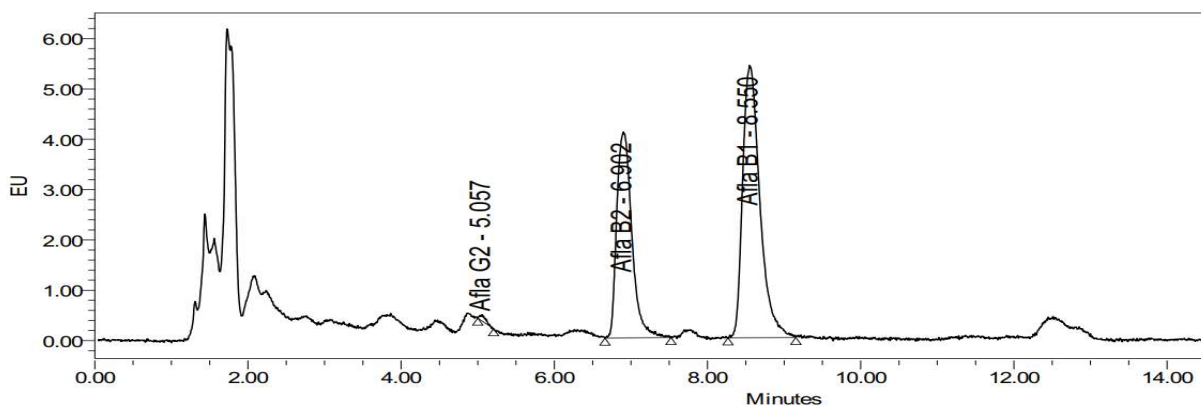
Hình PL3.5. Phổ sắc ký của mẫu bột ớt (MM12101_02027) phát hiện độc tố AFG1, AFB2 và AFB1; với nồng độ tương ứng là 2,26; 0,54 và 10,3 \mu\text{g/kg}
