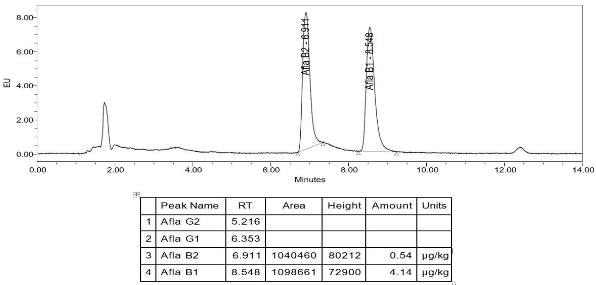
Hình PL3.2. Phổ sắc ký của mẫu đậu phộng thô (MM12101_02084) phát hiện độc tố AFB2 và AFB1, với nồng độ tương ứng là 0,54 và 4,14 µg/kg
