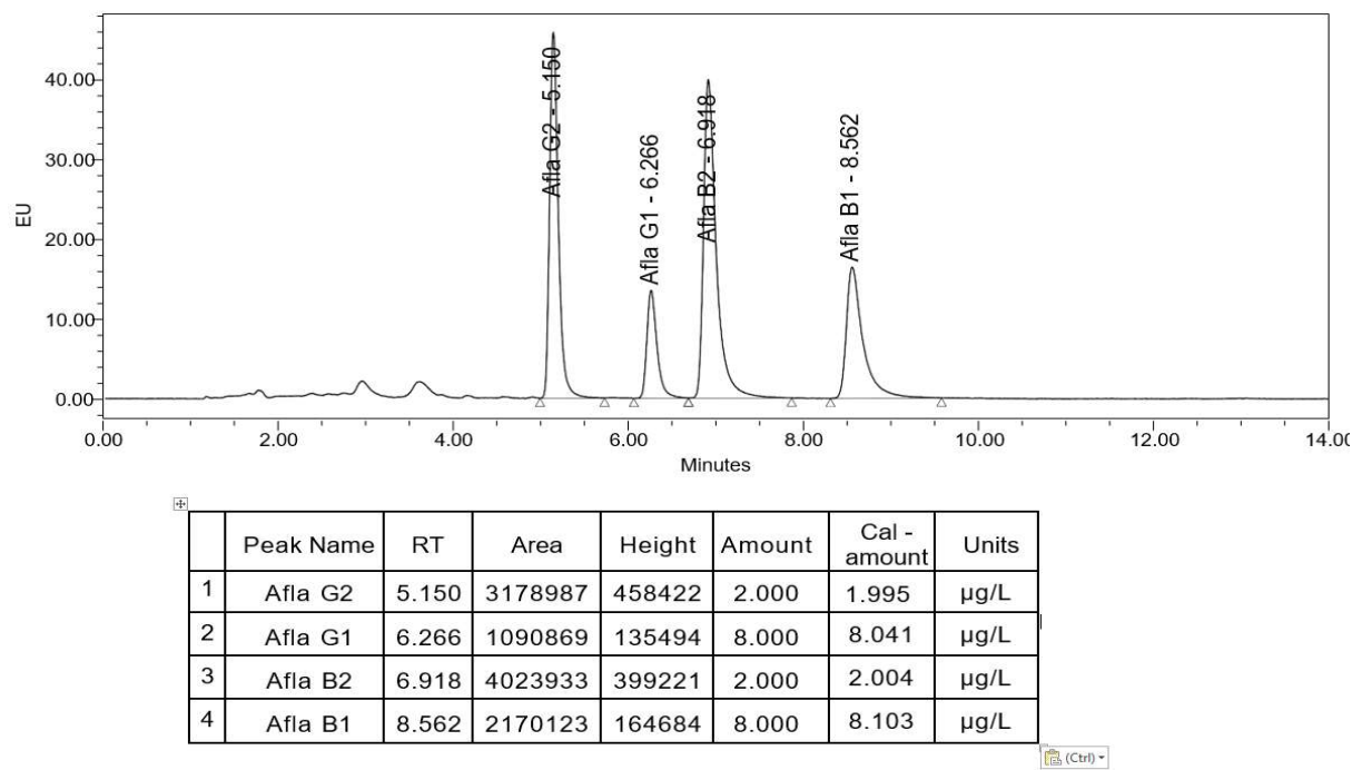
Hình PL3.1. Phổ sắc ký của dung dịch chuẩn hỗn hợp aflatoxin, nồng độ 20 µg/L (hình trên); và bảng tóm tắt thông số sắc ký của từng chất (hình dưới) bao gồm thời gian lưu (RT), diện tích (Area), chiều cao (Height), hàm lượng lý thuyết (Amount) và thực tế (Cal-amount), đơn vị (Units)
