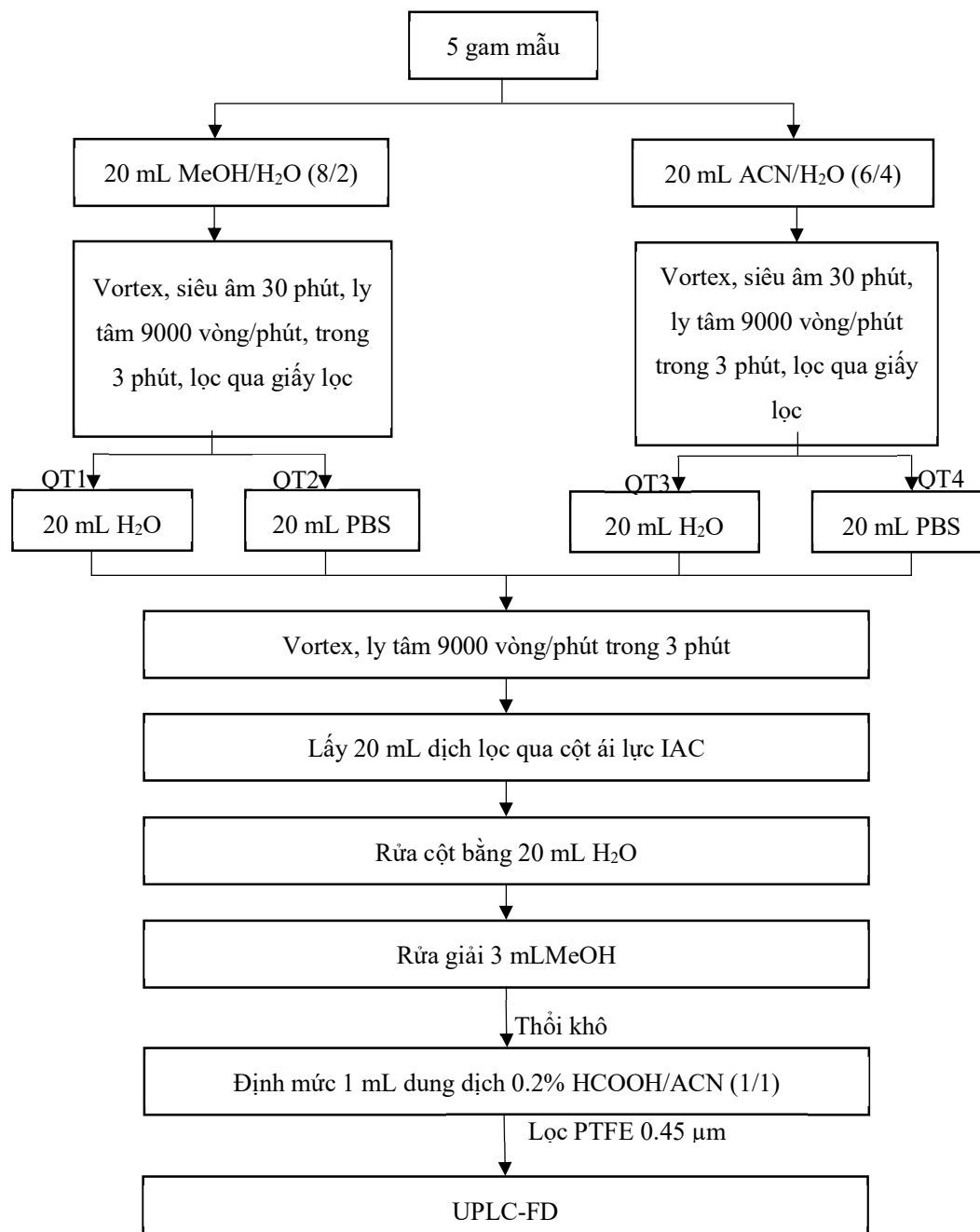
Hình 2.2: Lưu đồ qui trình chiết dự kiến AF trong nền mẫu đậu phộng bột ót, nho khô và bắp hạt
