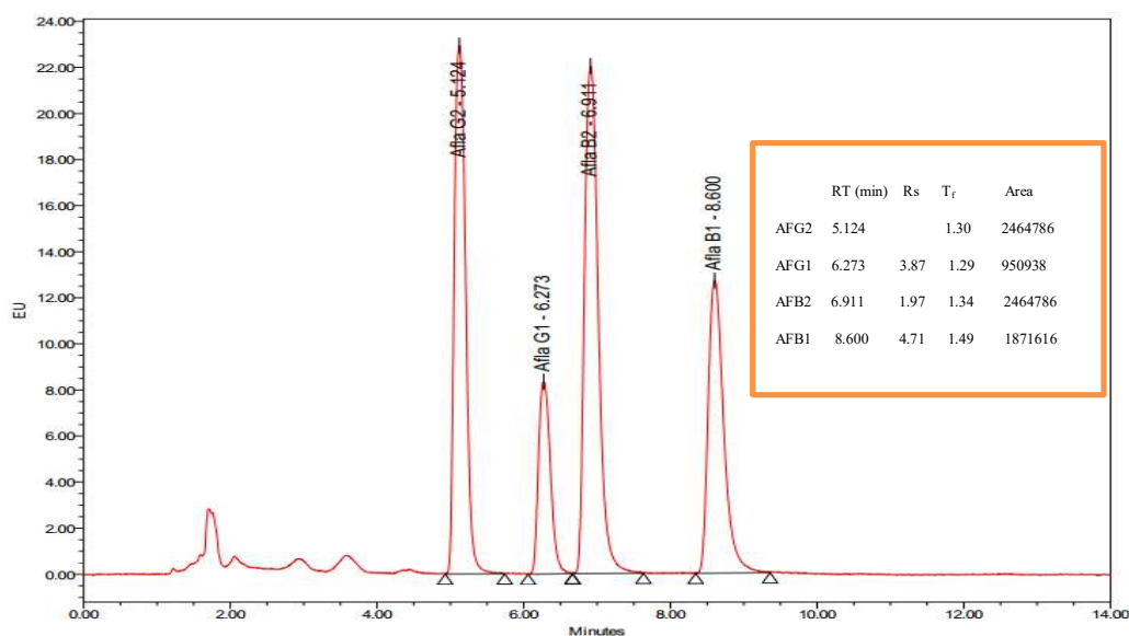
Hình 3.2: Sắc ký đồ chuẩn aflatoxin (B1, B2, G1 và G2) nồng độ 12,5 µg/L minh họa tính ổn định của tín hiệu các pic.
