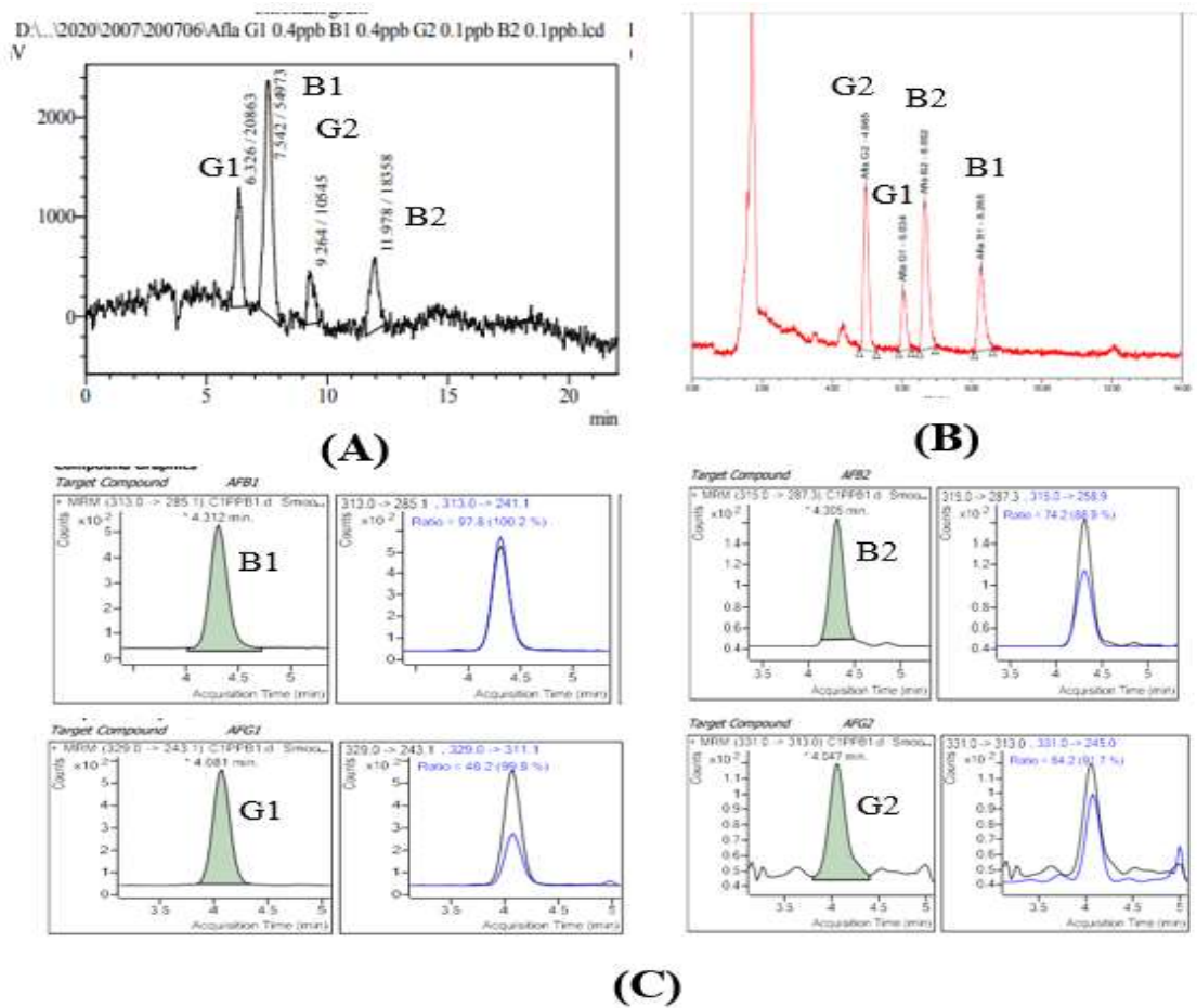
Hình 1.3: Sắc ký của dung dịch chuẩn aflatoxin (1 µg/L) được tiêm với ba phương pháp khác nhau: (A) HPLC-FD có tạo dẫn xuất trước cột; (B) UPLC-FD không tạo dẫn xuất; và (C) LC/MS/MS [97]
