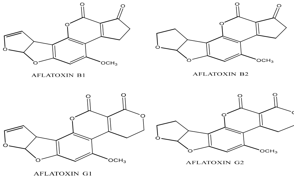
Hình 1.1: Cấu trúc phân tử các loại aflatoxin [63]
