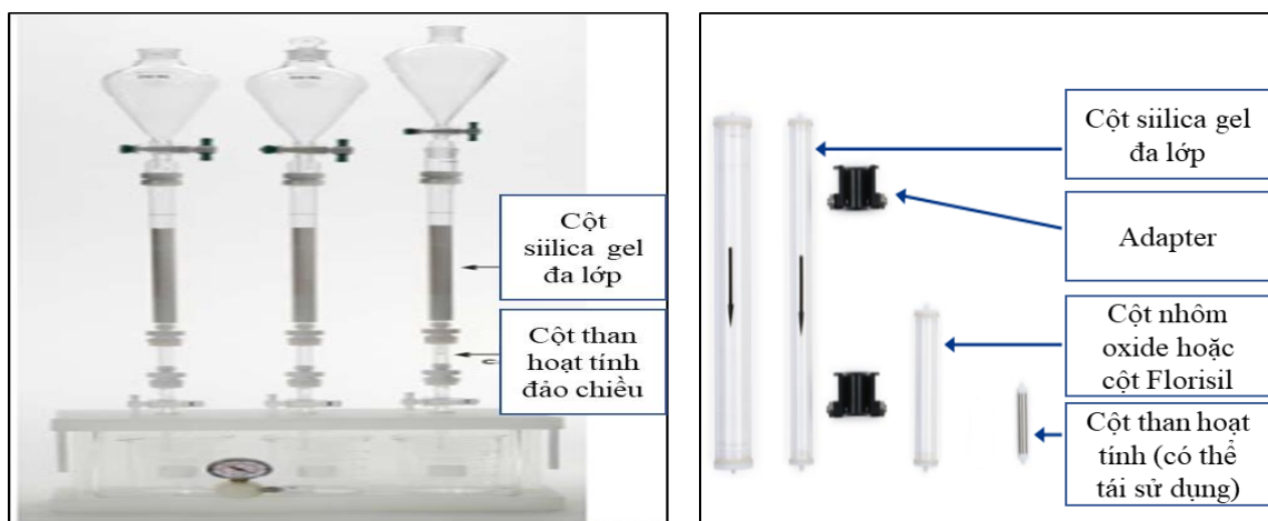
Hình 1.6 Cột làm sạch mẫu dùng một lần của hãng Supelco, LC Tech
