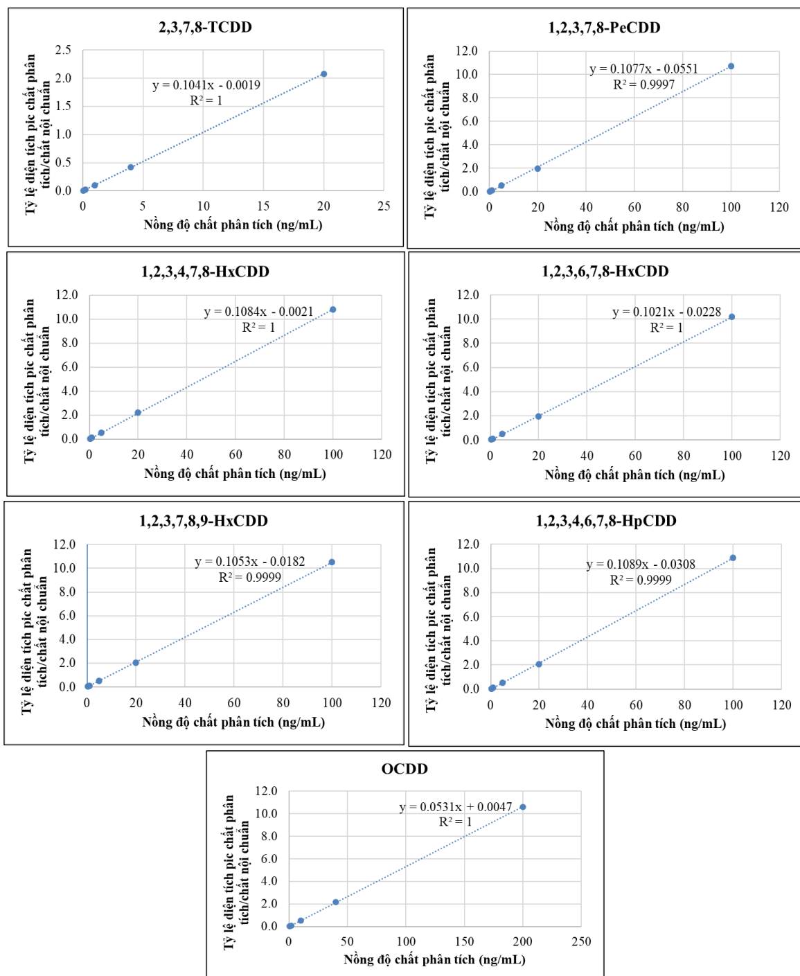
Hình PL1.1 Đường chuẩn của các đồng loại PCDDs
