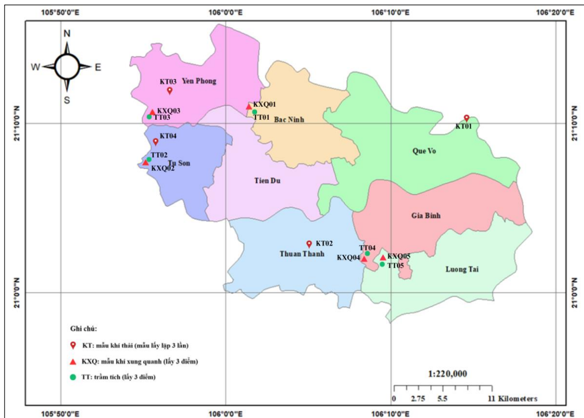
Hình 2.1 Các vị trí lấy mẫu khí thải, không khí xung quanh và trầm tích tại Bắc Ninh
