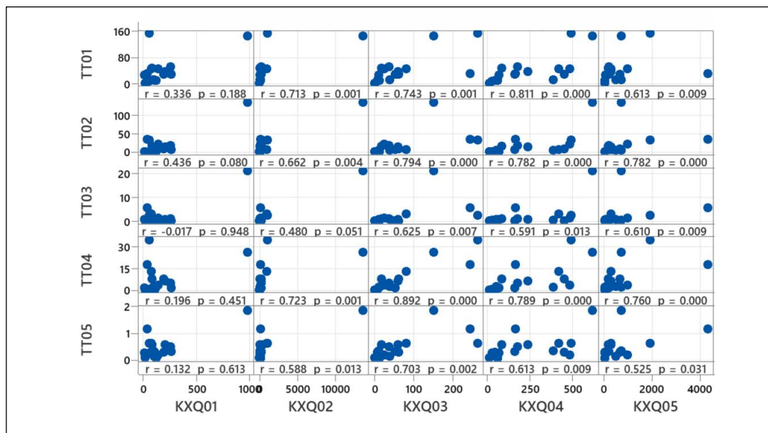
Hình 3.33 Tương quan Spearman về hàm lượng PCDD/Fs trong mẫu không khí xung quanh và trầm tích tại các làng nghề
