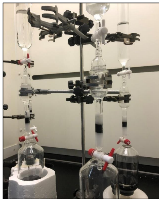
Rửa giải cột than hoạt tính
