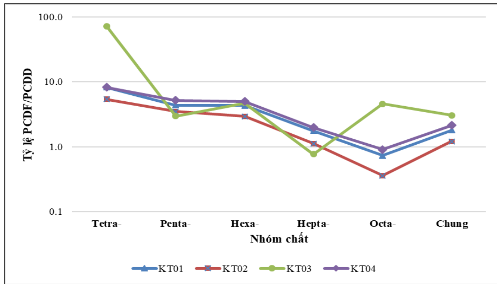
Hình 3.24 Tỷ lệ nồng độ PCDF và PCDD ( R_{DF/DD} ) trong mẫu khí thải
