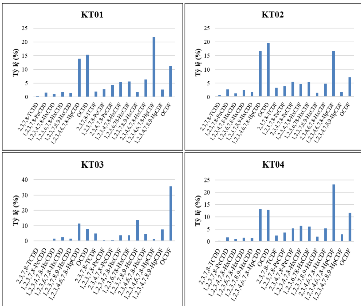
Hình 3.25 Tỷ lệ phần trăm về hàm lượng của các đồng loại PCDD/Fs
