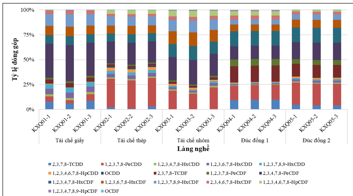
Hình 3.29 Tỷ lệ phần trăm về hàm lượng TEQ của các đồng loại PCDD/Fs trong các mẫu không khí xung quanh
