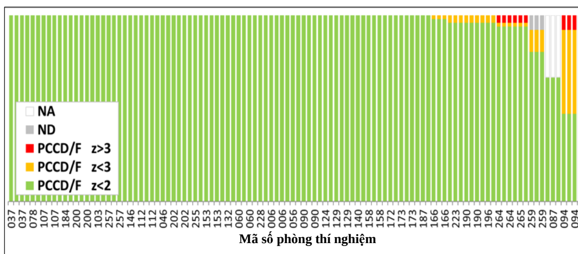
Hình 3.22 Kết quả phân tích PCDD/Fs của các phòng thí nghiệm đối với nền mẫu thử nghiệm thành thạo trầm tích
