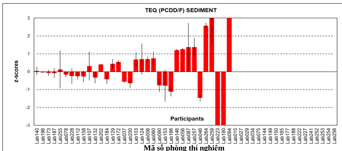
Hình 3.23 Kết quả TEQ-PCDD/Fs các phòng thí nghiệm tham gia phân tích mẫu thử nghiệm thành thạo trầm tích
