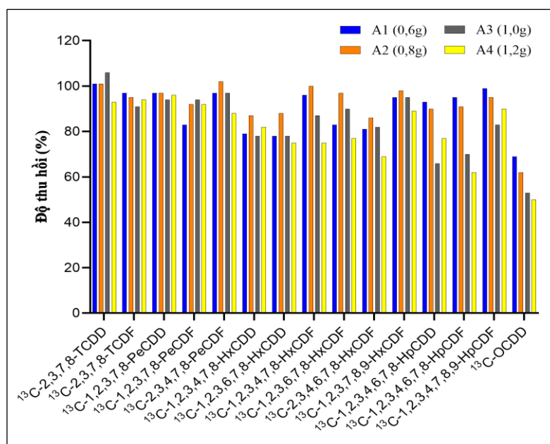
Hình 3.6 So sánh độ thu hồi các chất chuẩn 13 C 12 M1613 khảo sát khối lượng cột than hoạt tính
