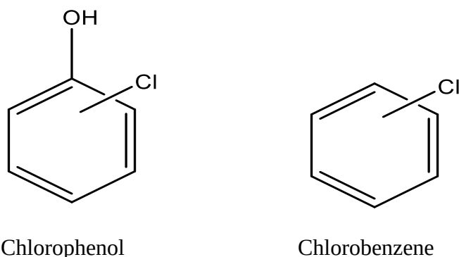
Hình 1.2 Các tiền chất hình thành PCDD/Fs
