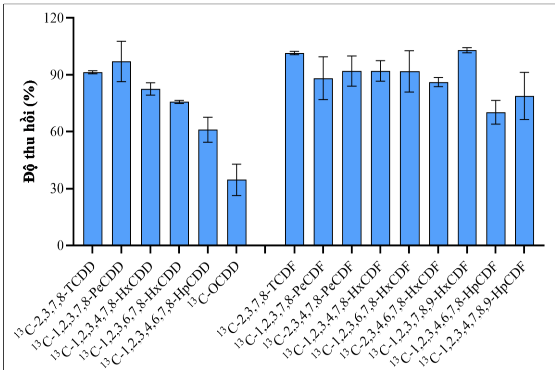
Hình 3.20 Độ thu hồi các chất chuẩn 13 C 12 trong mẫu trầm tích EDF-5184
