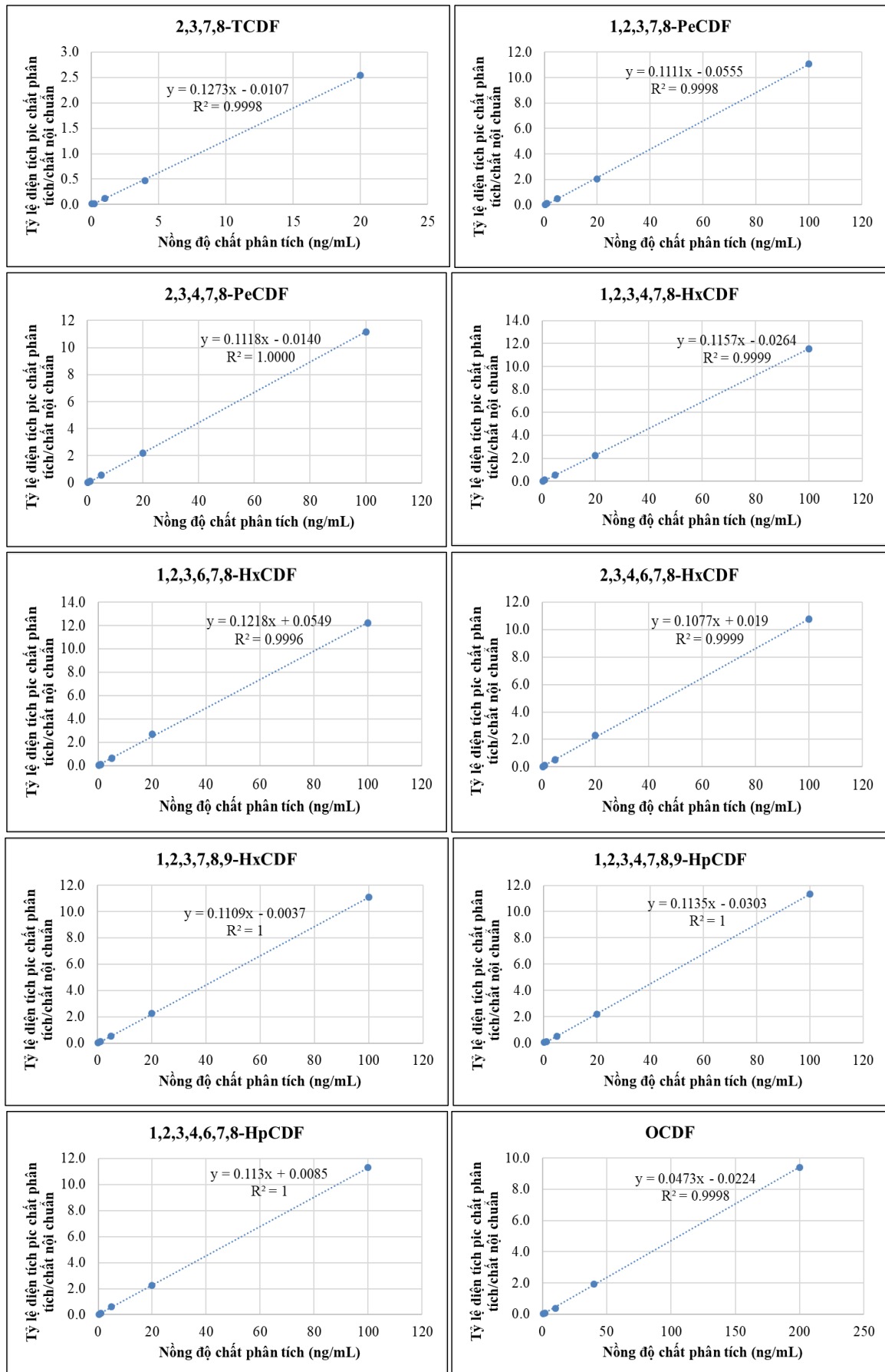
Hình PL1.2 Đường chuẩn của các đồng loại PCDFs
