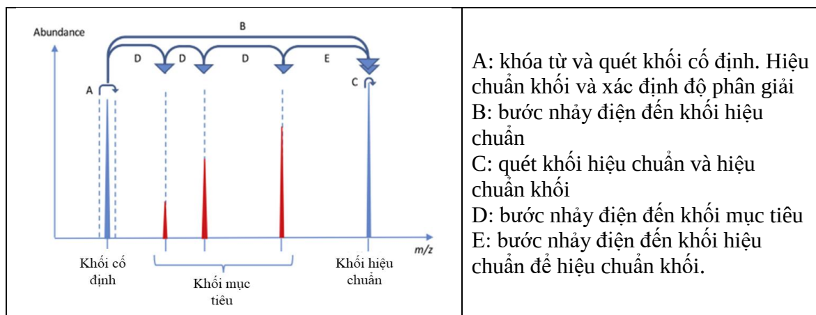
Hình 1.7 Hiệu chuẩn khối nội bộ và phát hiện khối mục tiêu trong quá trình MID trong thiết bị DFS
