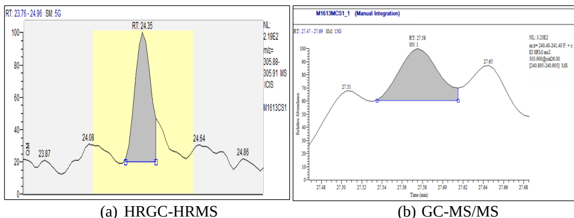
Hình 3.3 Sắc đồ chất chuẩn 2,3,7,8-TCDF tại điểm chuẩn MCS1 phân tích trên 2 thiết bị
