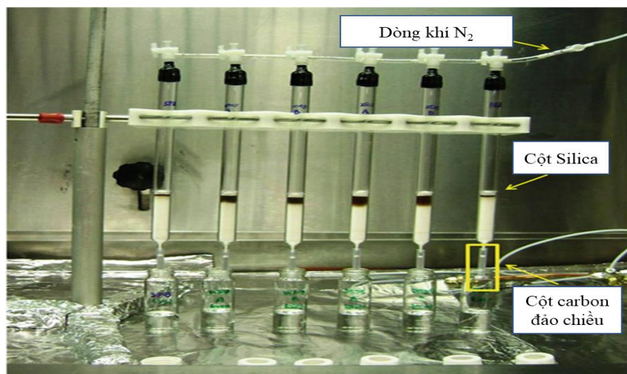
Hình 1.5 Hệ thống chuẩn bị mẫu dùng một lần của Cape Technologies
