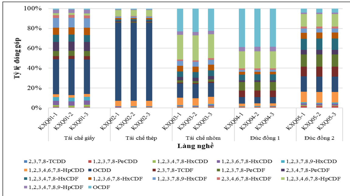
Hình 3.28 Cấu hình các đồng loại PCDD/Fs đóng góp vào tổng hàm lượng trong các mẫu không khí xung quanh
