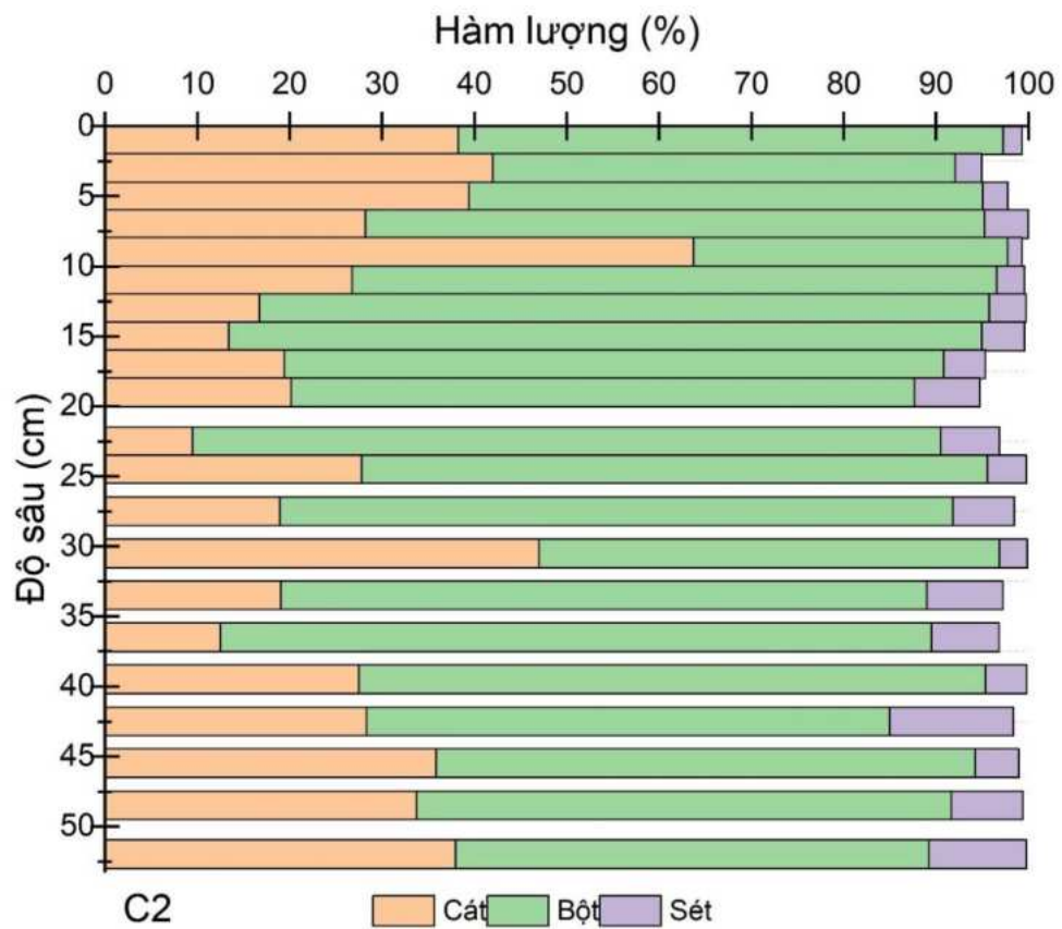
Hình 3.3. Sơ đồ phân bố hàm lượng các cấp hạt theo độ sâu cột C2
