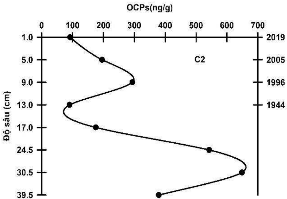
Hình 3.18.b. Phân bố các nhóm BHCs, DDTs, Drins và tổng OCPs trong cột C2
