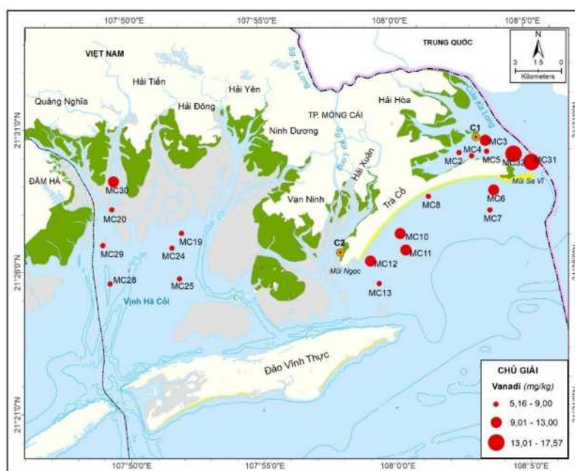
Hình 3.15. Phân bố molipden (a) và vanadi (b) trong trầm tích tầng mặt
