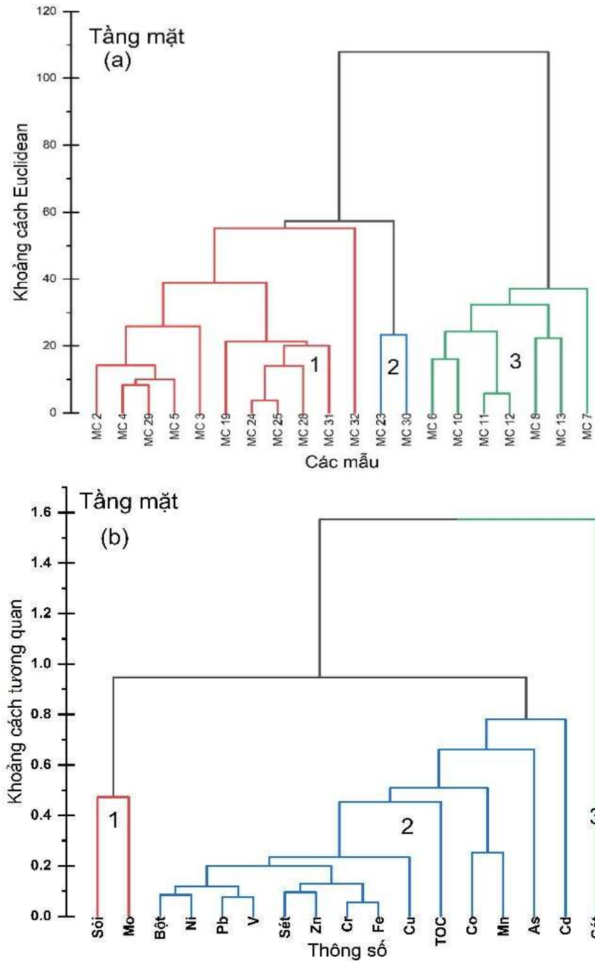
Hình 4.1. Các nhóm KLN và đặc điểm trong trầm tích tầng mặt (a - nhóm trầm tích, b - nhóm thông số trầm tích)
