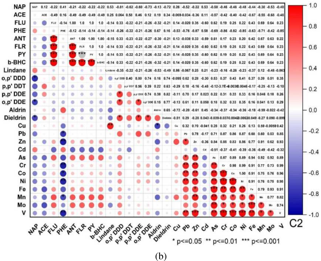
Hình 3.22. Tương quan giữa kim loại nặng, PAHs và OCPs trong cột trầm tích
