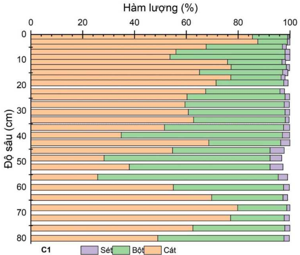
Hình 3.2. Sơ đồ phân bố hàm lượng các cấp hạt theo độ sâu cột C1
