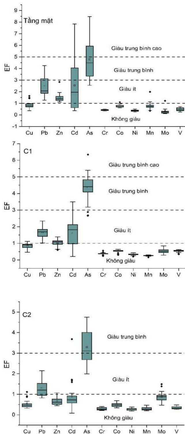
Hình 4.8. Chỉ số giàu kim loại nặng
