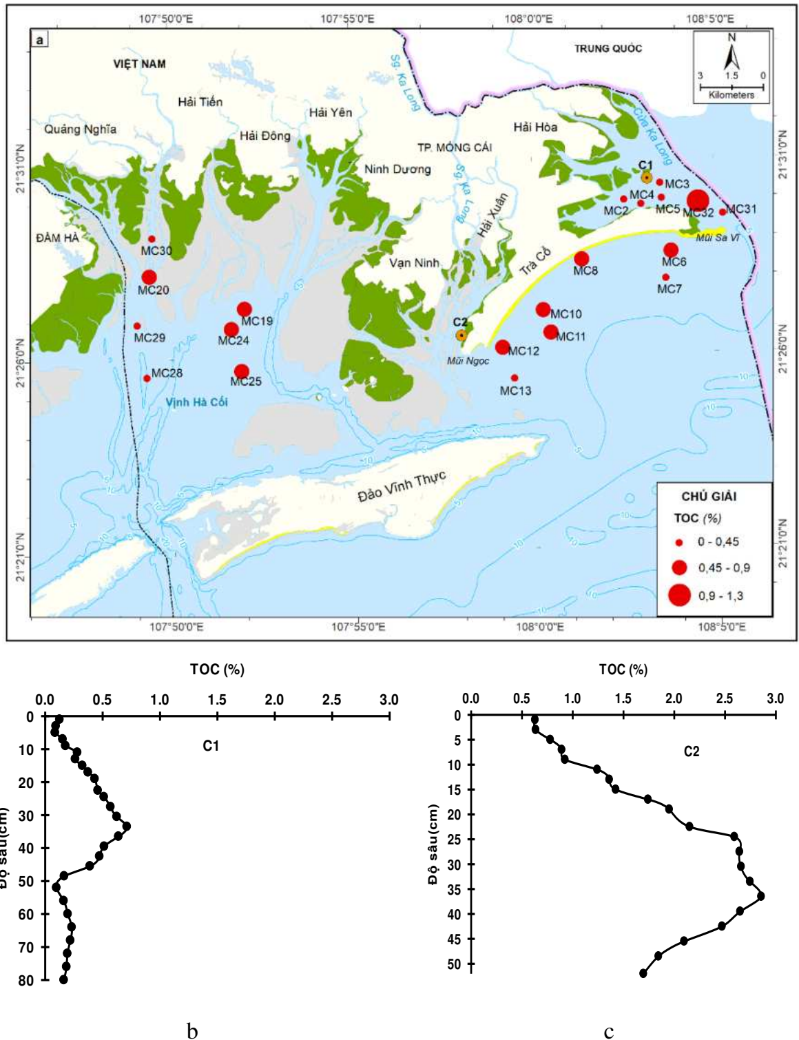
Hình 3.4. Phân bố TOC trong trầm tích vùng biển ven bờ Móng Cái (a- Trầm tích tầng mặt; b – Cột C1; c – Cột C2)
