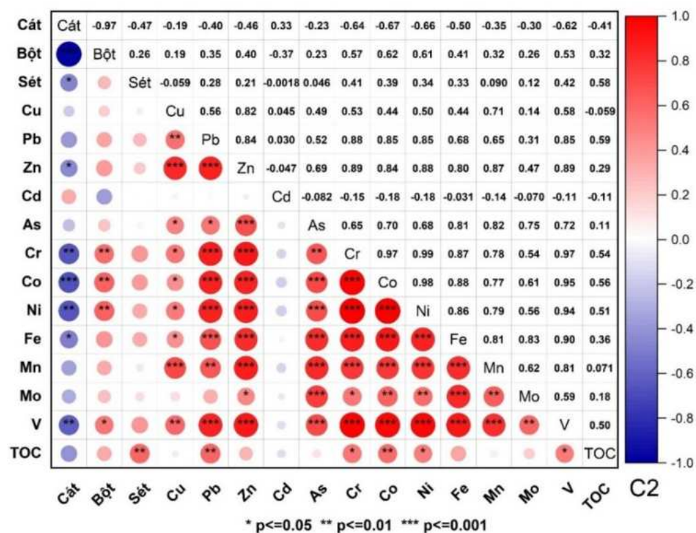
Hình 3.20. Tương quan giữa KLN, thành phần cấp hạt, các thông số trong các cột trầm tích
