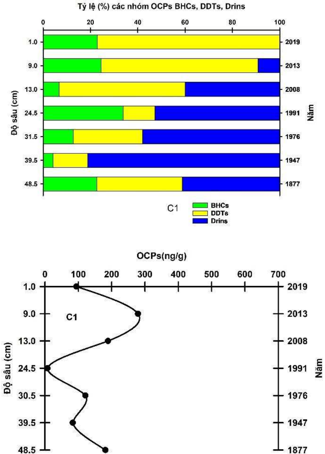
Hình 3.18.a. Phân bố các nhóm BHCs, DDTs, Drins và tổng OCPs trong cột C1
