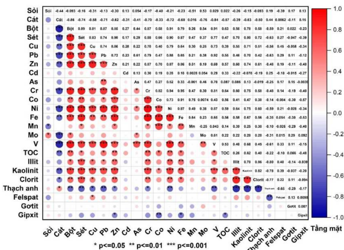
Hình 3.19. Tương quan giữa các thông số cấp hạt, khoáng vật và KLN trong trầm tích tầng mặt
