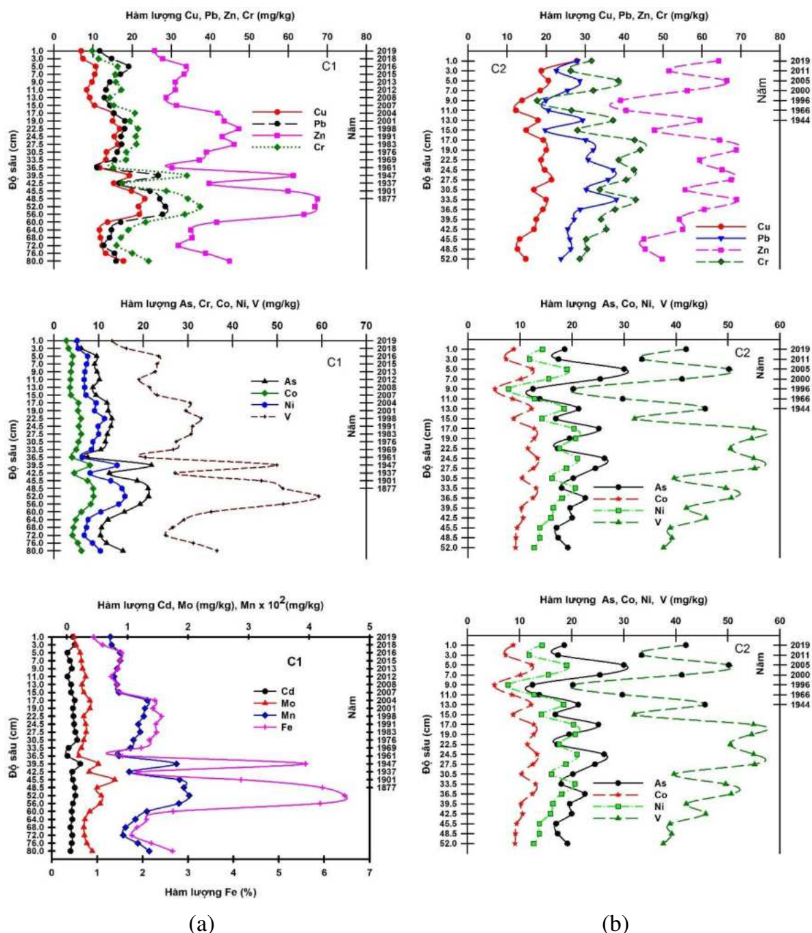
Hình 3.16. Phân bố kim loại nặng trong 2 cột trầm tích
