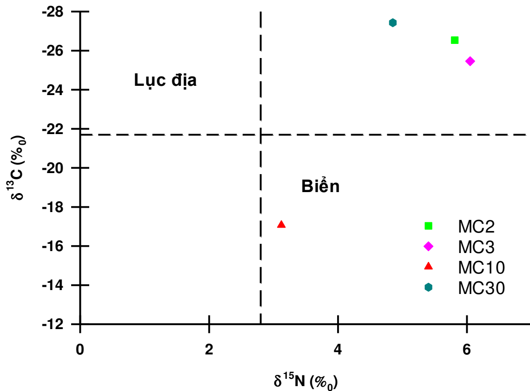
Hình 4.4. Đồ thị biplot của \delta^{13}\text{C} và \delta^{15}\text{N} trong trầm tích tầng mặt
