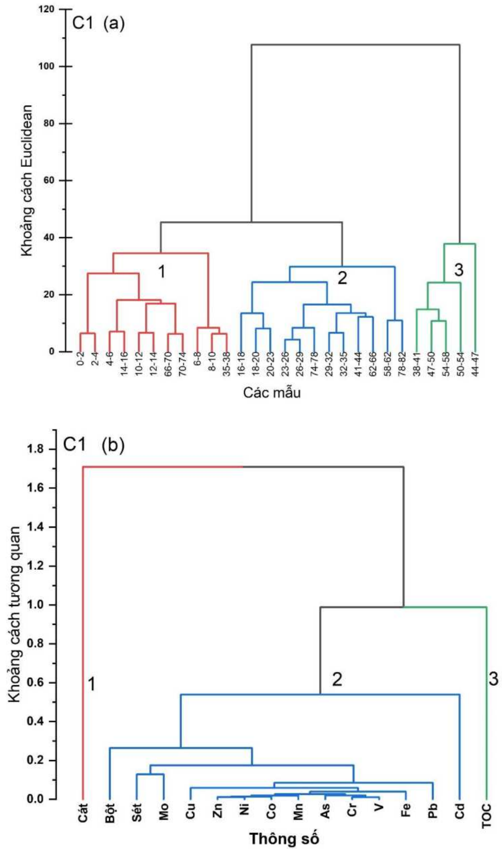
Hình 4.2. Các nhóm KLN và đặc điểm trong cột C1 (a - nhóm trầm tích, b - nhóm thông số trầm tích)
