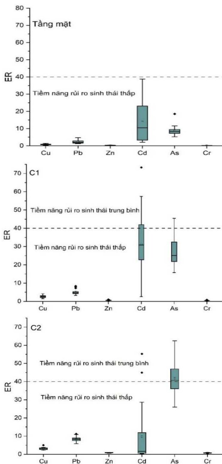
Hình 4.10. Chỉ số tiềm năng rủi ro sinh thái
