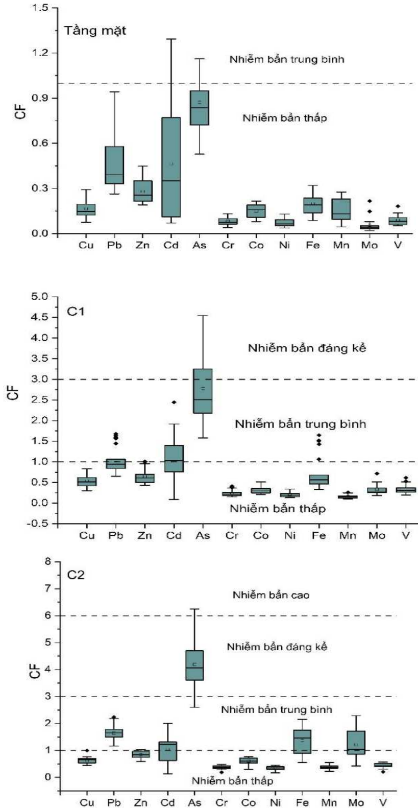
Hình 4.9. Chỉ số nhiễm bẩn kim loại
