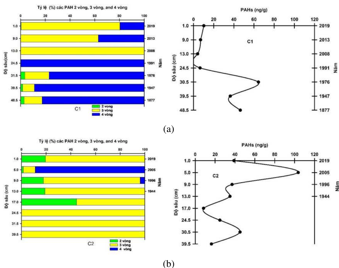
Hình 3.17. Sự phân bố PAHs trong cột trầm tích
