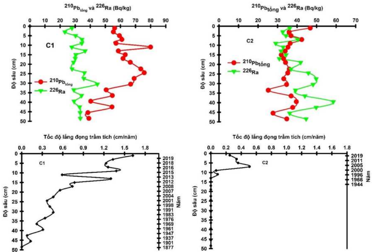
Hình 3.9. Phân bố hoạt độ phóng xạ ^{210}\text{Pb} tổng và ^{226}\text{Ra} , thời gian và tốc độ lắng đọng trầm tích
