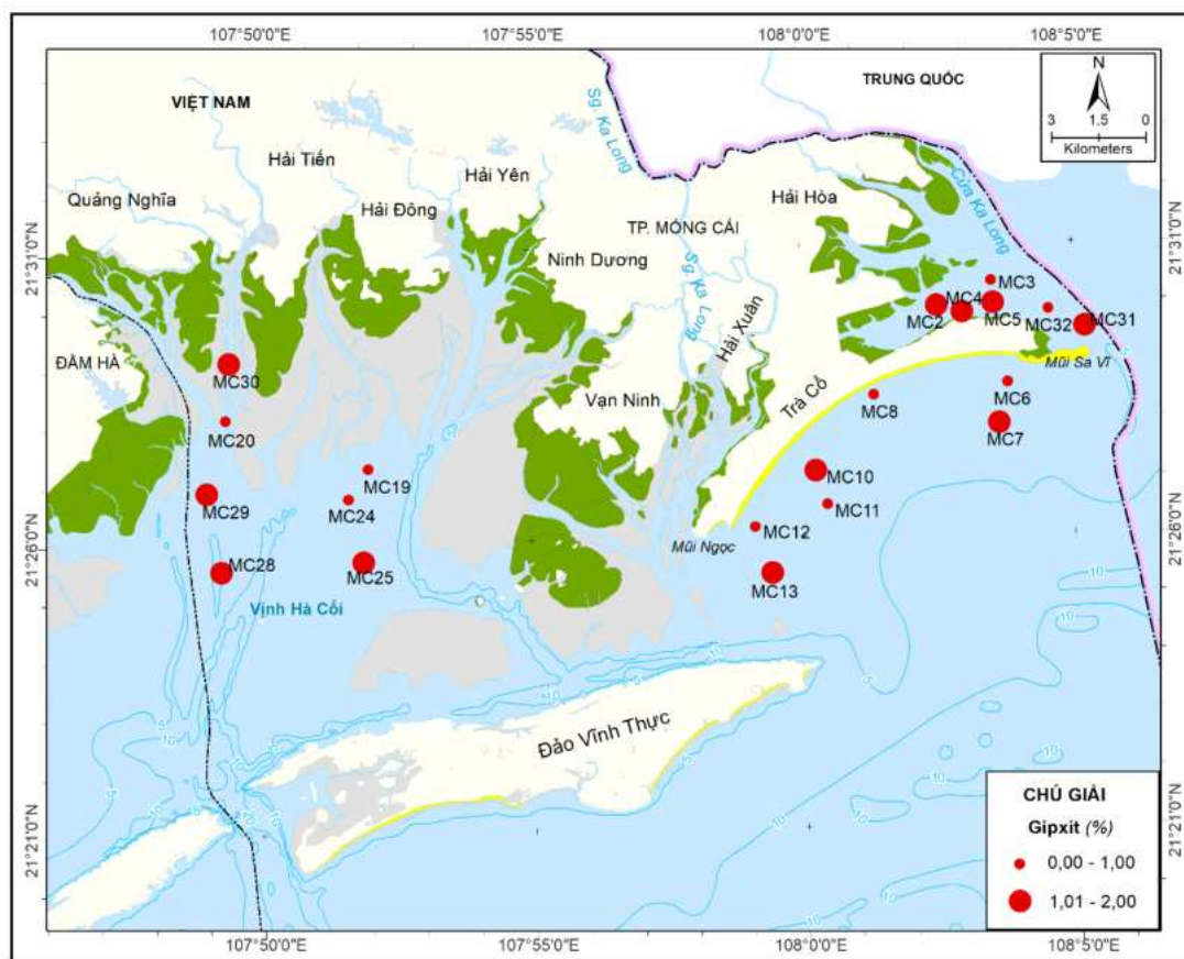
Hình 3.8. Phân bố gipxit trong trầm tích tầng mặt
