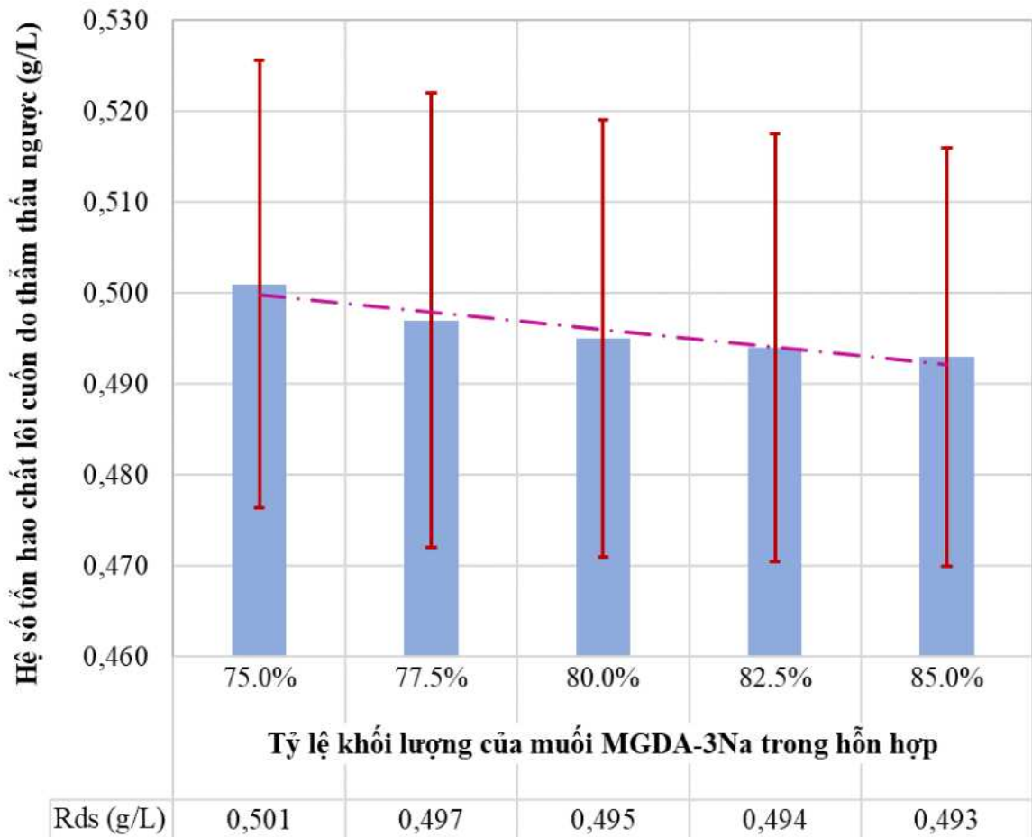
Hình 3.18. Đặc trưng tổn hao chất lồi cuốn do thẩm thấu ngược của dung dịch lồi cuốn MGDA 25% tại những tỷ lệ muối MGDA-3Na khác nhau
