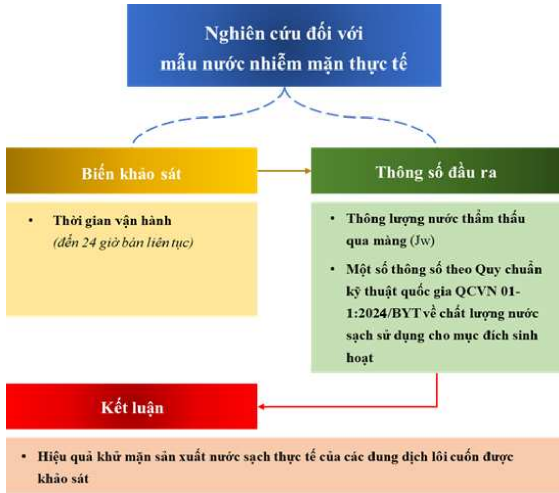
Hình 2.9. Các thông số biến khảo sát, thông số đầu ra, và nội dung kết luận của hệ thí nghiệm nghiên cứu hiệu quả vận hành trên mẫu nước nhiễm mặn thực tế của các dung dịch lõi cuộn
