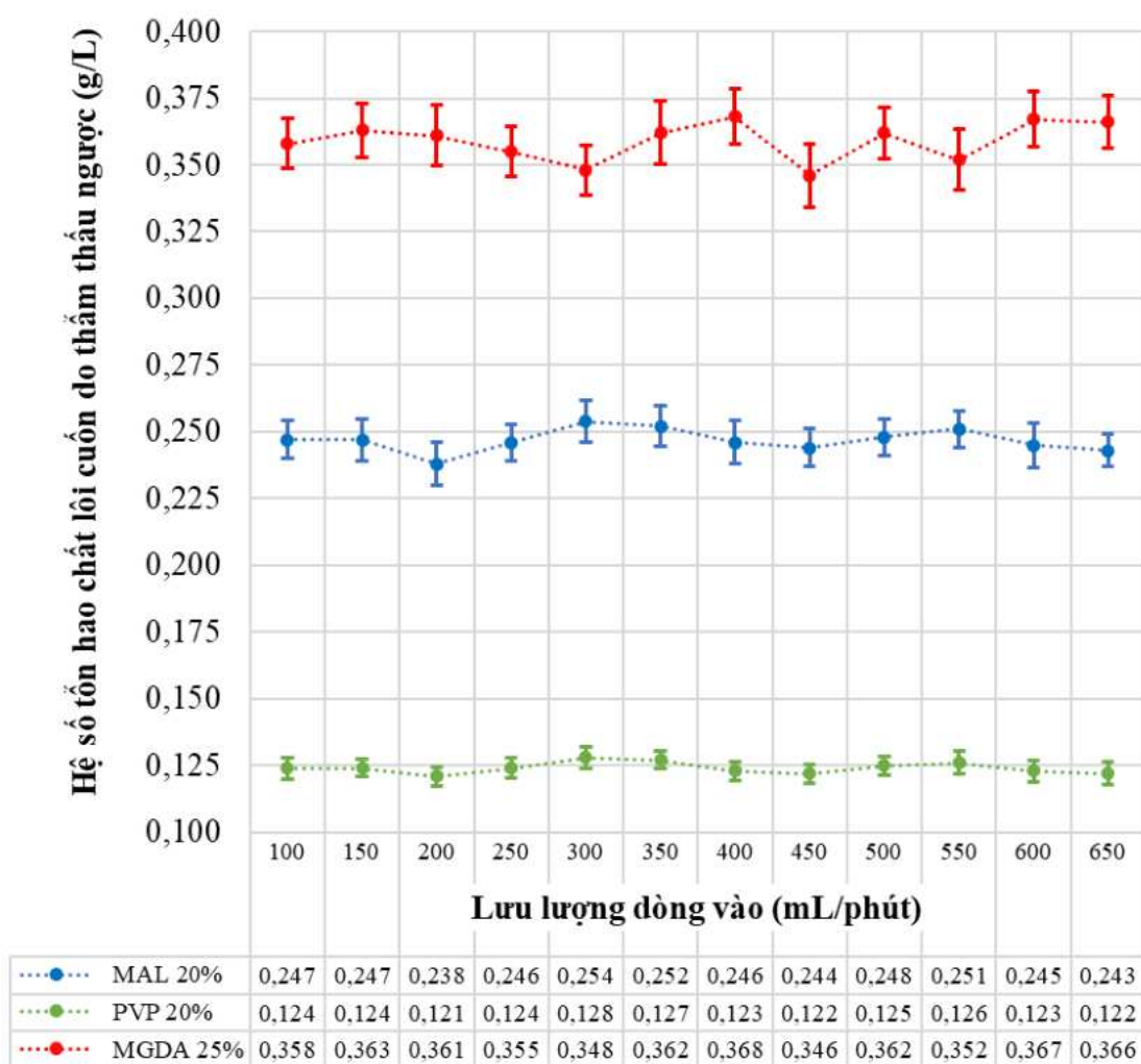
Hình 3.30. Ảnh hưởng của lưu lượng dòng vào lên hệ số tổn hao R_{ds} của dung dịch lõi cuộn MAL 20%, dung dịch lõi cuộn PVP 20%, và dung dịch lõi cuộn MGDA 25%
