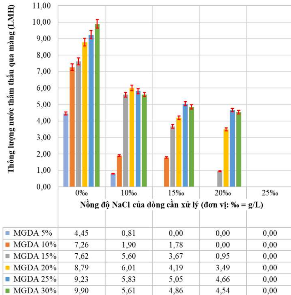
Hình 3.10. Đặc trưng thông lượng J_w của dung dịch lồi cuốn MGDA tại những nồng độ dung dịch lồi cuốn và độ mặn dòng cần xử lý khác nhau
