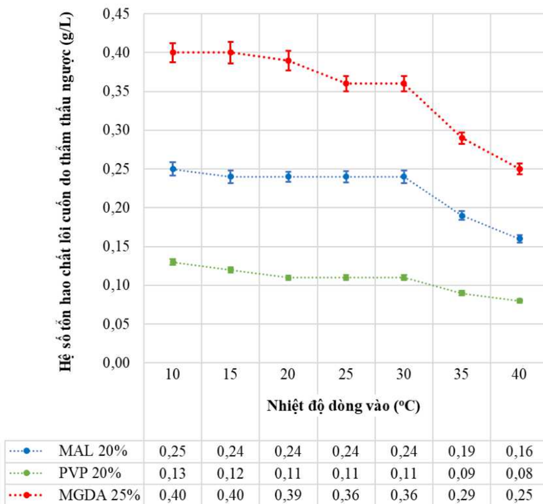
Hình 3.27. Ảnh hưởng của nhiệt độ vận hành lên hệ số tổn hao Rds của dung dịch lõi cuộn MAL 20%, dung dịch lõi cuộn PVP 20%, và dung dịch lõi cuộn MGDA 25%
