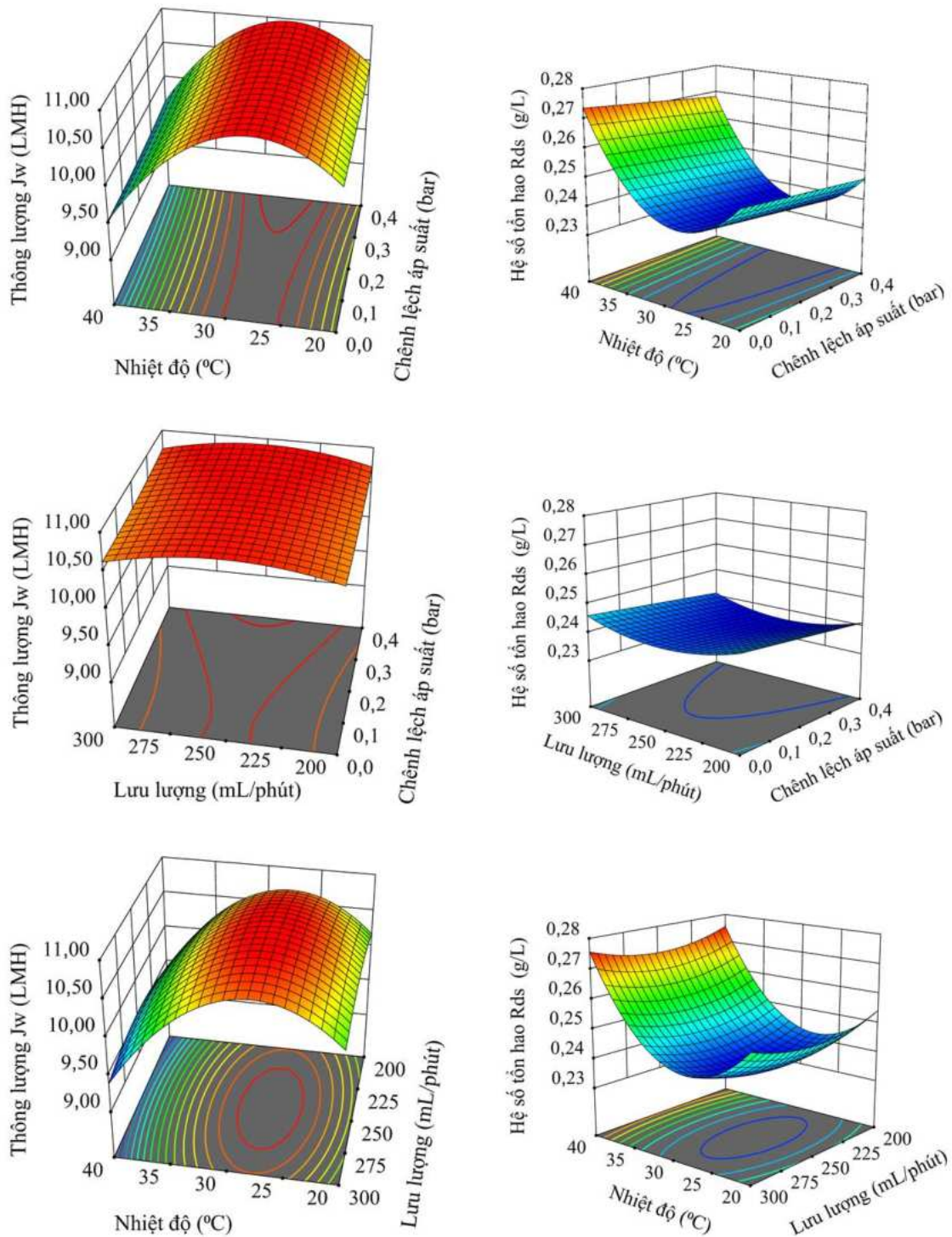
Hình 3.31. Kết quả phân tích bề mặt đáp ứng nhằm đánh giá ảnh hưởng của các thông số điều kiện vận hành lên thông lượng J_w (trái) và hệ số tổn hao R_{ds} (phải) khi sử dụng dung dịch lõi cuốn MAL 20%
