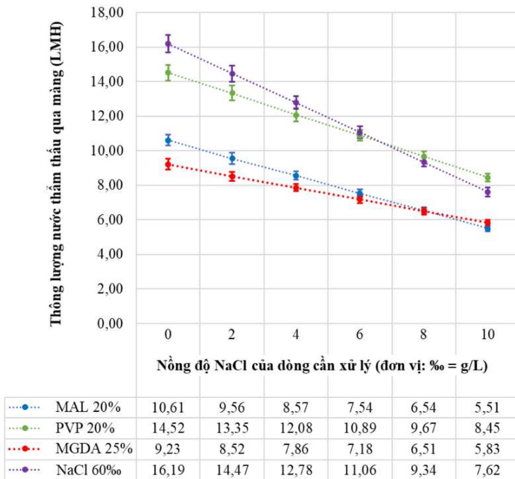
Hình 3.19. Đặc trưng thông lượng J_w của các dung dịch lồi cuốn tại những độ mặn dòng cần xử lý khác nhau
