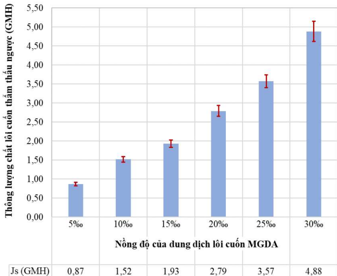
Hình 3.11. Thông lượng J_s của dung dịch lõi cuộn MGDA tại các nồng độ dung dịch lõi cuộn khác nhau
