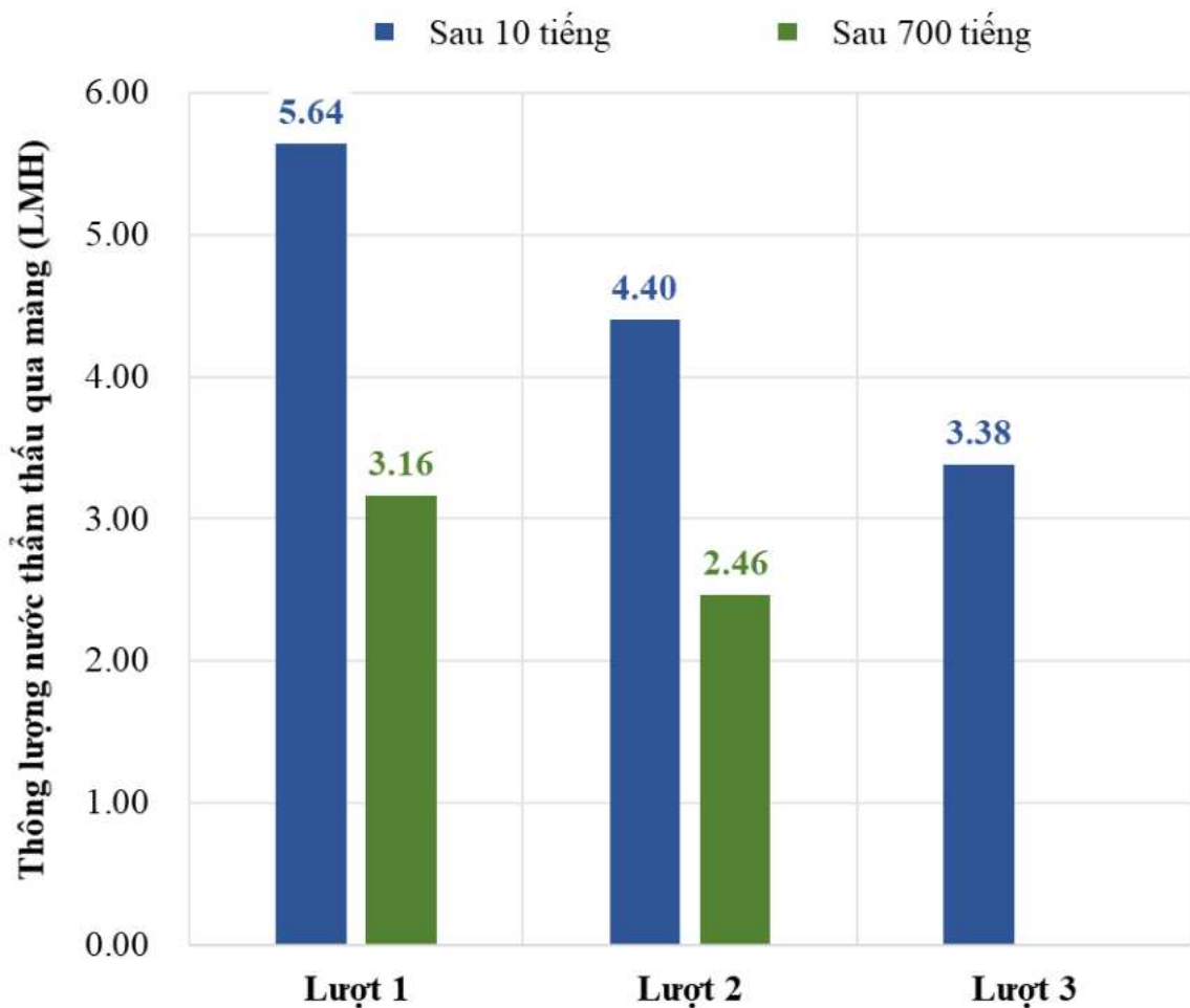
Hình 3.38. Ảnh hưởng của thời gian vận hành và phương pháp làm sạch rửa xuôi lên thông lượng J_w (dung dịch lõi cuộn MAL 20%)
