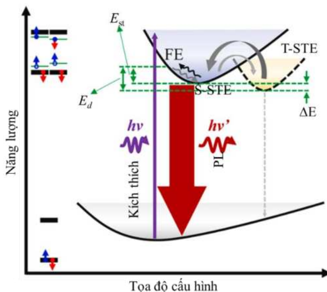
Hình 4.18. Sơ đồ tọa độ cấu hình FE: exciton tự do; S-STE: exciton tự bẫy spin-singlet; T-STE: exciton tự bẫy spin-triplet; E_{st} : năng lượng bẫy; E_d : năng lượng giải phóng khỏi bẫy; \Delta E : sự phân tách năng lượng giữa T-STE và S-STE; Hình nhỏ (góc dưới trái) thể hiện các mức năng lượng và các trạng thái điện tử cho trạng thái cơ bản; hình nhỏ (góc trên trái) thể hiện các mức năng lượng và các trạng thái điện tử cho các trạng thái kích thích (singlet spin và triplet spin).
