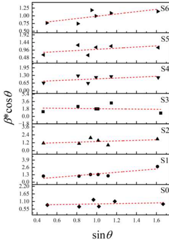
Hình 4.6. Đồ thị biểu diễn mối liên hệ giữa \beta^*\cos\theta và \sin\theta của các mẫu S0 đến S6
