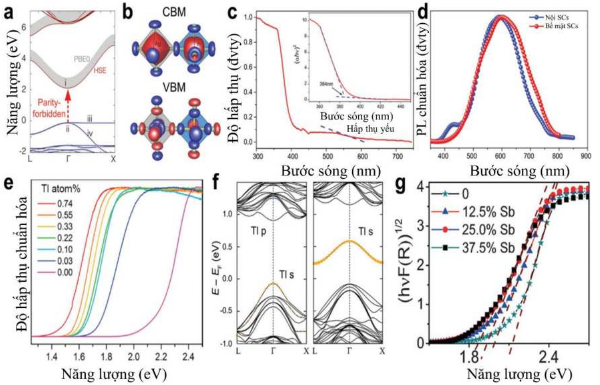
Hình 1.18. (a) Cấu trúc vùng năng lượng, (b) Minh hoạ các hàm sóng điện tử tại đáy CB và đỉnh VB, (c) Phổ hấp thụ của NC \text{Cs}_2\text{AgInCl}_6 (Hình nhỏ bên trong: Đồ thị Tauc xác định năng lượng vùng cấm là 3,2 eV), (d-e) Phổ PL và phổ hấp thụ của NC \text{Cs}_2\text{AgInCl}_6 , (f) Cấu trúc vùng năng lượng của \text{Cs}_2(\text{Ag}_{1-a}\text{Bi}_{1-b})\text{Tl}_x\text{Br}_6 ( x = 0,06 ), (g) Đồ thị Tauc của \text{Cs}_2\text{Ag}(\text{Bi}_{1-x}\text{Sb}_x)\text{Br}_6 [54,78–80].
