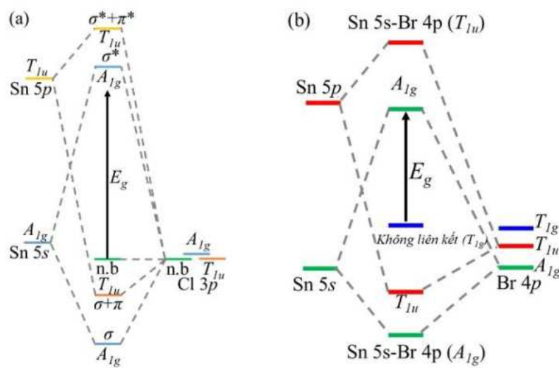
Hình 3.16. Sự tương tác giữa các quỹ đạo trong tinh thể \text{Cs}_2\text{SnX}_6 : (a) \text{Cs}_2\text{SnCl}_6 ; (b) \text{Cs}_2\text{SnBr}_6 .
