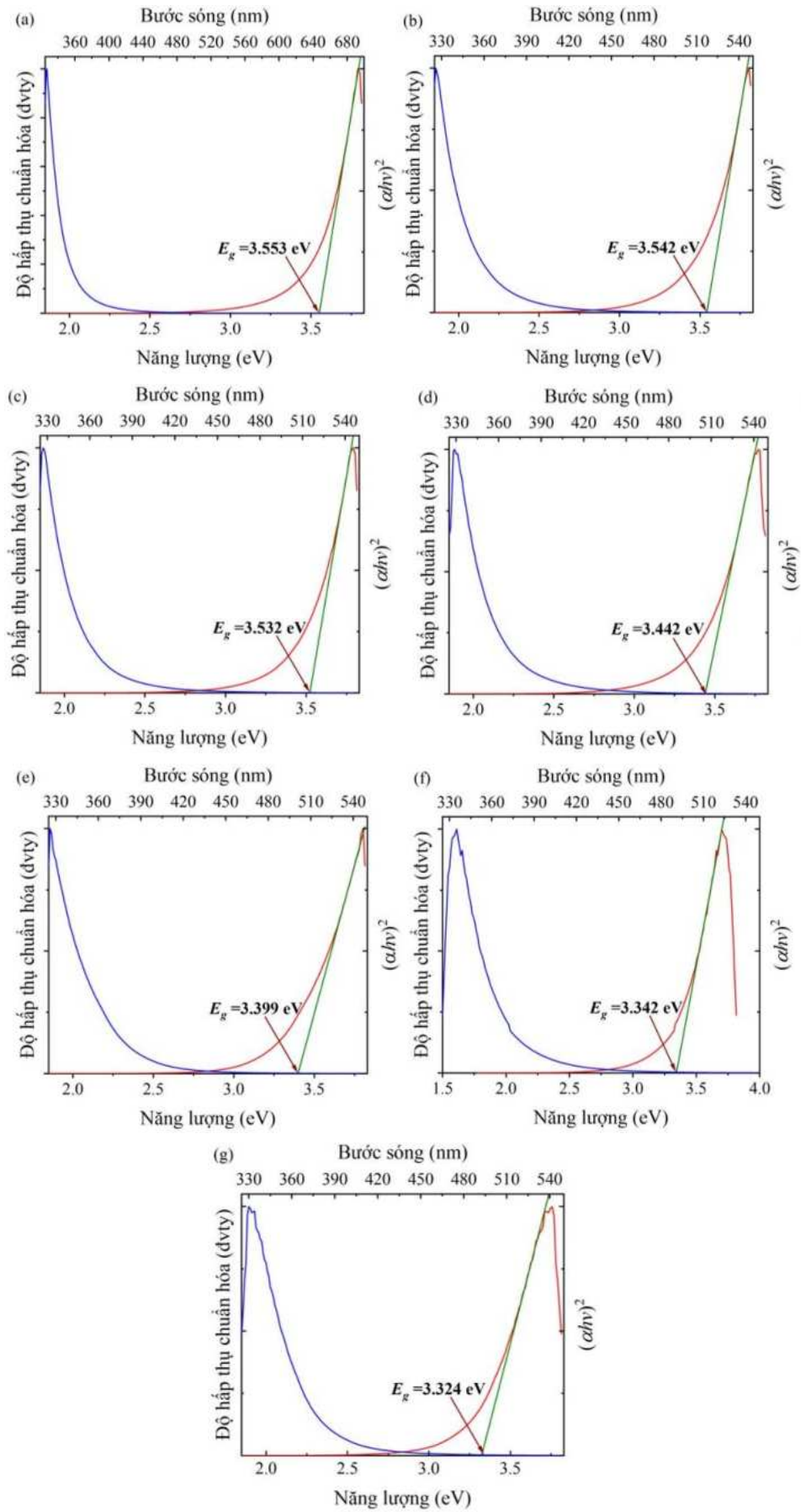
Hình 4.13. Phổ hấp thụ và Đồ thị Tauc của các mẫu (a) S0, (b) S1, (c) S2, (d) S3, (e) S4, (f) S5, (g) S6.
