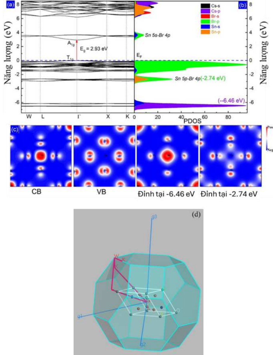
Hình 3.14. (a) Cấu trúc vùng năng lượng, (b) mật độ trạng thái của mẫu \text{Cs}_2\text{SnBr}_6 , (c) trạng thái lai hóa giữa quỹ đạo Sn 5s và quỹ đạo Br 4p đặc trưng đối xứng A_{1g} , và mật độ điện tích một phần của quỹ đạo CB và VB. Màu đỏ tượng trưng cho nồng độ điện tích cao hơn, trong khi màu xanh tượng trưng cho mật độ thấp hơn, (d) Vùng Brillouin bậc nhất của mạng FCC ( Fm-3m ) với các điểm đối xứng cao \Gamma , X, W, K, L.
