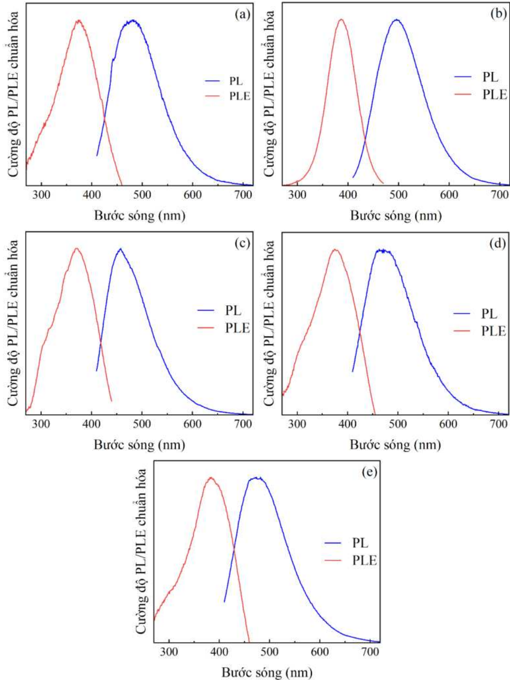
Hình 2.5. Phổ PL của các mẫu \text{Cs}_2\text{SnBr}_6 chế tạo ở các nhiệt độ khác nhau:
