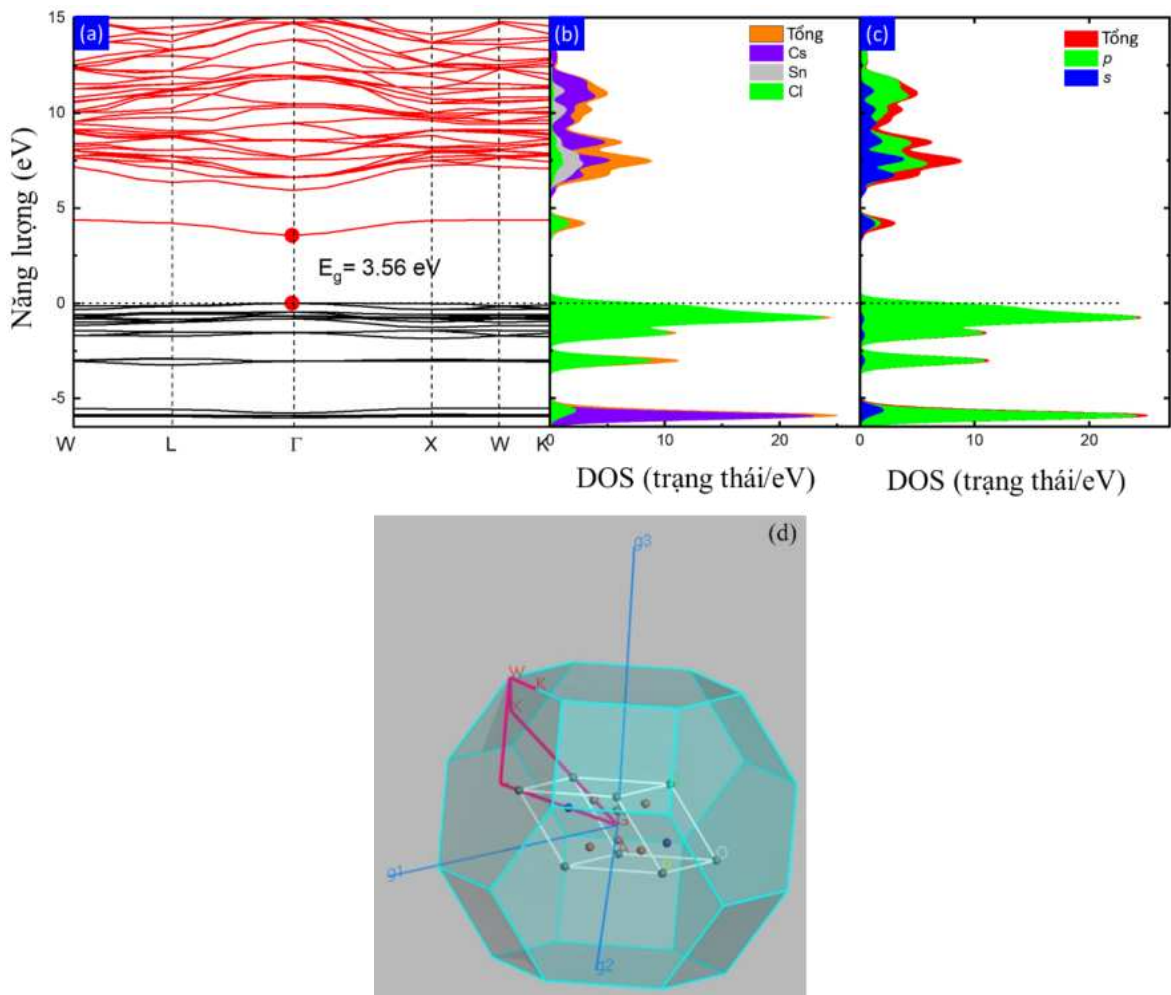
Hình 3.13. (a) Cấu trúc vùng năng lượng, (b,c) mật độ các trạng thái tổng và riêng phần của vật liệu \text{Cs}_2\text{SnCl}_6 , (d) Vùng Brillouin bậc nhất của mạng FCC (Fm-3m) với các điểm đối xứng cao \Gamma , X, W, K, L.
