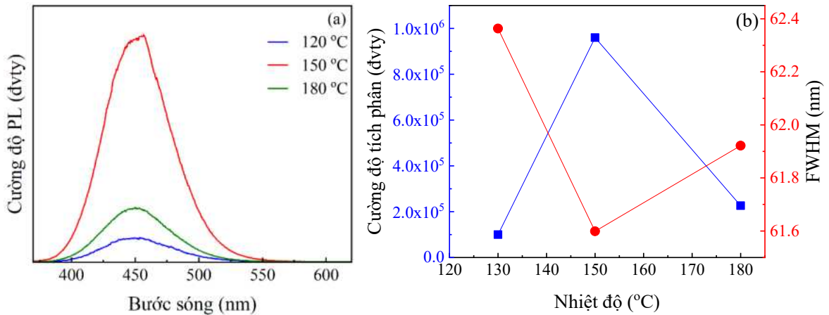
Hình 2.3. (a) Phổ PL và (b) cường độ tích phân và FWHM của các mẫu \text{Cs}_2\text{SnCl}_6 chế tạo ở các nhiệt độ khác nhau.
