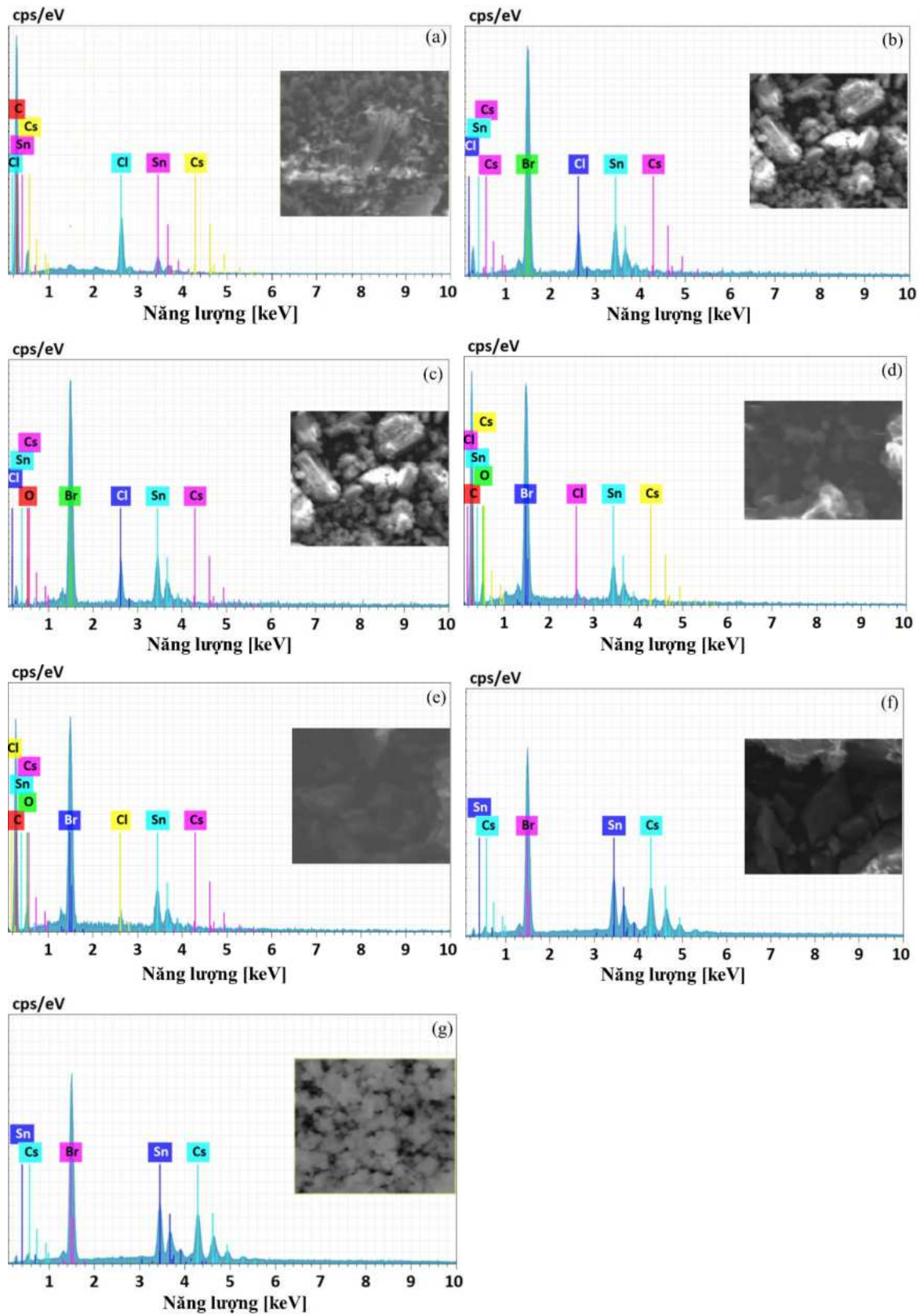
Hình 4.9. Ảnh EDS của các mẫu \text{Cs}_2\text{SnCl}_{6-x}\text{Br}_x ( x = 0, 1, 2, 3, 4, 5, 6 ).
