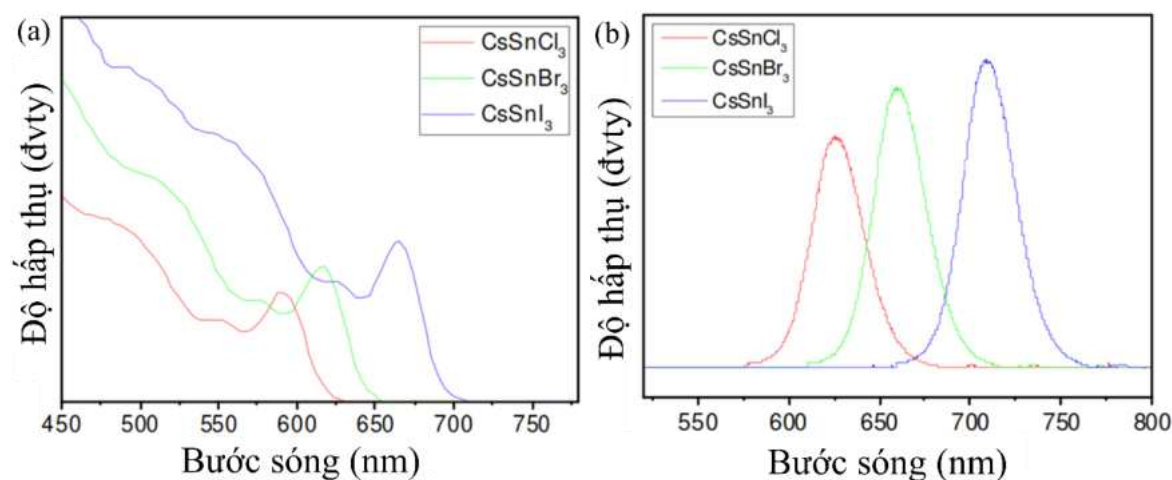
Hình 1.20. (a) Phổ hấp thụ và (b) phổ huỳnh quang của các tinh thể \text{CsSnX}_3 ( \text{X} = \text{Cl}, \text{Br} và \text{I} ) [93].
