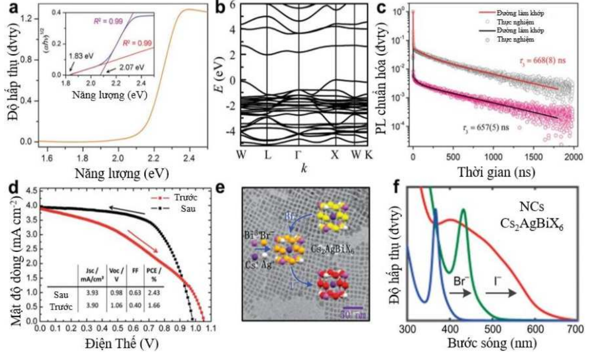
Hình 1.17. (a) Phổ hấp thụ của bột \text{Cs}_2\text{AgBiBr}_6 (Hình nhỏ bên trong: đồ thị Tauc xác định năng lượng vùng cấm), (b) Cấu trúc vùng năng lượng của \text{Cs}_2\text{AgBiBr}_6 , (c) PL phân giải theo thời gian tại nhiệt độ phòng của mẫu bột và đơn tinh thể \text{Cs}_2\text{AgBiBr}_6 , (d) Đường cong J–V của pin mặt trời trên cơ sở NC \text{Cs}_2\text{AgBiBr}_6 , (e) Ảnh TEM của NC \text{Cs}_2\text{AgBiBr}_6 , (f) Phổ hấp thụ của NC \text{Cs}_2\text{AgBiX}_6 [54].
