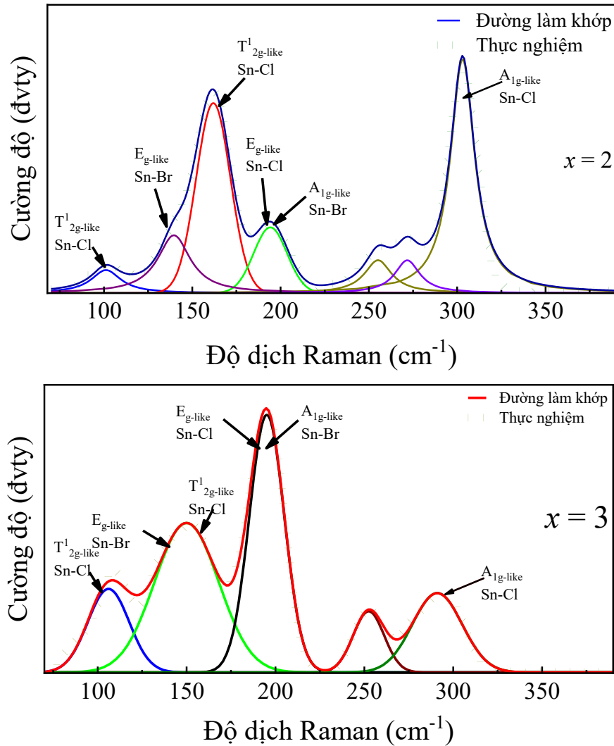
Hình 4.11. Đường làm khớp phổ Raman của mẫu S2 và S3
