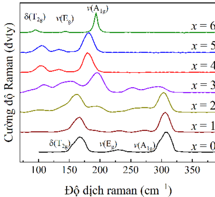
Hình 4.10. Phổ Raman của các mẫu Cs_2SnCl_{6-x}Br_x ( x = 0, 1, 2, 3, 4, 5, 6 ).
