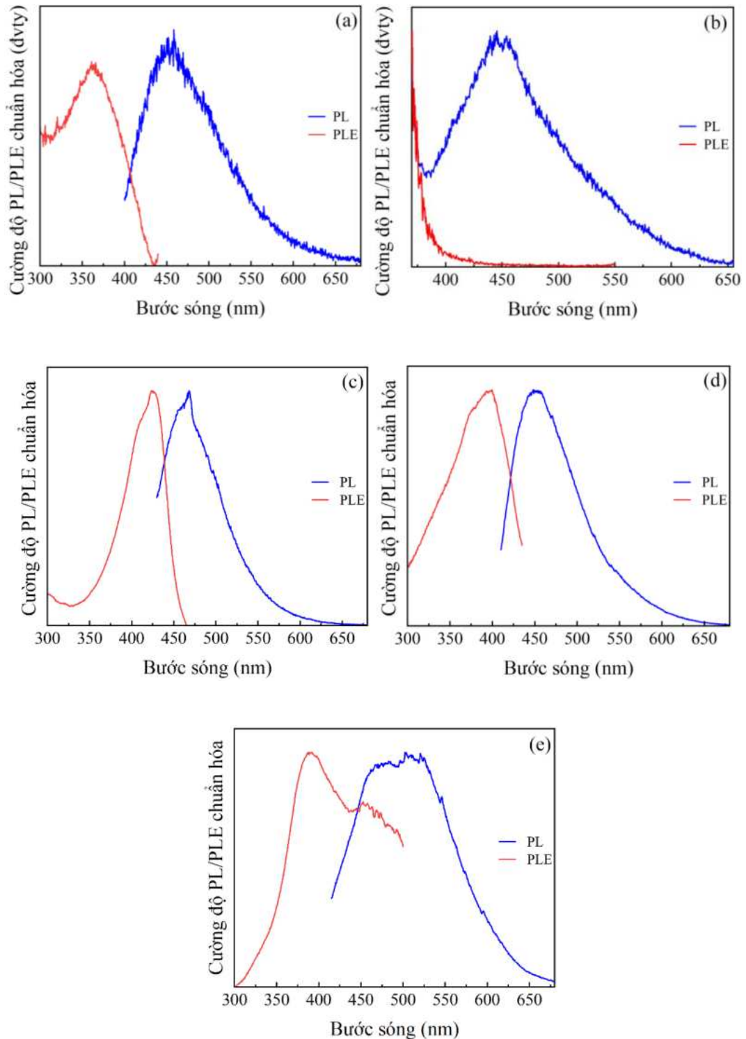
Hình 2.8. Phổ PL của các mẫu \text{Cs}_2\text{SnBr}_6 tái phân tán với các dung môi khác nhau (a) methanol, (b) ethanol, (c) DMF, (d) axeton, (e) toluen.
