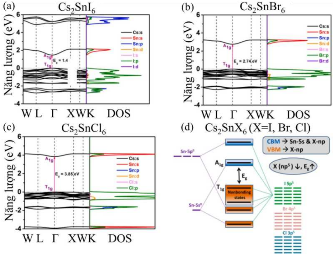
Hình 1.24. (a-c) Cấu trúc vùng năng lượng của các NC \text{Cs}_2\text{SnX}_6 ( \text{X} = \text{I}, \text{Br}, \text{Cl} ) và (d) Sơ đồ quỹ đạo của \text{Cs}_2\text{SnX}_6 ( \text{X} = \text{I}, \text{Br}, \text{Cl} ) [100].
