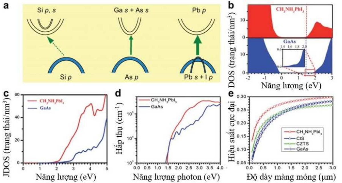
Hình 1.7. (a) Sơ đồ cấu trúc vùng năng lượng của các vật liệu Si (bên trái), GaAs (giữa) và \text{MAPbI}_3 (bên phải) [48], (b) Mật độ trạng thái của tinh thể \text{MAPbI}_3 và GaAs, (c) Mật độ trạng thái kết hợp của mẫu \text{MAPbI}_3 và GaAs, (d) Hấp thụ quang của của \text{MAPbI}_3 và GaAs, (e) Hiệu suất cực đại của các vật liệu \text{MAPbI}_3 , CIS, CZTS và GaAs theo độ dày màng [49].
