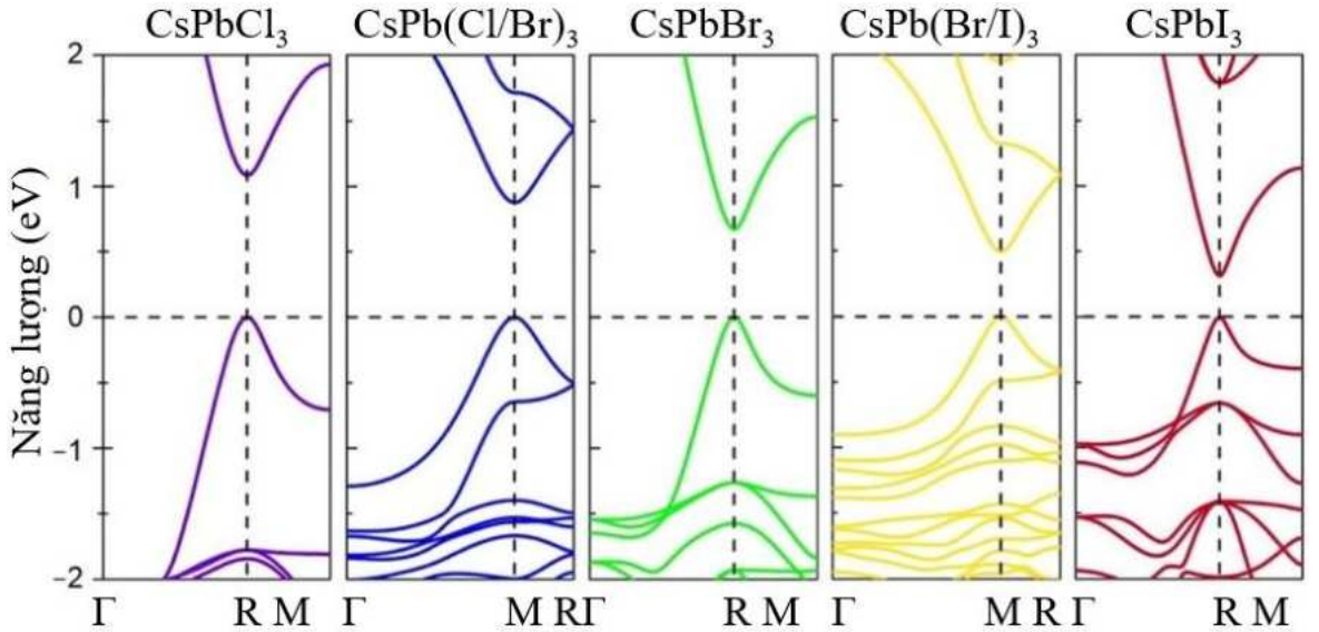
Hình 1.8. Cấu trúc vùng năng lượng của perovskite CsPbX 3 (X = Cl, Br, I) [31].
