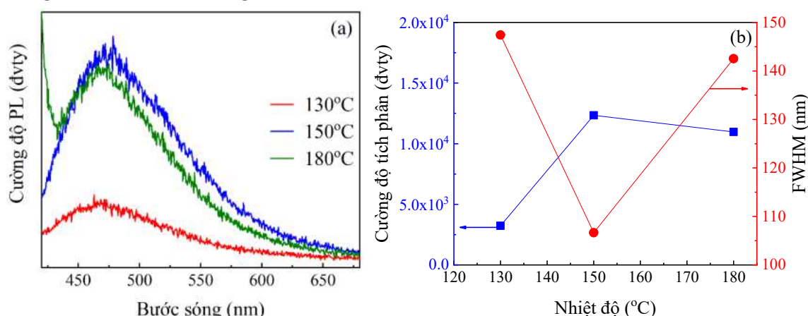
Hình 2.4. (a) Phổ PL và (b) cường độ tích phân và FWHM của các mẫu \text{Cs}_2\text{SnBr}_6 chế tạo ở các nhiệt độ khác nhau.
