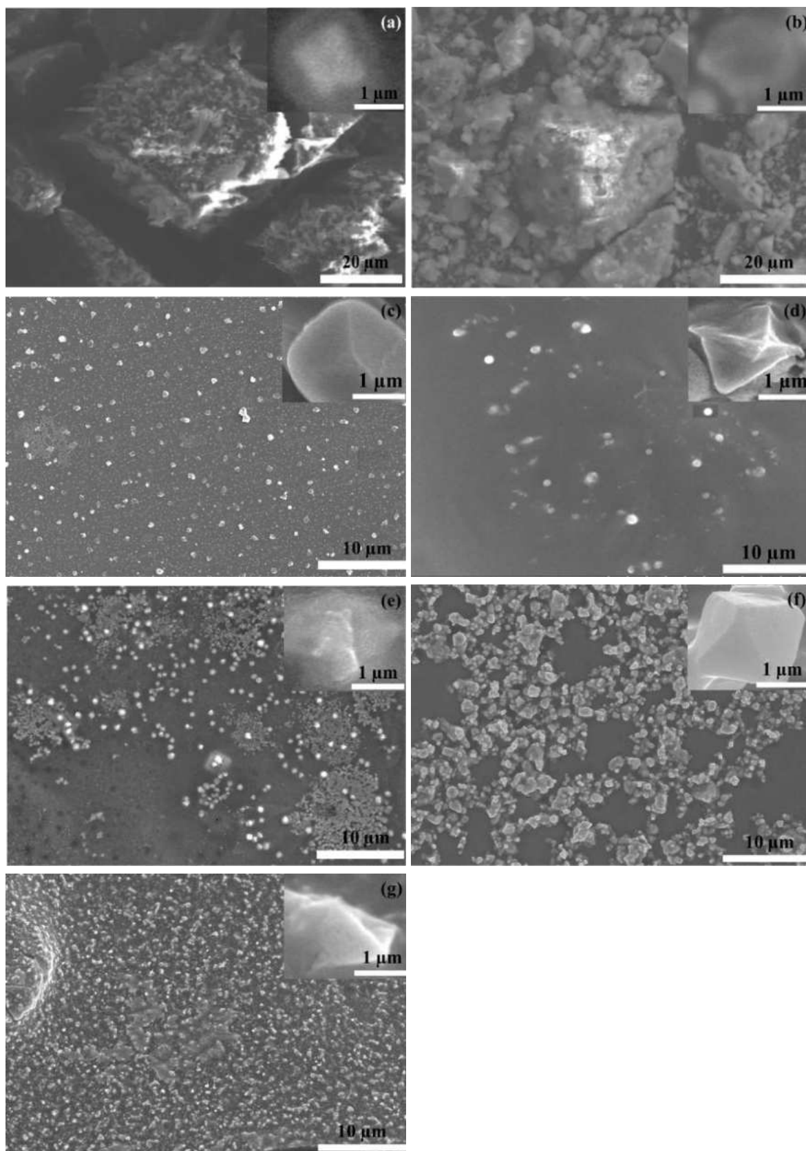
Hình 4.8. Ảnh SEM của các tinh thể \text{Cs}_2\text{SnCl}_{6-x}\text{Br}_x ( x = 0, 1, 2, 3, 4, 5, 6 ).
