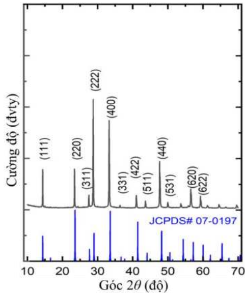
Hình 3.2. Giảm nhiễu xạ tia X của các mẫu Cs_2SnCl_6 .
