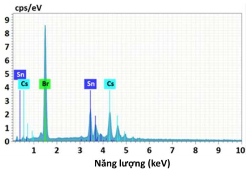
Hình 3.7. Phổ EDS của mẫu tinh thể \text{Cs}_2\text{SnBr}_6
