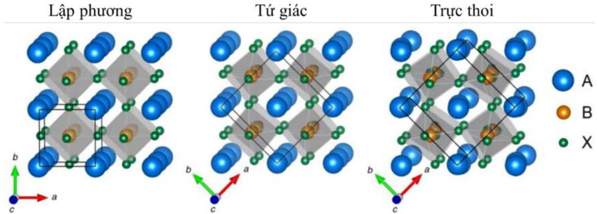
Hình 1.3. Minh họa các cấu trúc perovskite lập phương, tứ giác và trực thoi [30].
