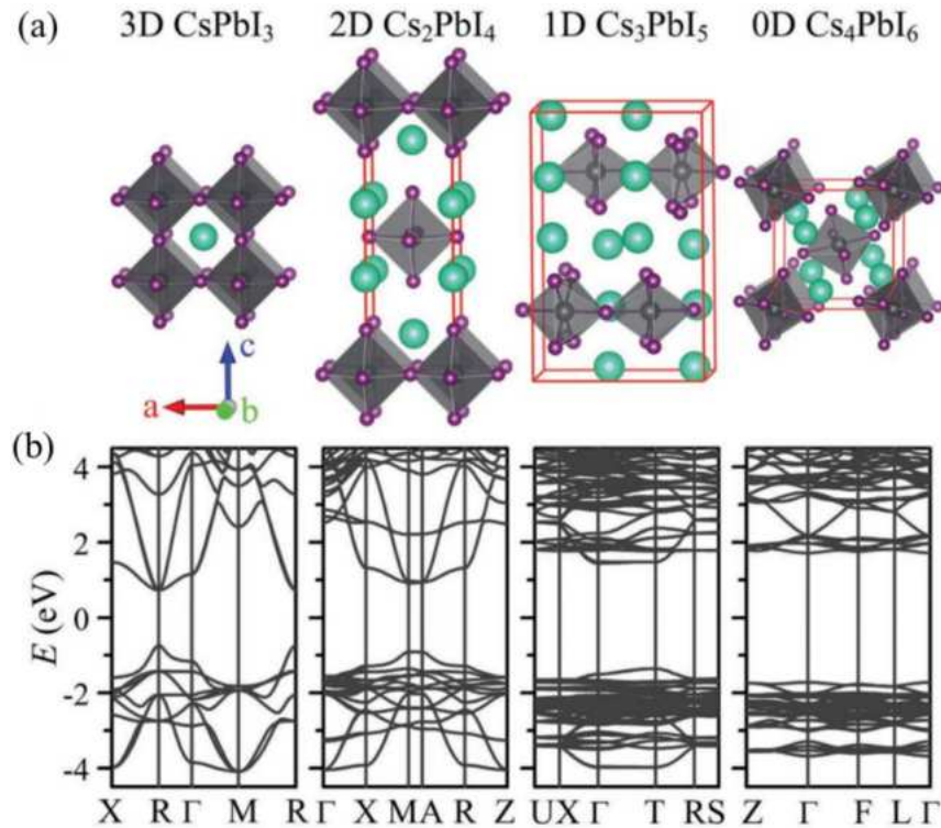
Hình 1.9. (a) Cấu trúc tinh thể, (b) cấu trúc vùng năng lượng của các tinh thể CsPbI 3 , Cs 2 PbI 4 , Cs 3 PbI 5 và Cs 4 PbI 6 [56].
