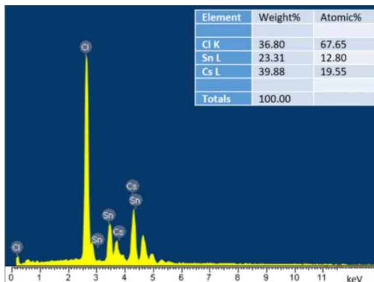
Hình 3.5. Phổ EDX của mẫu tinh thể \text{Cs}_2\text{SnCl}_6 .
