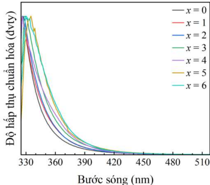
Hình 4.12. Phổ hấp thụ của hệ mẫu \text{Cs}_2\text{SnCl}_{6-x}\text{Br}_x ( x = 0, 1, 2, 3, 4, 5, 6 ).
