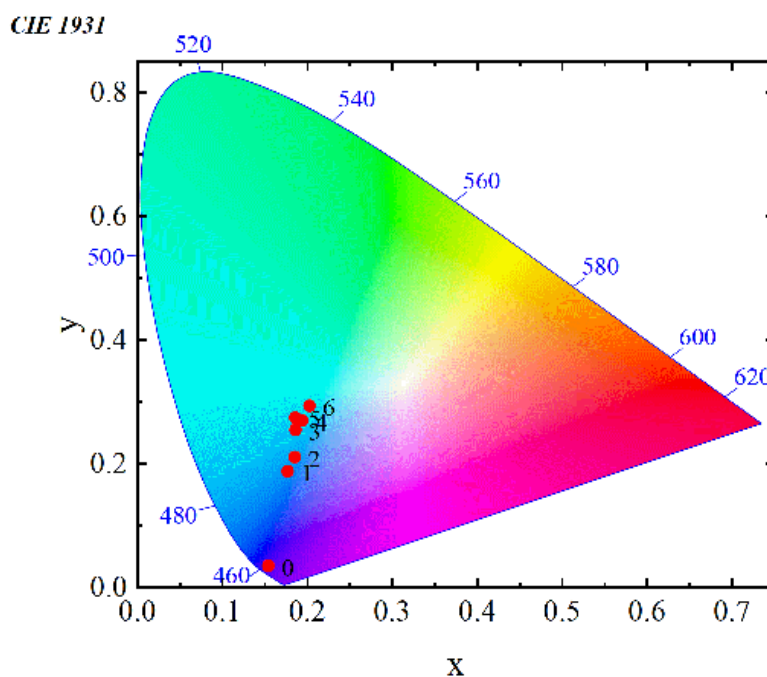
Hình 4.19. Biểu đồ tọa độ màu CIE của các hệ mẫu \text{Cs}_2\text{SnCl}_{6-x}\text{Br}_x ( x = 0, 1, 2, 3, 4, 5, 6 ).
