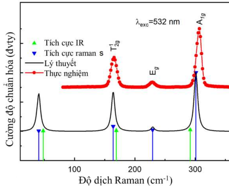
Hình 3.10. Phổ Raman tính toán và thực nghiệm của tinh thể \text{Cs}_2\text{SnCl}_6 .
