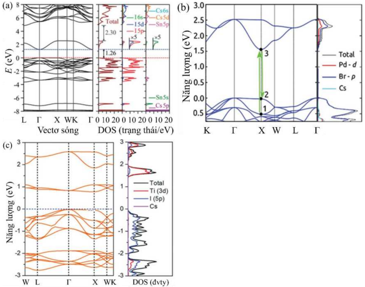
Hình 1.19. Cấu trúc vùng năng lượng và mật độ trạng thái của các tinh thể: (a) \text{Cs}_2\text{SnI}_6 ; (b) \text{Cs}_2\text{PdBr}_6 ; (c) \text{Cs}_2\text{TiBr}_6 [54].
