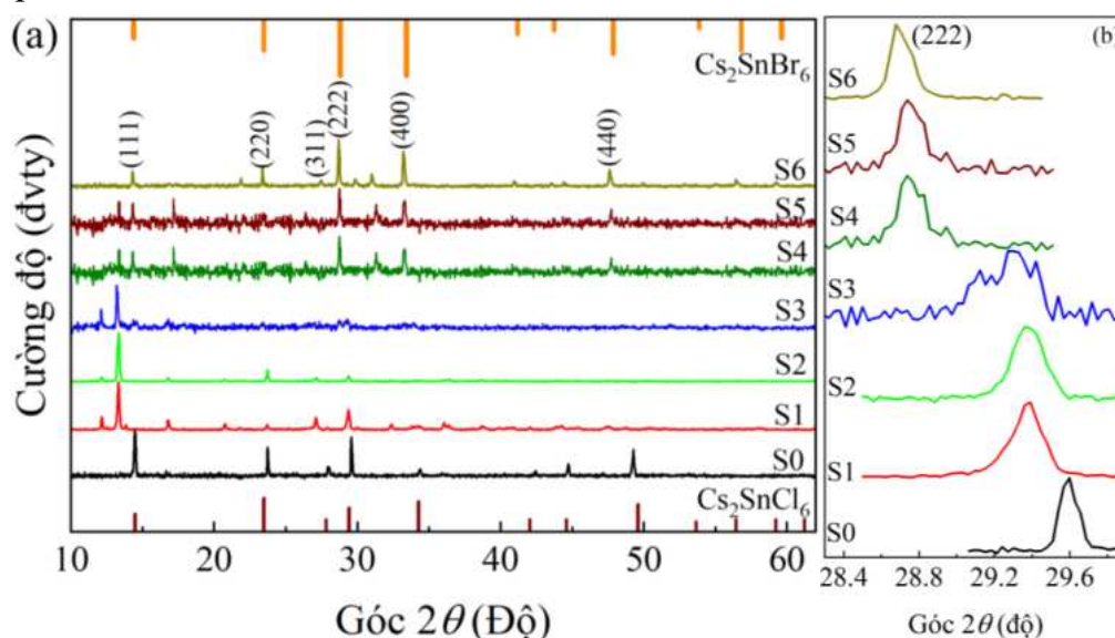
Hình 4.3. (a) Giải đồ nhiễu xạ XRD, (b) các đỉnh nhiễu xạ (222) của mẫu \text{Cs}_2\text{SnCl}_{6-x}\text{Br}_x ( x = 0, 1, 2, 3, 4, 5, 6 ).
