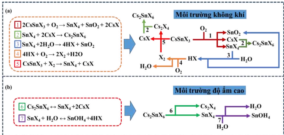
Hình 1.21. (a) Cơ chế phân hủy tuần hoàn của NC CsSnX_3 trong không khí, và (b) NC Cs_2SnX_6 trong môi trường độ ẩm cao [94].
