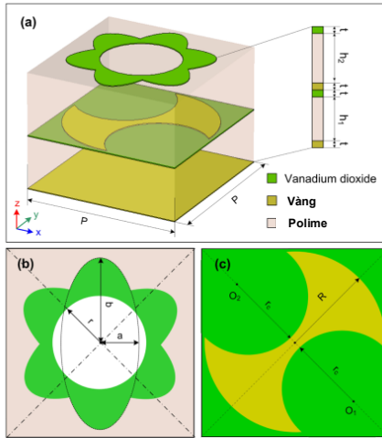
Hình 4.18. Cấu trúc ô cơ sở của MMs: (a) Hình ảnh 3D, góc nhìn từ trên xuống của (b) tám cộng hưởng cho chế độ hấp thụ và (c) tám cộng hưởng cho chế độ chuyển đổi phân cực.
