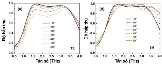
Hình 4.18. Sự phụ thuộc của độ hấp thụ vào góc tới
