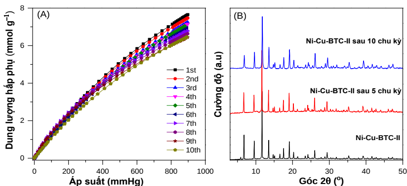
Hình 3.71. (A) Đường đẳng nhiệt hấp phụ \text{CO}_2 ở các chu kỳ hấp phụ khác nhau và (B) Giảm đồ XRD của Ni-Cu-BTC-II trước và sau các chu kỳ hấp phụ \text{CO}_2
