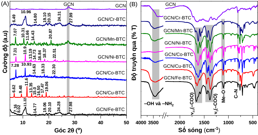
Hình 3.1. Giản đồ XRD (A) và phổ FTIR (B) của vật liệu GCN và GCN/Me-BTC
