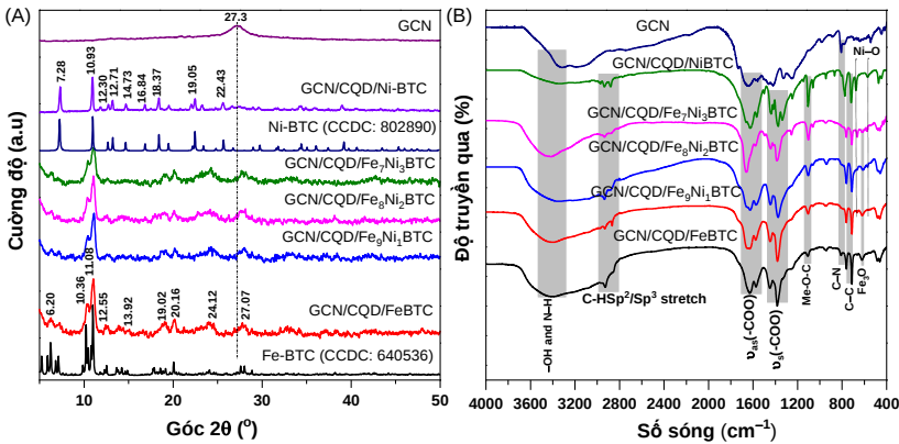
Hình 3.10. (A) Giản đồ XRD và (B) phổ FTIR của vật liệu GCN,
