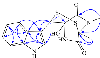
Hình 3.7. Tương tác HMBC trên hợp chất MO-01
