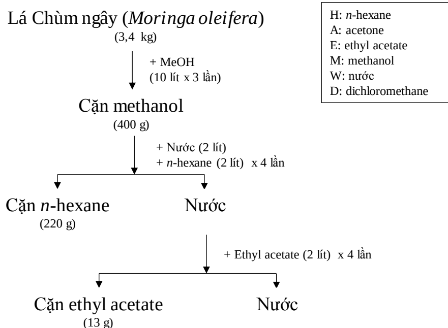
Hình 2.5. Sơ đồ chiết lá cây Chùm ngây
