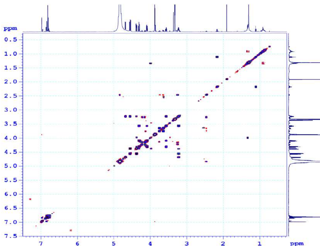
Hình 3.34. Phổ COSY của hợp chất MO-14
