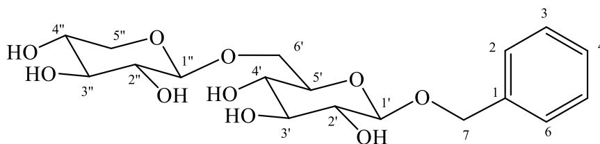
Hình 3.68. Cấu trúc hợp chất MO-30
