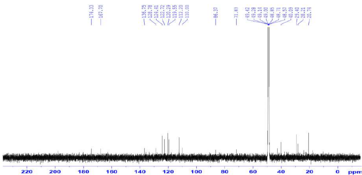
Hình 3.4. Phổ 13 C-NMR hợp chất MO-01
