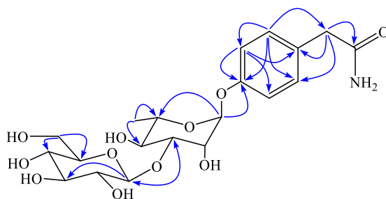
Hình 3.40. Tương tác HMBC của hợp chất MO-15
