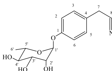
Hình 3.45. Cấu trúc của hợp chất MO-19
