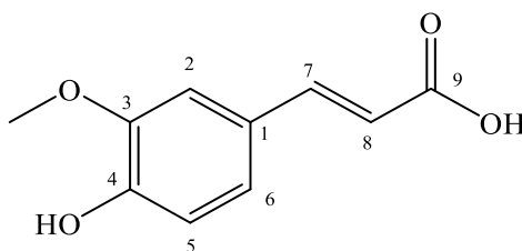
Hình 3.27. Cấu trúc hợp chất MO-13
