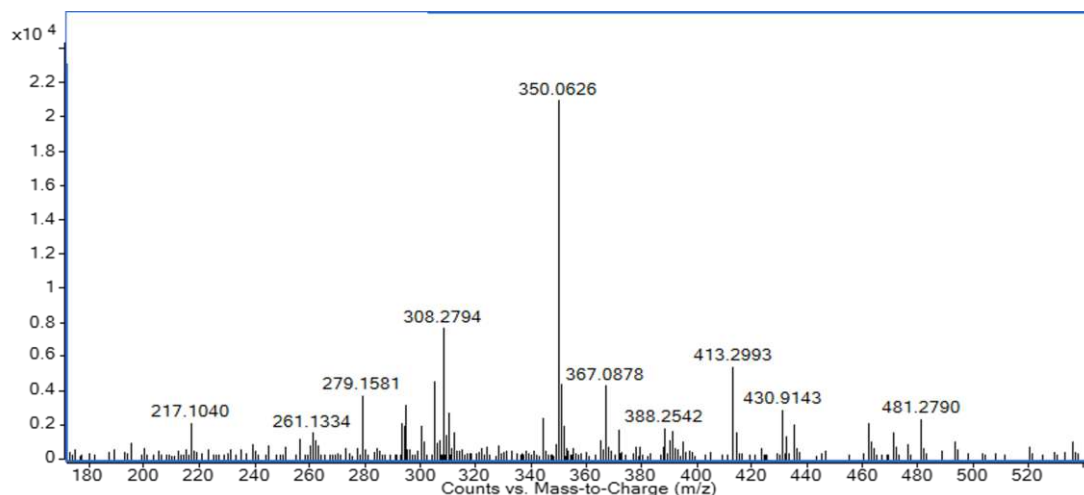
Hình 3.9. Phổ khối lượng phân giải cao HR-ESI-MS của hợp chất MO-02
