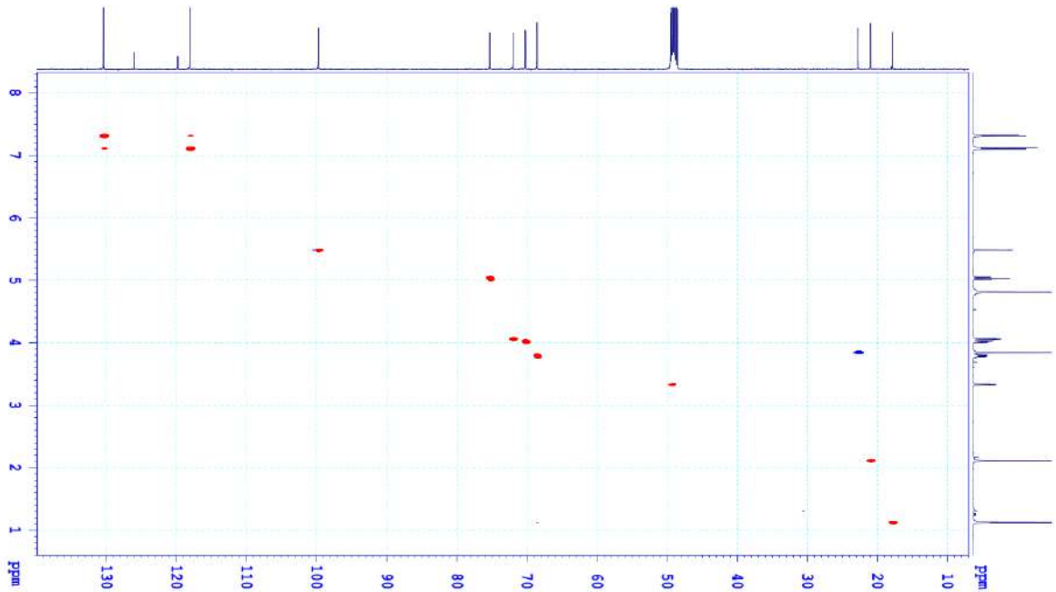
Hình 3.49. Phổ HSQC hợp chất MO-20
