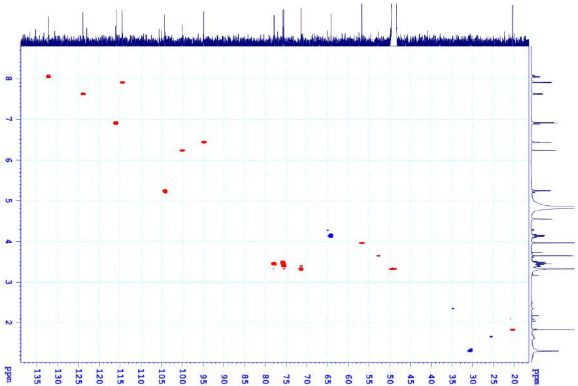
Hình 3.59. Phổ HSQC hợp chất MO-24
