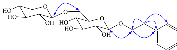
Hình 3.21. Tương tác HMBC trên hợp chất MO-08
