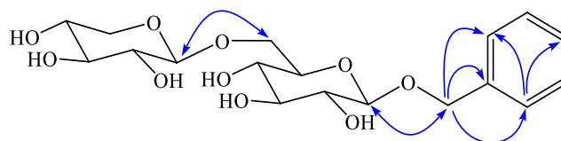
Hình 3.69. Tương tác HMBC trên hợp chất MO-30
