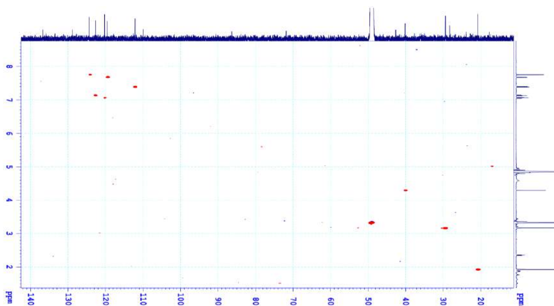
Hình 3.5. Phổ HSQC hợp chất MO-01
