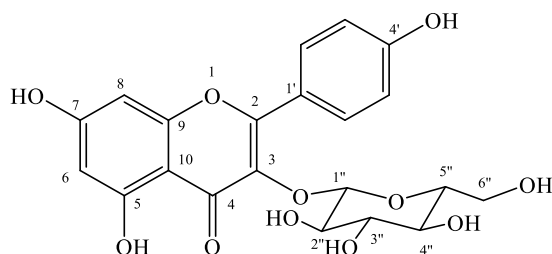
Hình 3.52. Cấu trúc hợp chất MO-21
