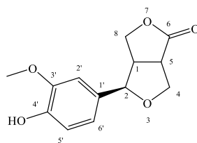
Hình 3.28. Cấu trúc hợp chất MO-14
