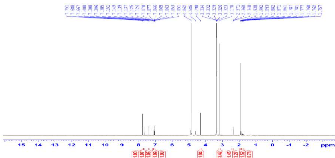
Hình 3.3. Phổ 1 H-NMR hợp chất MO-01
