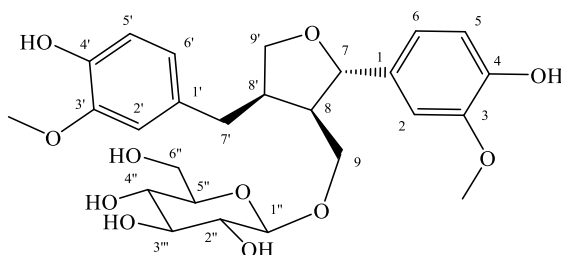
Hình 3.63. Cấu trúc hợp chất MO-26
