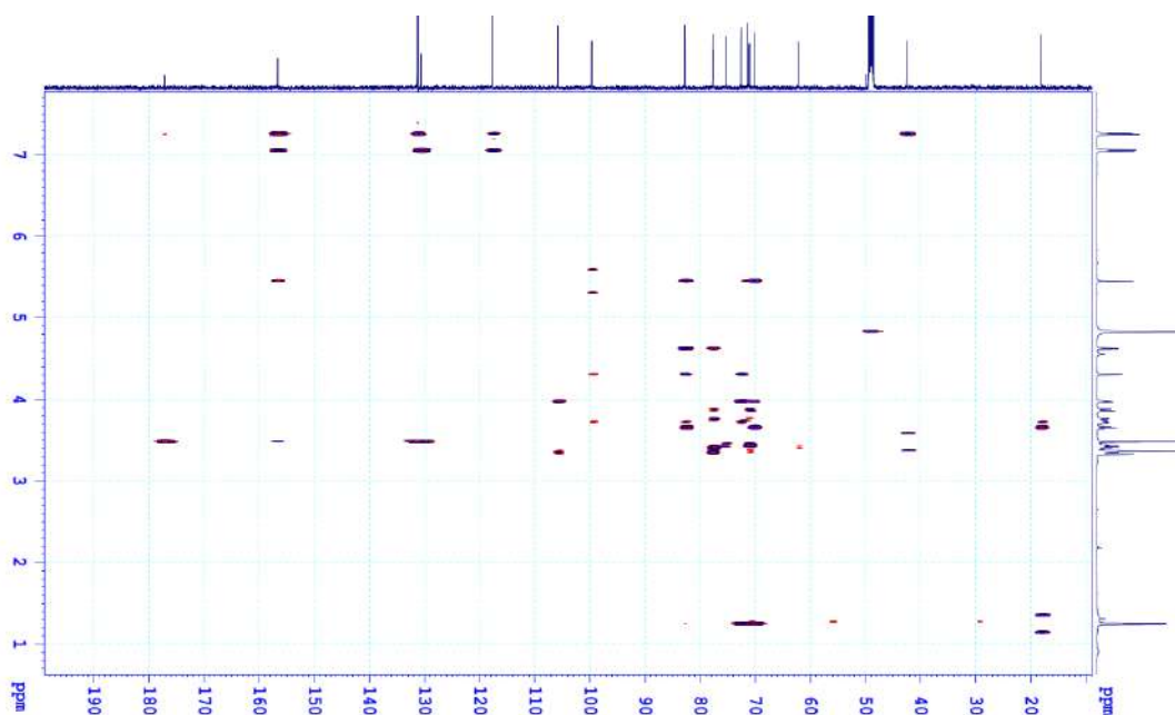
Hình 3.39. Phổ HMBC hợp chất MO-15
