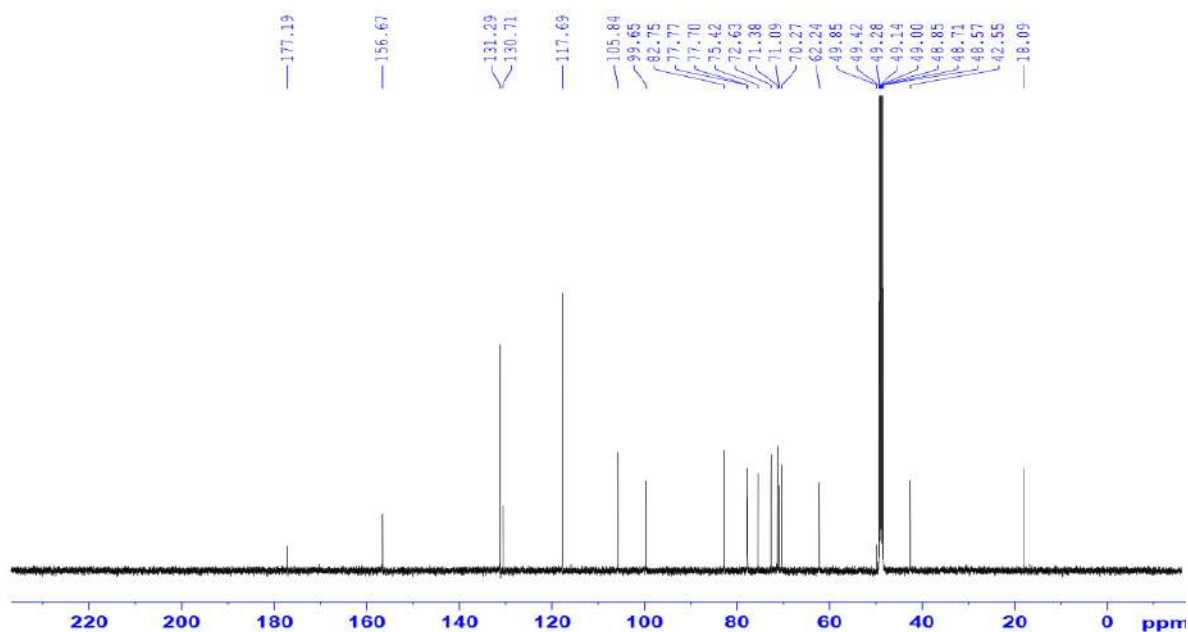
Hình 3.37. Phổ ^{13}\text{C} -NMR hợp chất MO-15
