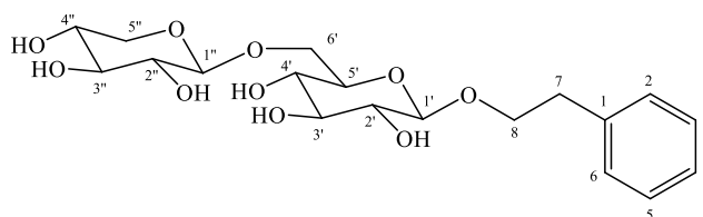
Hình 3.20. Cấu trúc hợp chất MO-08
