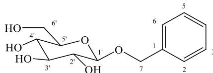
Hình 3.22. Cấu trúc hợp chất MO-09
