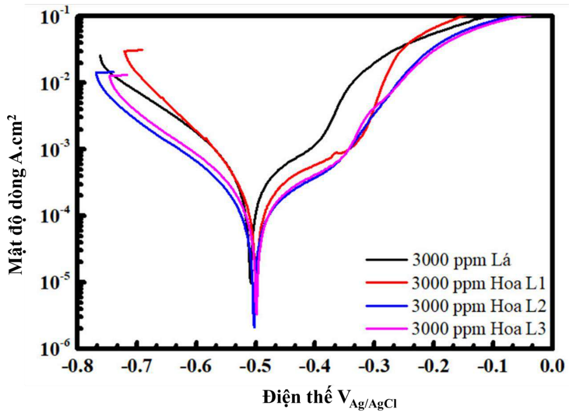
Phụ lục 48. So sánh đường cong phân cực thế động của hai nồng độ phù hợp nhất 3000 ppm cao nước hoa và lá Lộc vùng.
