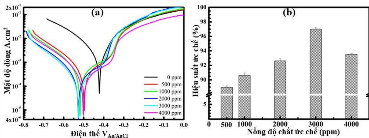
Hình 3.32. Đường cong phân cực thế động (a) và hiệu suất ức chế của thép (b) sau 24 giờ ngâm trong dung dịch HCl 1 M chứa các nồng độ BALE khác nhau.
