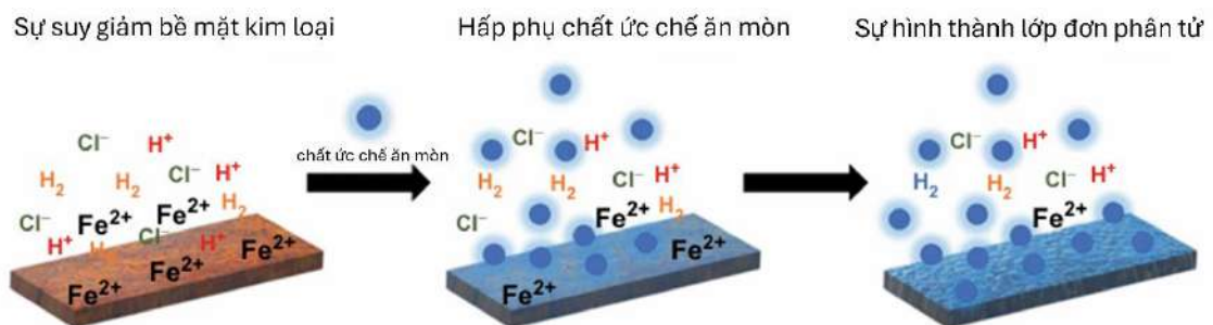
Hình 1.5. Sự hình thành lớp bảo vệ đơn phân tử trên bề mặt kim loại. (Nguồn: Ma et al. 2020 [57])
