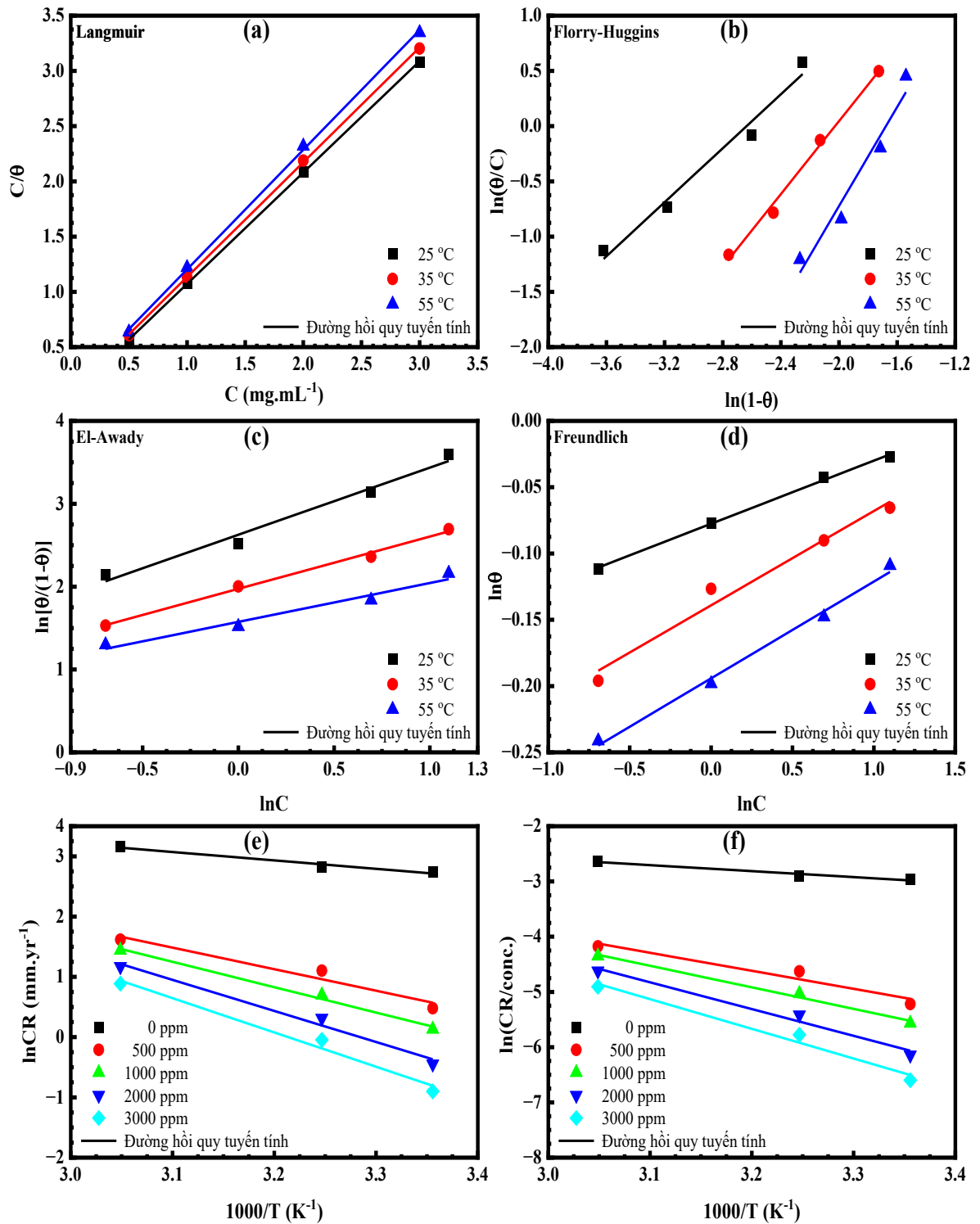
Hình 3.42. Đường tuyến tính theo mô hình hấp phụ đẳng nhiệt của (a) Langmuir, (b) Flory-Huggins, (c) El-Awady, (d) Freundlich; mối quan hệ giữa tốc độ ăn mòn - nhiệt độ trong suốt các biểu đồ (e) 1000/T so với \ln CR và (f) 1000/T so với \ln(CR/conc.) .
