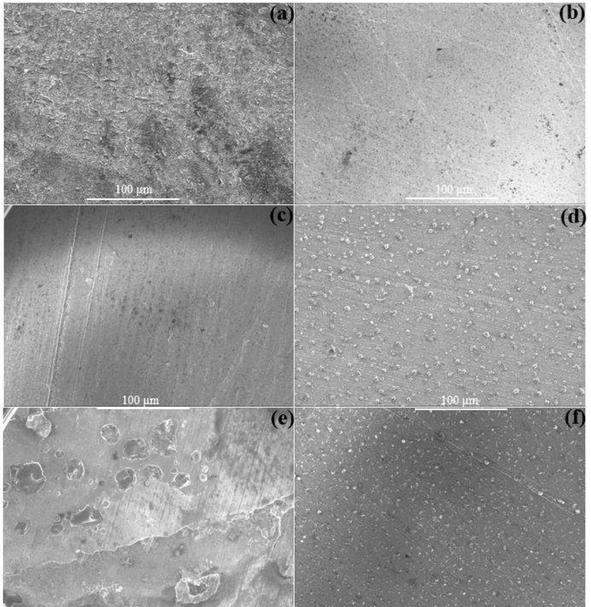
Phụ lục 46. Kết quả SEM của nền thép trong dung dịch HCl 1 M sau khi ăn mòn với độ phân giải 100 μm: (a) 0, (b) 500, (c) 1000, (d) 2000, (e) 3000 và (f) 4000 ppm BAFE.
