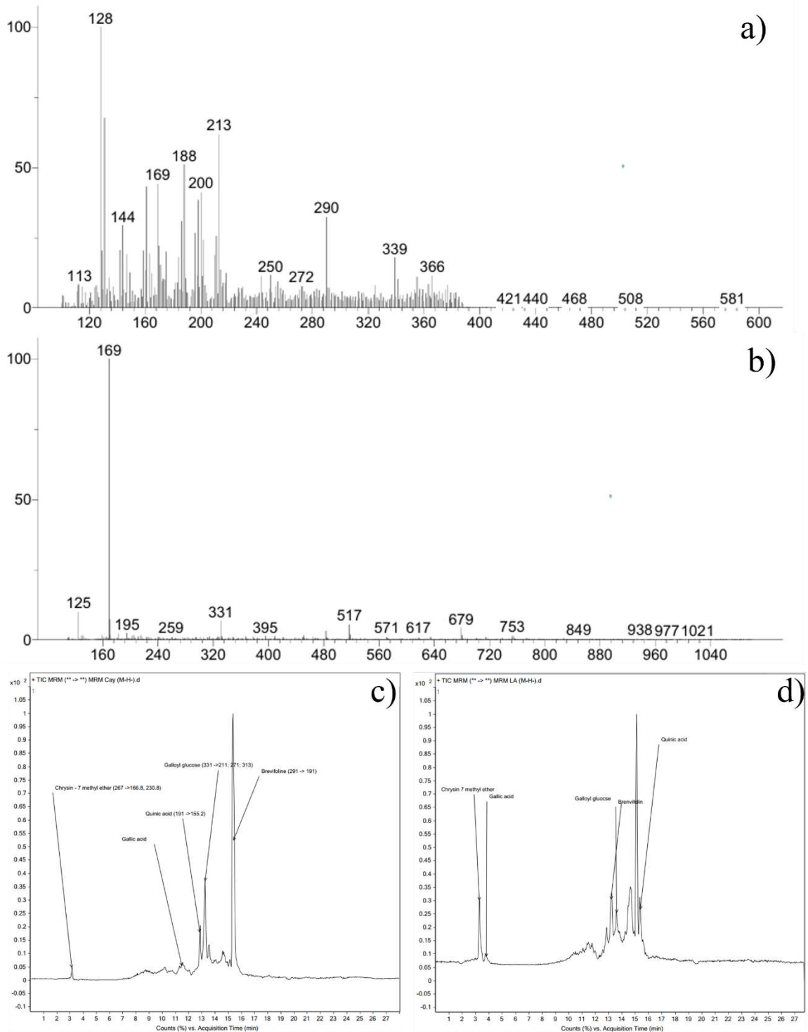
Hình 3.2. Sắc ký đồ LC-MS/MS của cao nước (a và c) hoa, (b và d) lá Lộc vùng
