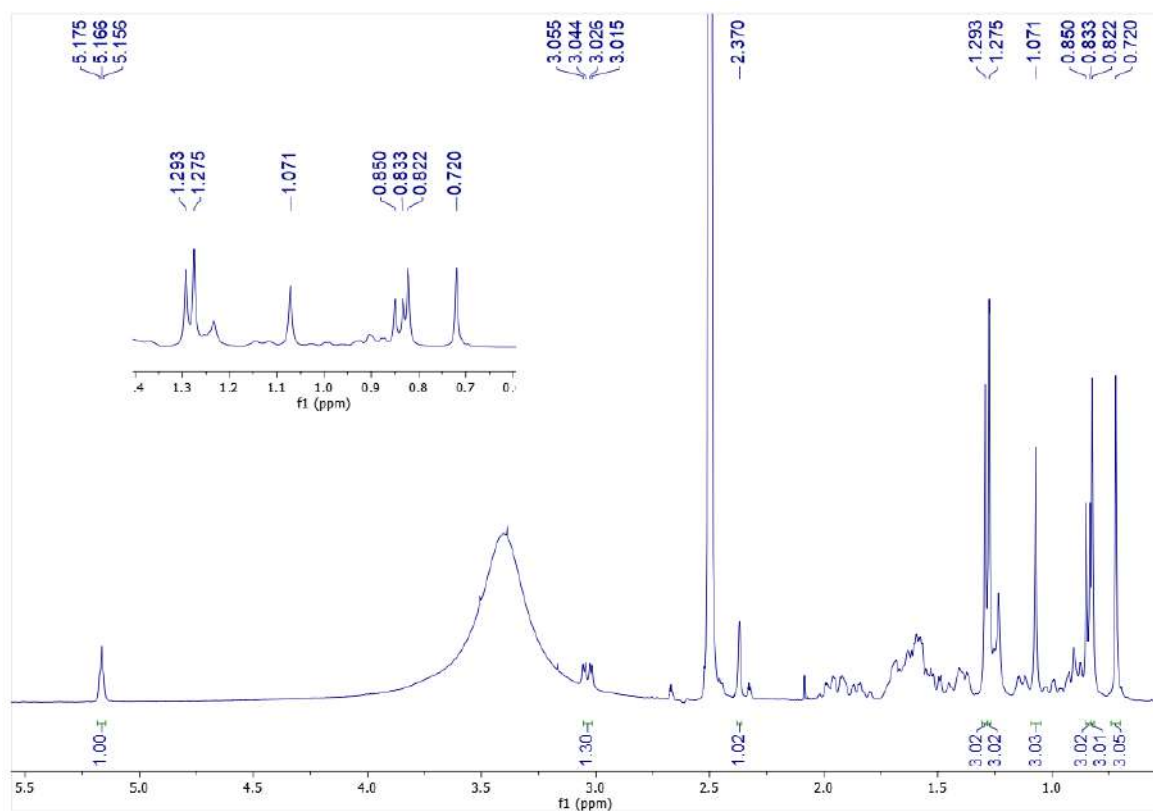
Phụ lục 36. Phổ 1 H-NMR của hợp chất 9 trong DMSO.
