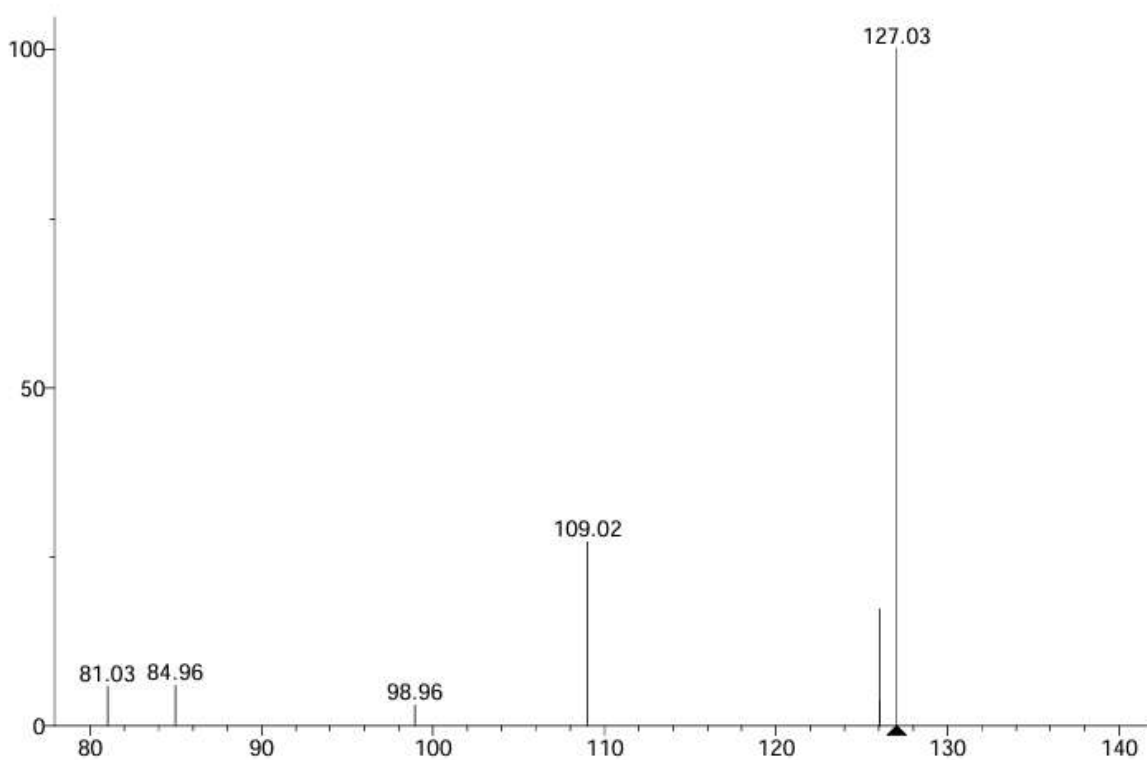
Phụ lục 8. Kết quả LC-MS/MS của cao nước hoa Lộc vùng khẳng định sự xuất hiện của hợp chất Pyrogallol tại mồi ion giả phân tử [\text{M}+\text{H}]^+ 127,03 tính cho toán [\text{C}_6\text{H}_6\text{O}_3 + \text{H}]^+ 127,0395.
