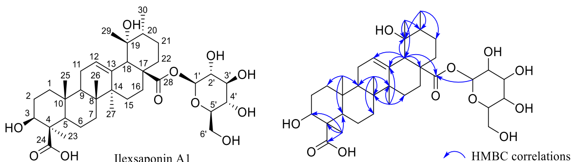
Hình 3.6. Cấu trúc hóa học và tương quan HMBC hợp chất ilexaponin A1 ( 3 ).
