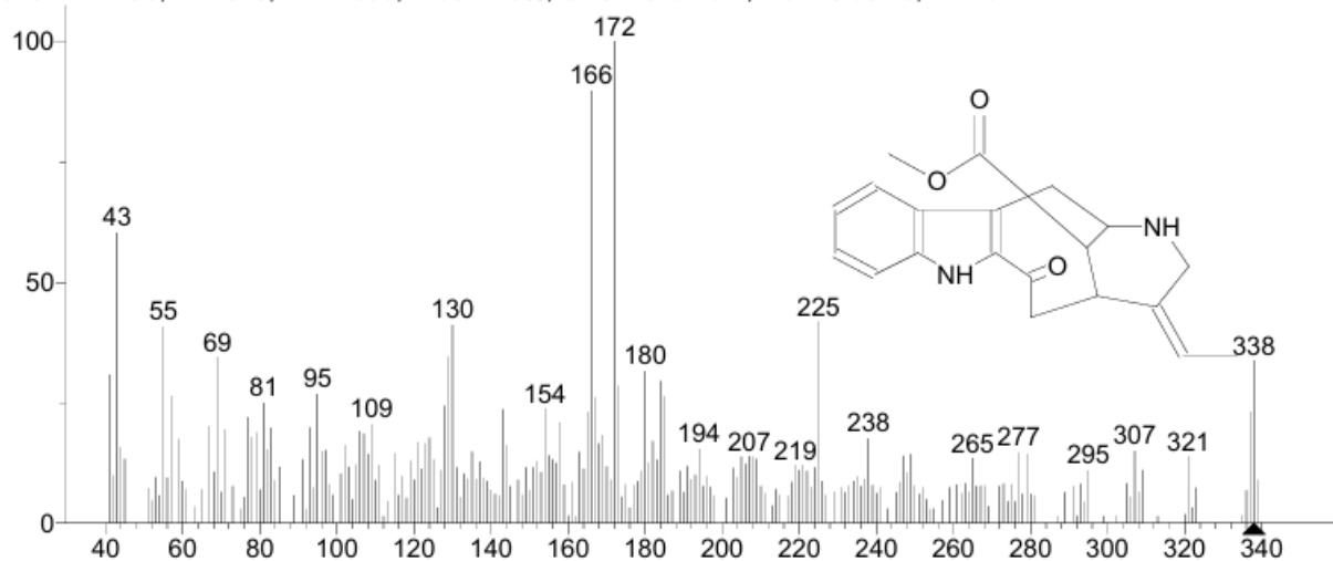
Phụ lục 2. Kết quả LC-MS/MS trên cao nước lá Lộc vùng (tiết theo).
