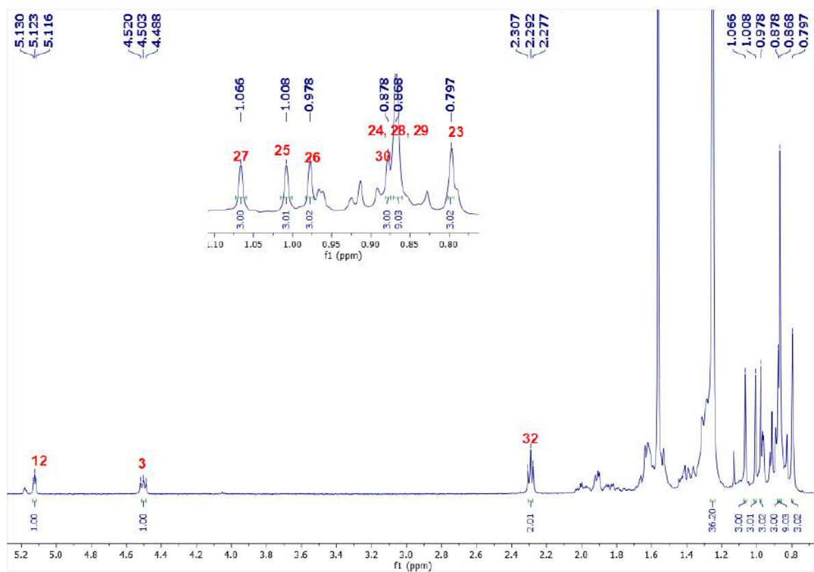
Phụ lục 33. Phổ 1 H-NMR của hợp chất 8 trong CDCl 3 .
