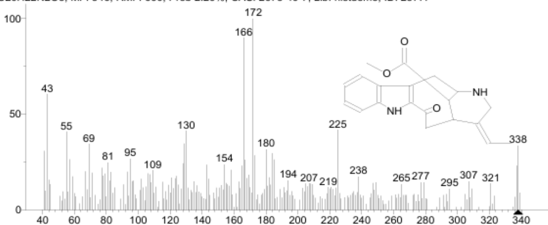
Phụ lục 1. Kết quả LC-MS/MS chi tiết trên cao nước hoa Lộc vùng.
