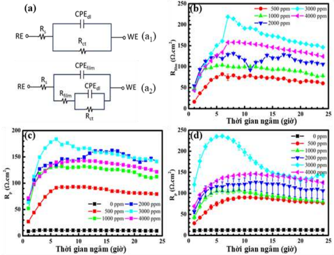
Hình 3.31. Các mạch tương đương dùng mô tả và khớp dữ liệu thực nghiệm từ phép đo EIS với mô hình mạch điện lý thuyết (a), ảnh hưởng của nồng độ BALE đến R_{film} (b), R_p từ phép đo EIS (c) và R_p phép đo LPR (d).
