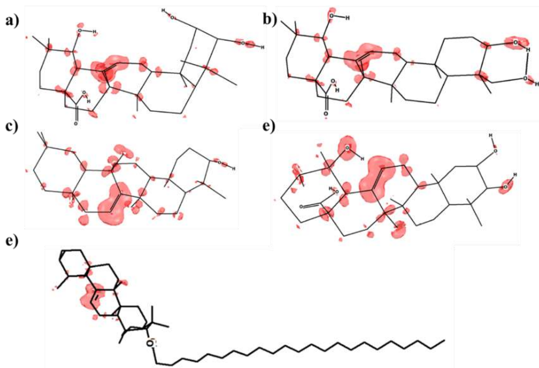
Hình 3.24. Vùng electrophile của arjunic acid (a), ilexosapogenin A (b), taraxerol (c), tormentic acid (d), 3 \beta -Docosanoyloxy-urs-12-ene (e). Chỉ các giá trị dương mới được hiển thị trong hình ảnh.
