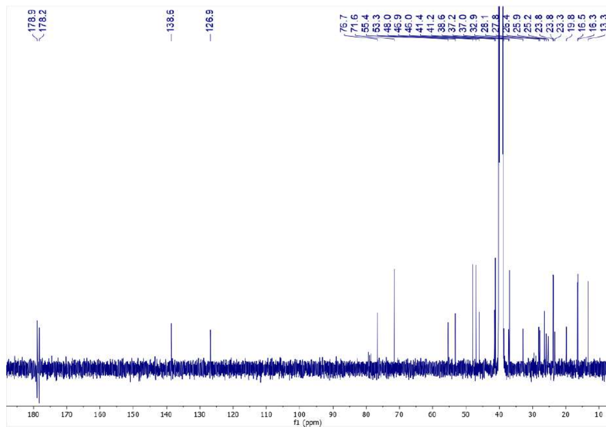
Phụ lục 37. Phổ 13 C-NMR của hợp chất 9 trong DMSO.
