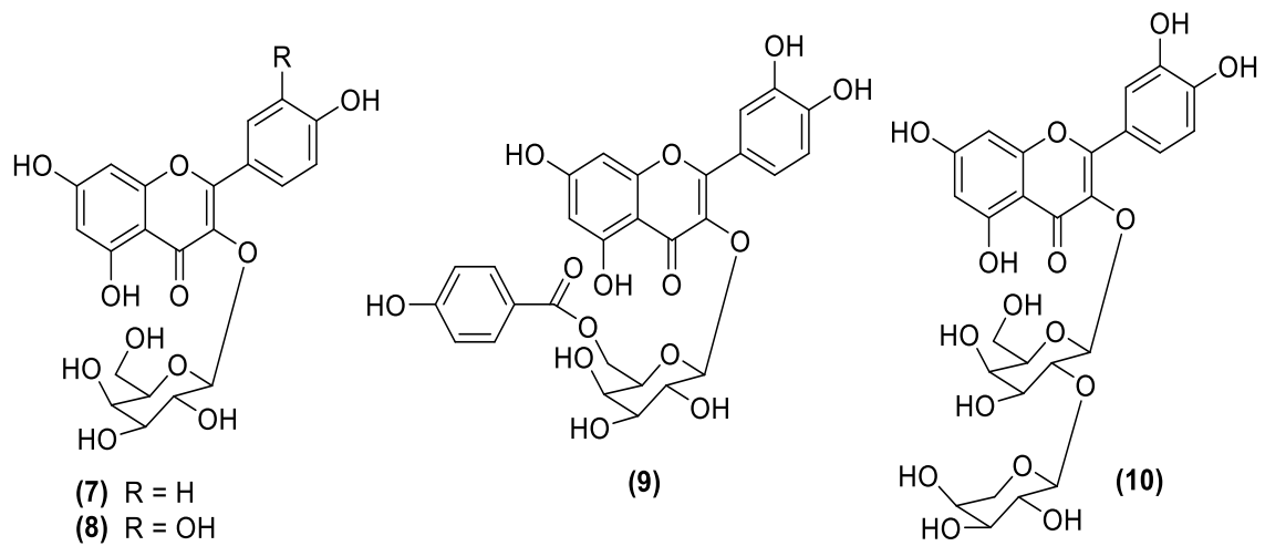
Hình 1.8. Các hợp chất được cô lập từ lá cây Lộc vừng.
