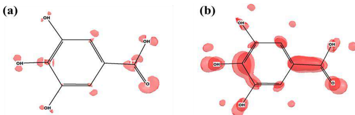
Hình 3.19. Vùng electrophile và nucleophile của GA (a và b). Chỉ các giá trị dương mới được hiển thị trong hình ảnh.
