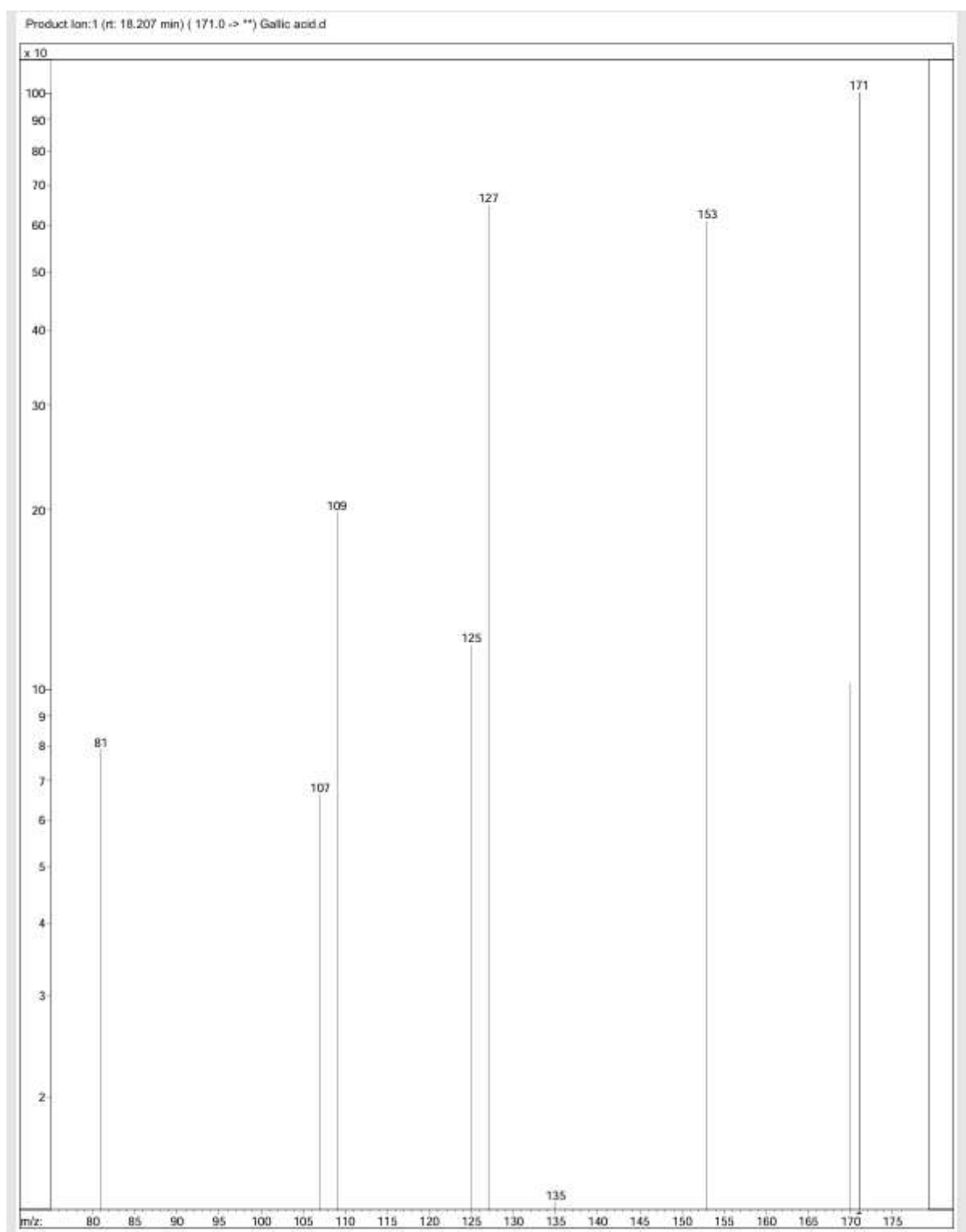
Phụ lục 4. Kết quả LC-MS/MS của cao nước hoa Lộc vùng khẳng định sự xuất hiện của hợp chất Gallic acid tại mồi ion giả phân tử [M+H]^+ 171,0 tính cho toán [C_7H_6O_5+H]^+ 171,0293.
