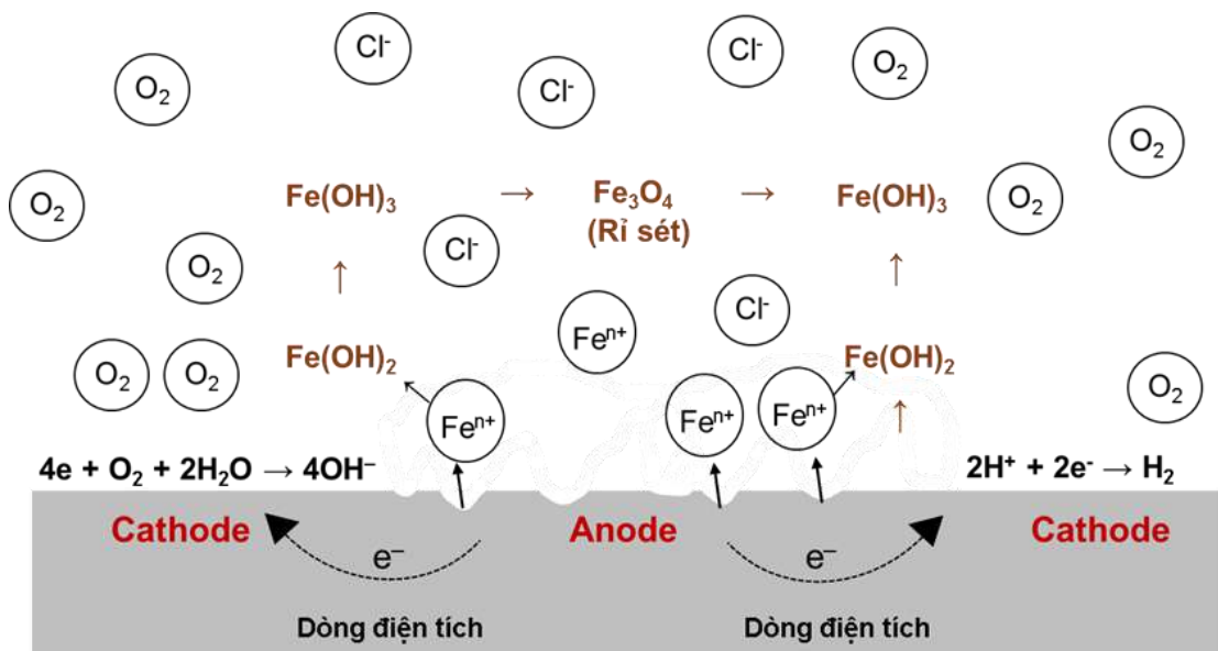
Hình 3.43. Mô phỏng cơ chế ăn mòn thép trong dung dịch HCl 1 M.
