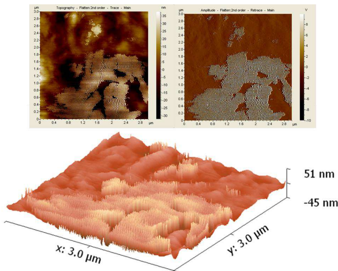
Hình 3.34. Kính hiển vi lực nguyên tử (AFM) của bề mặt thép sau 24 giờ ngâm trong dung dịch HCl 1 M chứa BAFE 3000 ppm.
