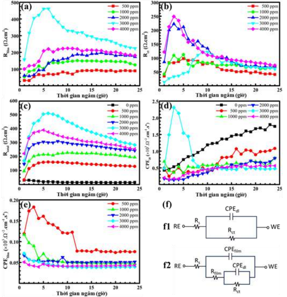
Hình 3.27. Ảnh hưởng của nồng độ BAFF và thời gian ngâm đến (a) R_{film} , (b) R_{ct} , (c) R_{total} , (d) CPE_{dl} và (e) giá trị CPE_{film} của thép carbon trong dung dịch HCl 1 M. (f) Các mạch tương đương dùng mô tả và khớp dữ liệu thực nghiệm từ phép đo EIS với mô hình mạch điện lý thuyết.
