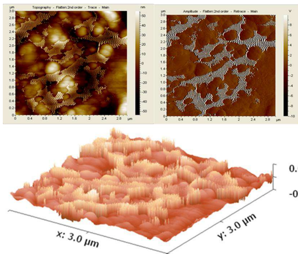
Hình 3.37. Kết quả phân tích hiển vi lực nguyên tử (AFM) của bề mặt thép sau 24 giờ ngâm trong dung dịch HCl 1 M chứa 3000 ppm BALE.
