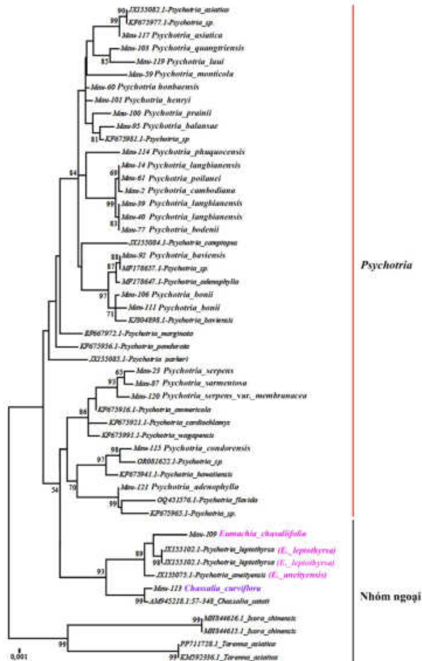
Hình 3.9. Cây phả hệ xây dựng cho các loài trong chi Psychotria được xây dựng dựa trên trình tự ITS2, theo phương pháp Maximum likelihood, bootstrap 1000 lần lặp lại với các giá trị trên 50% được giữ lại.
