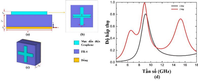
Hình 3.18. Cấu trúc MA, MMA được đề xuất (a) MA đơn lớp, (b) thiết kế lớp cộng hưởng, (c) MMA, (d) phổ hấp thụ của MA và MMA với lớp hấp thụ Graphene ( 2\Omega/\text{sq} ).
