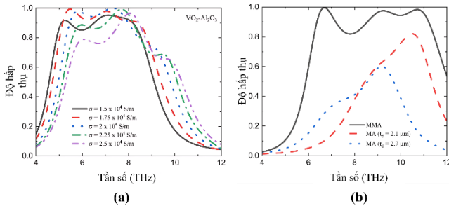
Hình 4.7. Phổ hấp thụ của MA và MMA với lớp hấp thụ VO_2 ( \sigma = 25000 \text{ S/m} )
