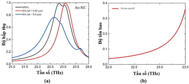
Hình 4.12. (a) Phổ hấp thụ của MA và MMA Al-SiC, (b) độ tổn hao của SiC
