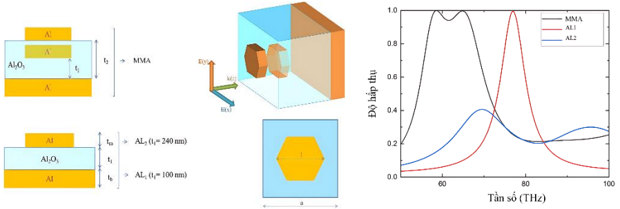
Hình 4.23. Cấu trúc MA đơn lớp và MMA, phổ hấp thụ của MA lục giác đơn lớp có độ dày khác nhau và MMA.
