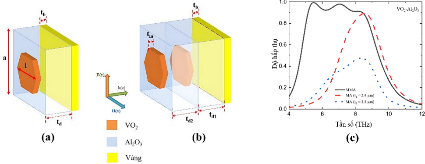
Hình 4.1. Sơ đồ cấu trúc (a) MA đơn lớp, (b) MMA hai lớp với lớp hấp thụ VO_2 , (c) phổ hấp thụ của MMA và MA đơn lớp
