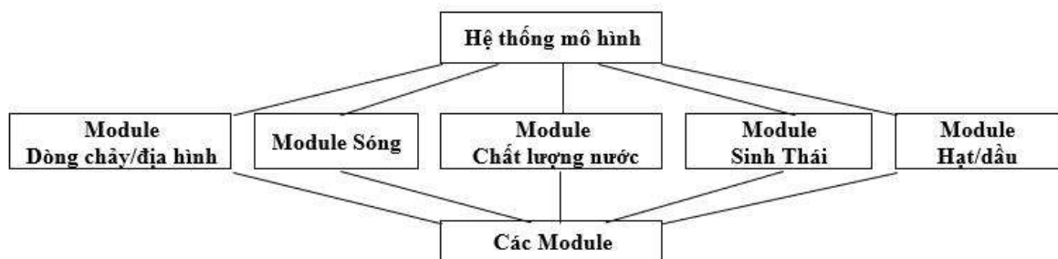
Hình 2.2. Các module trong mô hình Delft3D [133]
