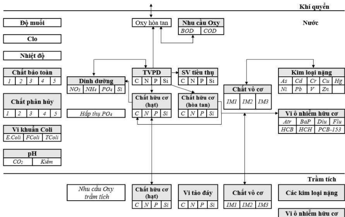
Hình 2.3. Tổng quan chung về các chất trong mô hình chất lượng nước [133]
