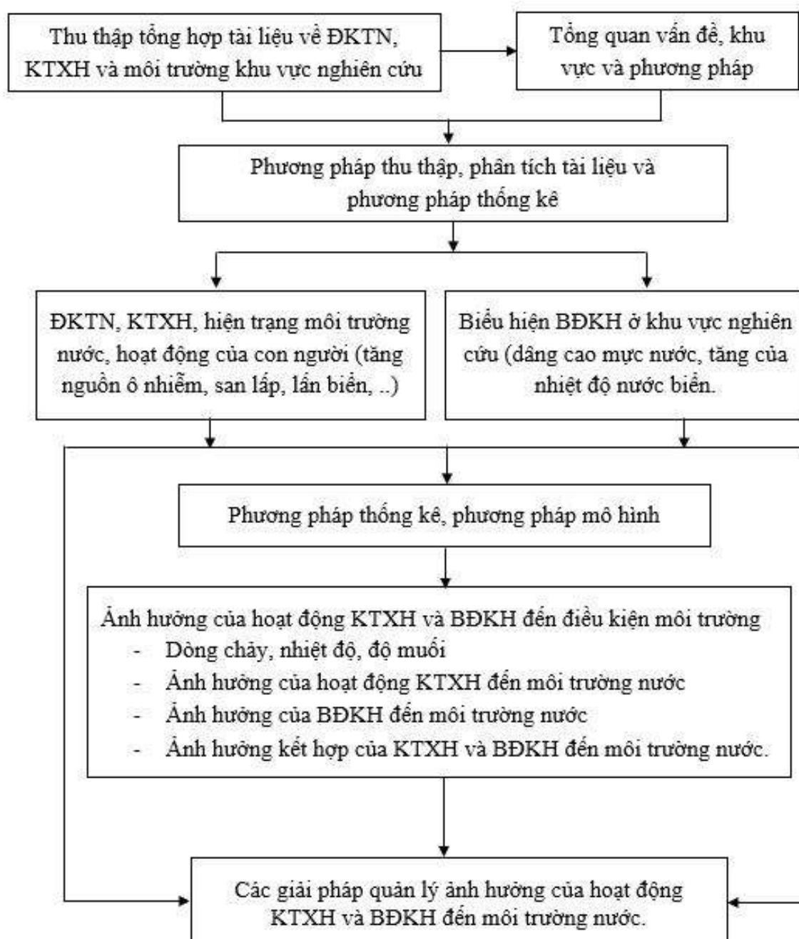
Hình 2.1. Sơ đồ tóm tắt nội dung và phương pháp nghiên cứu của luận án
