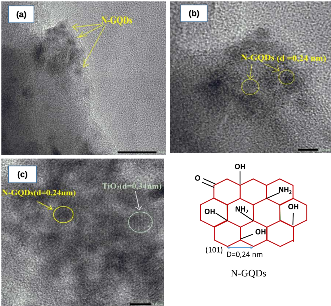
Hình 3.26. Ảnh HRTEM của (a) vật liệu N-GQDs và (b) vật liệu biến tính N-GQDs/ \text{TiO}_2
