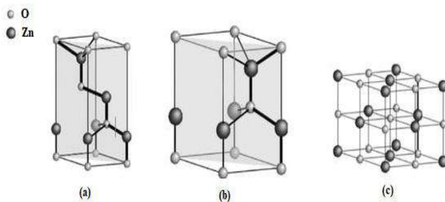
Hình 1.11. Các mô hình cấu trúc tinh thể của ZnO (a) blende (b) wurtzite và (c) rock salt [60].
