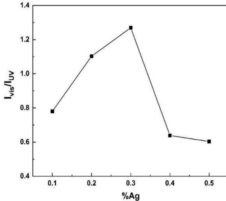
Hình 3.15. Đồ thị tỷ lệ cường độ đỉnh phát xạ bẫy sâu và bẫy nông theo hàm lượng Ag
