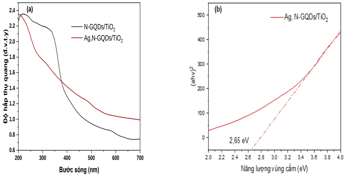
Hình 3.35. (a) Phổ hấp thụ UV-Vis và (b) đường Tauc của vật liệu Ag, N-GQDs/TiO 2
