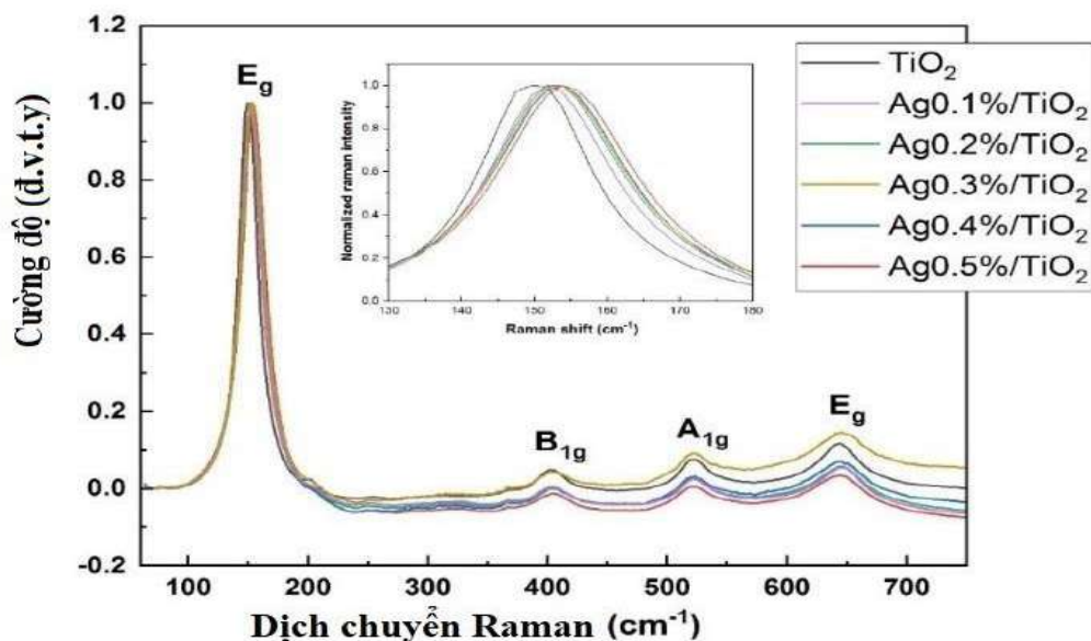
Hình 3.10. Phổ Raman của TiO 2 , Ag/TiO 2 và chi tiết các đỉnh Raman tại 150 cm -1 (hình nhỏ)
