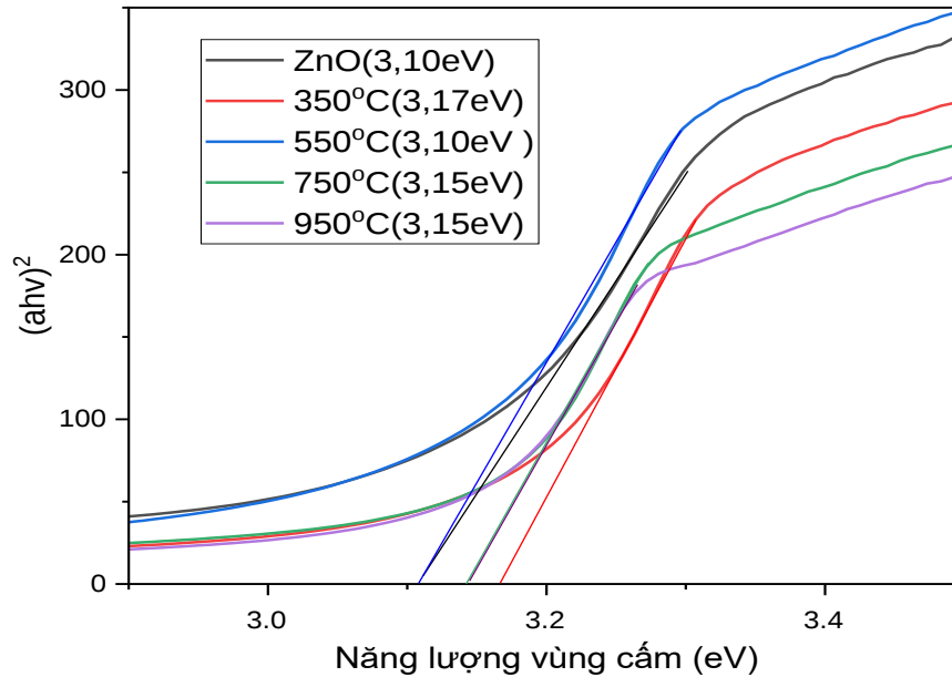
Hình 3.49. Đường Tauc và năng lượng vùng cấm của các vật liệu ZnO
