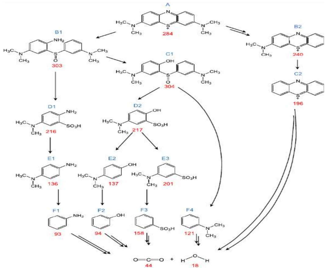
Hình 1.7. Cơ chế phân hủy MB trong phản ứng xúc tác quang [50]
