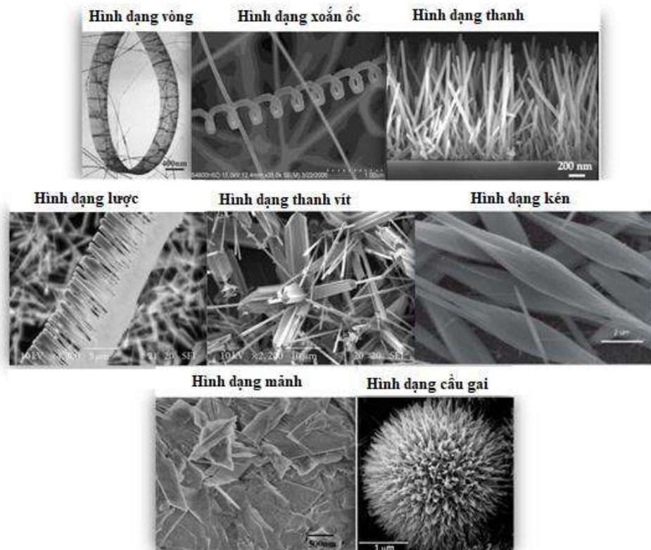
Hình 1.12. Một số hình thái cấu trúc của nano ZnO [66]
