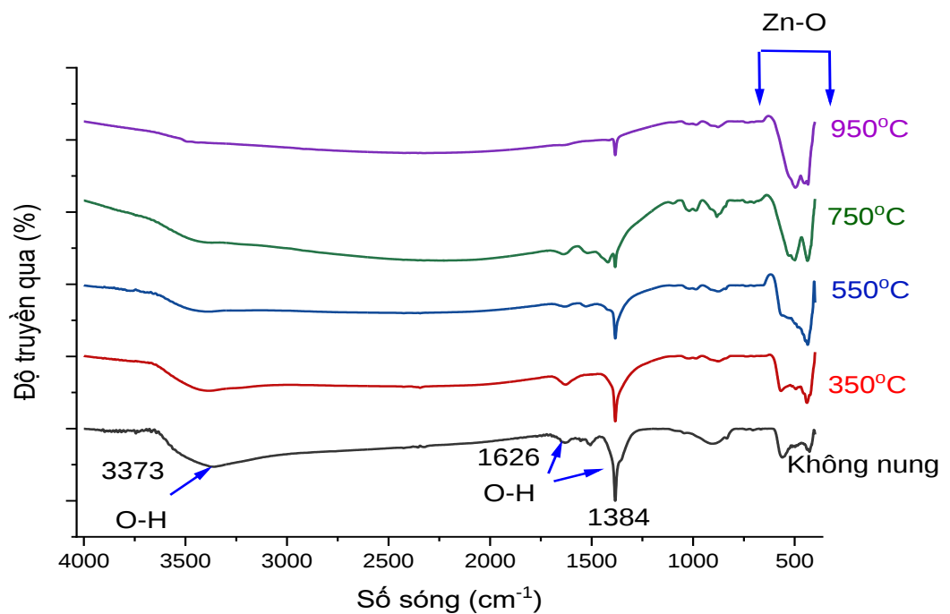
Hình 3.45. Phổ FTIR của các vật liệu ZnO
