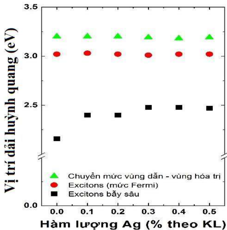
Hình 3.14. Vị trí tín hiệu PL của vật liệu \text{TiO}_2 và \text{Ag}/\text{TiO}_2
