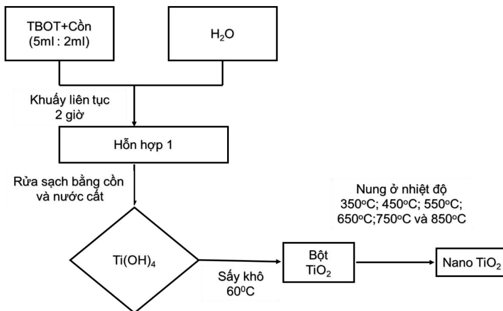
Hình 2.1. Sơ đồ chế tạo vật liệu \text{TiO}_2
