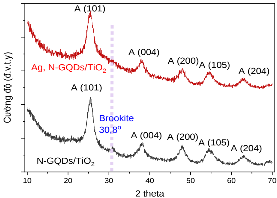
Hình 3.33. Giảm đồ XRD của vật liệu \text{N-GQDs/TiO}_2 và \text{Ag, N-GQDs/TiO}_2
