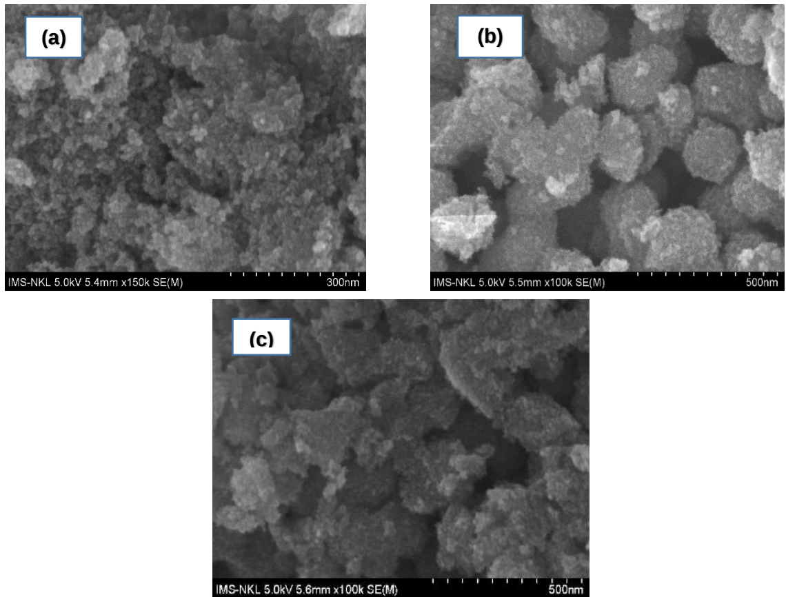
Hình 3.36. Ảnh SEM của (a) \text{TiO}_2 (b) \text{N-GQDs/TiO}_2 và (c) \text{Ag,N-GQDs/TiO}_2
