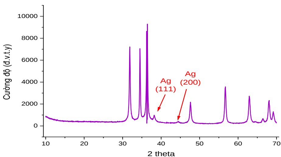
Hình 3.55. Giảm nhiễu xạ tia X của Ag5%/ZnO
