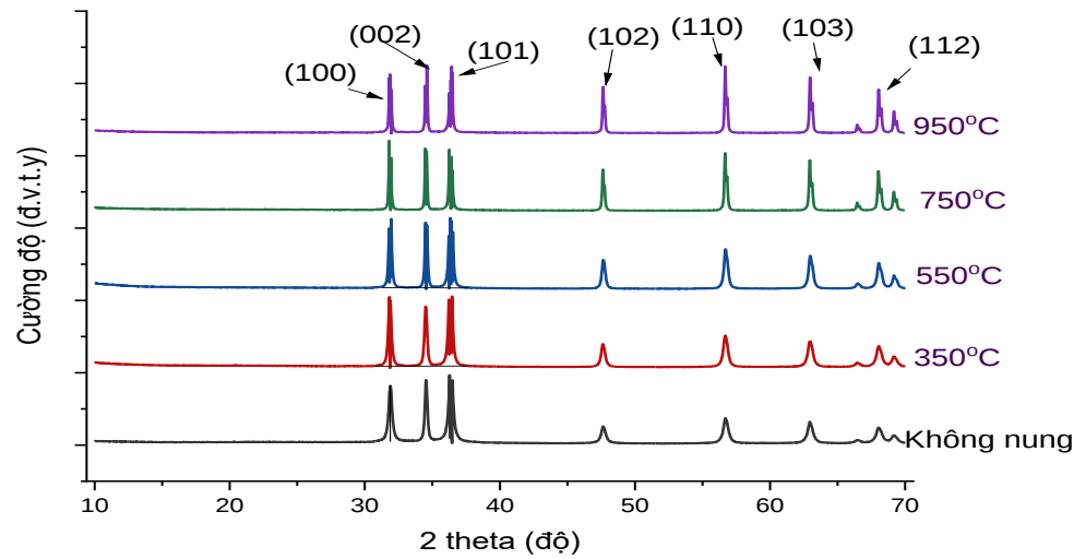
Hình 3.44. Giảm đồ nhiễu xạ tia X của ZnO không nung và nung ở các nhiệt độ khác nhau
