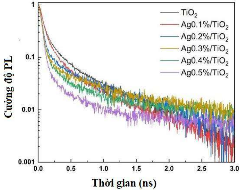
Hình 3.18. Phổ TRPL của vật liệu \text{TiO}_2 và \text{Ag/TiO}_2 tại bước sóng 496 - 516 nm
