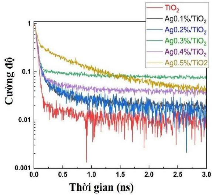
Hình 3.16. Phổ TRPL của vật liệu \text{TiO}_2 và \text{Ag/TiO}_2 tại bước sóng 410 nm
