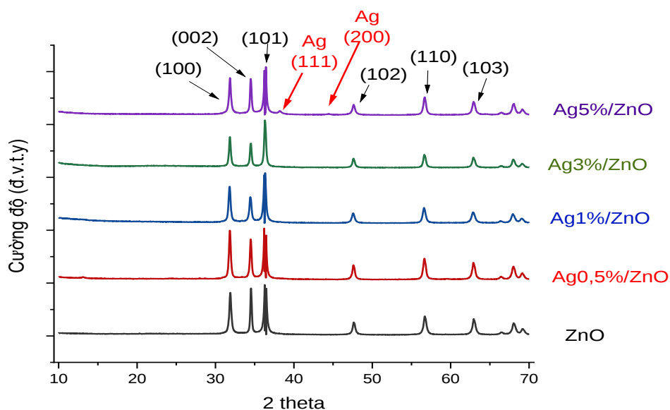
Hình 3.54. Giảm nhiễu xạ tia X của vật liệu ZnO và Ag/ZnO
