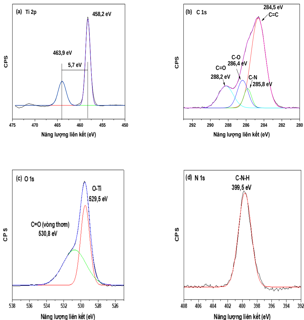
Hình 3.27. Phổ XPS (a) Ti 2p, (b) C 1s, (c) O 1s và (d) N 1s của vật liệu N-GQDs/TiO 2
