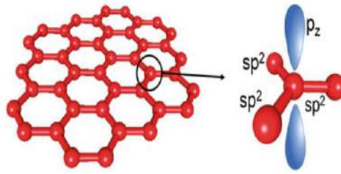
Hình 1.15. Mạng lưới tinh thể của cacbon (bên trái) và liên kết của nguyên tử tạo bởi các electron hóa trị của nguyên tử cacbon [79]
