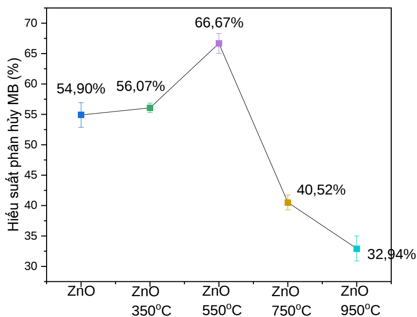
Hình 3.53. Hiệu suất phân hủy MB của các vật liệu ZnO không nung và nung ở nhiệt độ khác nhau sau 50 phút chiếu UV
