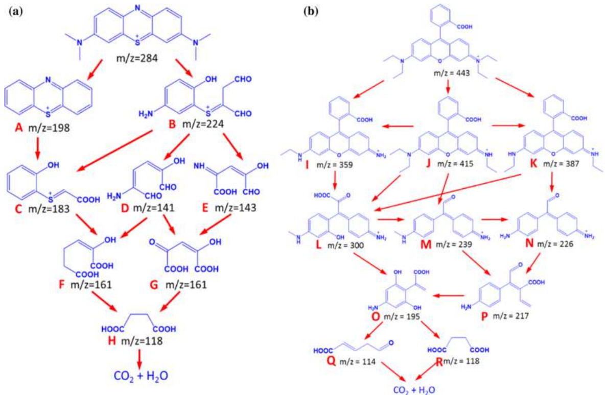
Hình 1.8. Cơ chế phân hủy (a) MB và (b) RhB trong phản ứng xúc tác quang [51]
