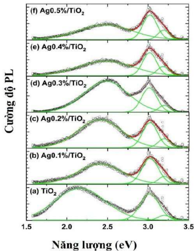
Hình 3.13. Phổ phát quang PL của \text{TiO}_2 (a), \text{Ag}0.1\%/\text{TiO}_2 (b), \text{Ag}0.2\%/\text{TiO}_2 (c), \text{Ag}0.3\%/\text{TiO}_2 (d), \text{Ag}0.4\%/\text{TiO}_2 (e) và \text{Ag}0.5\%/\text{TiO}_2 (f). Đường mở rộng là đường thực nghiệm và các đường thành phần là đỉnh phát xạ được khớp theo Gauss
