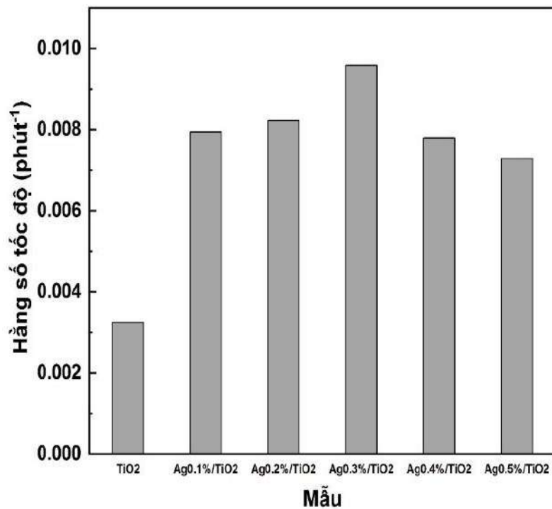
Hình 3.20. Hằng số tốc độ phản ứng phân hủy MB của vật liệu \text{TiO}_2 và các vật liệu Ag/ \text{TiO}_2
