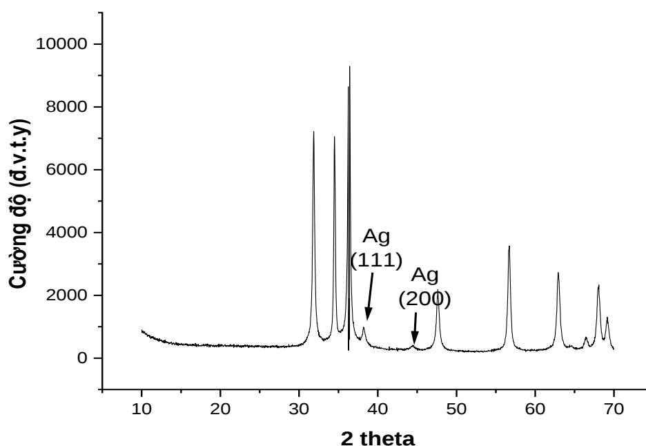
Hình 3.70. Giản đồ XRD của vật liệu Ag, N-GQDs/ZnO
