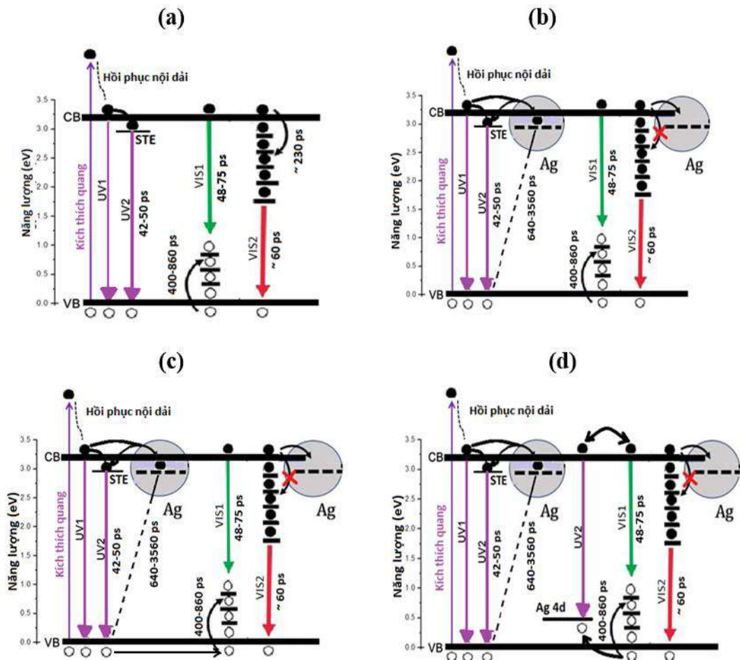
Hình 3.17. Mô hình các đường phân rã có thể trong quá trình kích thích quang của vật liệu (a) \text{TiO}_2 , (b) \text{Ag}0,1\%-0,2\%/\text{TiO}_2 , (c) \text{Ag}0,3\%/\text{TiO}_2 , (d) \text{Ag}0,4\%-0,5\%/\text{TiO}_2
