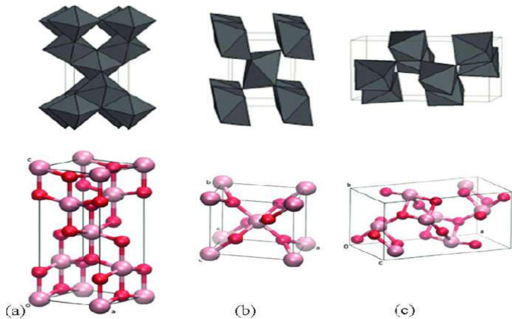
Hình 1.10. Cấu trúc tinh thể của \text{TiO}_2 (a) anatase (b) rutile (c) brookite [54]
