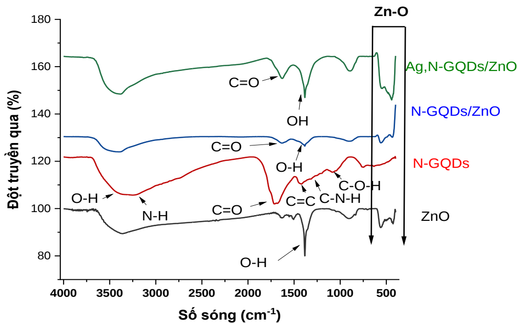
Hình 3.68. Phổ FTIR của ZnO, N-GQDs/ZnO và Ag, N-GQDs/ZnO
