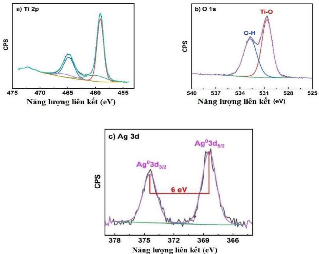
Hình 3.12. Phổ XPS phân giải cao của Ti 2p, O 1s và Ag 3d của vật liệu \text{Ag}/\text{TiO}_2
