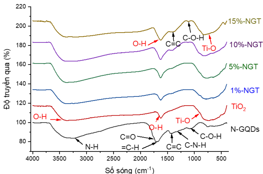
Hình 3.22. Phổ FTIR của vật liệu \text{TiO}_2 và vật liệu N-GQDs/ \text{TiO}_2
