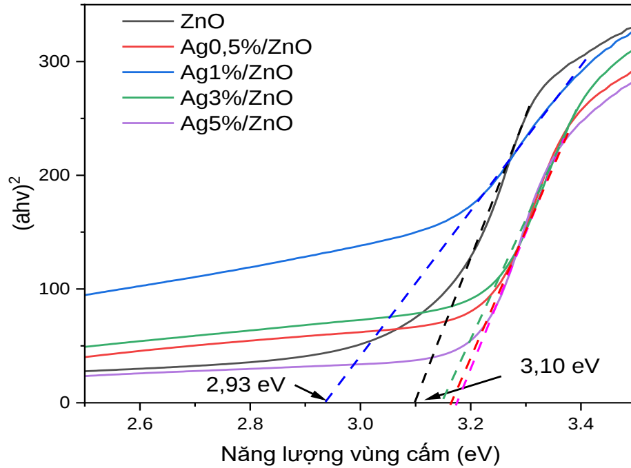
Hình 3.57. Đường Tauc và năng lượng vùng cấm của ZnO và Ag/ZnO hàm lượng khác nhau
