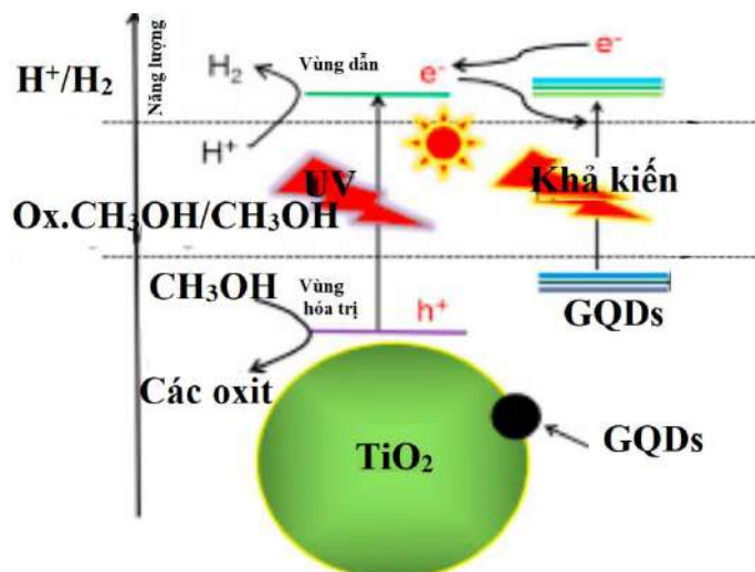
Hình 1.21. Cơ chế vận chuyển điện tích của GQDs và \text{TiO}_2 [90]
