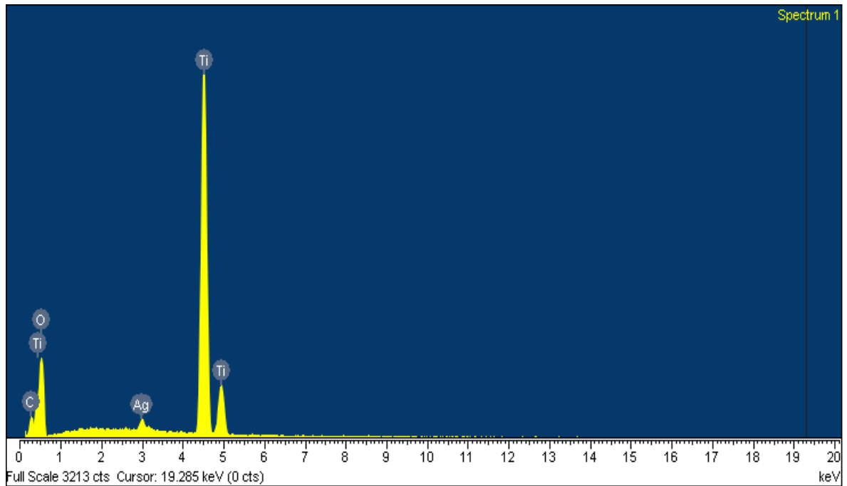
Hình 3.38. Phổ EDX của vật liệu Ag, N-GQDs/TiO 2
