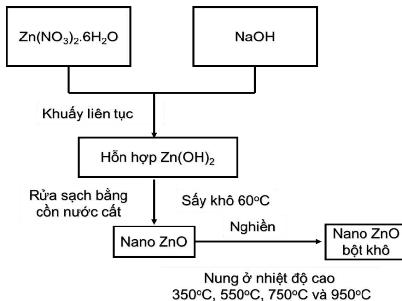
Hình 2.6. Sơ đồ chế tạo vật liệu ZnO
