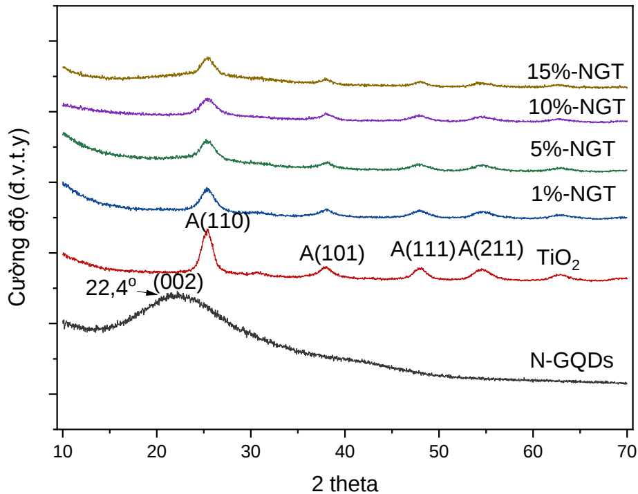
Hình 3.21. Giản đồ XRD của \text{TiO}_2 và các vật liệu N-GQDs/ \text{TiO}_2
