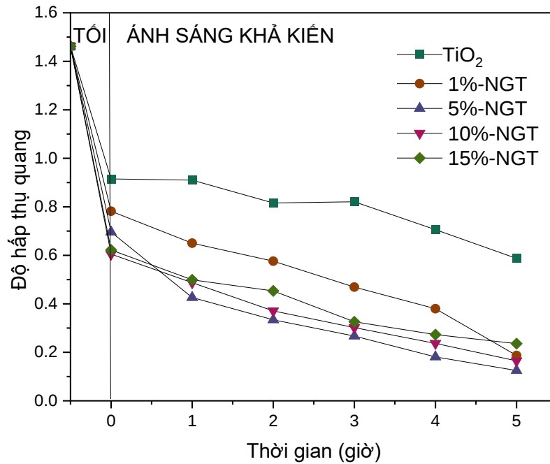
Hình 3.28. Độ hấp thụ quang của quá trình phân hủy MB dưới sự chiếu xạ của ánh sáng khả kiến sử dụng xúc tác TiO 2 và xúc tác N-GQDs/TiO 2
