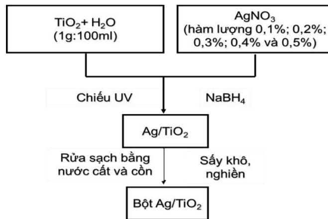
Hình 2.2. Sơ đồ chế tạo vật liệu \text{TiO}_2 biến tính kim loại quý Ag
