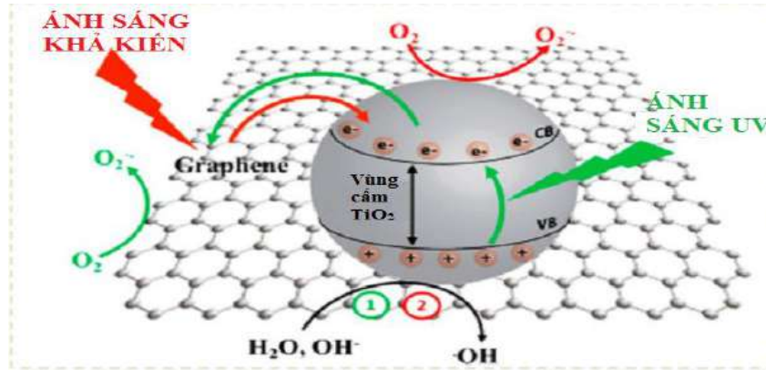
Hình 1.19. Cơ chế hoạt động xúc tác quang của vật liệu \text{TiO}_2/\text{graphene} dưới sự chiếu xạ ánh sáng UV và khả kiến [89]
