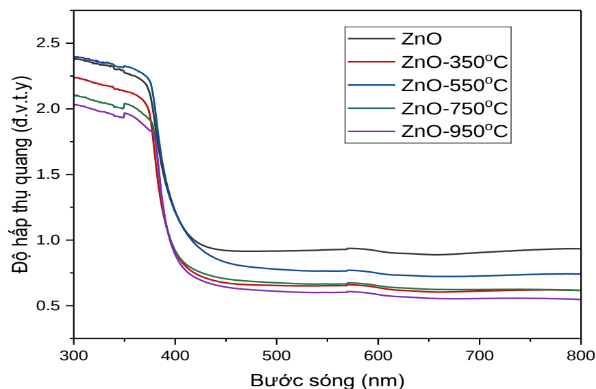
Hình 3.48. Phổ hấp thụ quang UV-Vis của ZnO không nung và ZnO được nung ở các nhiệt độ khác nhau
