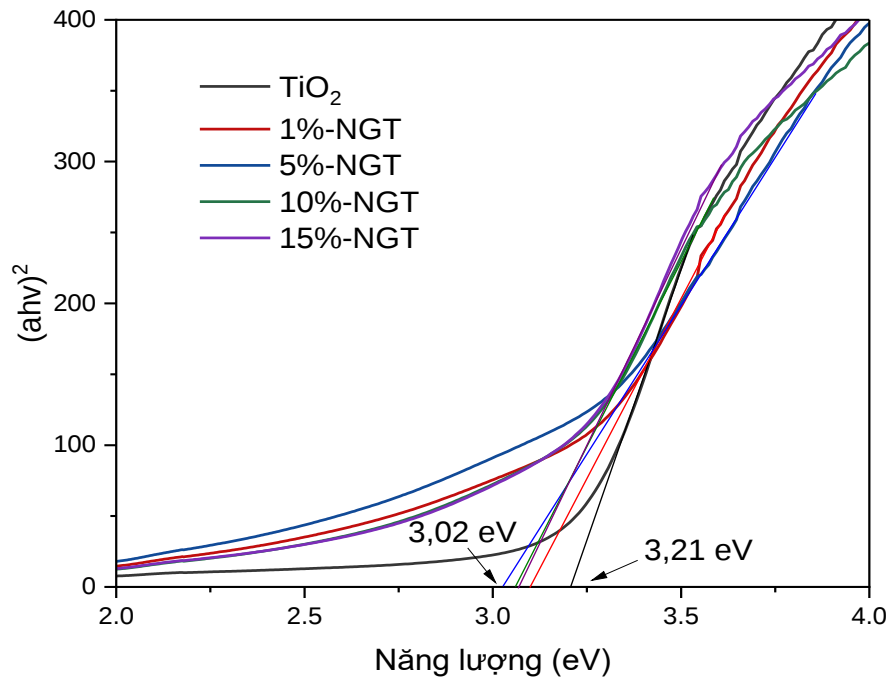
Hình 3.24. Đường Tauc và năng lượng vùng cấm của vật liệu \text{TiO}_2 và vật liệu N-GQDs/ \text{TiO}_2
