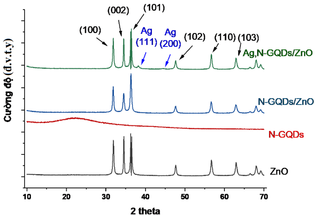
Hình 3.69. Giản đồ XRD của vật liệu ZnO, N-GQDs/ZnO và Ag, N-GQDs/ZnO
