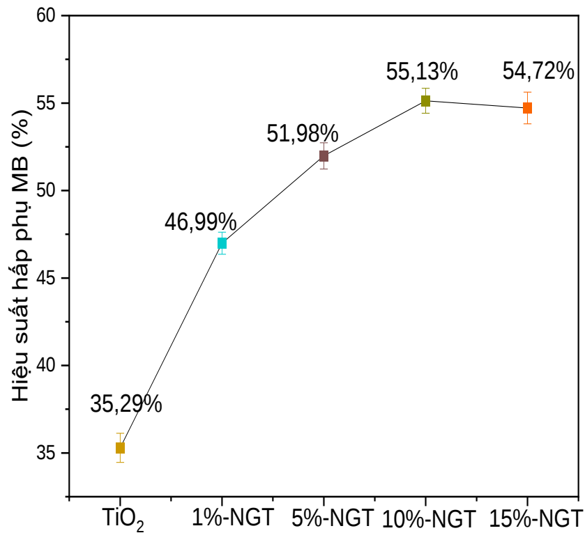
Hình 3.29. Khả năng hấp phụ MB của vật liệu TiO 2 và N-GQDs/TiO 2
