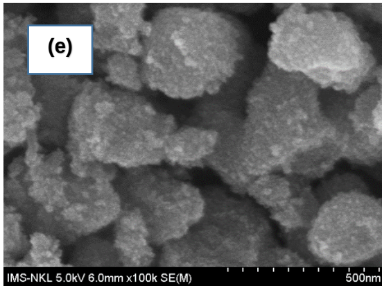
Hình 3.25. Ảnh SEM của (a) \text{TiO}_2 (b) 1%-NGT (c) 5%-NGT (d) 10%-NGT và (e) 15%-NGT
