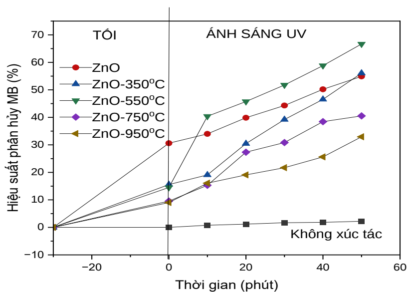
Hình 3.51. Đồ thị hiệu suất phân hủy MB sử dụng xúc tác ZnO nung ở nhiệt độ khác nhau
