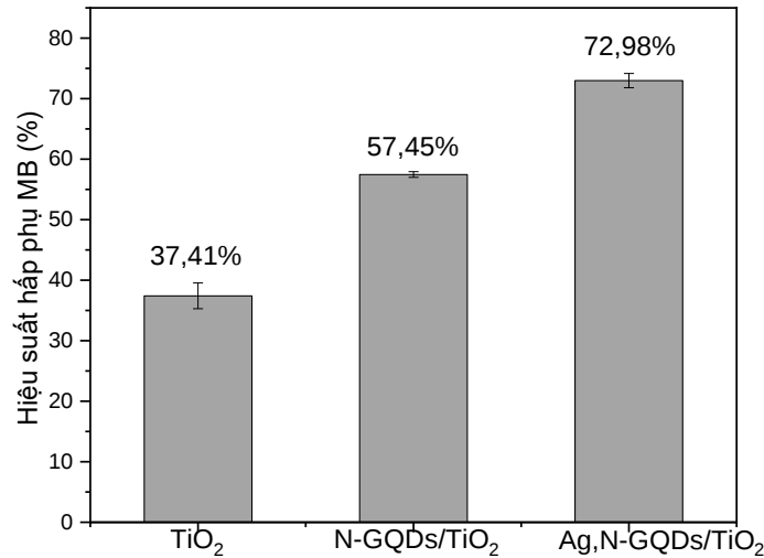
Hình 3.41. Khả năng hấp phụ MB lên trên bề mặt vật liệu TiO 2 , N-GQDs/TiO 2 và Ag, N-GQDs/TiO 2
