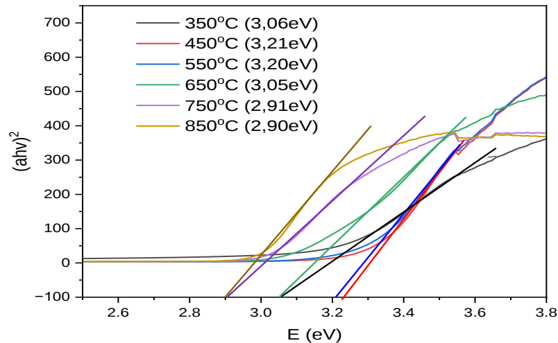
Hình 3.4. Đường Tauc và năng lượng vùng cấm (eV) của các mẫu \text{TiO}_2 nung ở nhiệt độ khác nhau
