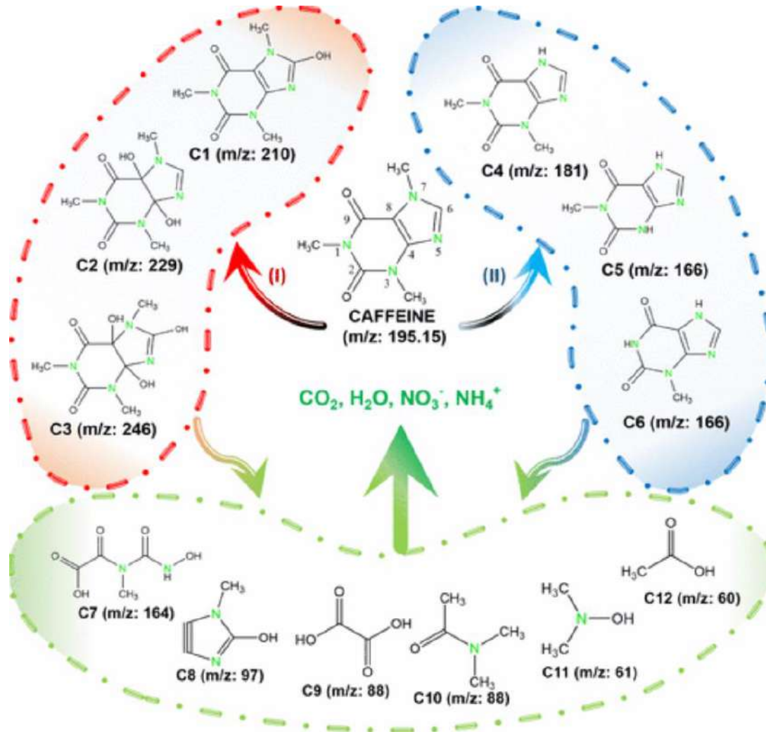
Hình 1.9. Cơ chế phân hủy caffeine trong phản ứng xúc tác quang [52]
