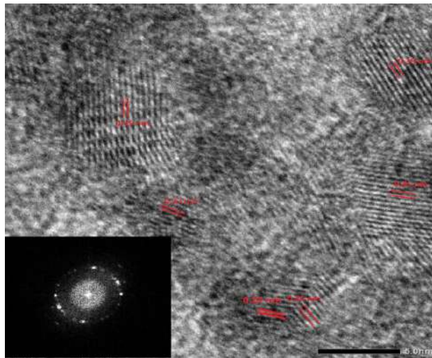
Hình 3.11. Ảnh HRTEM ở độ phóng đại cao của vật liệu Ag/TiO 2
