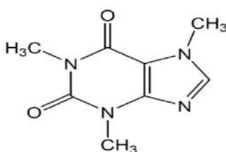
Hình 1.6. Cấu trúc hóa học của caffeine [48]
