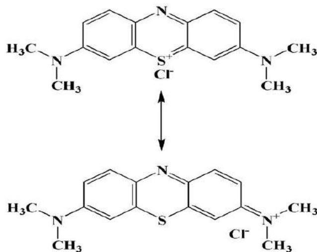
Hình 1.4. Cấu trúc hóa học của xanh methylene [44]
