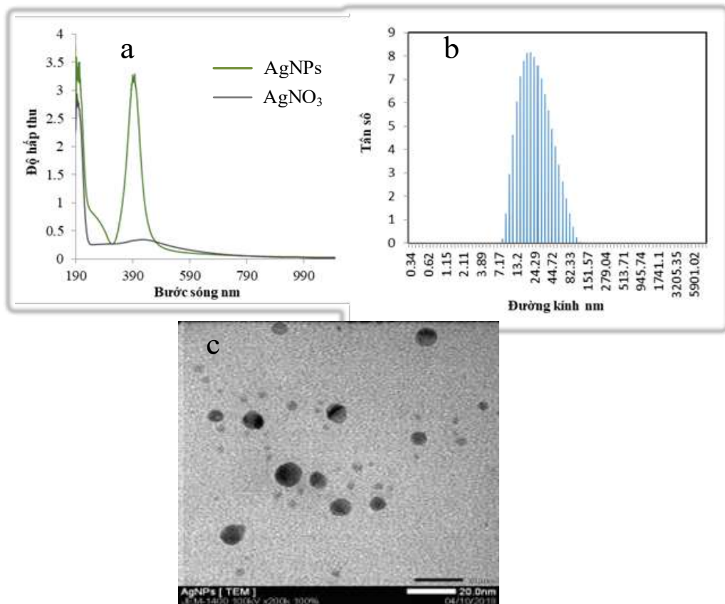
Hình 3.36. (a) Phổ UV-Vis của AgNPs; (b) biểu đồ phân bố kích thước hạt; (c) ảnh TEM của AgNPs.
