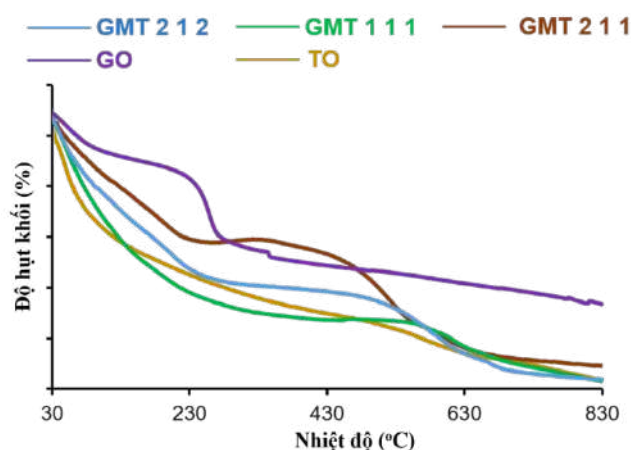
Hình 3.35. Đồ thị TGA của các mẫu GMT 111, GMT 211, GMT 212, so sánh với nano TiO 2 anatase (TO) và GO.
