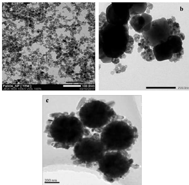
Hình 3.12. Ảnh TEM của nano \text{Fe}_3\text{O}_4 (a) và vật liệu \text{Fe}_3\text{O}_4\text{@TiO}_2 (MT@ 12) (b) và \text{Fe}_3\text{O}_4\text{@TiO}_2 (c) tổng hợp bởi Q. Zhang và cộng sự [45].
