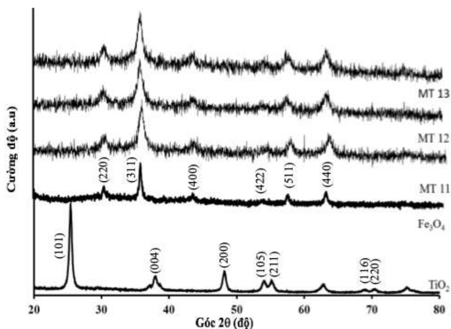
Hình 3.9. Giải đồ XRD của \text{Fe}_3\text{O}_4 , \text{TiO}_2 anatase và vật liệu \text{MT@} ở các tỷ lệ 1:1, 1:2, 1:3
