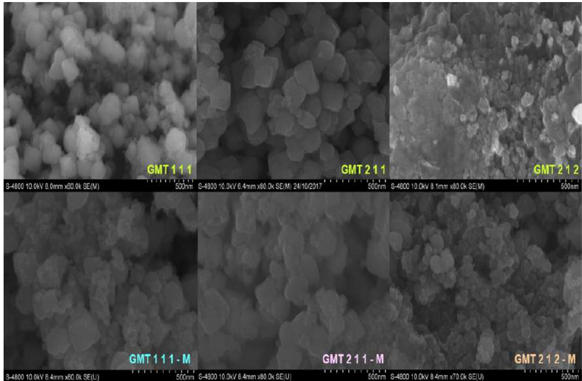
Hình 3.32. Ảnh SEM của các mẫu vật liệu GMT ( bên trên ) và GMT-M ( bên dưới ). Các mẫu đều có tỷ lệ các thành phần tương ứng như nhau
