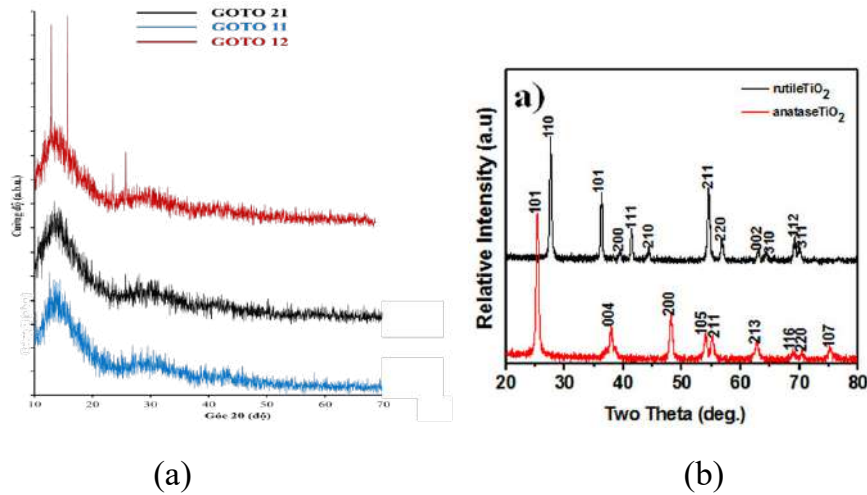
Hình 3.17. Giản đồ XRD của các mẫu GO- \text{TiO}_2 ở các tỷ lệ 11, 12, 21 (a); nano \text{TiO}_2 anatase và rutile tham khảo (b) [102].
