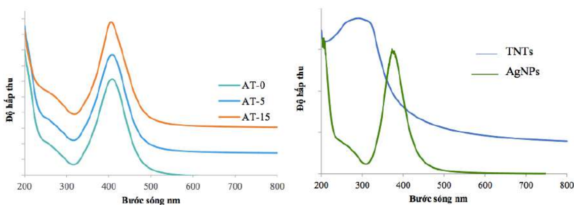
Hình 3.45. Phổ hấp thụ UV-Vis của mẫu AgNPs-TNTs ở hai liều xạ và hai nguyên liệu TNTs, AgNPs.
