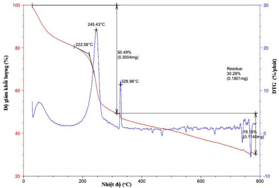
Hình 3.7. Giảm đồ TGA của sản phẩm GO.
