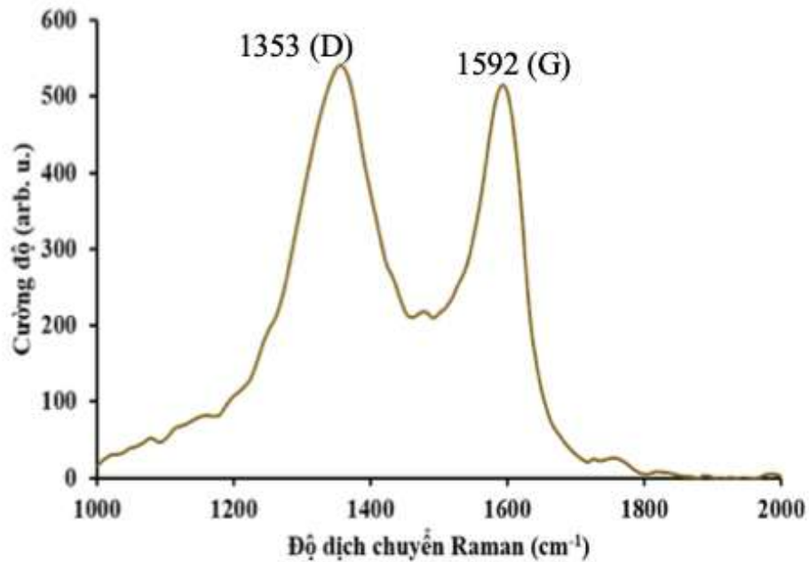
Hình 3.4. Phổ Raman của sản phẩm GO
