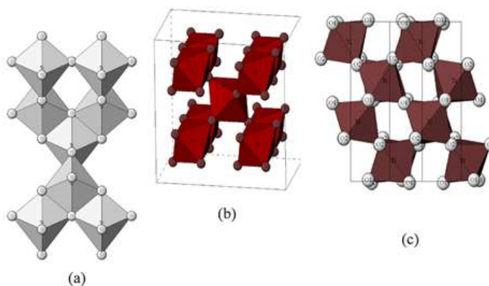
Hình 1.4. Cấu trúc tinh thể của nano \text{TiO}_2 a) pha anatase (quadratic), b) pha rutile (quadratic), c) pha brookite (orthorhombic) [18].
