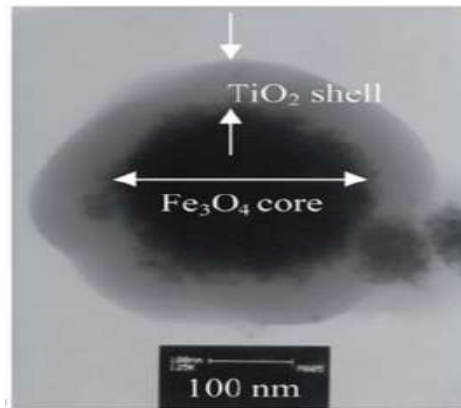
Hình 1.11. Ảnh TEM của vật liệu \text{Fe}_3\text{O}_4@\text{TiO}_2 [40].
