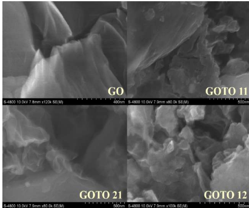
Hình 3.19. Ảnh SEM (từ trái qua phải) của GO và các mẫu GO-TiO 2 ở các tỷ lệ 11, 21, 12 (ký hiệu lần lượt GOTO11; GOTO21; GOTO12).
