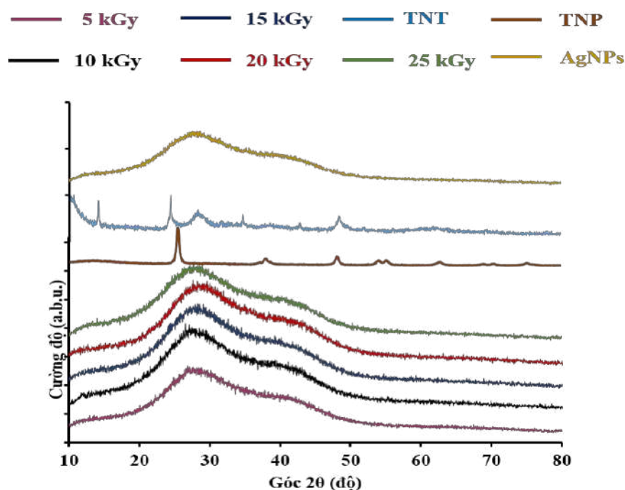
Hình 3.59. Giảm độ nhiễu xạ tia X của các mẫu vật liệu GO-AgNPs-TNTs với các liều chiếu xạ 5 kGy, 10 kGy, 15 kGy, 20 kGy và 25 kGy và vật liệu \text{TiO}_2 nano ống sau chiếu xạ, \text{TiO}_2 nano bột ban đầu và dung dịch AgNPs sau chiếu xạ.
