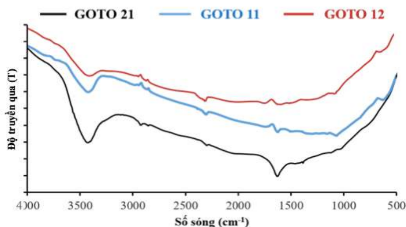
Hình 3.16. Phổ FTIR của các mẫu GO- \text{TiO}_2 ở các tỷ lệ 11, 12, 21.
