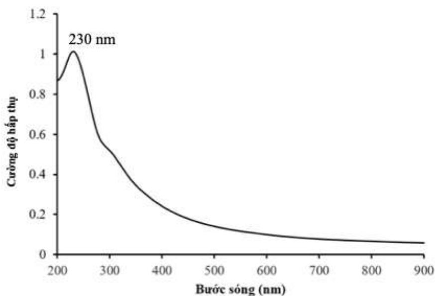
Hình 3.3. Phổ UV-Vis của sản phẩm GO.
