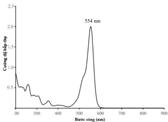
Hình 2.4. Phổ hấp thu UV-Vis của dung dịch RhB 10 ppm.
