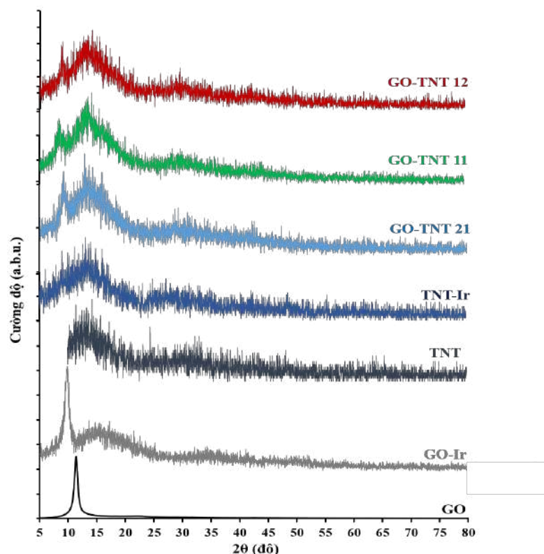
Hình 3.49. Giản đồ XRD của các mẫu vật liệu GO-TNTs 11; GO-TNTs 21; GO-TNTs 12 so sánh với các nguyên liệu GO, TNTs trước chiếu xạ và GO-Ir, TNTs-Ir sau khi chiếu xạ.
