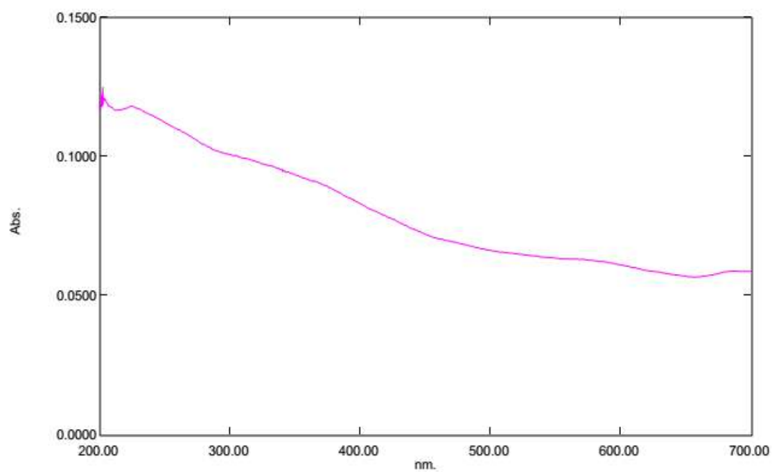
Phổ UV-Vis của GO-Fe 3 O 4 -TiO 2 (1:1:3)
