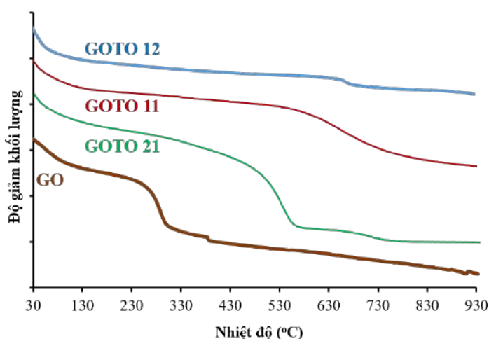
Hình 3.21. Giản đồ TGA của GO và các mẫu GO-TiO 2 ở các tỷ lệ 11, 21, 12 (ký hiệu lần lượt GOTO11; GOTO21; GOTO12).
