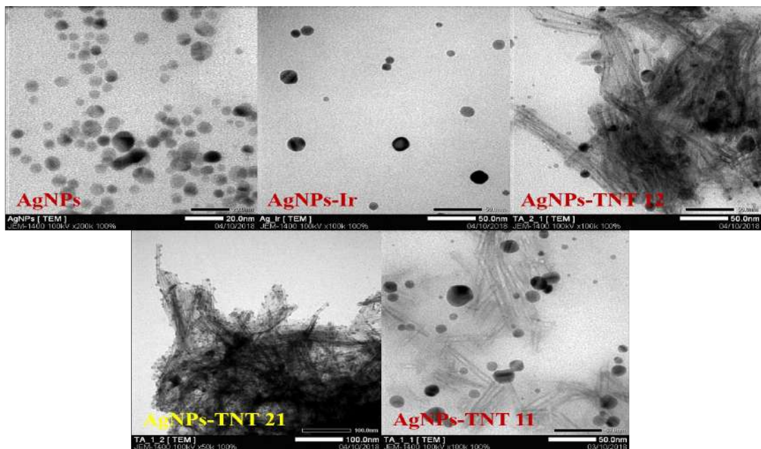
Hình 3.44. Ảnh TEM của các mẫu vật liệu AgNPs-TNTs 11; AgNPs-TNTs 21; AgNPs-TNTs 12 so sánh với các nguyên liệu AgNPs trước chiếu xạ và AgNPs-Ir sau khi chiếu xạ.
