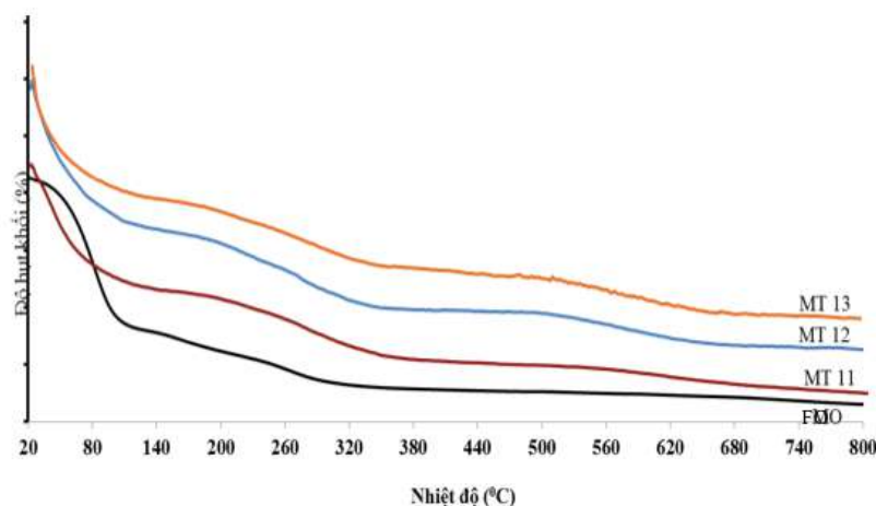
Hình 3.13. Giảm đồ phân tích nhiệt trọng lượng của Fe 3 O 4 và các vật liệu MT@ ở các tỷ lệ 1:1, 1:2, 1:3.
