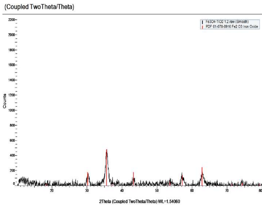
Phổ XRD của GO-Fe 3 O 4 @TiO 2
