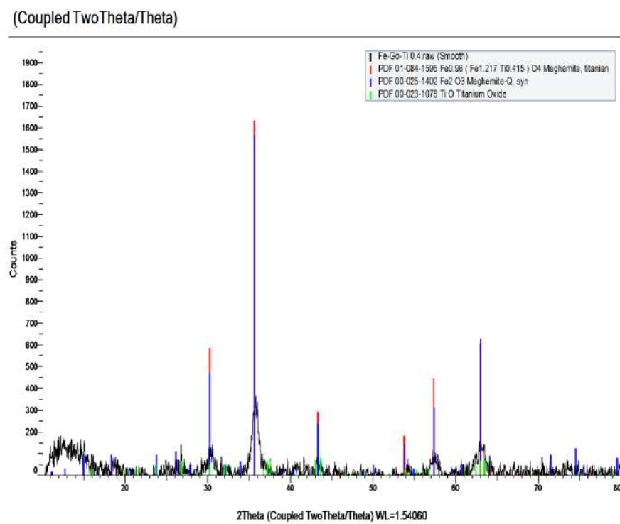
Phổ XRD của GO-Fe 3 O 4 @TiO 2
