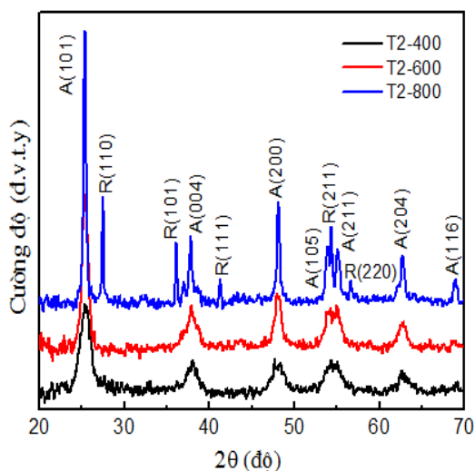
Hình 3.1. Giản đồ nhiễu xạ tia X (XRD) của các mẫu \text{TiO}_2 được tổng hợp trong môi trường có pH = 2 và nung ở các nhiệt độ 400 °C, 600 °C, 800 °C.
