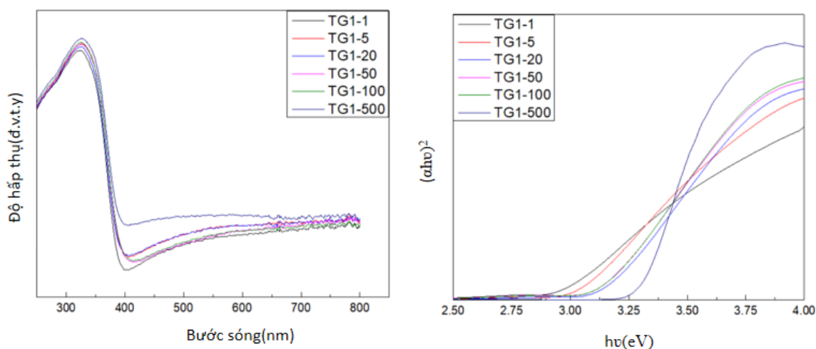
Hình 4.10. Phổ hấp thụ và năng lượng của các tổ hợp \text{TiO}_2/\text{GQDs} với tỉ lệ khác nhau.
