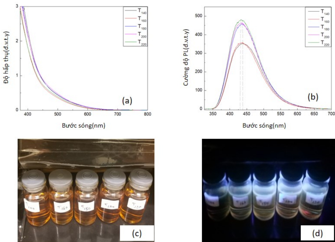
Hình 4.8. Phổ hấp thụ (a) và huỳnh quang (b) của GQDs tại các nhiệt độ khác nhau; GQDs được quan sát bằng mắt thường (c) và được chiếu bằng tia tử ngoại (d).
