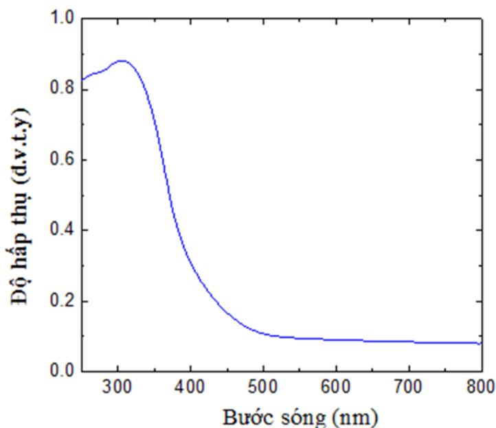
Hình 1.3. Phổ hấp thụ của tinh thể anatase tinh khiết [7].
