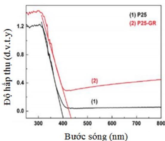
Hình 1.15. Phổ hấp thụ của vật liệu P25, P25-GR [56].
