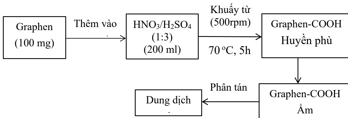
Hình 2.4. Sơ đồ quy trình biến tính graphen.
