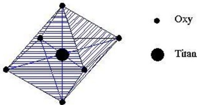
Hình 1.1. Cấu trúc bát diện \text{TiO}_6 [4].
