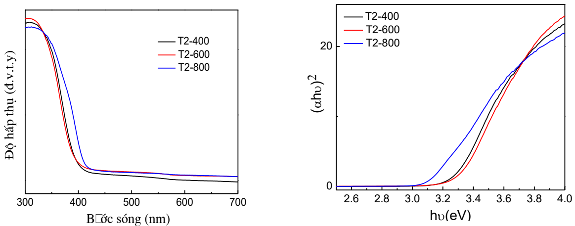
Hình 3.6. Phổ hấp thụ của các mẫu \text{TiO}_2 (a) theo bước sóng và (b) theo năng lượng.
