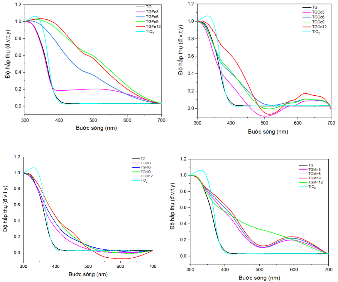
Hình 4.21. Phổ hấp thụ của hệ vật liệu: (a) \text{TiO}_2/\text{GQDs}/\text{Fe} , (b) \text{TiO}_2/\text{GQDs}/\text{Co} , (c) \text{TiO}_2/\text{GQDs}/\text{Ni} , (d) \text{TiO}_2/\text{GQDs}/\text{Mn} .
