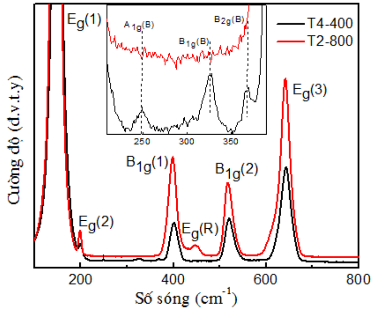
Hình 3.5. Phổ tán xạ Raman của mẫu T4-400 và T2-800.
