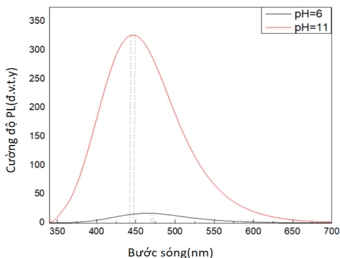
Hình 4.7. Phổ huỳnh quang của GQDs tại pH = 6 và pH = 11 (bước sóng kích thích 365 nm).
