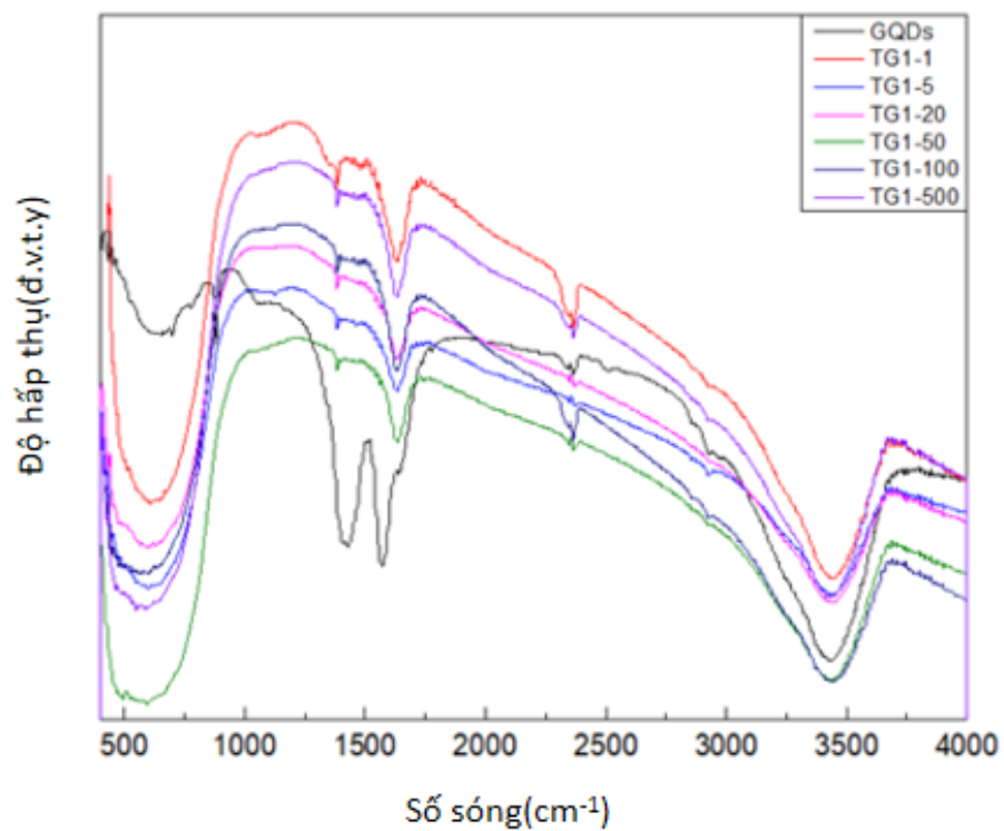
Hình 4.12. Phổ FTIR của GQDs và các tổ hợp \text{TiO}_2/\text{GQDs} với tỉ lệ khác nhau.
