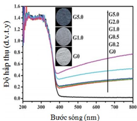
Hình 1.14. Phổ hấp thụ của hệ vật liệu \text{TiO}_2/\text{graphen} [57].
