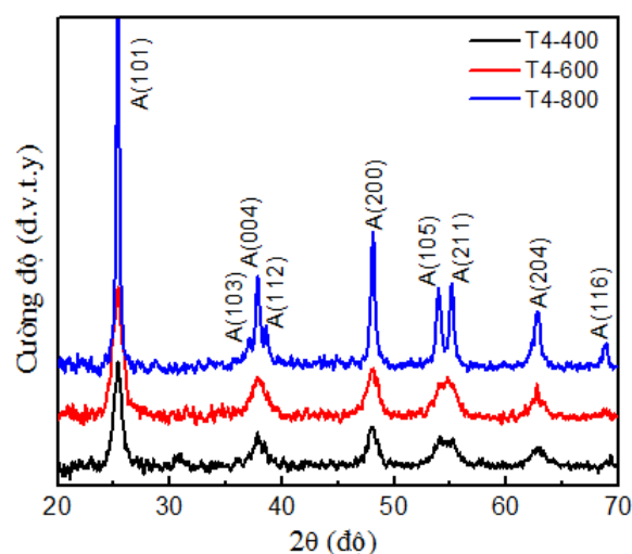
Hình 3.2. Giản đồ nhiễu xạ tia X (XRD) của các mẫu \text{TiO}_2 được tổng hợp trong môi trường có pH = 4 và nung ở các nhiệt độ 400 °C, 600 °C, 800 °C.
