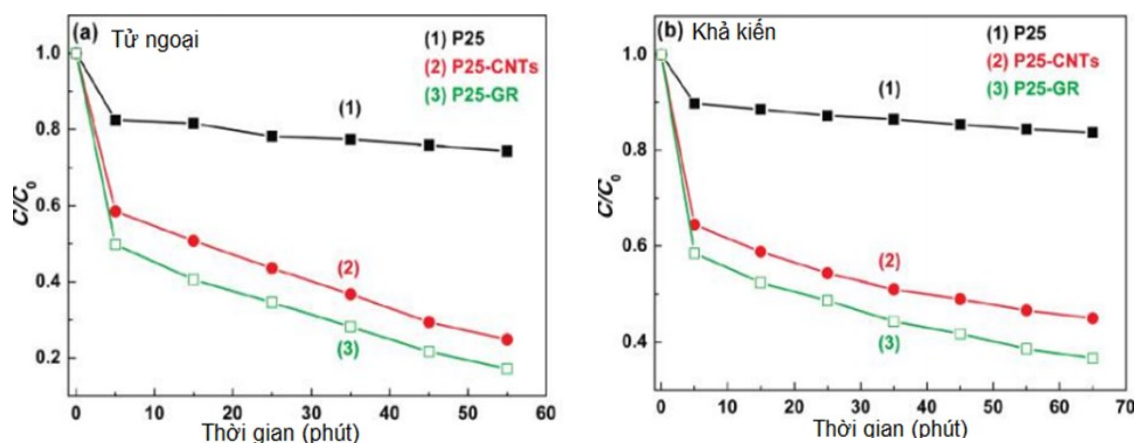
Hình 1.17. Hiệu suất phân hủy MB dưới bức xạ tử ngoại và nhìn thấy ( \lambda > 400 nm) của P25, P25-CNTs và P25-GR [56].
