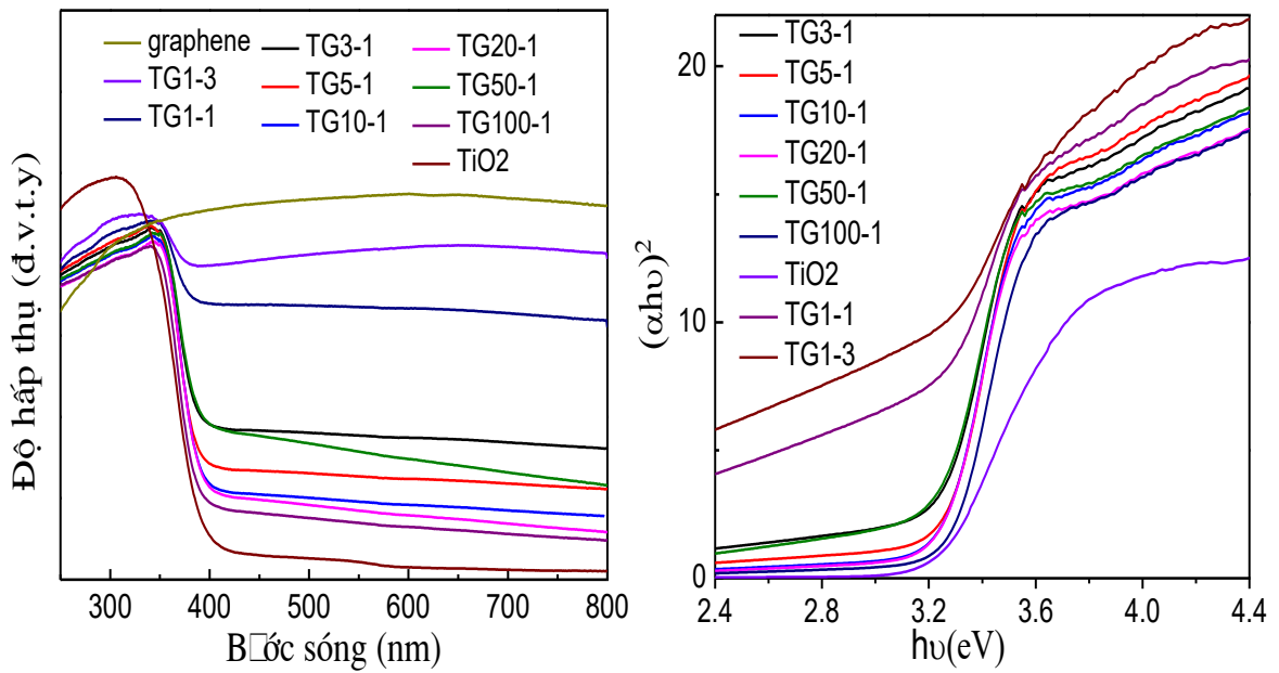
Hình 3.17. Phổ hấp thụ theo bước sóng và theo năng lượng của hệ mẫu \text{TiO}_2/\text{graphen} .
