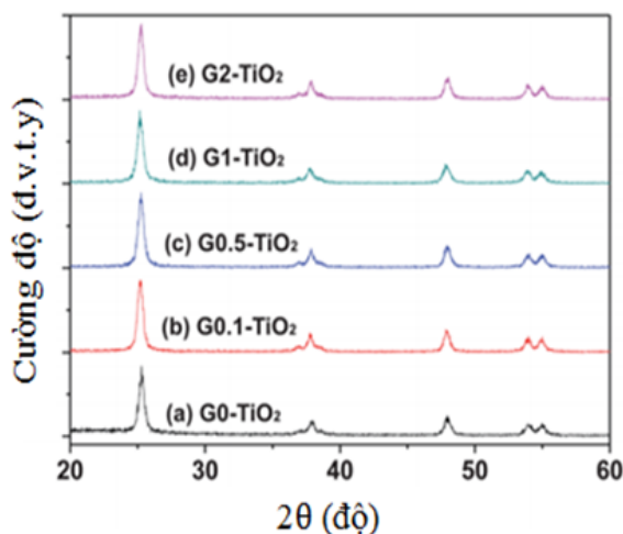
Hình 1.9. Giản đồ nhiễu xạ tia X của hệ vật liệu Gx-TiO 2 [70].
