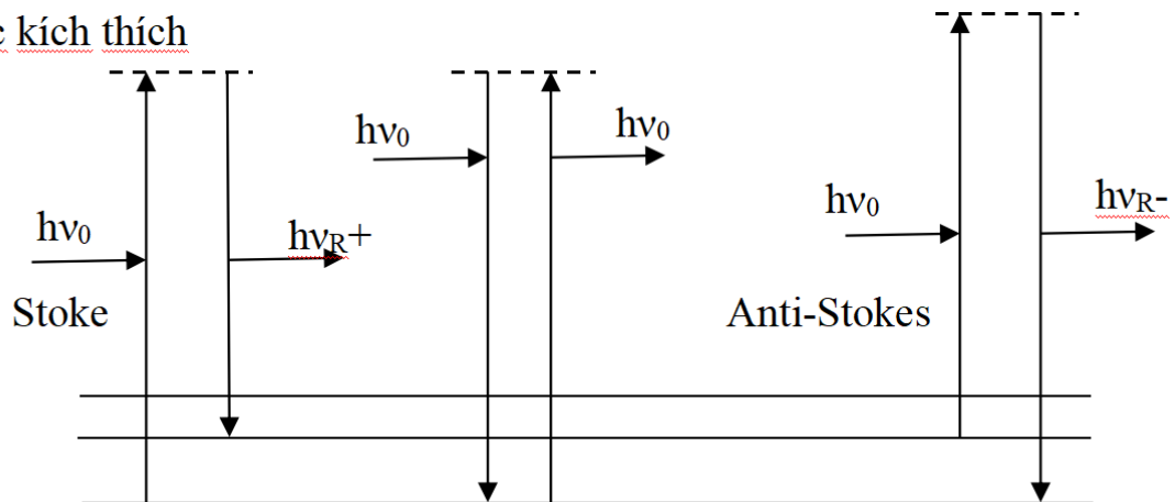
Hình 2.10. Sơ đồ cơ chế của tán xạ Raman.
