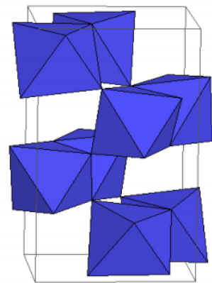
Brookite
