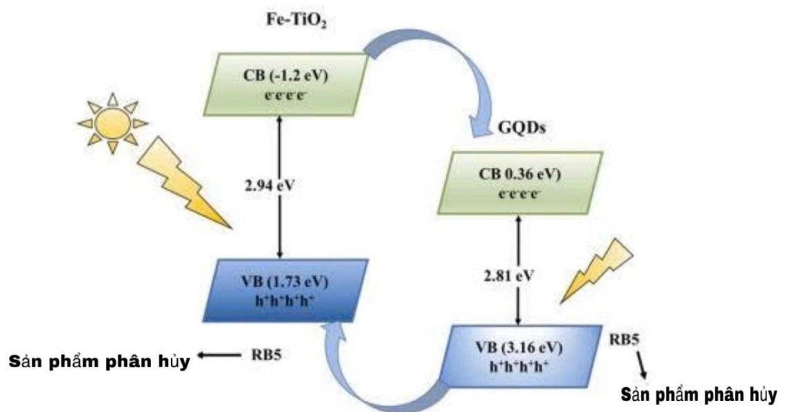
Hình 4.23. Cơ chế chuyển điện tích của hệ vật liệu \text{TiO}_2/\text{GQDs}/\text{Fe} trong quá trình phân hủy thuốc nhuộm RB5 dưới ánh sáng khả kiến [109].
