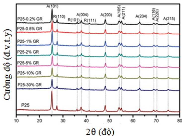
Hình 1.11. Giản đồ nhiễu xạ tia X của hệ vật liệu P25-RG [62].
