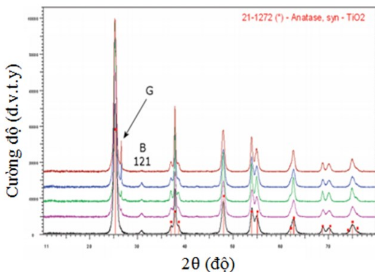
Hình 1.12. Giản đồ nhiễu xạ tia X của hệ vật liệu P25-RG [73].
