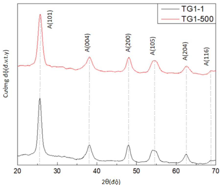
Hình 4.13. Giản đồ nhiễu xạ tia X của các mẫu tổ hợp \text{TiO}_2/\text{GQDs} .
