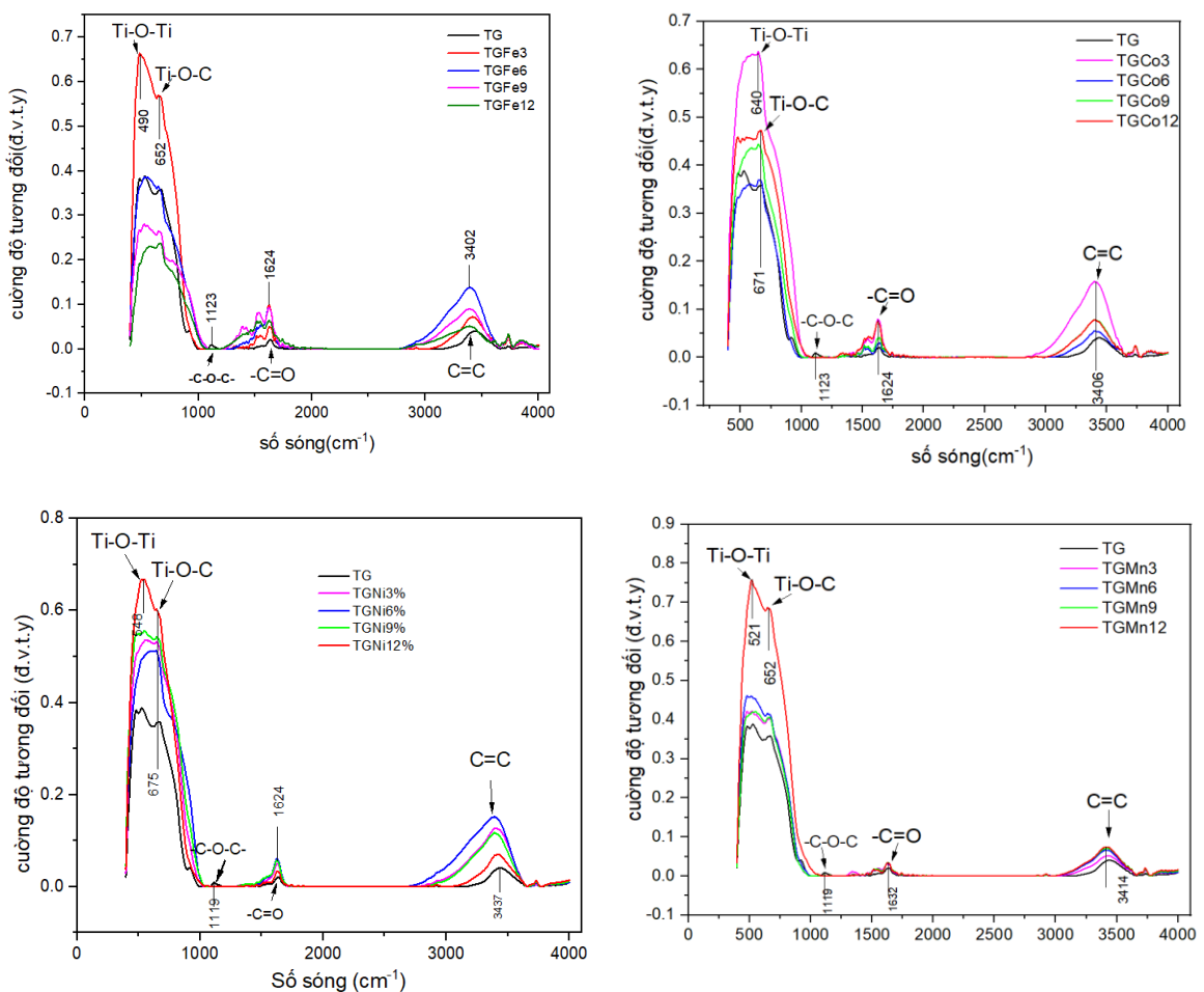
Hình 4.20. Phổ FTIR của hệ vật liệu: (a) \text{TiO}_2/\text{GQDs}/\text{Fe} , (b) \text{TiO}_2/\text{GQDs}/\text{Co} , (c) \text{TiO}_2/\text{GQDs}/\text{Ni} , (d) \text{TiO}_2/\text{GQDs}/\text{Mn} .
