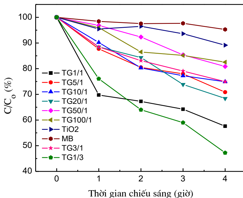
Hình 3.20. Tổng hợp kết quả xử lý MB của các mẫu theo thời gian chiếu sáng.
