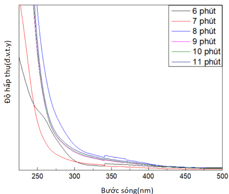
Hình 4.1. Phổ hấp thụ UV–Vis của GQDs tại công suất 500 W và thời gian khác nhau của lò vi sóng.
