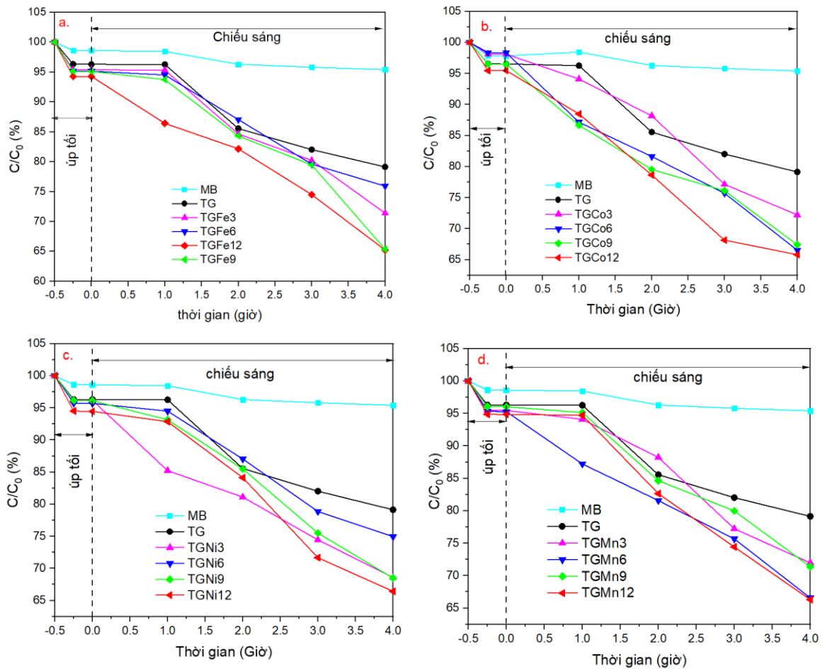
Hình 4.24. Tổng hợp kết quả xử lý MB của các mẫu theo thời gian chiếu sáng.
