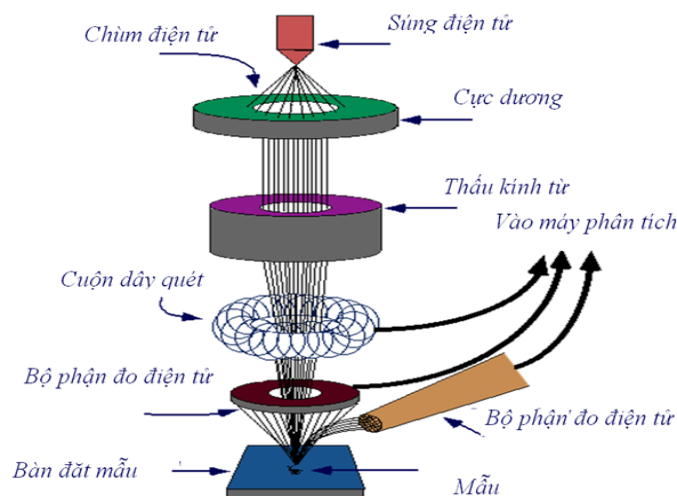
Hình 2.11. Sơ đồ nguyên tắc hoạt động của kính hiển vi điện tử quét.
