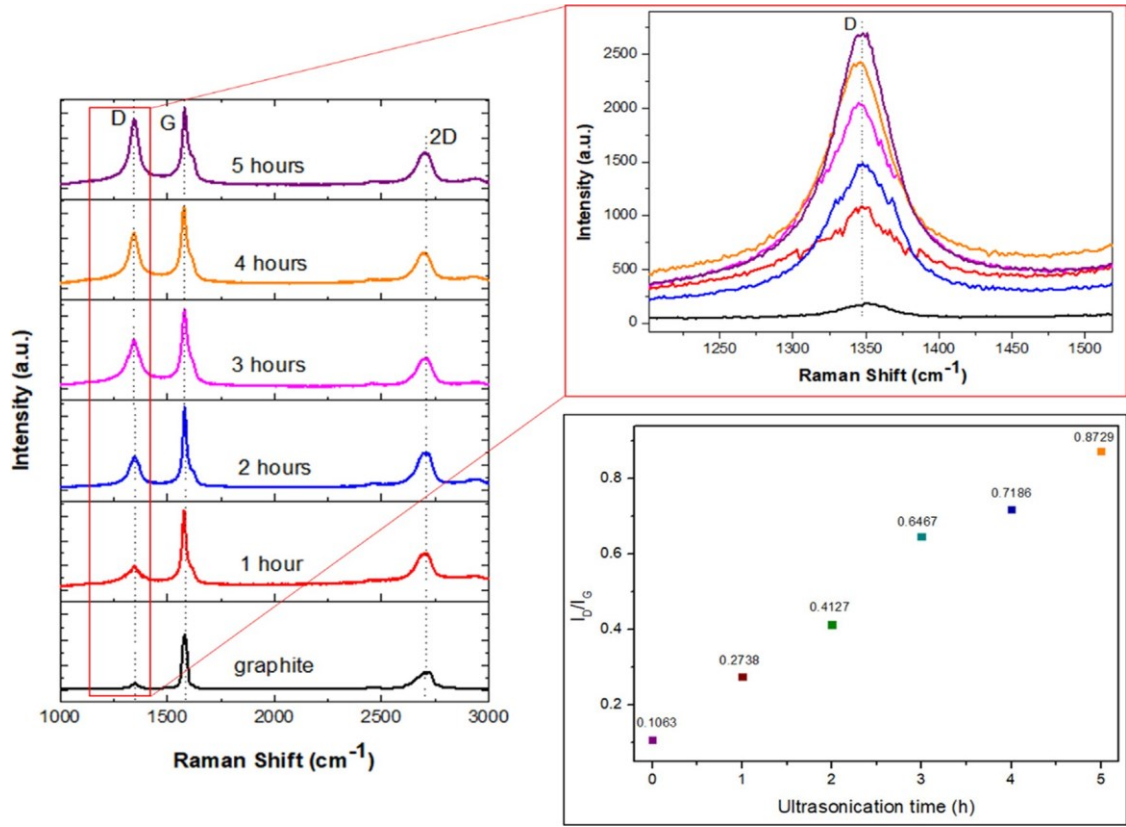
Hình 3.9. Phổ Raman của graphit với các thời gian siêu âm khác nhau.
