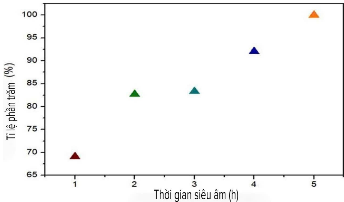
Hình 3.11. Phân bố kích thước (100–500 nm) của graphen tại các thời gian siêu âm khác nhau.
