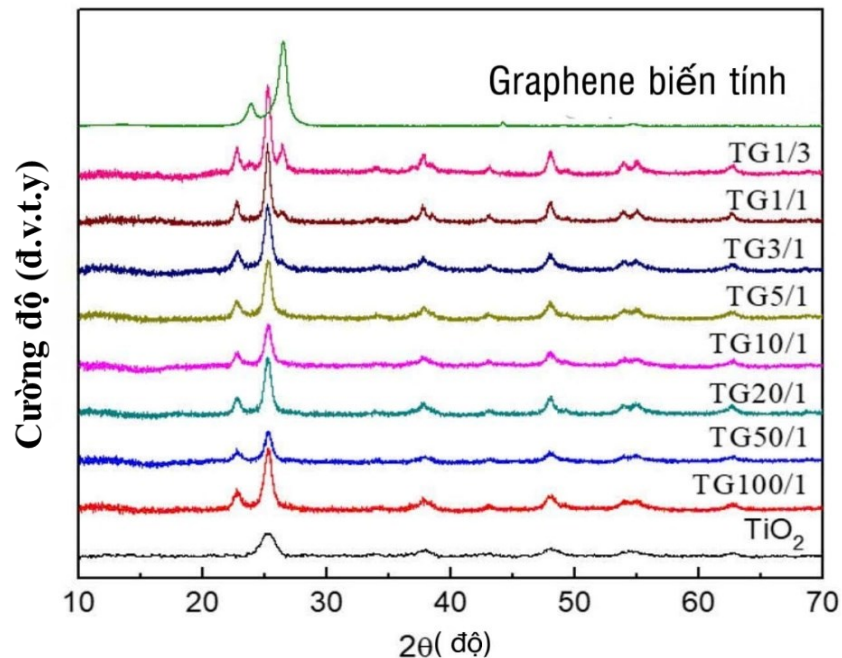
Hình 3.14. Giản đồ nhiễu xạ tia X (XRD) của tổ hợp các mẫu \text{TiO}_2 /graphen.
