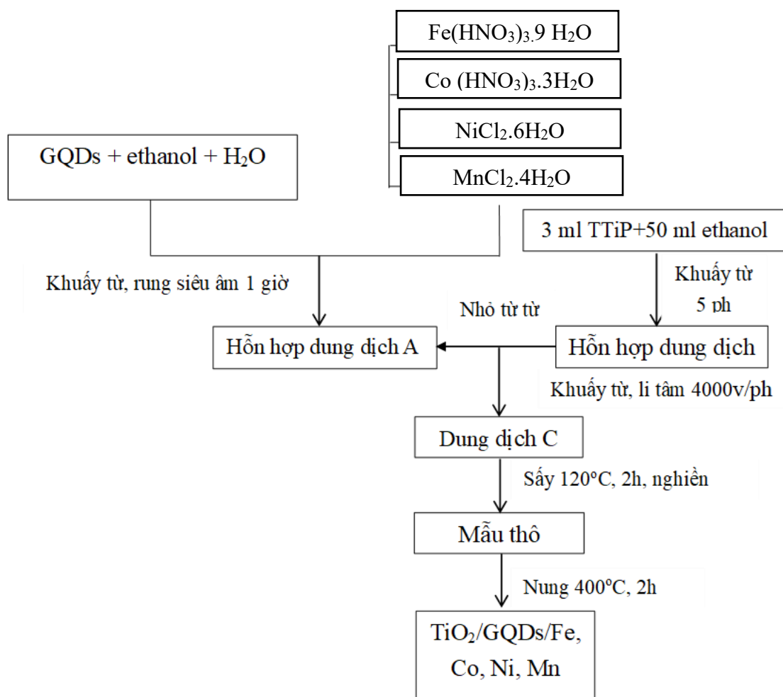
Hình 2.8. Sơ đồ quy trình chế tạo vật liệu tổ hợp \text{TiO}_2/\text{GQDs} (1:20) pha tạp Fe, Co, Ni, Mn.
