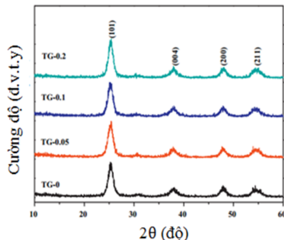
Hình 1.10. Giản đồ nhiễu xạ tia X của hệ vật liệu TG-x [71].
