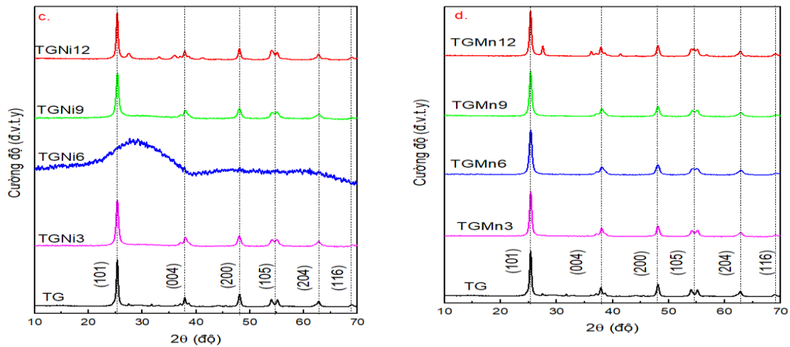
Hình 4.17. Giải đồ nhiễu xạ tia X của hệ vật liệu: (a) \text{TiO}_2/\text{GQDs}/\text{Fe} , (b) \text{TiO}_2/\text{GQDs}/\text{Co} , (c) \text{TiO}_2/\text{GQDs}/\text{Ni} , (d) \text{TiO}_2/\text{GQDs}/\text{Mn} .
