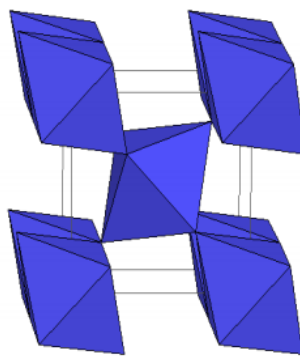
Rutile
