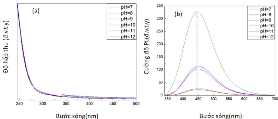
Hình 4.6. Phổ hấp thụ (a) và huỳnh quang (b) của GQDs trong môi trường bazơ.
