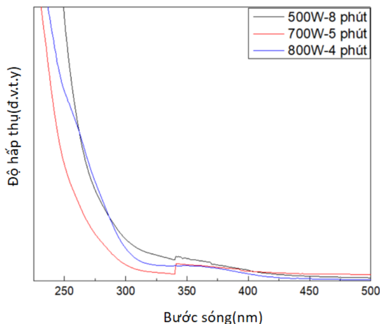
Hình 4.4. Phổ hấp thụ UV–Vis của GQDs tại công suất và thời gian khác nhau của lò vi sóng.
