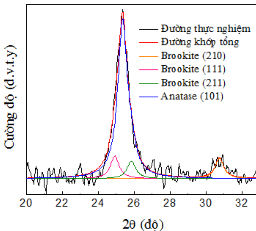
Hình 3.4. Khớp các đỉnh nhiễu xạ anatase (101) và đỉnh brookite (211) bằng hàm Pseudo Voigt của mẫu T4-400 khi tính đến đỉnh brookite ở vị trí 25,36° và 25,71° gần với đỉnh (101) của pha anatase.
