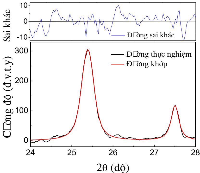
Hình 3.3. Khớp các đỉnh nhiễu xạ anatase (101), rutile (110) bằng hàm Pseudo Voigt của mẫu T2-800.
