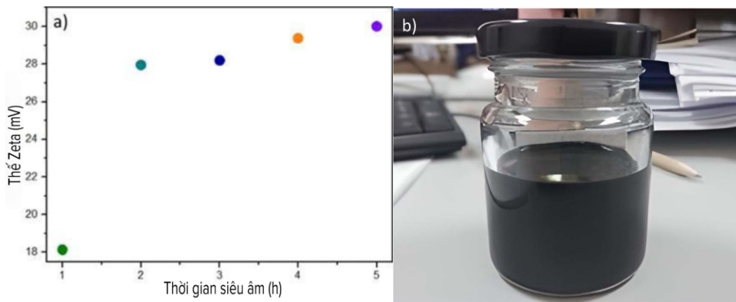
Hình 3.12. (a) Kết quả đo thế zeta tại các thời gian siêu âm khác nhau; (b) Quan sát bằng mắt thường mẫu graphene sau 5 giờ siêu âm được lưu trữ sau 5 tháng.
