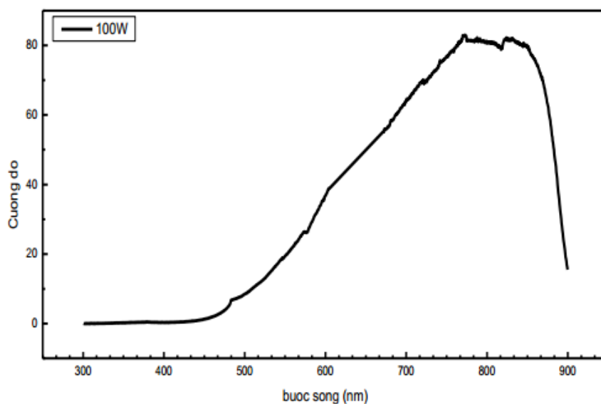
Hình 3.19. Phổ phát xạ của đèn dây tóc.
