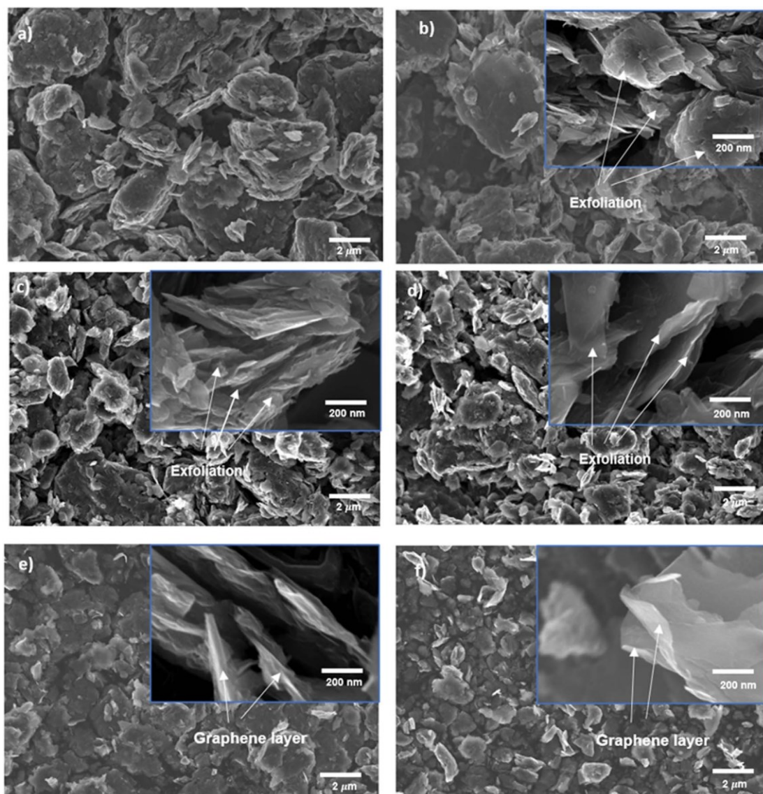
Hình 3.8. Kết quả ảnh FESEM của graphen với các thời gian rung siêu âm khác nhau (a) graphit ban đầu (chưa xử lý), (b–f) Sau khi siêu âm lần lượt trong 1, 2, 3, 4 và 5 giờ.
