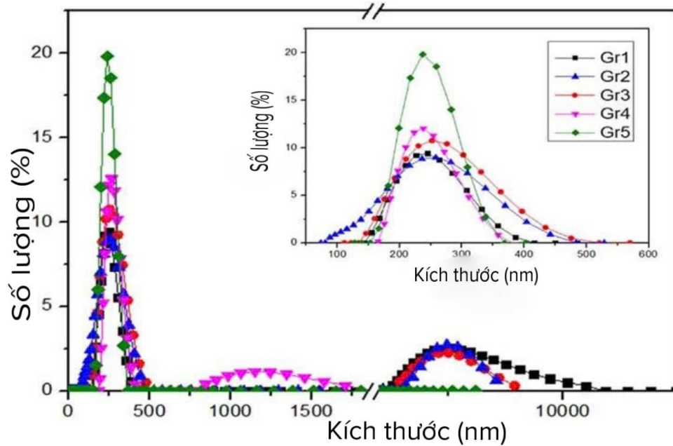
Hình 3.10. Phân bố kích thước của graphene tại các thời gian siêu âm khác nhau.
