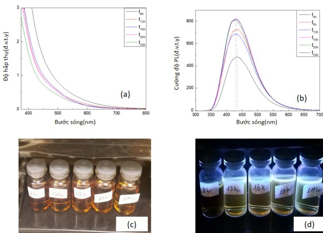
Hình 4.9. Phổ hấp thụ (a) và huỳnh quang (b) của GQDs tại các thời gian khác nhau; GQDs được quan sát bằng mắt thường (c) và được chiếu bằng tia tử ngoại (d).
