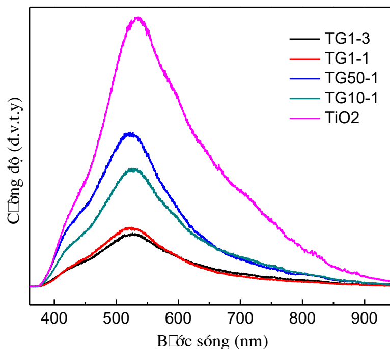
Hình 3.18. Phổ huỳnh quang của vật liệu \text{TiO}_2 và \text{TiO}_2/\text{graphen} .
