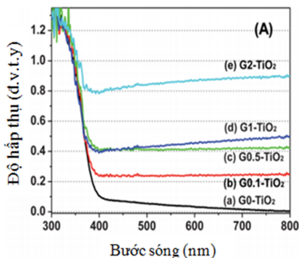
Hình 1.13. Phổ hấp thụ của hệ vật liệu \text{Gx-TiO}_2 [71].
