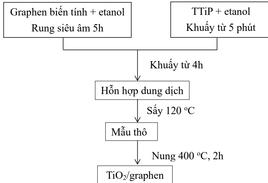
Hình 2.5. Sơ đồ quy trình chế tạo vật liệu tổ hợp \text{TiO}_2/\text{graphen} .
