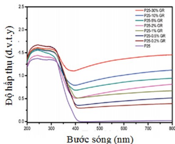
Hình 1.16. Phổ hấp thụ của hệ vật liệu P25-GR [62].
