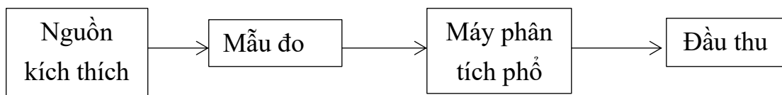
Hình 2.12. Sơ đồ khối của hệ đo huỳnh quang.
