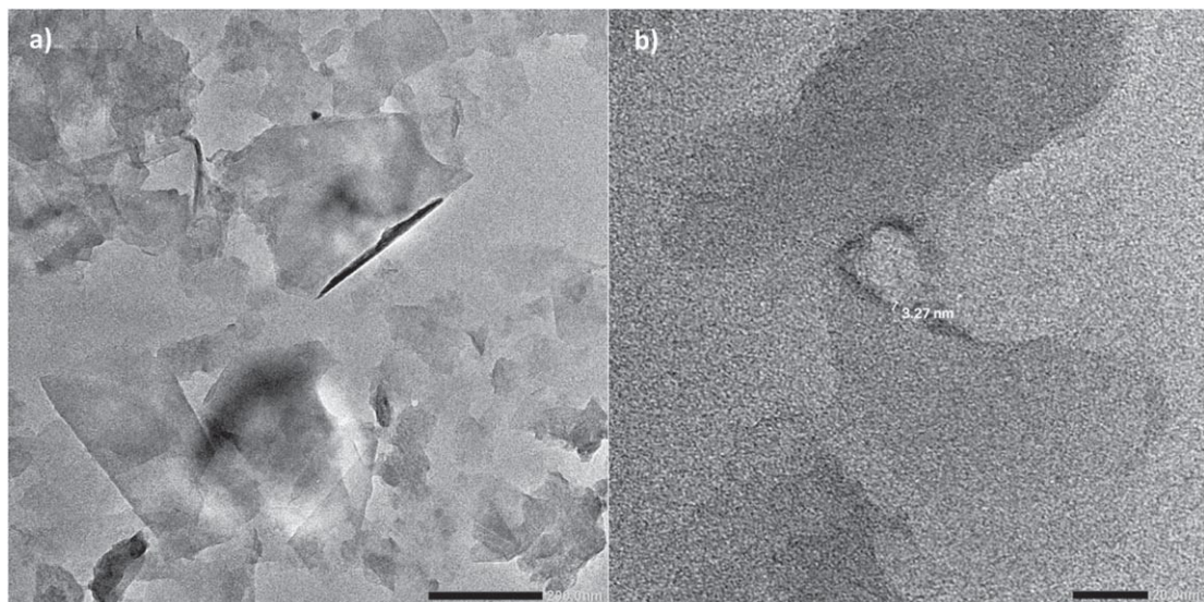
Hình 3.13. Kết quả ảnh TEM của graphene sau 5 giờ siêu âm, với độ phân giải 200 nm (bên trái) và 20 nm (bên phải).
