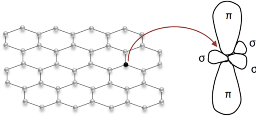
Hình 1.6. Cấu trúc của graphen [14].
