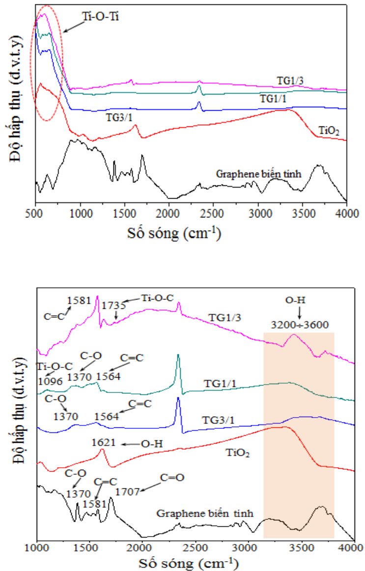
Hình 3.16. Phổ hồng ngoại biến đổi Fourier (FTIR) của các mẫu \text{TiO}_2 , graphen biến tính, và tổ hợp \text{TiO}_2 /graphen được ghi nhận trong hai dải bước sóng: (a) từ 500–4000 nm, và (b) trong khoảng 1000–4000 nm.
