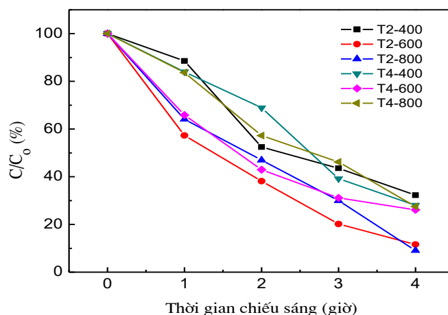
Hình 3.7. Kết quả xử lý xanh methylen theo thời gian của các mẫu \text{TiO}_2 .
