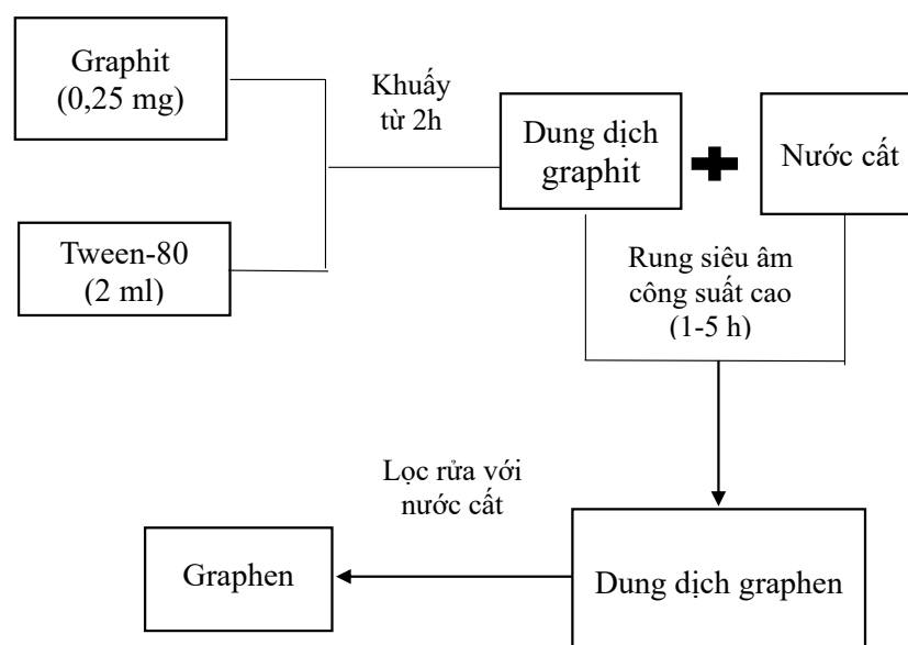
Hình 2.3. Quy trình chế tạo graphene từ graphite bằng phương pháp siêu âm mật độ công suất lớn.
