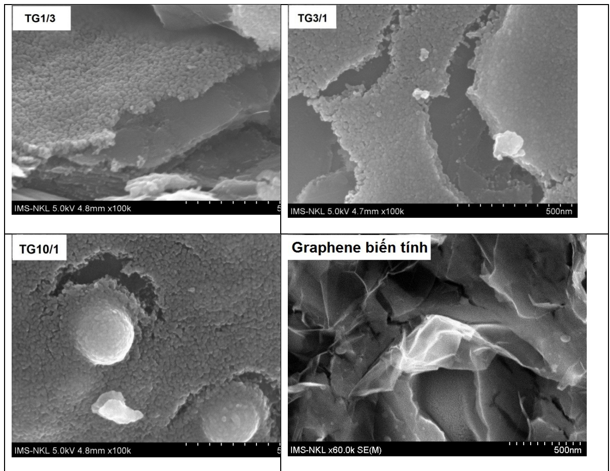
Hình 3.15. Ảnh hiển vi điện tử quét SEM của mẫu TG1/3, TG3/1, TG10/1, TG100/1 và của graphene.
