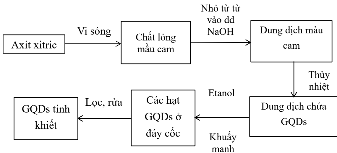
Hình 2.6. Sơ đồ quy trình chế tạo GQDs.
