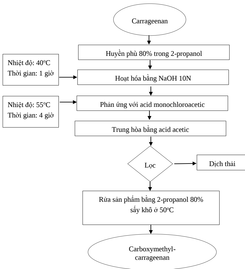
Hình 2.8. Sơ đồ quy trình tổng hợp carboxymethyl-carrageenan.
