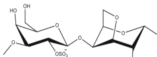
\theta -carrageenan G2S - DA2S
