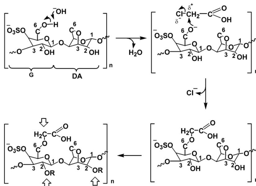
Hình 2.7. Tổng hợp carboxymethyl \kappa -carrageenan, DA là 3,6-anhydro- \alpha -D-galactopyranose; G là \beta -D-galactopyranose-4-sulfate. Các số từ 1 đến 6 hiển thị số carbon. R: CH 2 COOH hoặc H; n: số đơn vị lặp lại; mũi tên: các vị trí có thể có sự carboxymethyl hóa.
