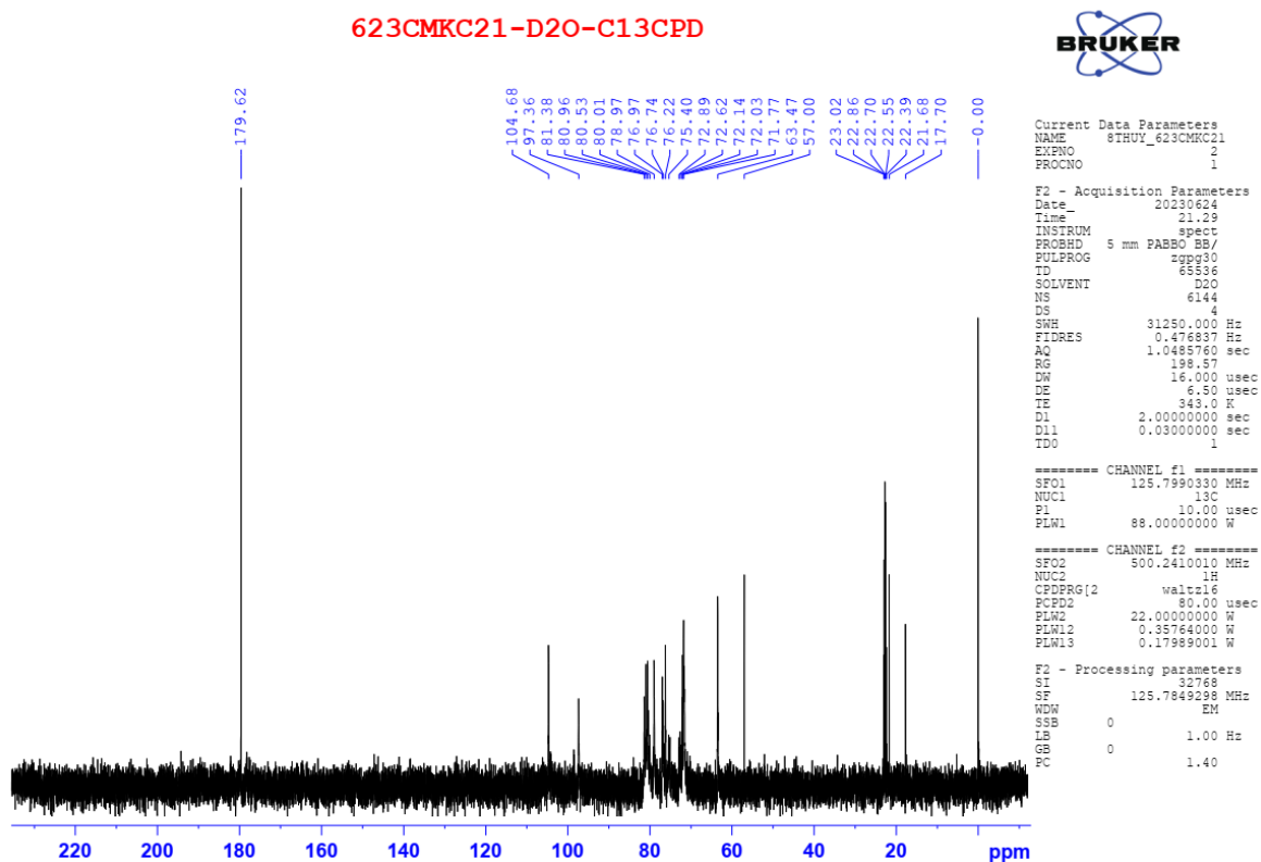
Phụ lục 14. Phổ NMR ^1\text{H} và ^{13}\text{C} của CMKC-2/1.
