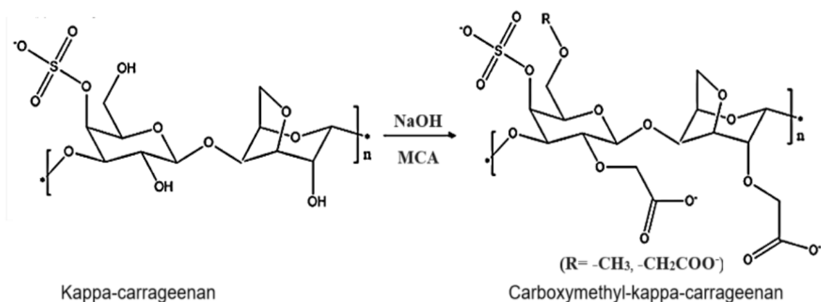
Hình 3.17. Tổng hợp carboxymethyl-kappa-carrageenan.
