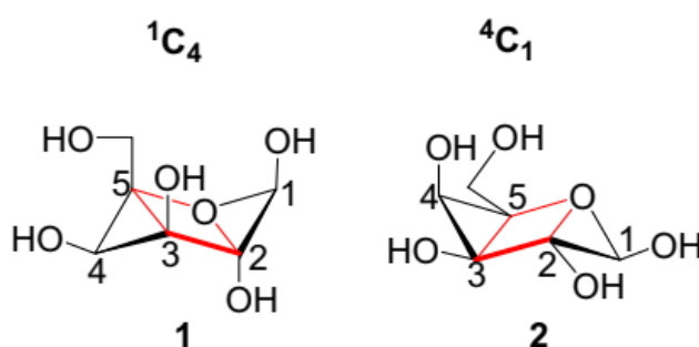
Hình 1.2. Mô tả cấu trúc {}^1C_4 và {}^4C_1 của \beta -D-galactopyranose. Cấu trúc được xác định bằng các chữ số chỉ các nguyên tử vòng nằm trên hoặc dưới một mặt phẳng chuẩn xác định (màu đỏ) chứa các nguyên tử C-2, C-3, C-5 và O. Trong cấu trúc 1, C-1 ở trên mặt phẳng và C-4 ở dưới và do đó, ký hiệu là {}^1C_4 , cấu trúc 2 là {}^4C_1 .
