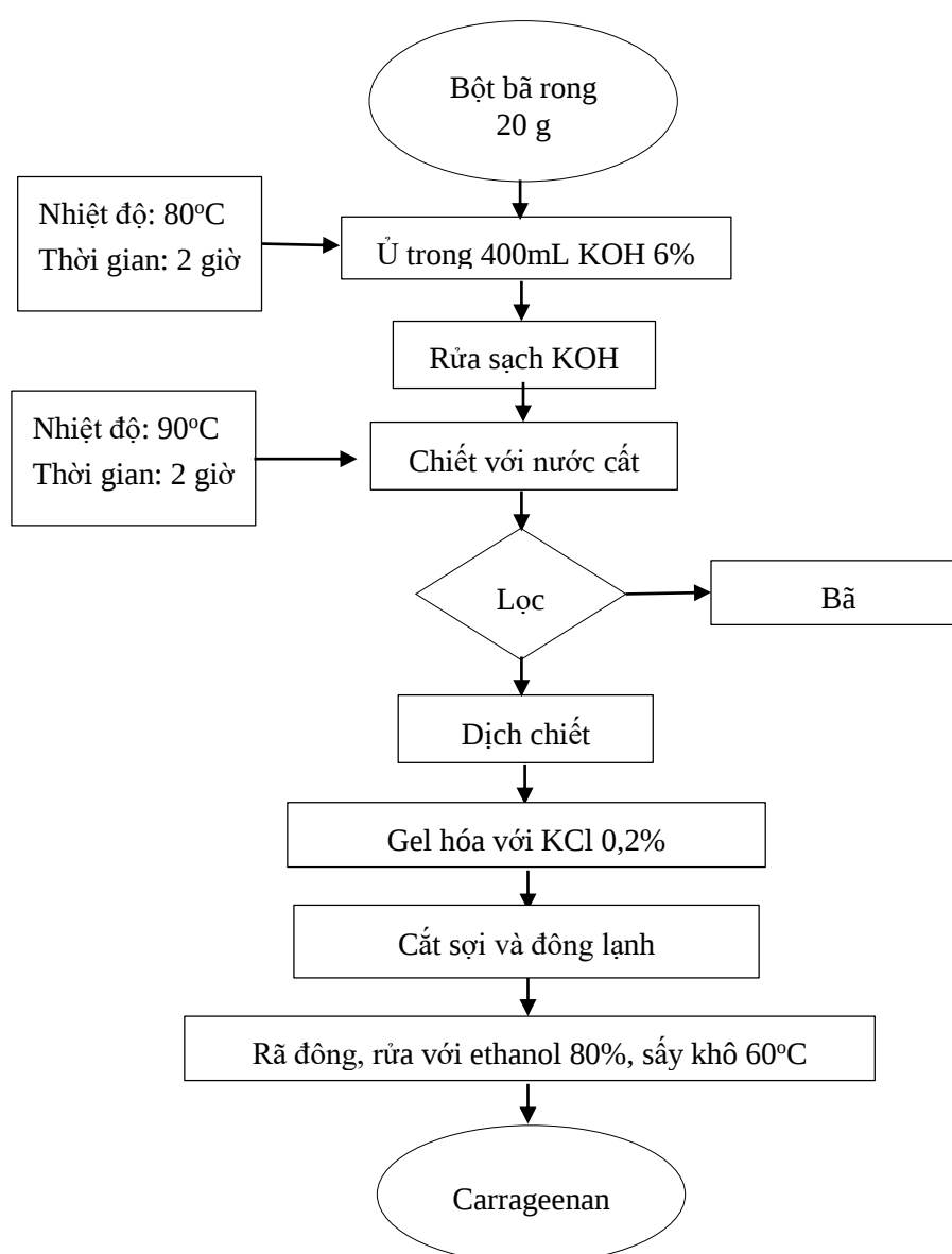
Hình 2.6. Sơ đồ quy trình chiết carrageenan từ bã rong xử lý kiềm.
