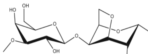
\alpha -carrageenan G - DA2S
