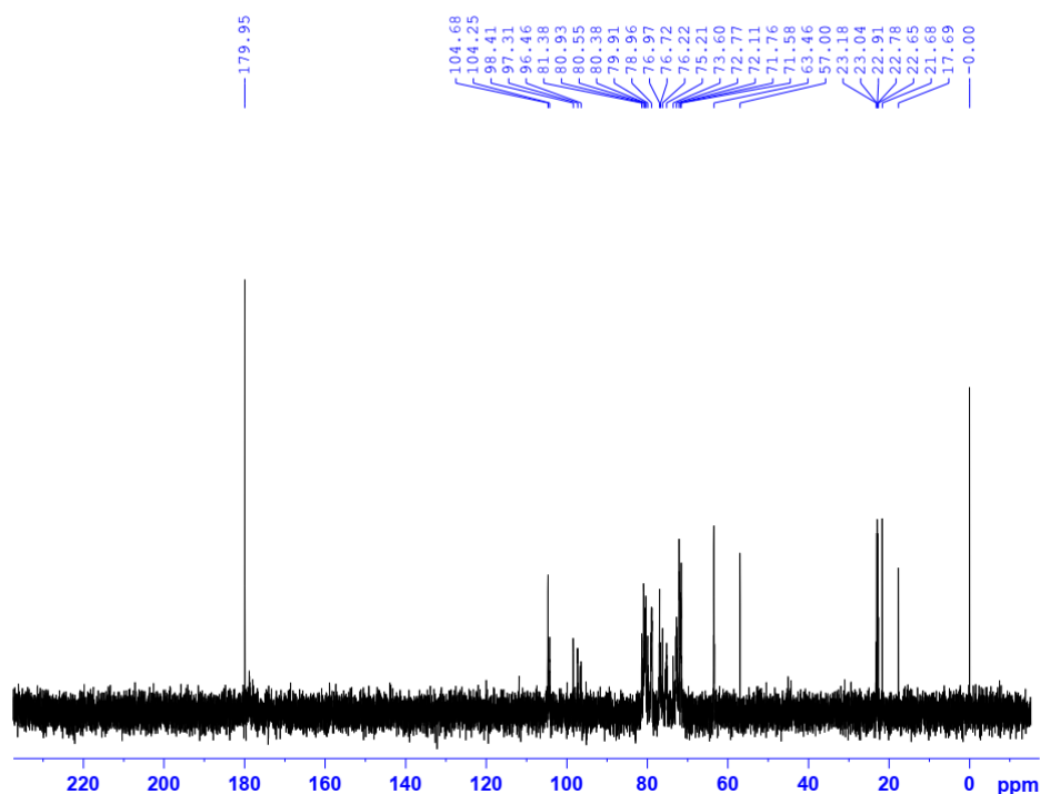
Phụ lục 15. Phổ NMR ^1\text{H} và ^{13}\text{C} của CMKC-3/1.
