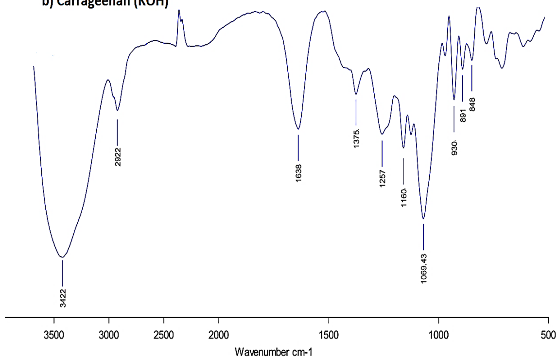
Hình 3.9. Phổ FT-IR của carrageenan từ rong B. gelatinus : a) carrageenan chiết tự nhiên, b) carrageenan chiết xử lý với dung dịch kiềm (KOH).
