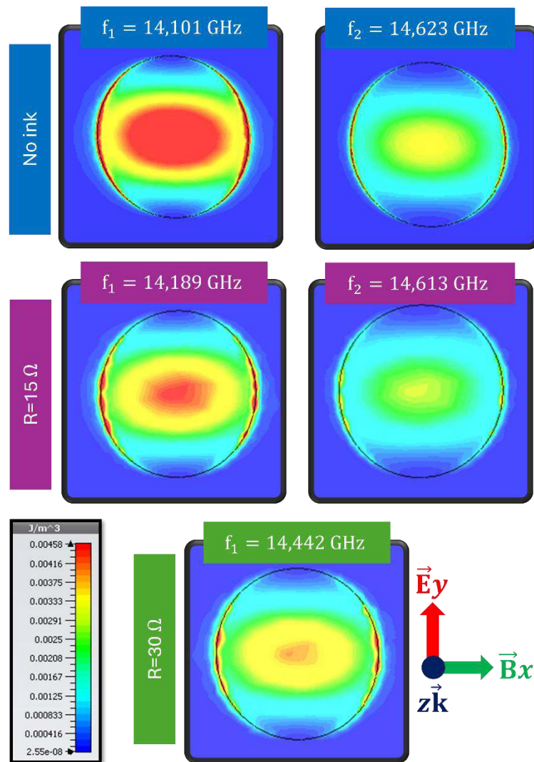
Hình 4.11. Mô phỏng phân bố từ trường tại các đỉnh không truyền qua của cấu trúc cặp đĩa hai lớp khi điện trở lớp mực dẫn thay đổi
