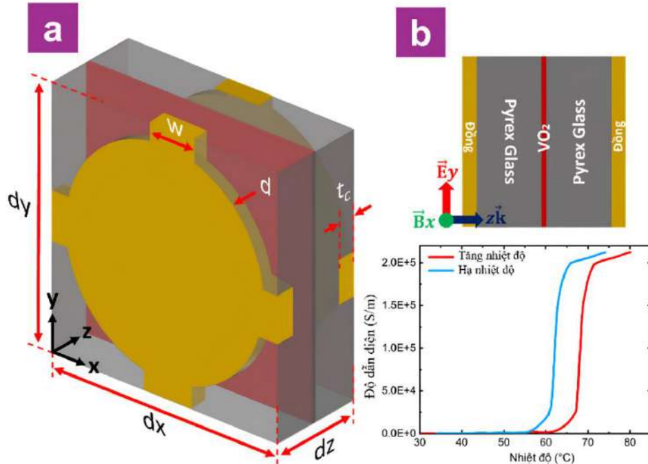
Hình 3.23. (a) Cấu trúc vật liệu biến hóa dạng lưới đĩa kim loại tích hợp \text{VO}_2 với các tham số cấu trúc tối ưu (b) Mặt cắt của cấu trúc vật liệu biến hóa dạng lưới đĩa kim loại và sự phụ thuộc của độ dẫn điện \text{VO}_2 theo nhiệt độ
