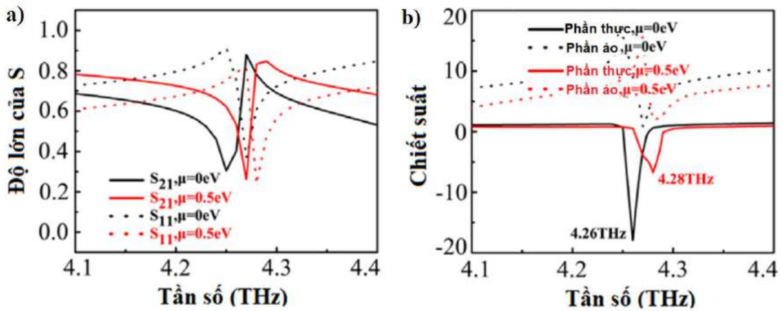
Hình 1.33. a) Giá trị của các tham số tán xạ S và b) tham số chiết suất của MM dưới hai thể hóa học khác nhau của graphene [68]
