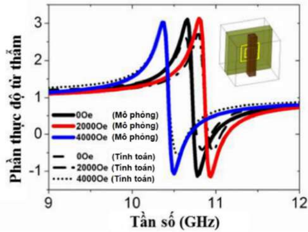
Hình 1.31. Kết quả mô phỏng độ từ thấm (đường liền nét) so sánh với kết quả tính toán theo công thức (2) (đường nét đứt) với các giá trị của từ trường ngoài: 0 Oe, 2000 Oe và 4000 Oe [19].
