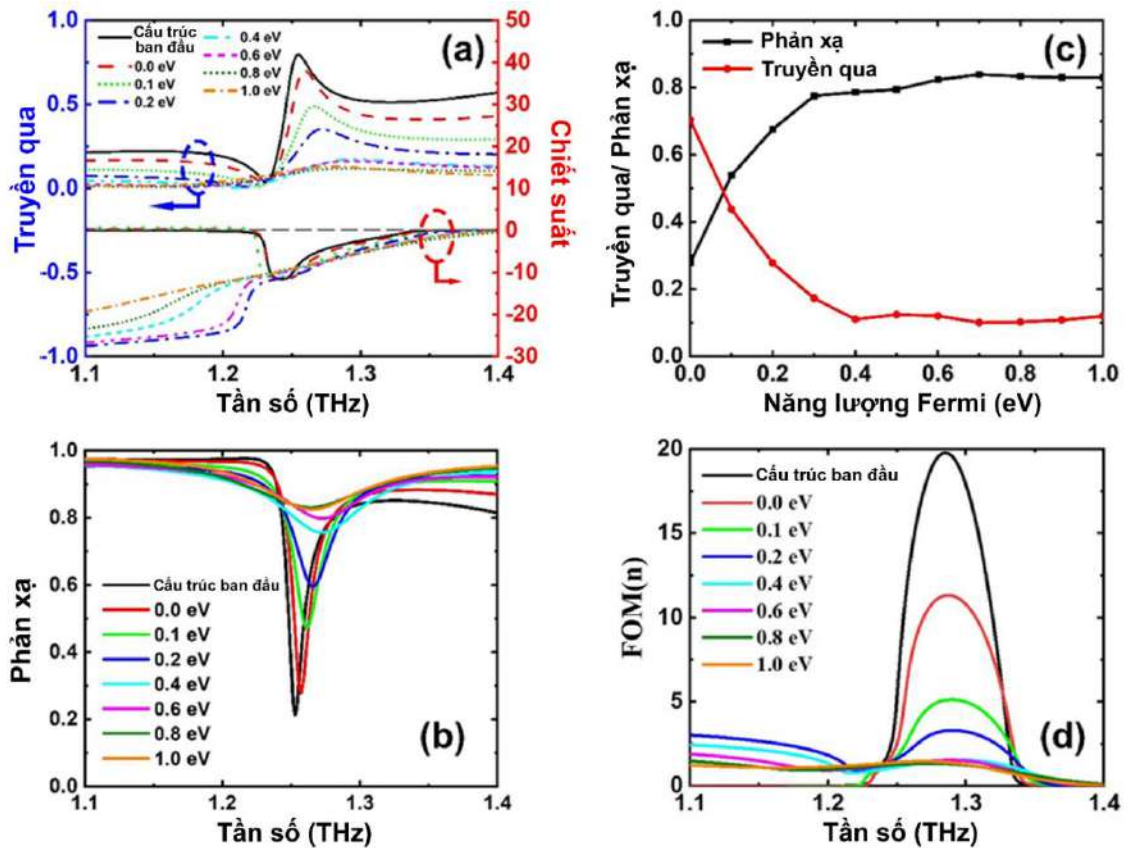
Hình 3.11. (a) Phổ truyền qua và phản xạ thực của chiết suất (b) phổ phản xạ (c) giá trị đỉnh truyền qua và phản xạ ở 1,25 THz và (d) hệ số phẩm chất (FOM) của chiết suất âm cho cấu trúc lưới đĩa kim loại và cấu trúc lưới đĩa kim loại tích hợp graphene tương ứng với các mức Fermi khác nhau.
