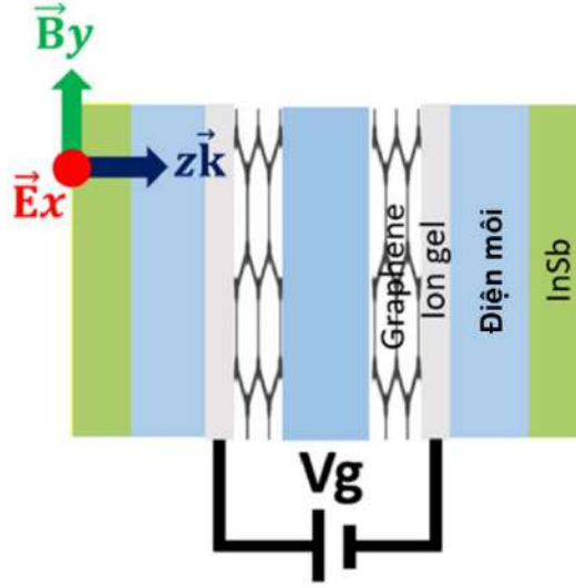
Hình 3.9. Mặt cắt của mẫu MM
