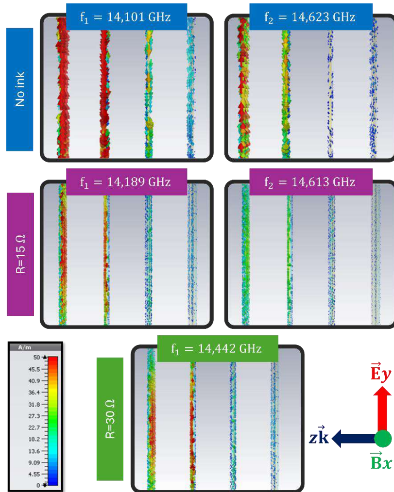
Hình 4.10. Phân bố dòng khi có mực dẫn tại các đỉnh không truyền qua khi điện trở lớp mực dẫn thay đổi
