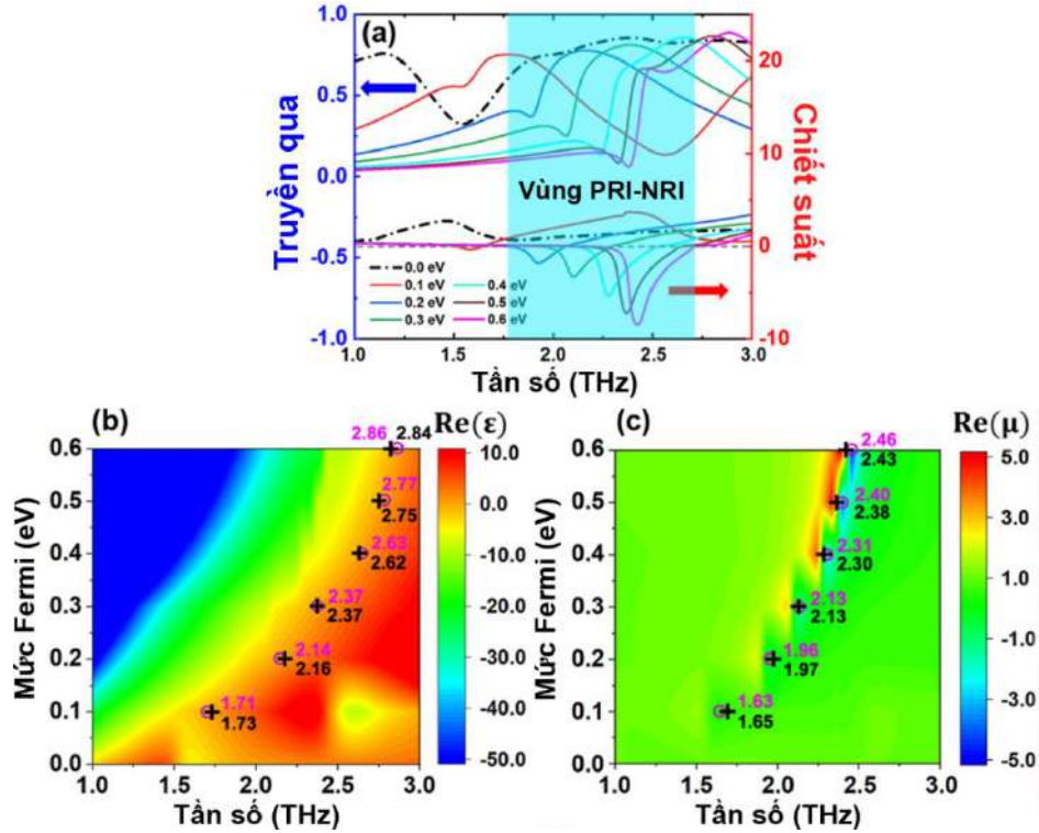
Hình 3.20. (a) Phổ truyền qua và phần thực của chiết suất [ Re(n) ] của MMHGC tương ứng với các mức Fermi khác nhau, phần thực của (b) hằng số điện môi và (c) độ từ thẩm của MMHGC tương ứng với các mức Fermi khác nhau. Ký hiệu 'o' đánh dấu bằng màu tím và ký hiệu '+' đánh dấu bằng màu đen chỉ ra các giá trị mô phỏng và tính toán của b và c, tương ứng.
