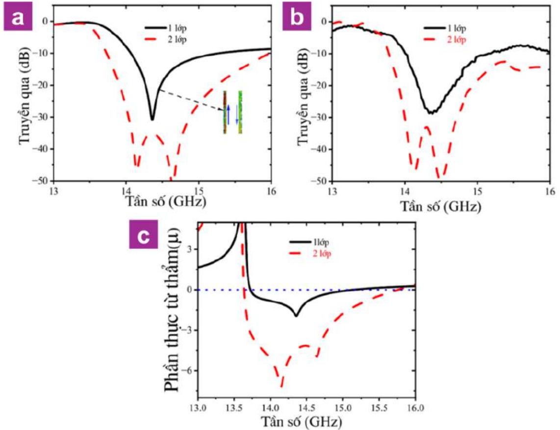
Hình 4.2. Phổ truyền qua a) mô phỏng, b) đo đạc và c) kết quả tính toán phần thực của độ từ thẩm cấu trúc cặp đĩa đề xuất 1 lớp và hai lớp
