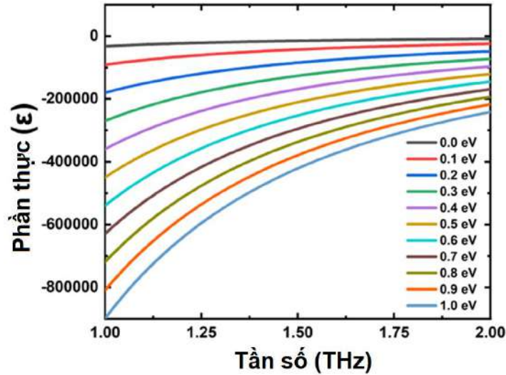
Hình 3.8. Phản thực của hằng số điện môi của graphene tương ứng với các thế hóa học từ 0,0 \text{ eV} đến 1,0 \text{ eV}
