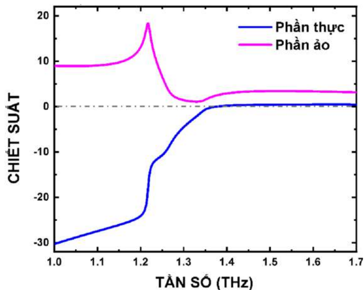
Hình 3.5. Phần thực và phần ảo của chiết suất (chọn nhánh m = -1 )
