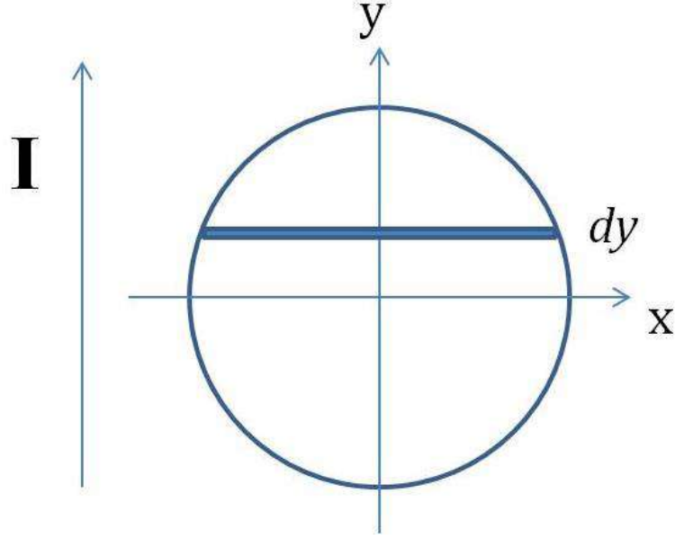
Hình 2.7. Tính toán độ tự cảm động lượng của đĩa tròn [80]
