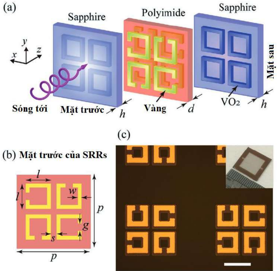
Hình 1.21. a) Cấu trúc ô cơ sở của MM, bao gồm các cặp SRR bằng vàng, kẹp giữa các vòng hình vuông \text{VO}_2 , phân tách bởi lớp điện môi Polyimide, b) Mặt trước lớp SRR của ô cơ sở, với các SRR được đặt xoay với nhau 90^\circ để đạt được khả năng đáp ứng sóng điện từ đẳng hướng. c) Hình ảnh kính hiển vi quang học của các SRR vàng và các vòng vuông \text{VO}_2 với thang đo 40 \mu\text{m} . Khung nhỏ hiển thị ảnh của toàn bộ mẫu. [18]
