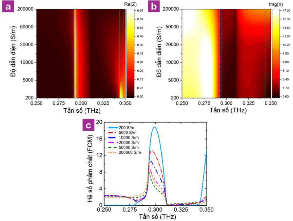
Hình 3.25. (a) Phần thực của trở kháng, (b) Phần ảo của chiết suất và (c) Hệ số phẩm chất (FOM) của cấu trúc vật liệu biến hóa theo tần số với các giá trị độ dẫn điện của \text{VO}_2 khác nhau
