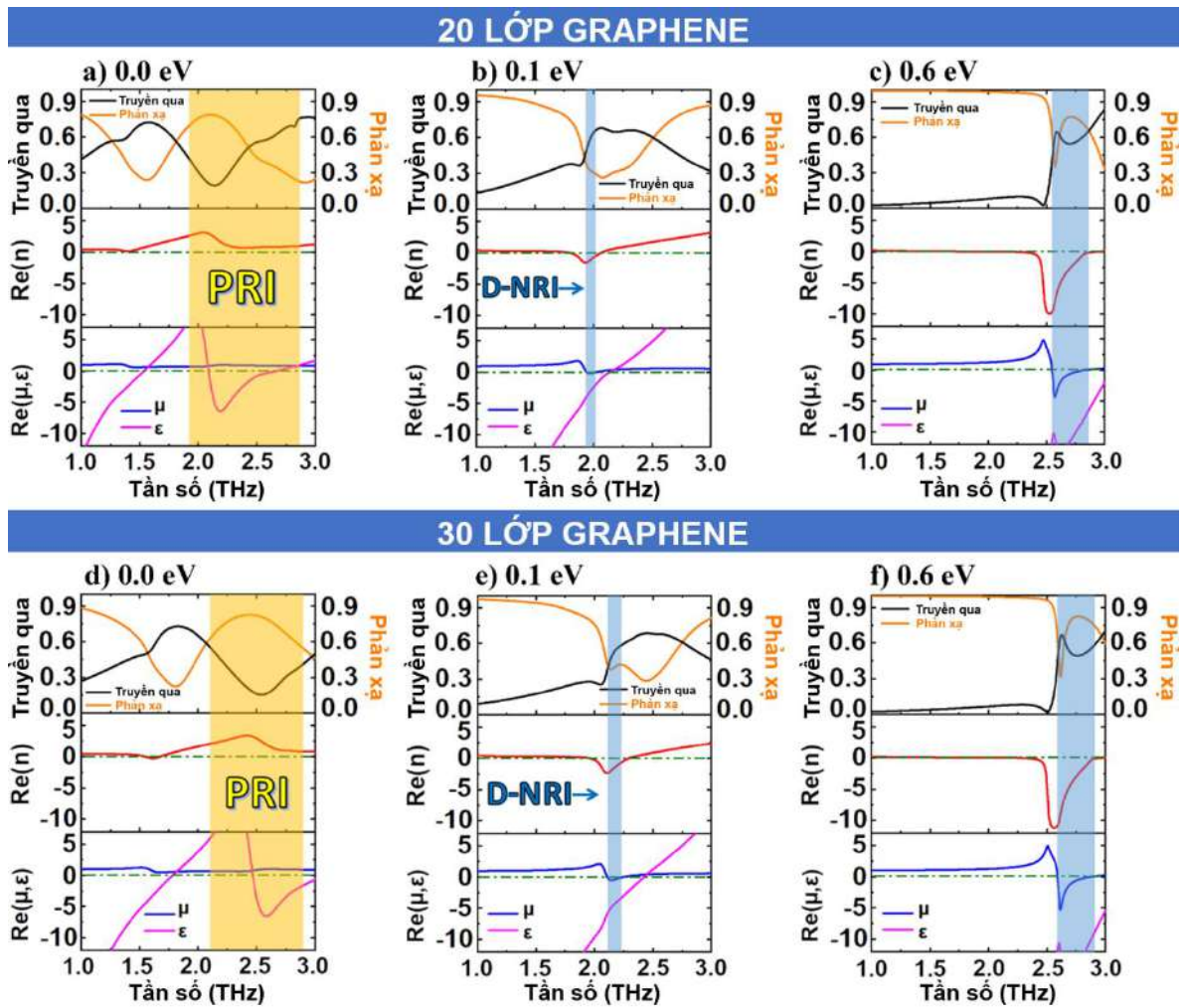
Hình 3.22. Phổ truyền qua mô phỏng và phần thực của chiết suất, từ thẩm và hằng số điện môi của cấu trúc đề xuất với 20 lớp graphene ở a) 0,0\text{ eV} , (b) 0,1\text{ eV} , (c) 0,6\text{ eV} và 30 lớp graphene ở (d) 0,0\text{ eV} , (e) 0,1\text{ eV} và (f) 0,6\text{ eV} .
