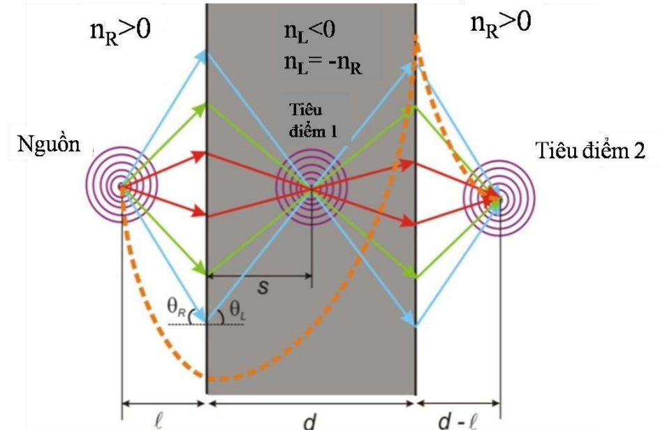
Hình 1.2. Siêu thấu kính dựa trên NRI-MM hoạt động như một thấu kính hội tụ, có khả năng khôi phục và khuếch đại sóng điện từ [26]
