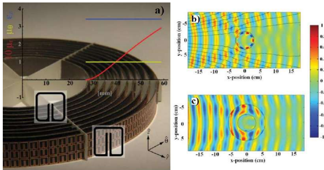
Hình 1.3. a) Cấu trúc của áo choàng tàng hình với các lớp MM có chiết suất khác nhau được sắp xếp một cách hợp lý xung quanh vật thể cần giấu b) đo đạc thực nghiệm của khối trụ dẫn điện và c) đo đạc thực nghiệm của khối trụ dẫn điện đã được bọc lớp vỏ tàng hình [28].
