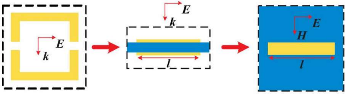
Hình 1.11. Sự biến đổi từ cấu trúc SRR sang cấu trúc CWP [49].
