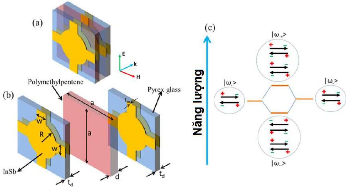
Hình 1.26. a) Cấu trúc ô cơ sở của cấu trúc MM dựa trên 2 cặp lưới đĩa kim loại và b) Thành phần của MM với các tham số cấu trúc và c) Giảm đồ lai hóa tương ứng. [67]
