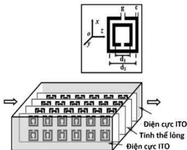
Hình 1.28. Mô hình sử dụng cấu trúc SRR để điều khiển độ từ thẩm âm được nhúng trong tinh thể lỏng [17].
