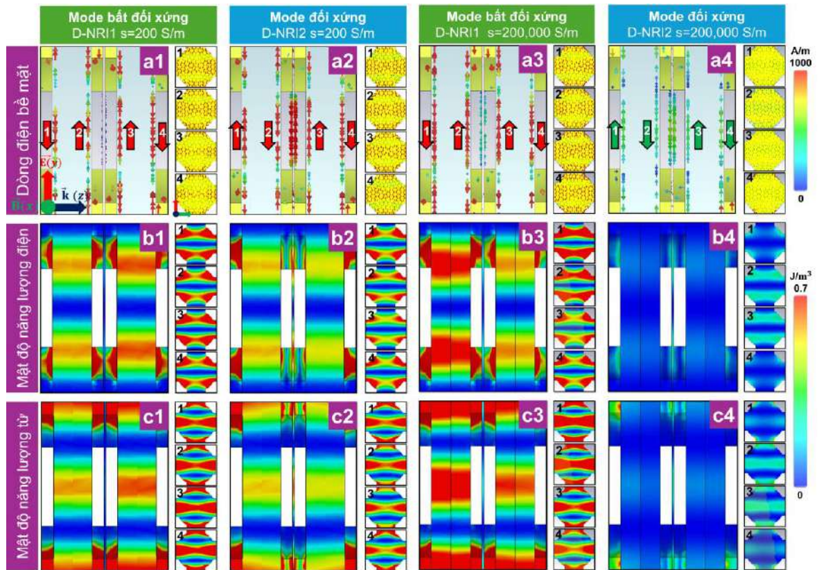
Hình 4.18. Phân bố dòng điện bề mặt (a1-a4), mật độ năng lượng điện trường (b1-b4) và mật độ năng lượng từ trường (c1-c4) tại đỉnh D-NRI 1 và đỉnh D-NRI 2 với hai trường hợp độ dẫn điện VO_2 200 S/m và 200,000 S/m. Các hình chú thích kèm theo thể hiện phân bố của từng lớp mặt cắt
