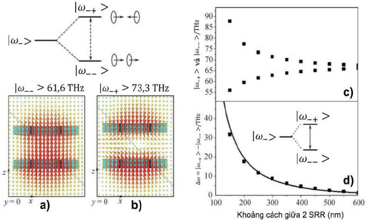
Hình 1.18. Các biểu đồ từ trường của (a) mode cộng hưởng liên kết và (b) mode cộng hưởng bất liên kết, sự phụ thuộc của (c) tần số cộng hưởng và (d) khoảng cách tần số cộng hưởng của các mode theo khoảng cách giữa hai SRR. [64]
