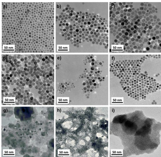
Hình 3.1. Ảnh TEM hạt nano GFO ở các tỉ lệ \text{Gd}^{3+}/\text{Fe}^{3+} lần lượt là 0/10 (a), 1/9 (b), 1.5/8.5 (c), 2/8 (d), 3/7 (e), 7/3 (f), 8/2 (g), 9/1 (h) và 10/0 (i).
