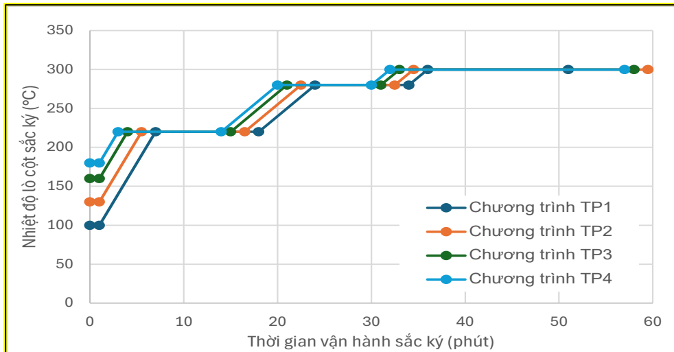
Hình 2.6. Các chương trình nhiệt độ lò cột khảo sát
