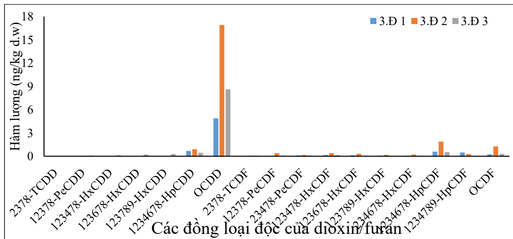
Hình 3.22: Hàm lượng PCDD/F trong mẫu đất làng nghề kim khí
