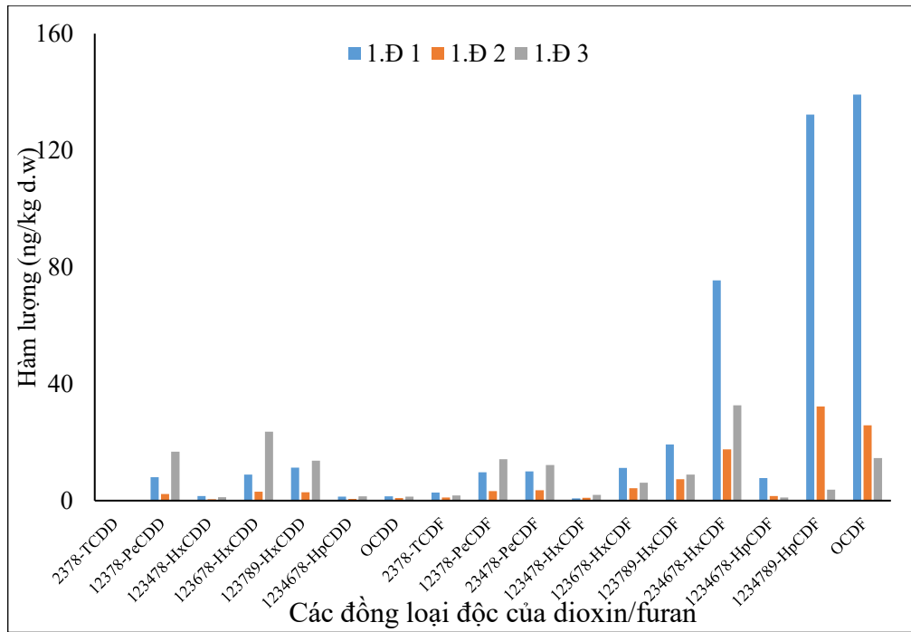
Hình 3.18: Tỷ lệ (%) hàm lượng PCDD/F trong mẫu đất tại làng tái chế nhôm
