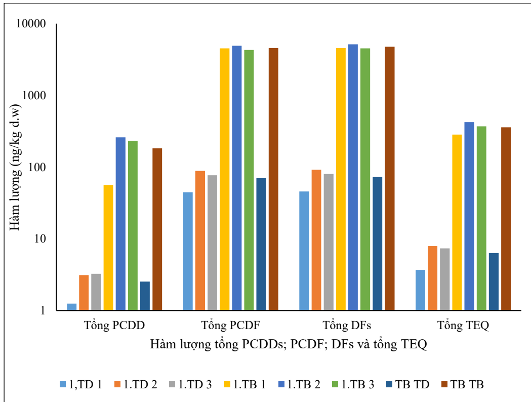
Hình 3.9: Phân bố PCDD/F trong các loại mẫu tro tại làng tái chế nhôm
