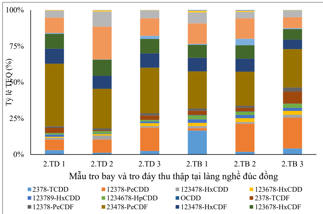
Hình 3.13: Tỷ lệ TEQ (%) các đồng loại độc PCDD/F trong mẫu tro bay và tro đáy
