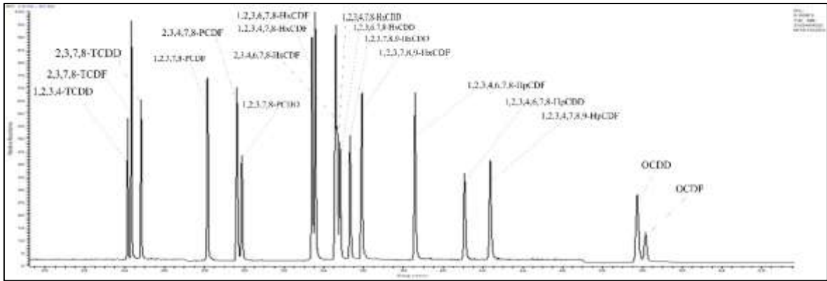
Hình P2.1 Sắc đồ phân tích mẫu chuẩn MCS 3
