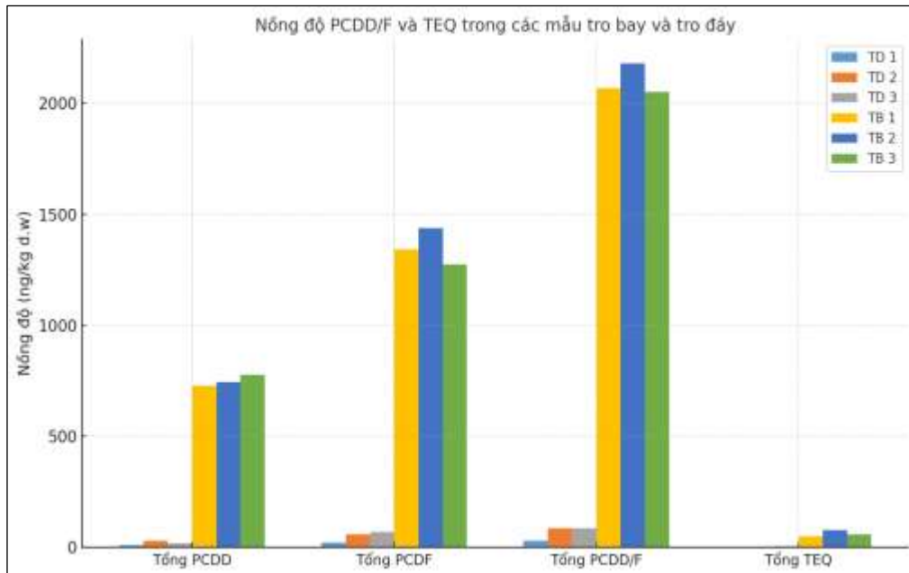
Hình 3.11: Phân bố dioxin và furan trong mẫu tro bay và tro đáy tại làng đúc đồng TD = Tro đáy; TB = Tro bay; TB TD = trung bình tro đáy; TB TB trung bình tro bay
