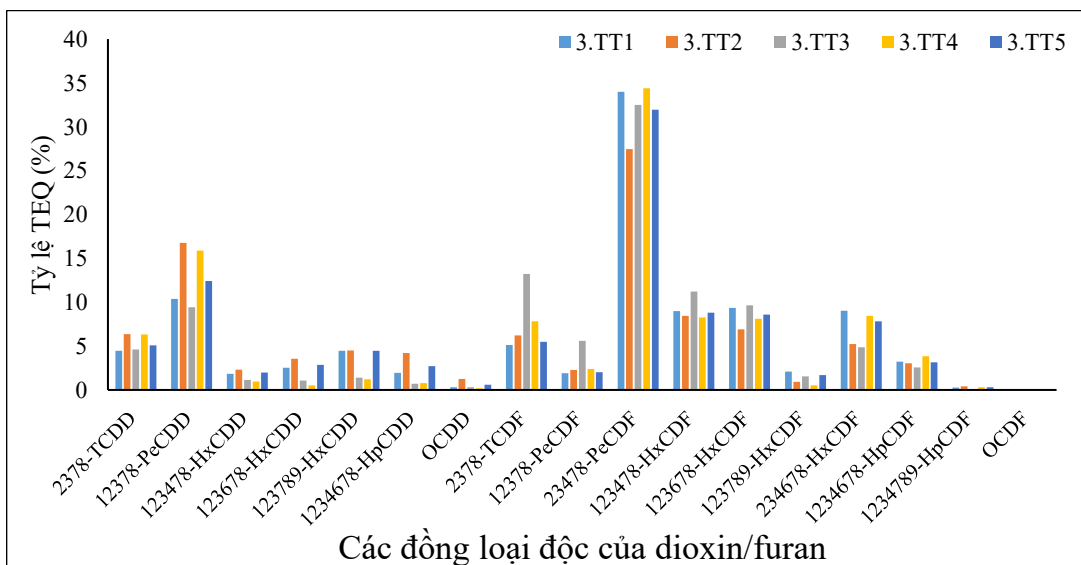
Hình 3.29: Tỷ lệ (%) TEQ của PCDD/F trong trầm tích tại làng nghề kim khí
