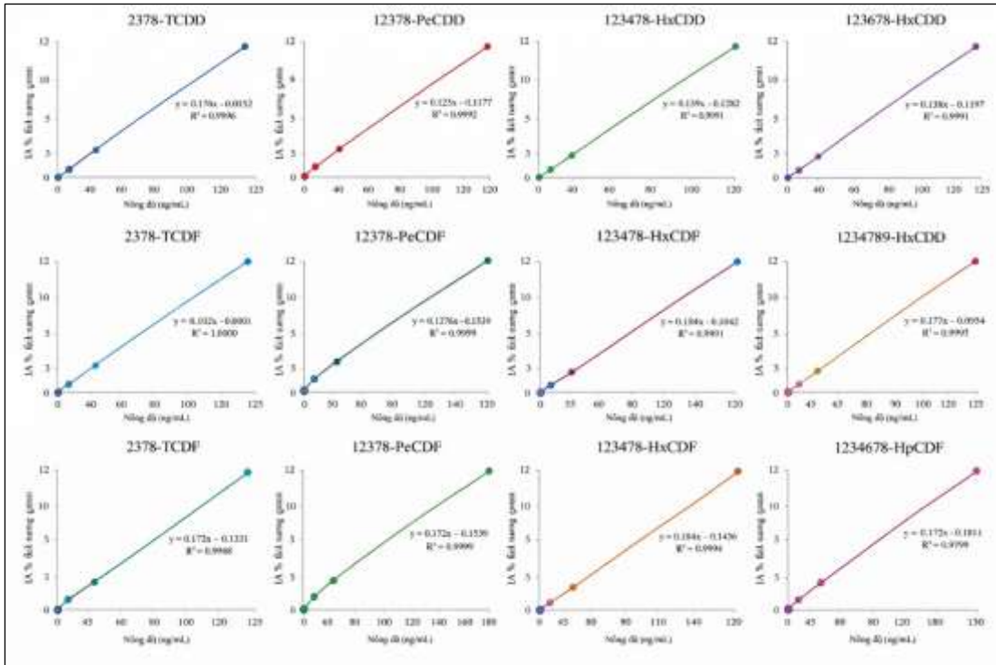
Hình 3.3: Đường chuẩn 17 đồng loại 2,3,7,8-PCDD/F
