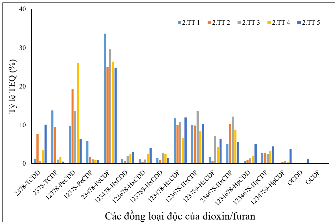
Hình 3.27: Tỷ lệ (%) TEQ của PCDD/F trong trầm tích tại làng đúc đồng
