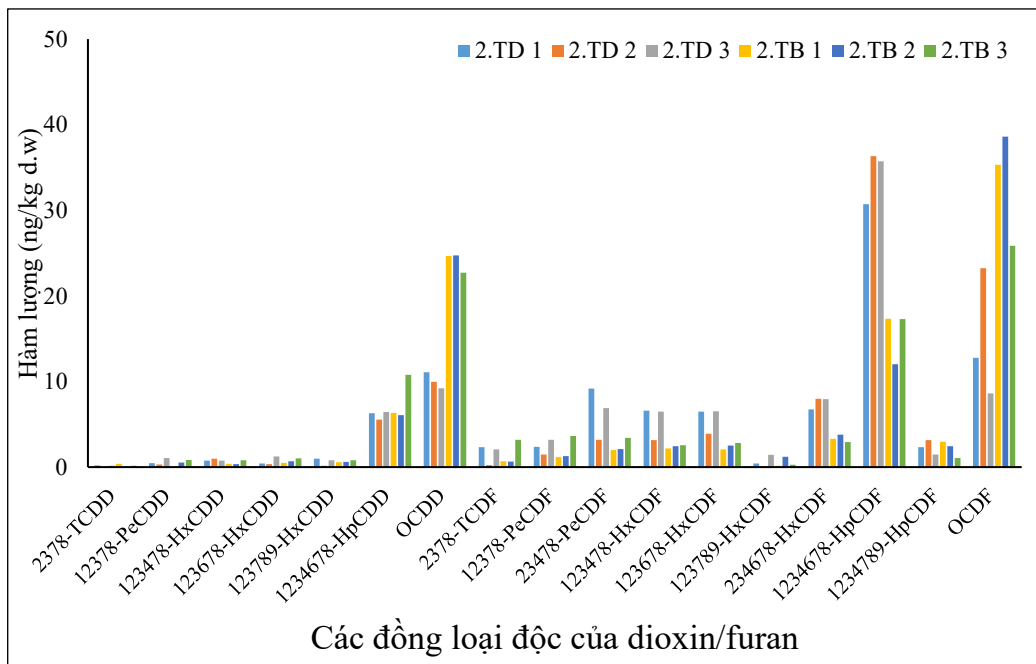
Hình 3.12: Tỷ lệ (%) hàm lượng PCDD/F trong mẫu tro tại làng đúc đồng (TD = tro đáy; TB = tro bay)
