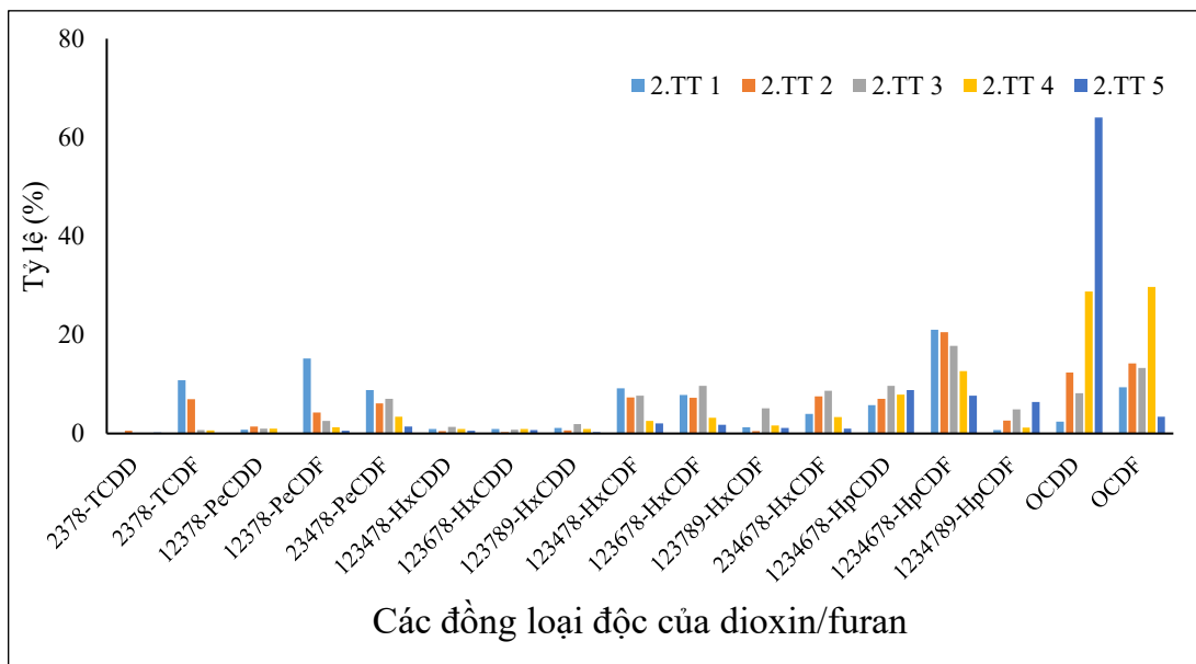
Hình 3.26: Tỷ lệ (%) hàm lượng PCDD/F trong mẫu trầm tích tại làng đúc đồng
