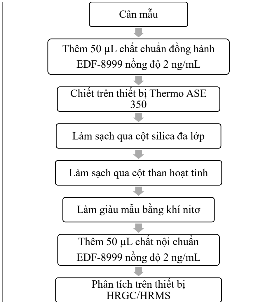
Hình 3.5: Sơ đồ quy trình phân tích PCDD/F
