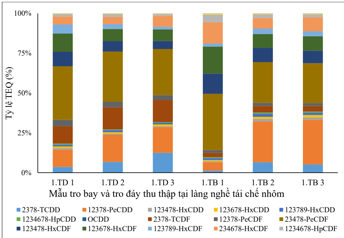
Hình 3.10: Tỷ lệ (%) TEQ của PCDD/Fs trong mẫu tro bay và tro đáy
