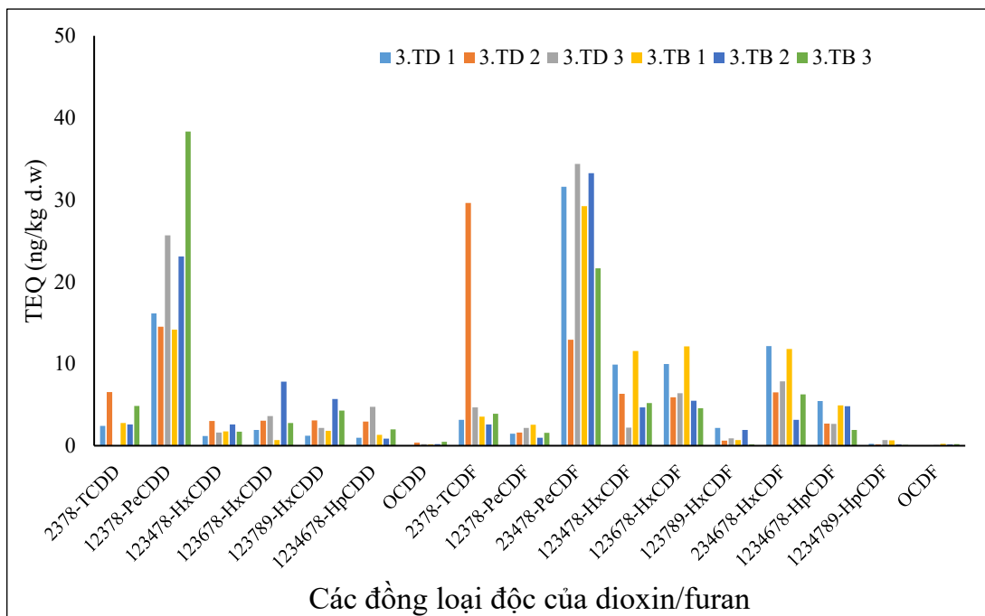
Hình 3.15: Tổng TEQ của PCDD/F trong mẫu tro tại làng kim khí
