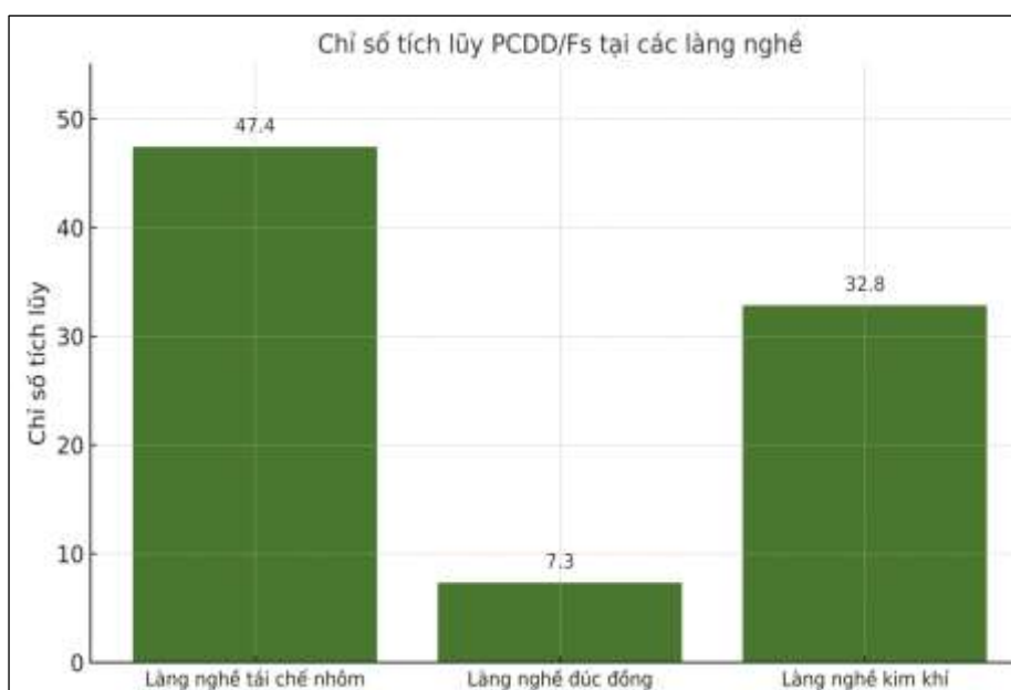
Hình 3.30: Chỉ số tích lũy PCDD/F tại các làng nghề tái chế kim loại
