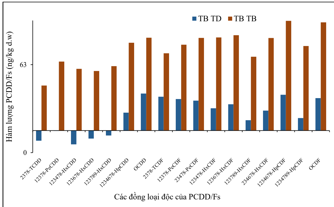
Hình 3.8: Hàm lượng trung bình PCDD/F trong mẫu tro tại làng tái chế nhôm (TB TD = trung bình nồng độ PCDD/F trong mẫu tro đáy; TB TB = trung bình nồng độ PCDD/F trong mẫu tro bay)
