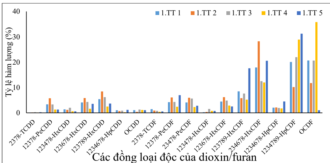
Hình 3.24: Tỷ lệ (%) hàm lượng dioxin/furan trong trầm tích tại làng tái chế nhôm
