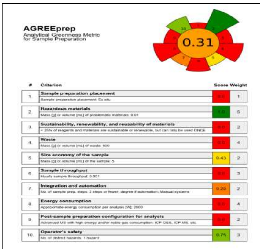
Hình 3.7: điểm “xanh” của phương pháp Soxhlet
