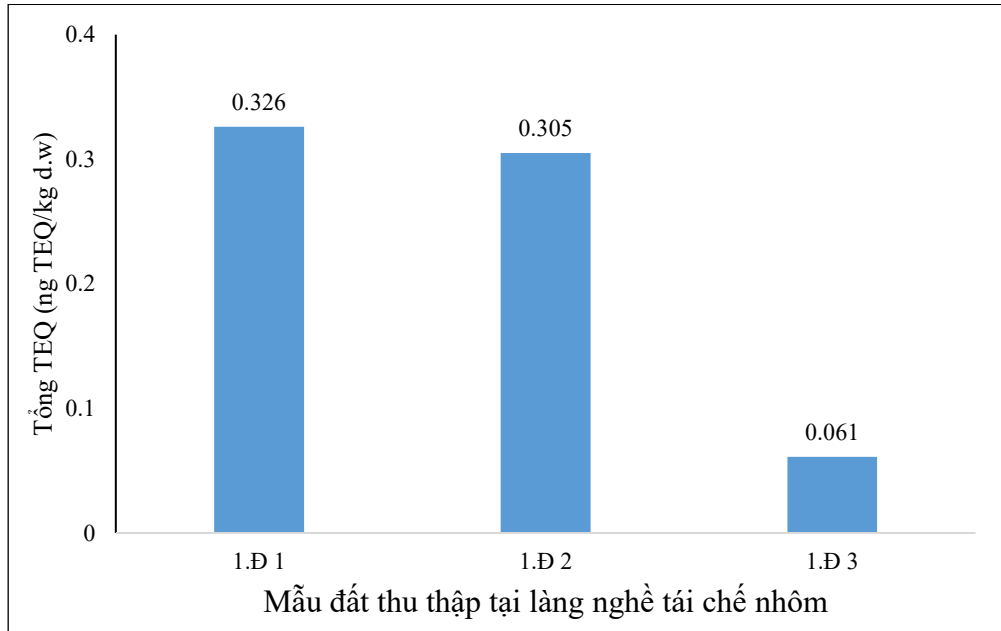
Hình 3.17: Trung bình TEQ của mẫu đất tại làng nghề tái chế nhôm
