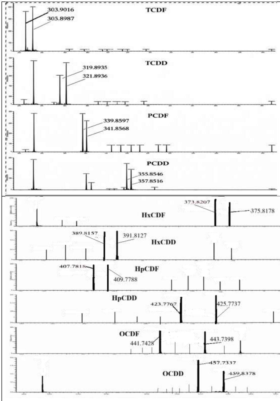
Hình 3.1: Phổ khối của các đồng loại dioxin và furan
