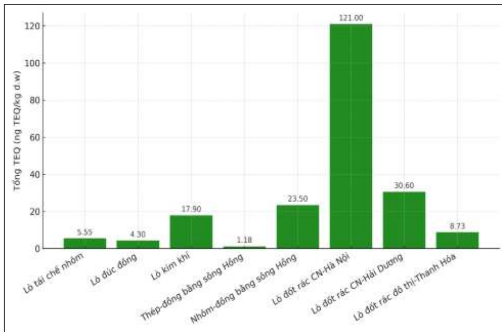
Hình 3.16: Tổng TEQ của PCDD/F trong mẫu tro đáy ở một số loại lò đốt
