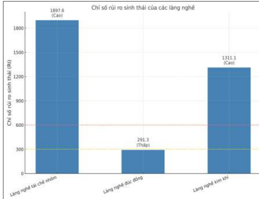
Hình 3.31: Chỉ số rủi ro sinh thái của PCDD/Fs tại các làng nghề.
