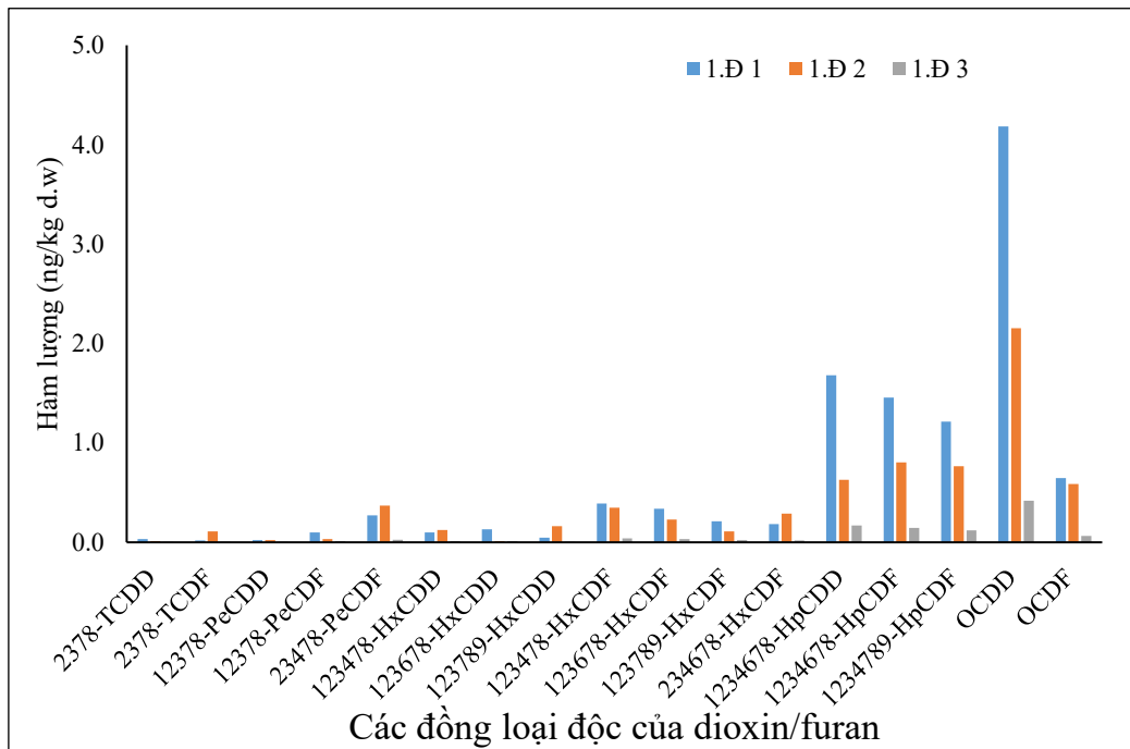
Hình 3.20: Hàm lượng của PCDD/F trong mẫu đất tại làng nghề đúc đồng
