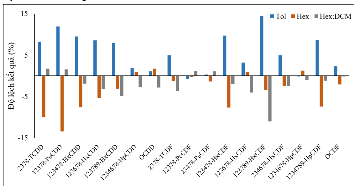
Hình 3.4: Độ lệch kết quả hàm lượng dioxin trong mẫu tro bay
