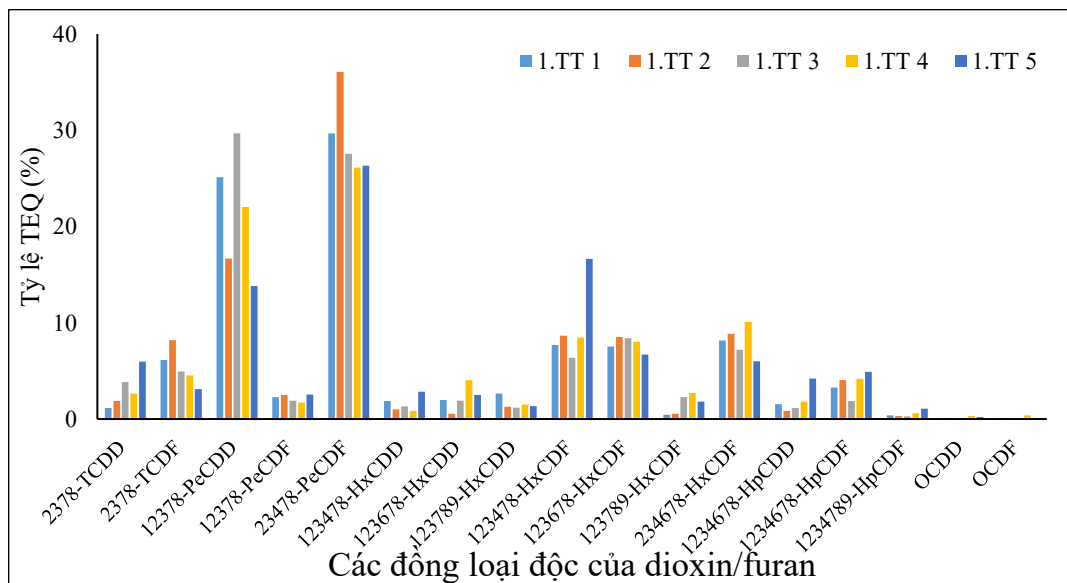
Hình 3.25: Tỷ lệ (%) TEQ của PCDD/F trong trầm tích tại làng nghề tái chế nhôm
