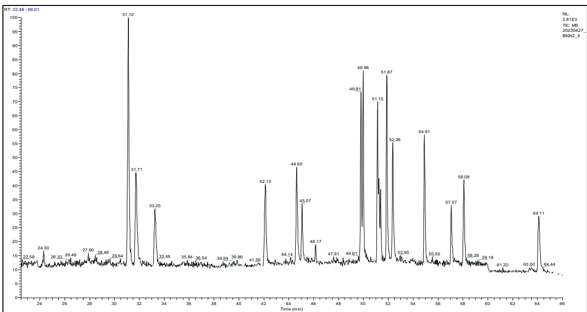
Hình P2.2: Sắc đồ phân tích mẫu tro bay
