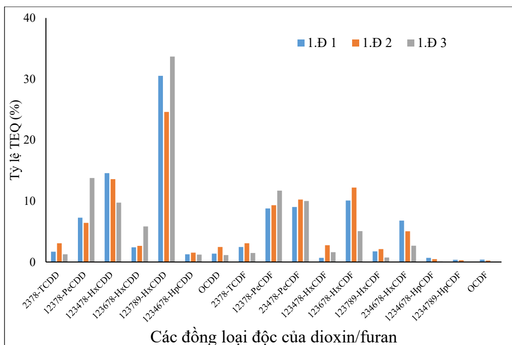
Hình 3.19: Tỷ lệ (%) TEQ của PCDD/F trong mẫu đất tại làng tái chế nhôm
