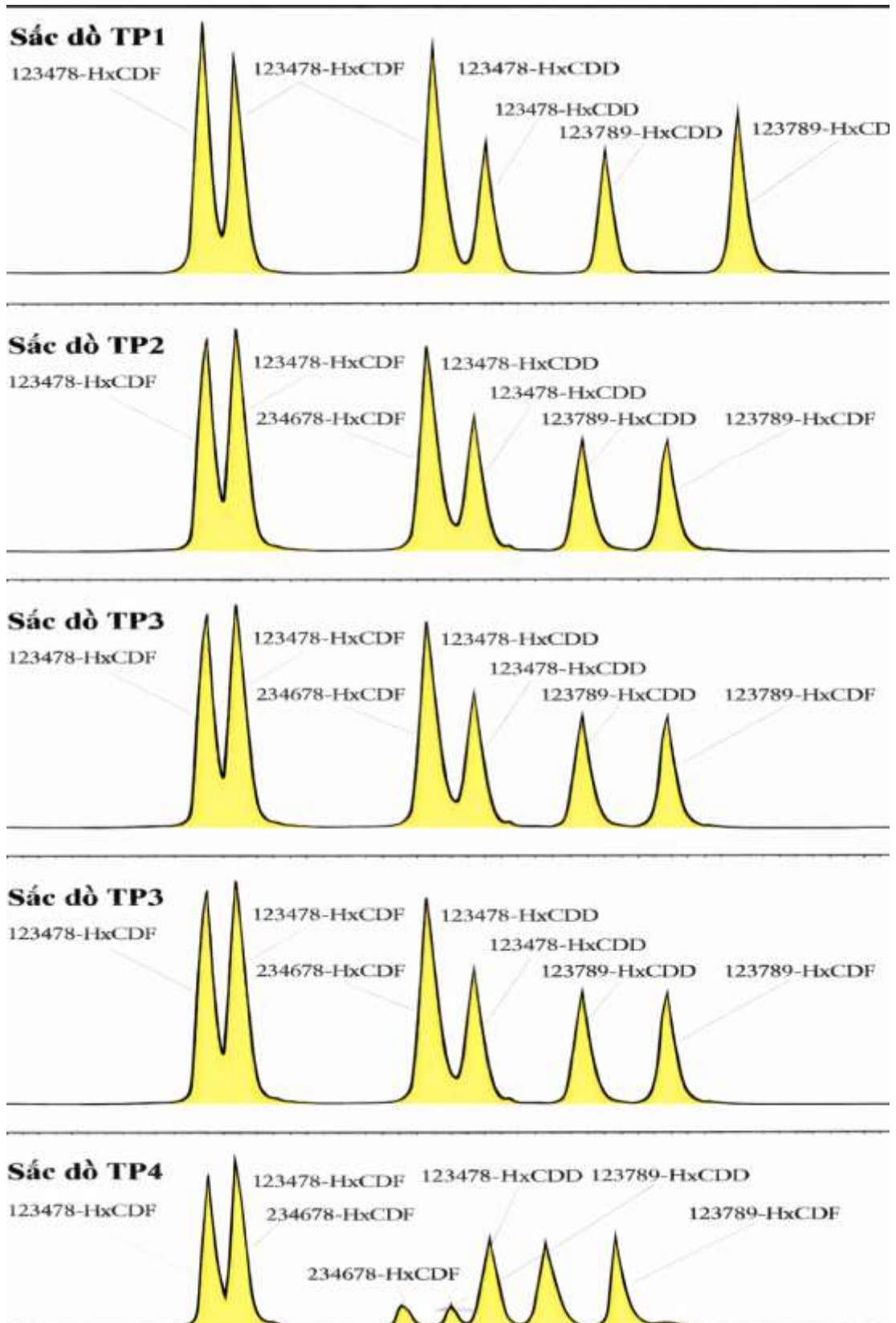
Hình 3.2: Sắc đồ dioxin/furan theo chương trình nhiệt độ TP1; TP2; TP3 và TP4
