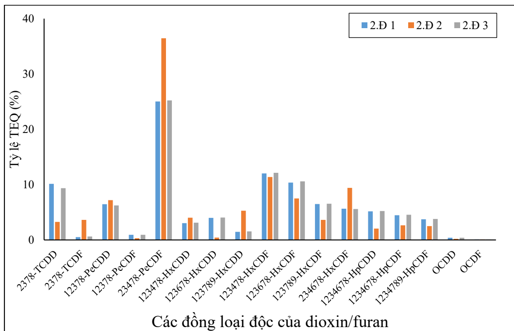
Hình 3.21: Tỷ lệ (%)TEQ của PCDD/F trong mẫu đất ở làng nghề đúc đồng
