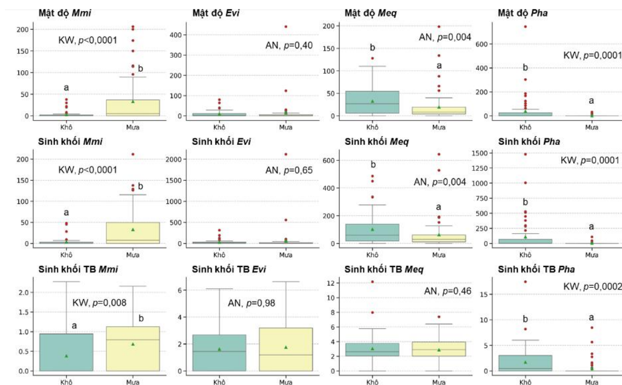
Hình 3.22. Mật độ (cá thể/1.000 m 2 ), sinh khối (g/1.000 m 2 ) và sinh khối trung bình (g) của 4 loài tôm điển hình cho 4 nhóm sinh thái tôm phân bố theo mùa. AN: ANOVA, KW: Kruskal-Wallis, các ký tự a , b là phân tích hậu kiểm, cùng ký tự là khác biệt không ý nghĩa thống kê ( p > 0,05 ). Tên loài viết tắt thể hiện trong Bảng 3.6. (Chú thích biểu đồ hộp: Chấm đỏ: Giá trị ngoại lệ, tam giác xanh lá: Giá trị trung bình, đường gạch ngang: Giá trị trung vị)
