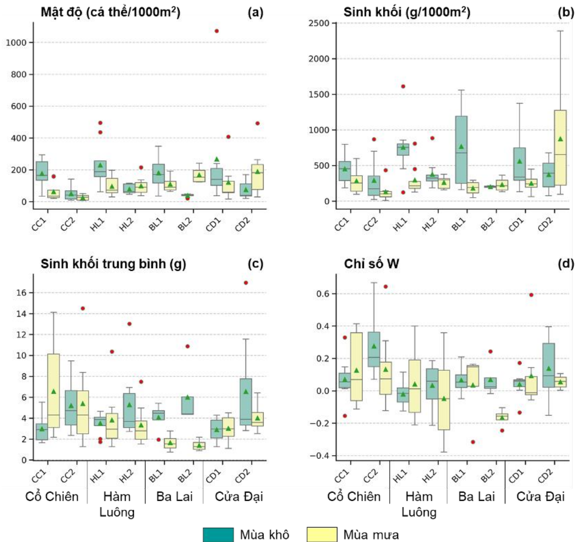
Hình 3.8. Mật độ và sinh khối khu hệ tôm cửa sông Mê Kông ở các vị trí thu mẫu trong 2 mùa khảo sát. (Chú thích biểu đồ hộp: Chấm đỏ: Giá trị ngoại lệ, tam giác xanh lá: Giá trị trung bình, đường gạch ngang: Giá trị trung vị)
