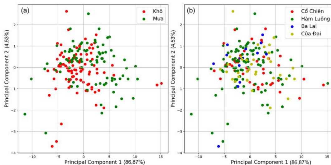
Hình 3.23. Biểu đồ phân tán thể hiện hai thành phần chính đầu tiên (PC1 và PC2) từ phân tích thành phần chính (PCA). (a) Theo thời gian (mùa), (b) theo không gian (cửa sông)
