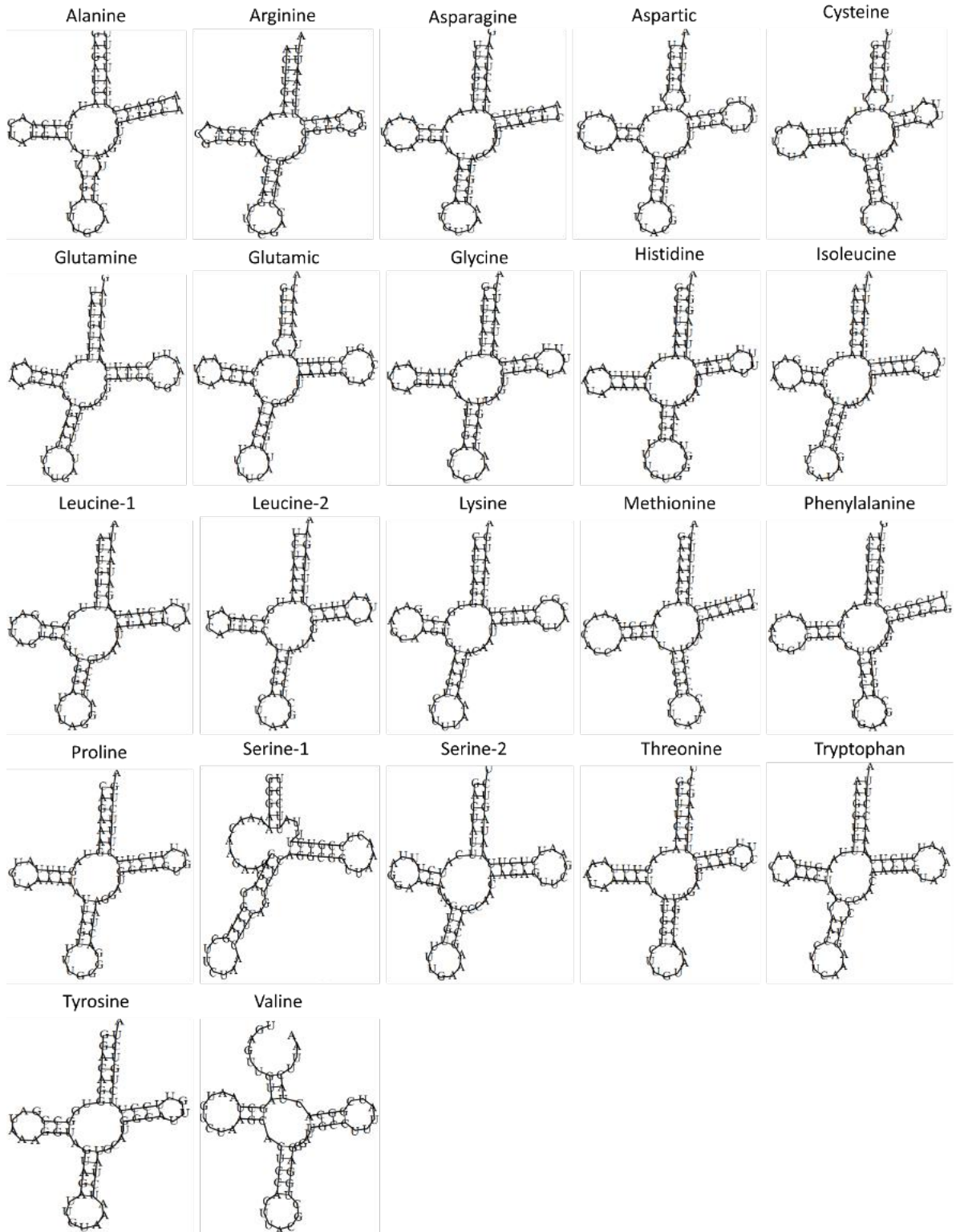
Hình 3.3. Cấu trúc bậc 2 của các tRNA trong bộ gen ty thể tôm càng xanh Mê Kông Sắp xếp gen
