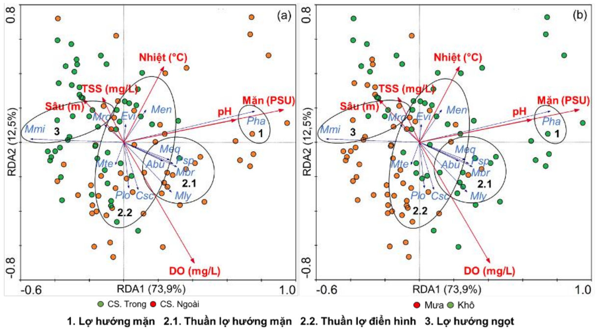
Hình 3.19. Phân tích RDA (Redundancy analysis) mô tả mối liên hệ đa biến giữa các loài điển hình trong khu hệ tôm và các thông số môi trường theo không gian (a) và thời gian (b). Tên loài viết tắt thể hiện trong Bảng 3.6
