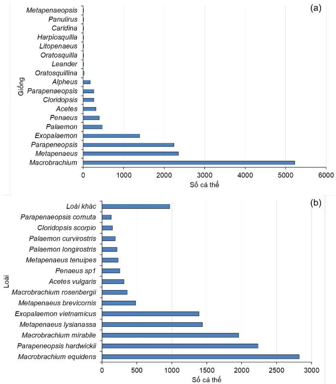
Hình 3.7. Số cá thể ghi nhận của các giống (a) và loài (b) trong quần xã tôm
