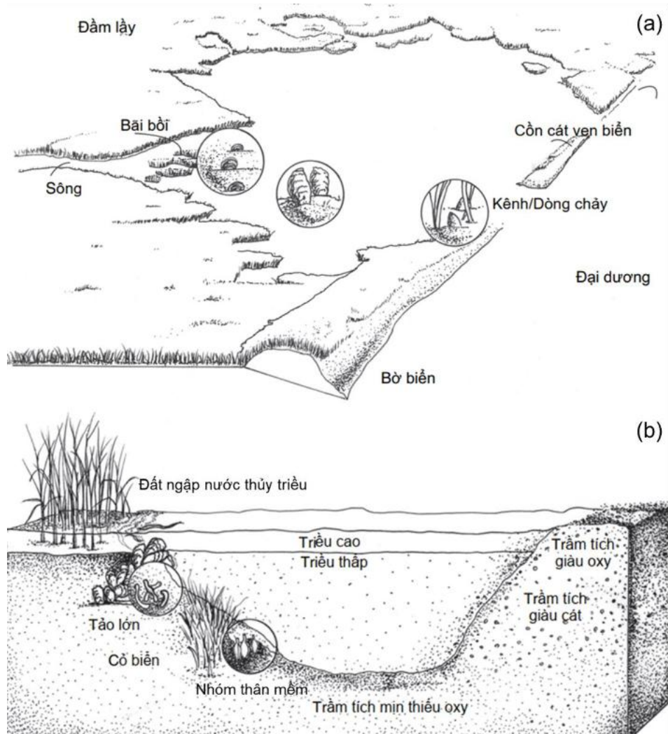
Phụ lục 1.4. Một số tiểu hệ sinh thái vùng cửa sông đồng bằng đầm lầy ven biển. (a) Theo mặt cắt ngang, (b) theo mặt cắt đứng [14]
