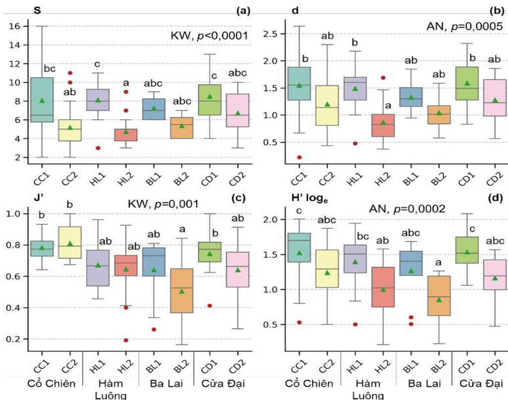
Hình 3.11. Các chỉ số đa dạng tổng hợp khu hệ tôm cửa sông Mê Kông ở các vị trí thu mẫu. AN: ANOVA, KW: Kruskal-Wallis, các ký tự a , b , c là phân tích hậu kiểm, cùng ký tự là khác biệt không ý nghĩa thống kê ( p > 0,05 )
