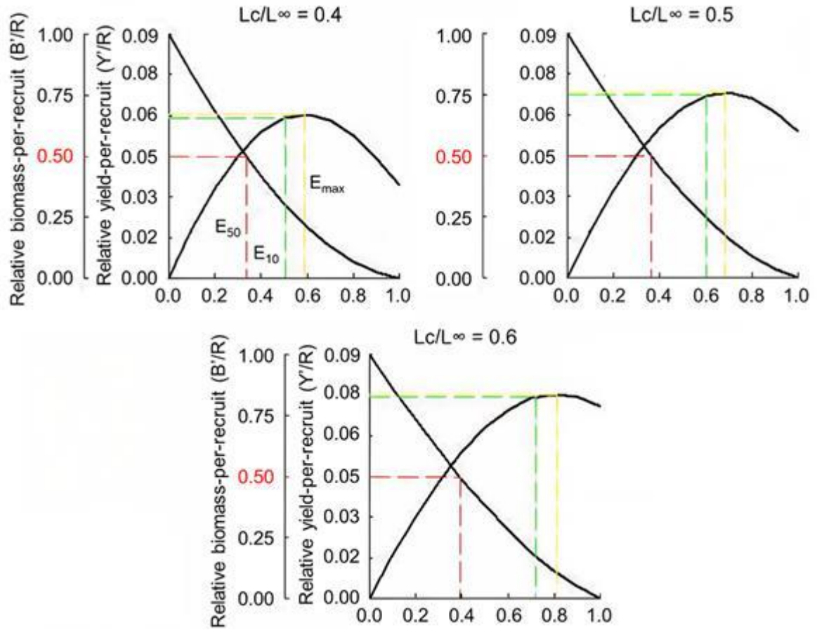
Hình 3.31. So sánh Y/R và B/R theo các kịch bản khai thác L_c/L_\infty
