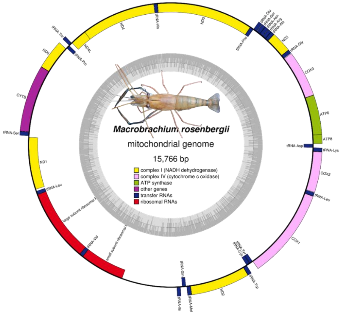
Hình 3.2. Sơ đồ thể hiện bộ gen ty thể dạng vòng của tôm càng xanh Mê Kông. Các gen nằm phía ngoài vòng tròn được phiên mã từ mạch nhẹ (L strand), trong khi các gen nằm phía trong được phiên mã từ mạch nặng (H strand). Vòng trong cùng thể hiện sự phân bố hàm lượng GC. Vùng điều hòa chưa được chú thích
