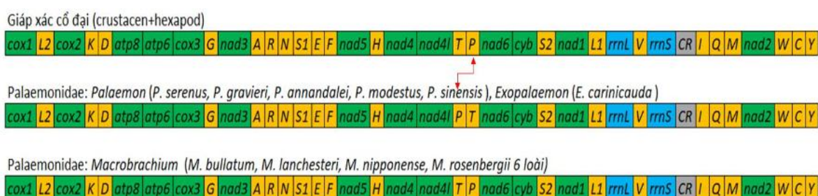
Hình 3.4. Kiểu sắp xếp các gen trong bộ gen ty thể các loài trong họ tôm càng Palaemonidae. Hình không mang tính so sánh theo kích thước
