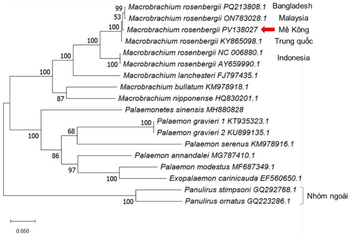
Hình 3.5. Cây phát sinh chủng loài được xây dựng theo phương pháp Maximum Likelihood (ML) dựa trên 13 gen mã hóa protein (PCGs) trong bộ gen ty thể của các loài thuộc họ Palaemonidae. Các con số bên cạnh các nút nhánh biểu thị giá trị bootstrap (%) từ phân tích ML
