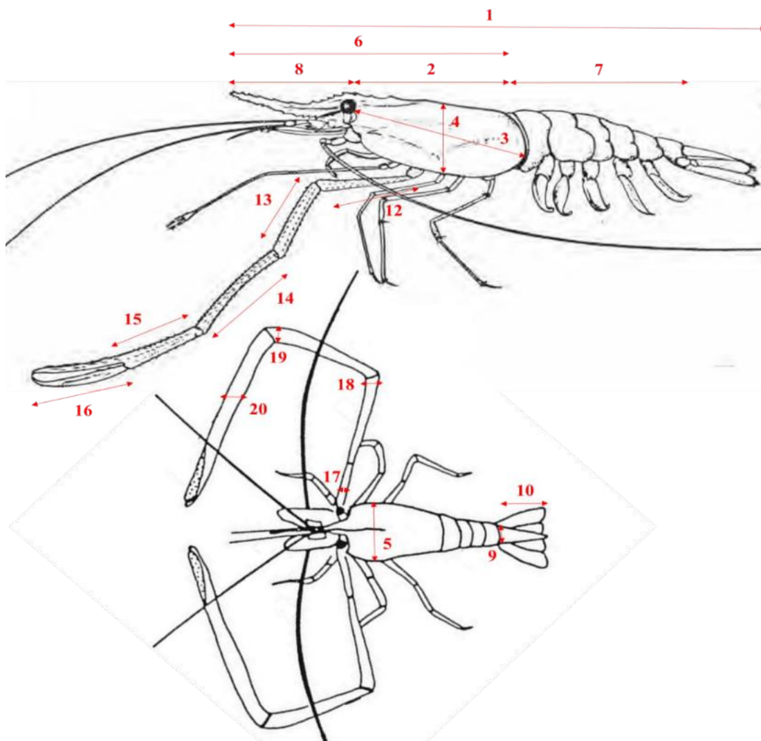
Hình 2.2. Các đặc điểm hình thái tôm càng xanh được sử dụng trong nghiên cứu.
