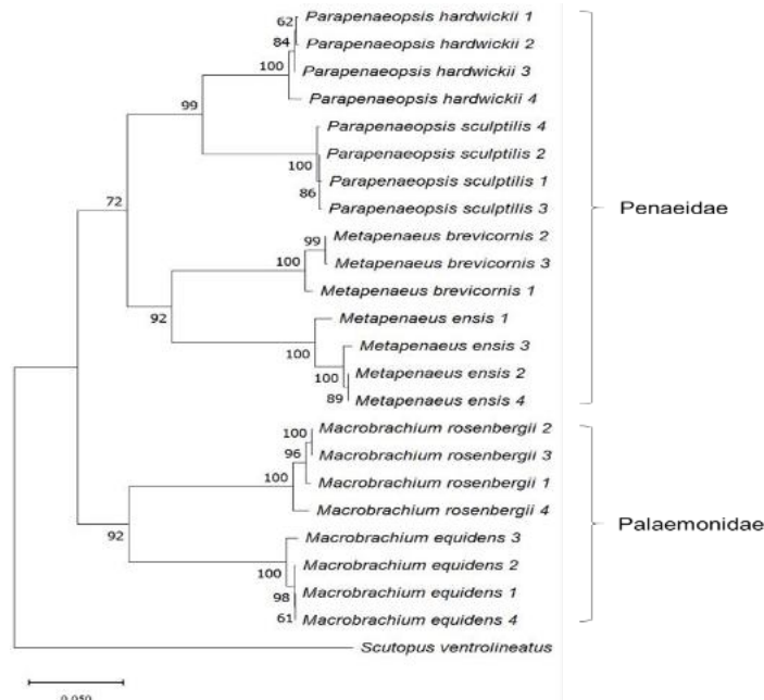
Hình 3.1. Quan hệ di truyền các loài có giá trị thương mại trong khu hệ tôm vùng cửa sông Mê Kông dựa vào gen COI . Phương pháp phân tích Maximum Likelihood + bootstrap 1.000 lần
