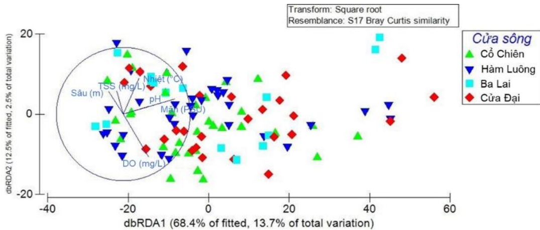
Hình 3.16. Phân tích DistLM (Distance based linear models) và minh họa qua biểu đồ dbRDA (Distance-based redundancy analysis) mô tả mối liên hệ đa biến giữa khu hệ tôm và các thông số môi trường theo cửa sông
