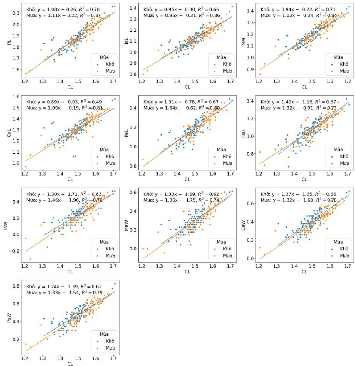
Hình 3.26. Mô hình hồi quy tuyến tính giữa các đặc điểm hình thái chân ngực thứ hai của tôm càng xanh (biến phụ thuộc y, PL, IsL, MeL, CaL, PaL, DaL, IsW, MeW, CaW, PaW) và chiều dài đầu ngực (biến độc lập x, CL). Tất cả các đặc điểm hình thái đều chuyển về dạng logarit (log). Mô hình dạng \log(y) = \log(a) + b \cdot \log(x) . Các đặc điểm hình thái viết tắt trong Bảng 2.1
