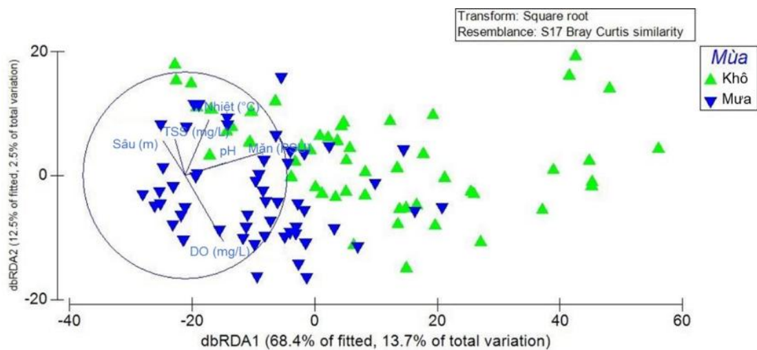
Hình 3.18. Phân tích DistLM (Distance based linear models) và minh họa qua biểu đồ dbRDA (Distance-based redundancy analysis) mô tả mối liên hệ đa biến giữa khu hệ tôm và các thông số môi trường theo mùa
