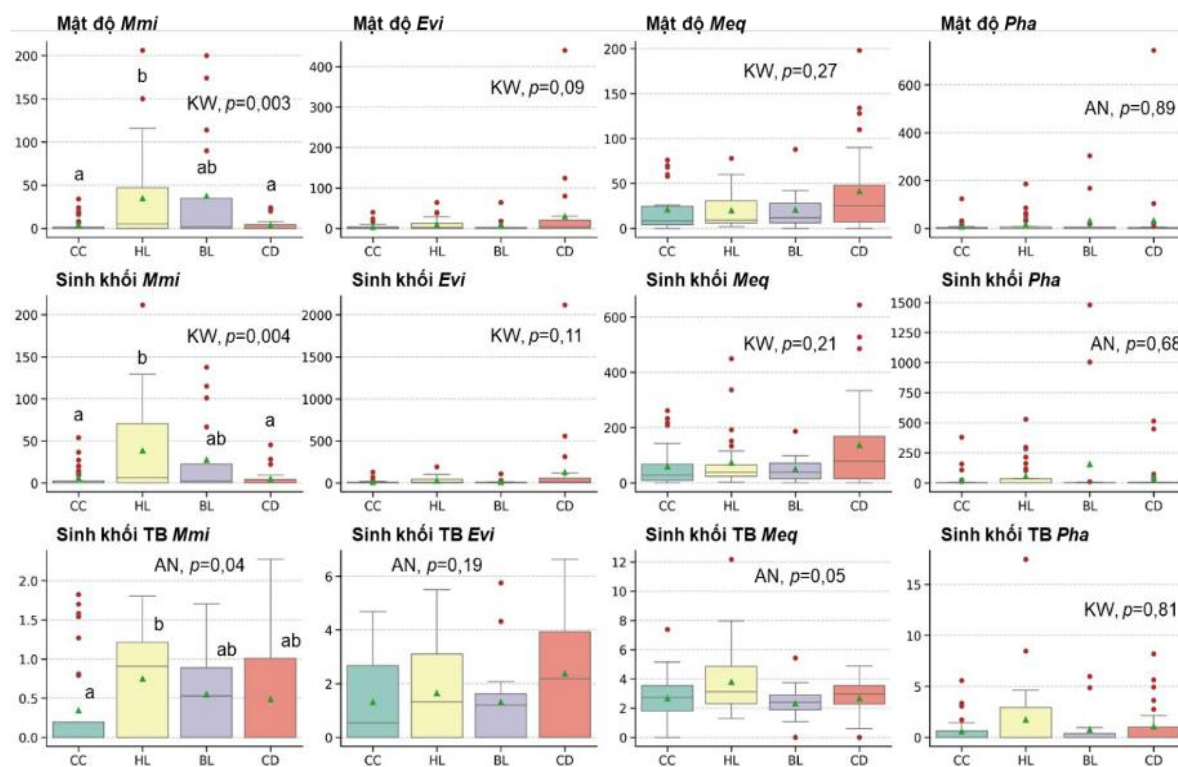
Hình 3.20. Mật độ ( cá thể/1.000 m 2 ), sinh khối (g/1.000 m 2 ) và sinh khối trung bình cá thể (g) của 4 loài tôm điển hình cho 4 nhóm sinh thái tôm phân bố theo cửa sông.
