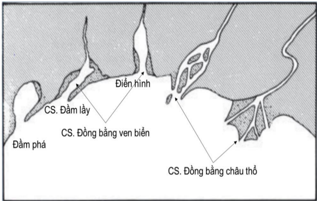
Phụ lục 1.2. Phân loại cửa sông [290]
