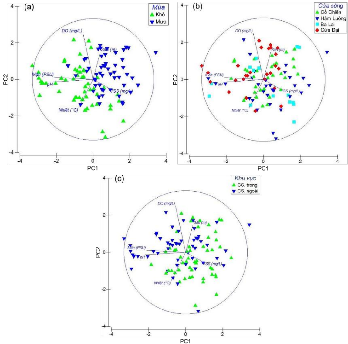
Hình 3.15. Biểu đồ PCA dựa trên các thông số môi trường sống của quần xã tôm cửa sông Mê Kông theo mùa (a), cửa sông (b) và khu vực khảo sát (c)
