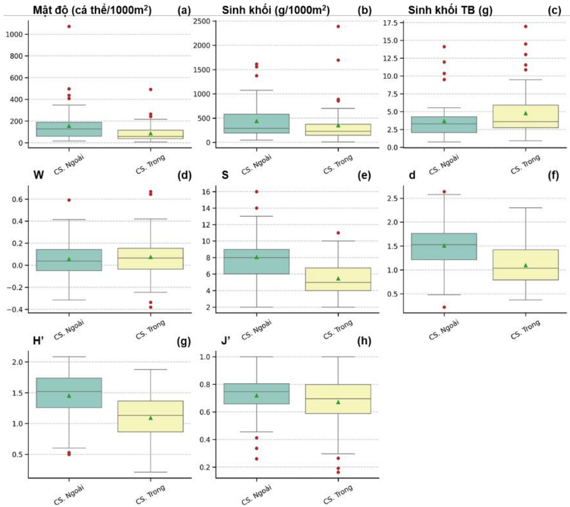
Hình 3.13. Các đặc điểm khu hệ tôm cửa sông Mê Kông phân bố theo khu vực khảo sát. (Chú thích biểu đồ hộp: Chấm đỏ: Giá trị ngoại lệ, tam giác xanh lá: Giá trị trung bình, đường gạch ngang: Giá trị trung vị)
