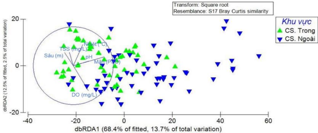
Hình 3.17. Phân tích DistLM (Distance based linear models) và minh họa qua biểu đồ dbRDA (Distance-based redundancy analysis) mô tả mối liên hệ đa biến giữa khu hệ tôm và các thông số môi trường theo khu vực khảo sát
