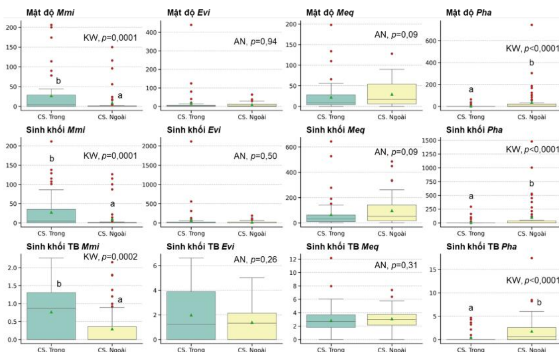
Hình 3.21. Mật độ (cá thể/1.000 m 2 ), sinh khối (g/1.000 m 2 ) và sinh khối trung bình (g) của 4 loài tôm điển hình cho 4 nhóm sinh thái tôm phân bố theo khu vực khảo sát. AN: ANOVA, KW: Kruskal-Wallis, các ký tự a , b là phân tích hậu kiểm, cùng ký tự là khác biệt không ý nghĩa thống kê ( p > 0,05 ). Tên loài viết tắt thể hiện trong Bảng 3.6. (Chú thích biểu đồ hộp: Chấm đỏ: Giá trị ngoại lệ, tam giác xanh lá: Giá trị trung bình, đường gạch ngang: Giá trị trung vị)
