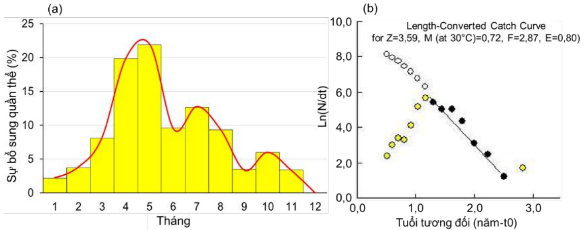
Hình 3.30. Sự bổ sung quần thể (recruitment patterns) của tôm càng xanh cửa sông Mê Kông trong 1 năm (a) và đường cong sản lượng chuyển đổi thành chiều dài (Length - converted catch curve) của tôm càng xanh (b)
