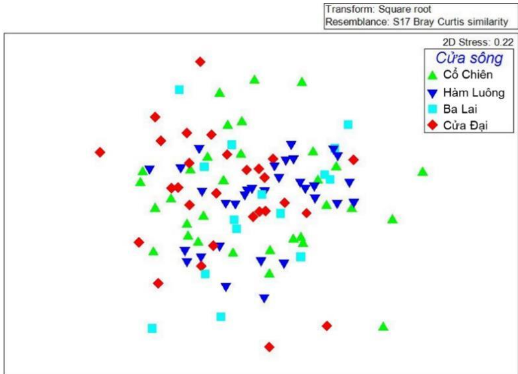
Phụ lục 3.6. Phân tích nMDS (Non- metric Multidimensional scaling) cấu trúc phân bố khu hệ tôm theo cửa sông
