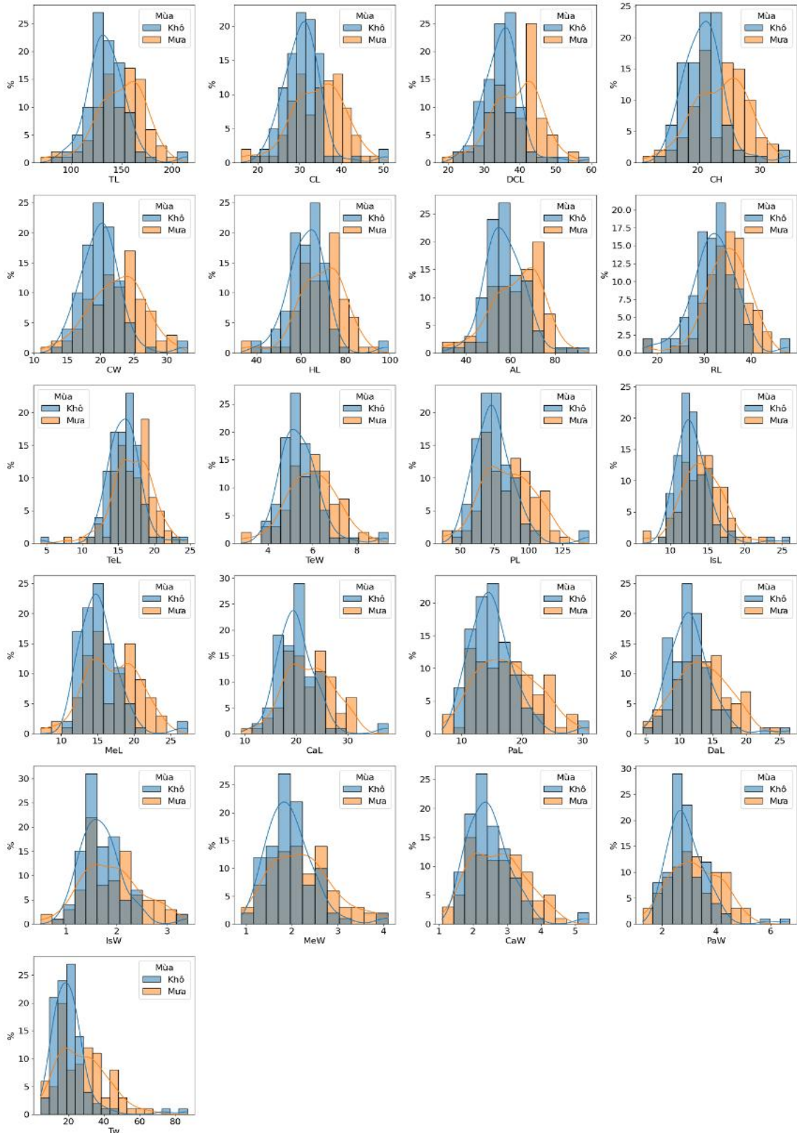
Hình 3.24. Phân phối tần suất của các đặc điểm hình thái tôm càng xanh theo mùa Mối quan hệ giữa các đặc điểm hình thái tôm càng xanh
