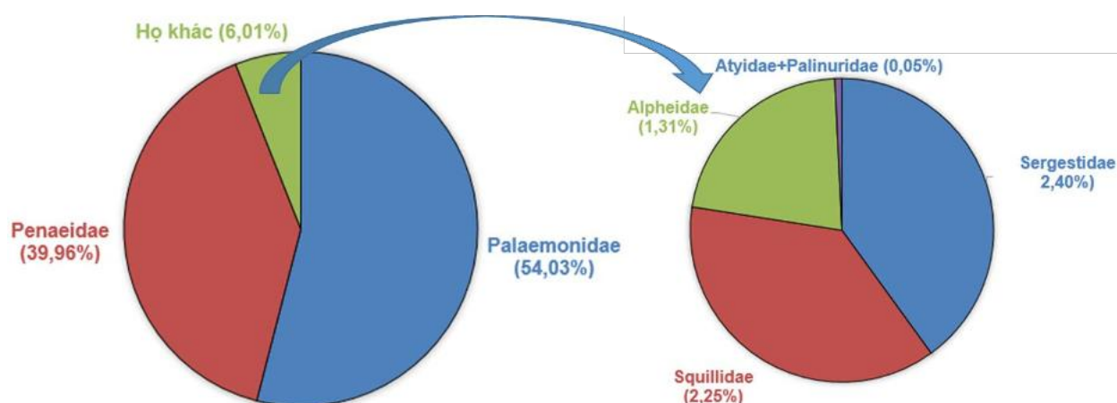
Hình 3.6. Tỷ lệ các họ trong quần xã tôm cửa sông Mê Kông
