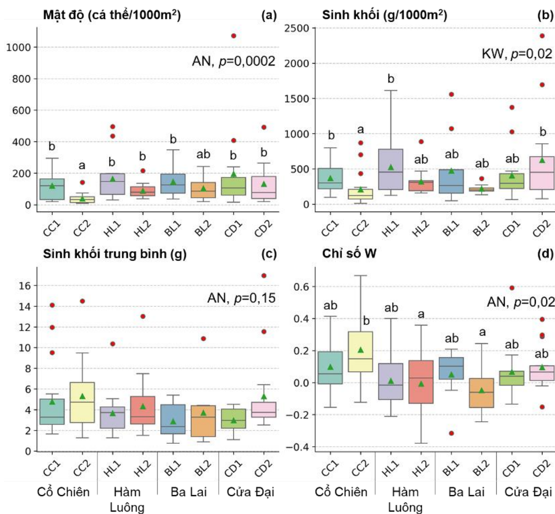
Hình 3.9. Mật độ, sinh khối và chỉ số W trung bình của khu hệ tôm cửa sông Mê Kông ở các vị trí thu mẫu. AN: ANOVA, KW: Kruskal-Wallis, các ký tự a, b là phân tích hậu kiểm, cùng ký tự là khác biệt không ý nghĩa thống kê ( p > 0,05 ). (Chú thích biểu đồ hộp: Chấm đỏ: Giá trị ngoại lệ, tam giác xanh lá: Giá trị trung bình, đường gạch ngang: Giá trị trung vị)
