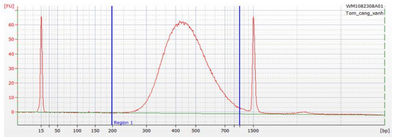
Phụ lục 3.2. Kết quả phân tích kích thước trung bình của thư viện bằng Bioanalyzer
