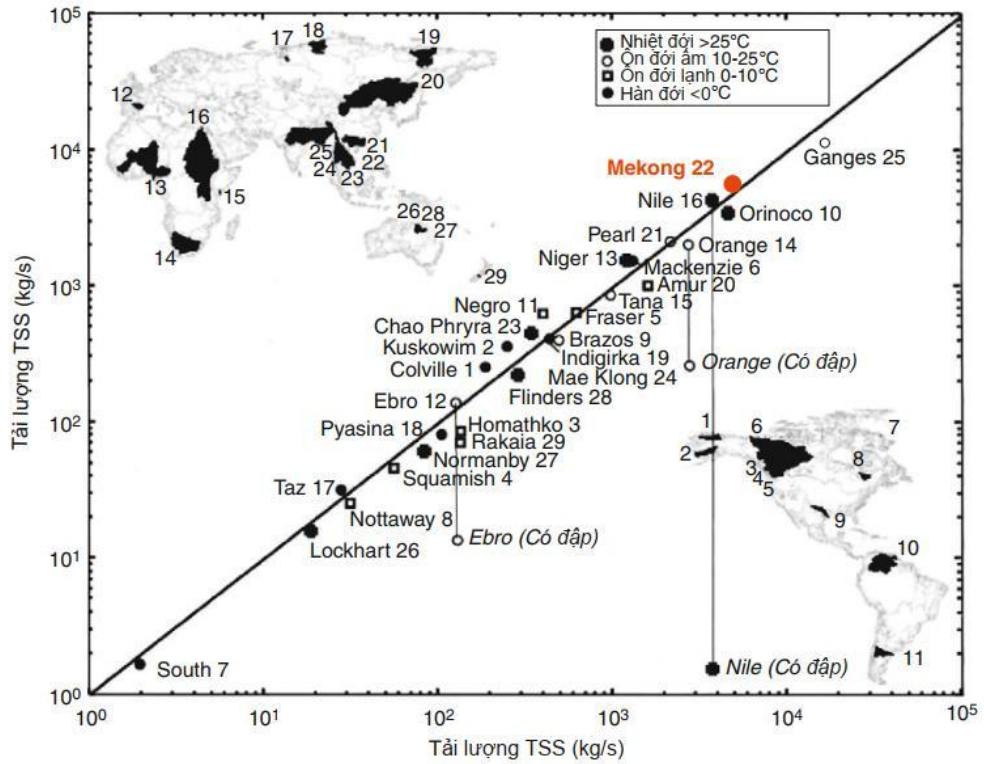
Phụ lục 1.11. So sánh tải lượng TSS của sông Mê Kông với các con sông khác trên thế giới [24]
