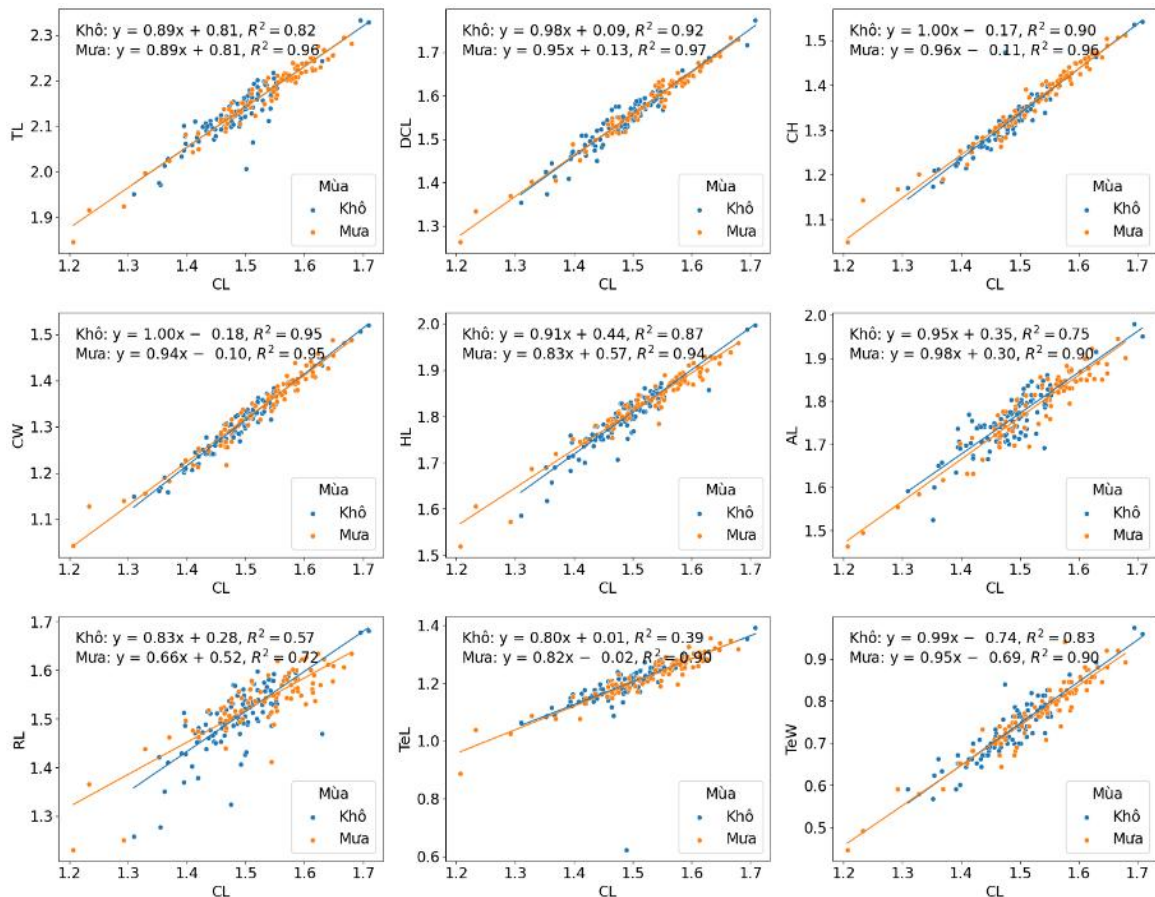
Hình 3.25. Mô hình hồi quy tuyến tính giữa các đặc điểm hình thái tôm càng xanh (biến phụ thuộc y, TL, DCL, CH, CW, HL, AL, RL, TeL, TeW) và chiều dài đầu ngược (biến độc lập x, CL). Tất cả các đặc điểm hình thái đều chuyển về dạng logarit (log). Mô hình dạng \log(y) = \log(a) + b \cdot \log(x) . Các đặc điểm hình thái viết tắt trong
