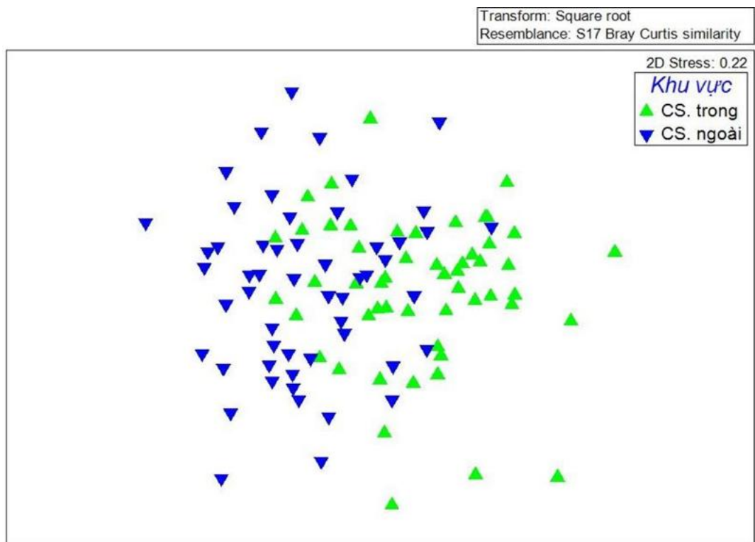
Phụ lục 3.7. Phân tích nMDS (Non-metric Multidimensional scaling) cấu trúc phân bố khu hệ tôm theo khu vực khảo sát
