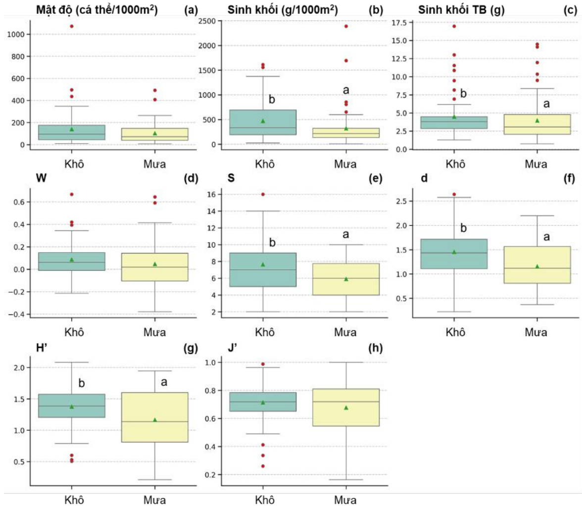
Hình 3.14. Các đặc điểm khu hệ tôm cửa sông Mê Kông phân bố theo mùa. (Chú thích biểu đồ hộp: Chấm đỏ: Giá trị ngoại lệ, tam giác xanh lá: Giá trị trung bình, đường gạch ngang: Giá trị trung vị)
