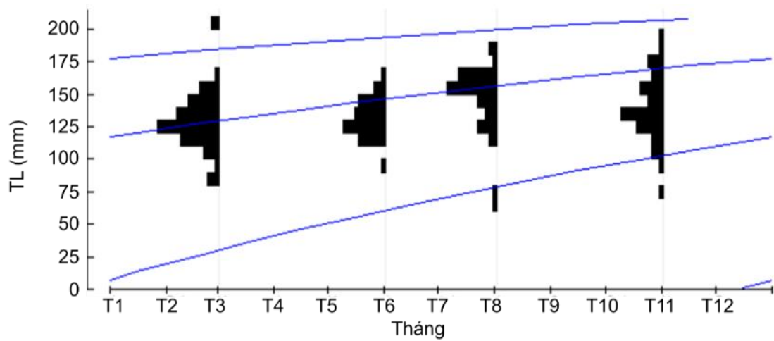
Hình 3.28. Phân phối tần số tổng chiều dài (TL, mm) và các đường cong tăng trưởng chiều dài lý thuyết (growth curves) theo mô hình von Bertalanffy của các nhóm tôm càng xanh ứng với các chiều dài khác nhau
