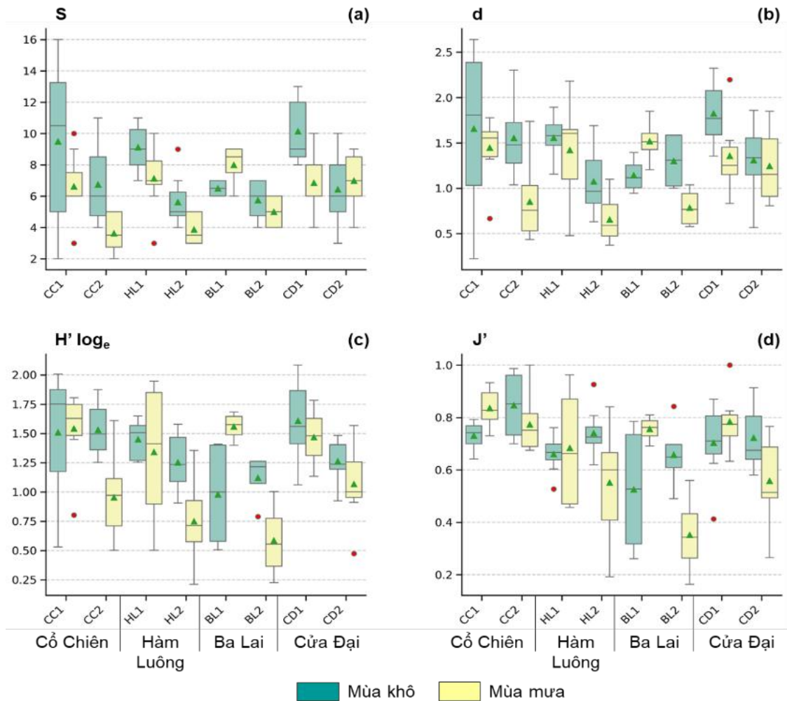
Hình 3.10. Các chỉ số đa dạng khu hệ tôm cửa sông Mê Kông ở các vị trí thu mẫu trong 2 mùa khảo sát. (Chú thích biểu đồ hộp: Chấm đỏ: Giá trị ngoại lệ, tam giác xanh lá: Giá trị trung bình, đường gạch ngang: Giá trị trung vị)
