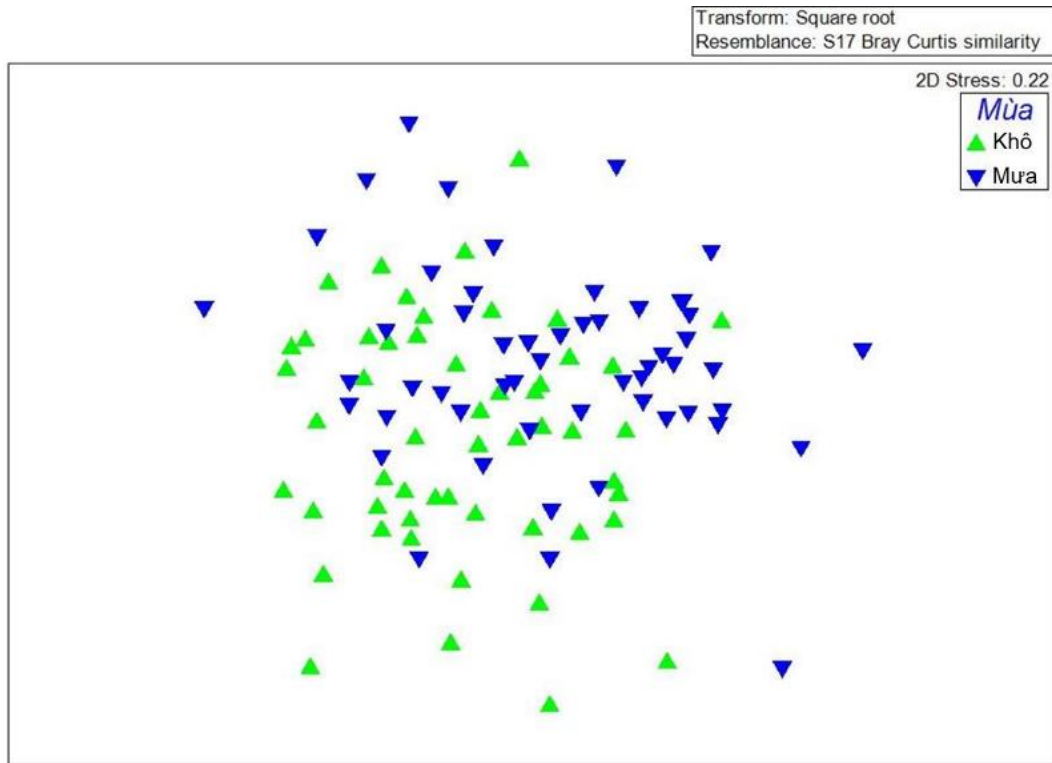
Phụ lục 3.8. Phân tích nMDS (Non-metric Multidimensional scaling) cấu trúc phân bố khu hệ tôm theo mùa khảo sát
