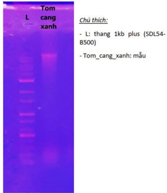
Phụ lục 3.1. Kết quả điện di mẫu DNA tôm càng xanh Mê Kông
