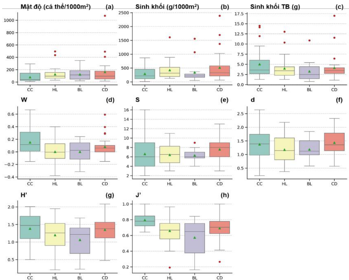
Hình 3.12. Các chỉ số sinh thái khu hệ tôm cửa sông Mê Kông phân bố theo cửa sông (Cỏ Chiên CC, Hàm Luông HL, Ba Lai BL, Cửa Đại CD). (Chú thích biểu đồ hộp: Chấm đỏ: Giá trị ngoại lệ, tam giác xanh lá: Giá trị trung bình, đường gạch ngang: Giá trị trung vị)
