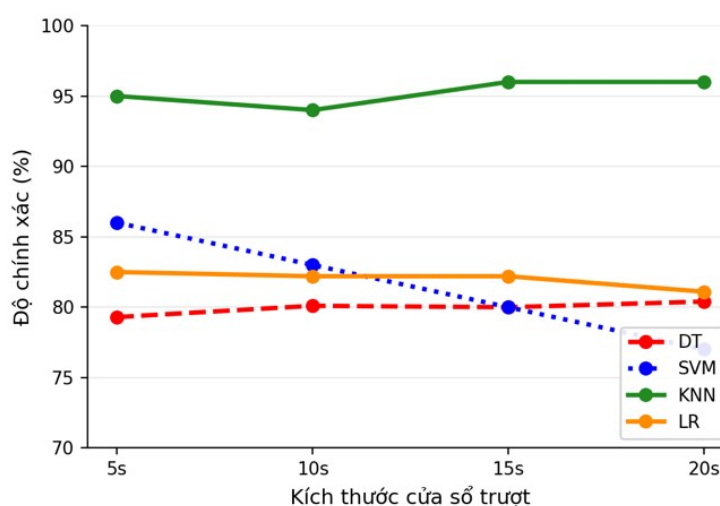
Hình 3.13 Độ chính xác của DT, SVM, KNN và LR trên tập dữ liệu công khai.
