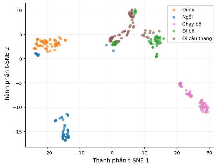
Hình 3.4. Tập dữ liệu WISDM được biểu diễn trong không gian 2 chiều: (a) không có các đặc trưng và (b) có các đặc trưng
