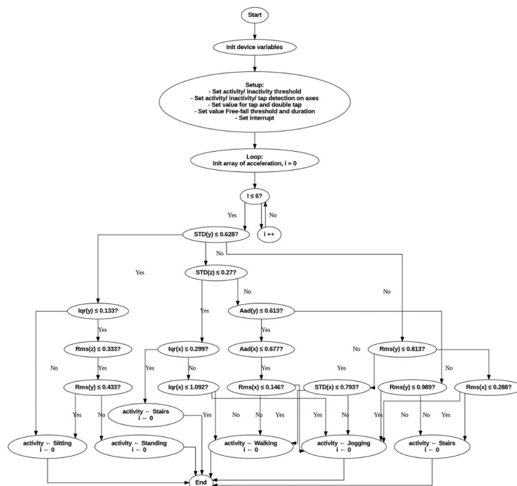
Hình 3.1 Chương trình nhúng để phân loại hoạt động thời gian thực
