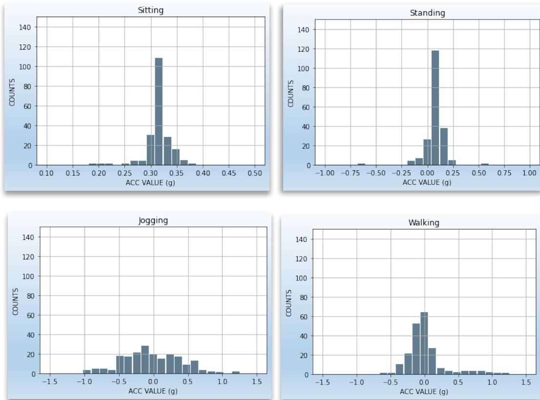
Hình 2.4 Phân phối dữ liệu gia tốc theo trục X của các hoạt động
