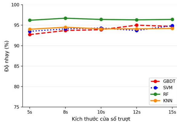
Hình 2.8 Độ nhạy của dữ liệu công khai
