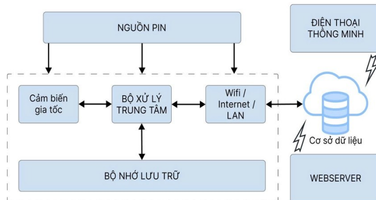
Hình 2.1 Sơ đồ khối của quá trình phân loại hoạt động
